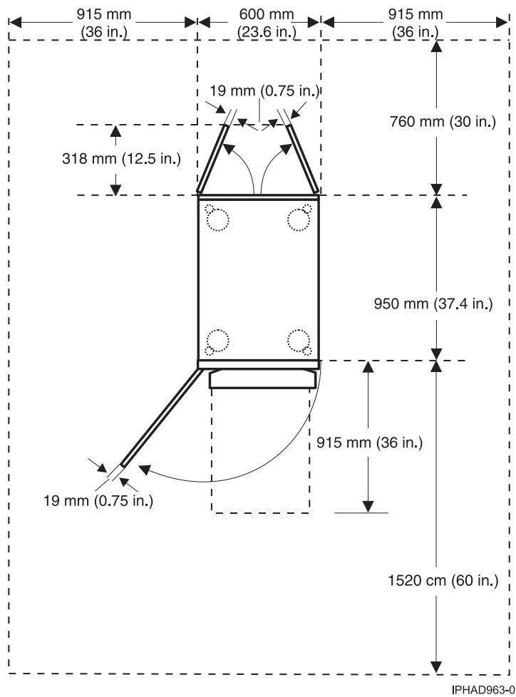
20. ábra: 0555 és 7014-S25 modell tervezési nézete
