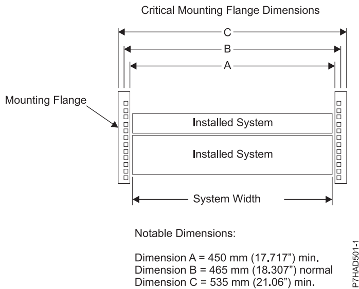
30. ábra: Kritikus beszerelési peremméreteket
