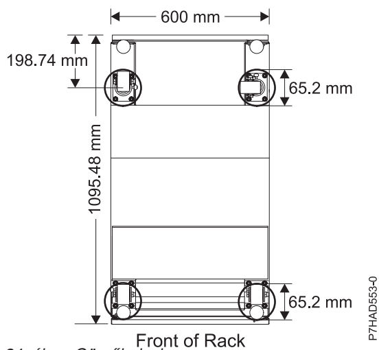
24. ábra: Görgőhelyek
