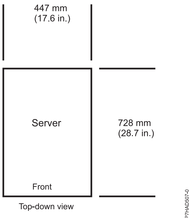
1. ábra: 8231-E2B, 8231-E1C, 8231-E1D, 8231-E2C, 8231-E2D, and 8268-E1D modell tervezési nézete (rackbe szerelt szerver)
