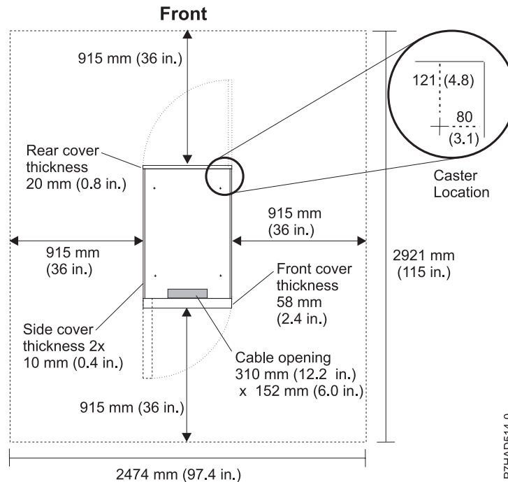
23. ábra: Szerviz térközök és görgőhelyek a 7014-T00, 7014-T42 és 0553 rack szekrény estén
