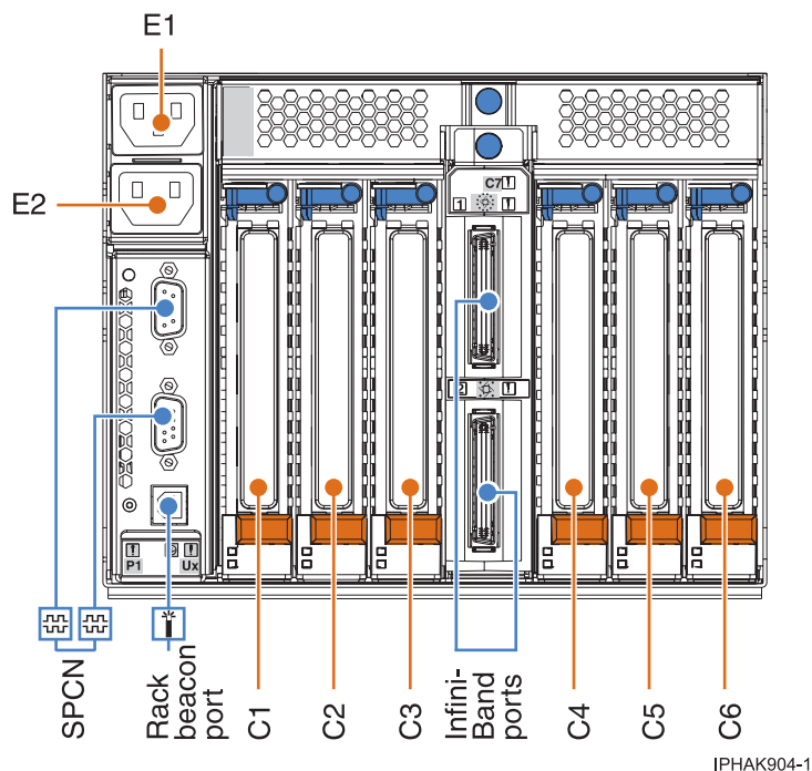
5. ábra: Hátulnézet
