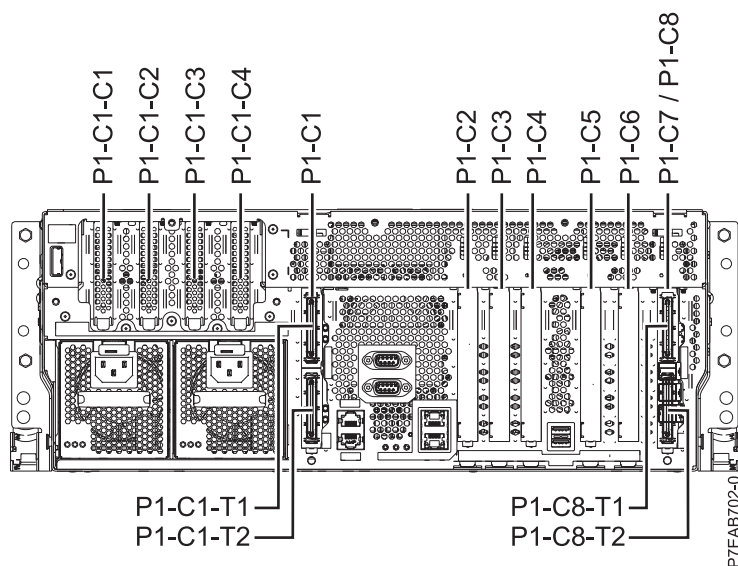
4. ábra: A rendszer hátulnézete a PCI bővítőhelyekkel és azok elhelyezési kódjaival
