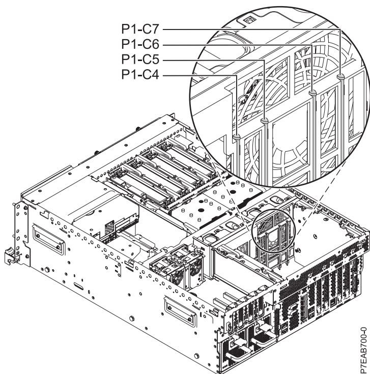
2. ábra: PCI bővítőhelyek elhelyezési kódja 8202-E4B és 8205-E6B rendszerekben
