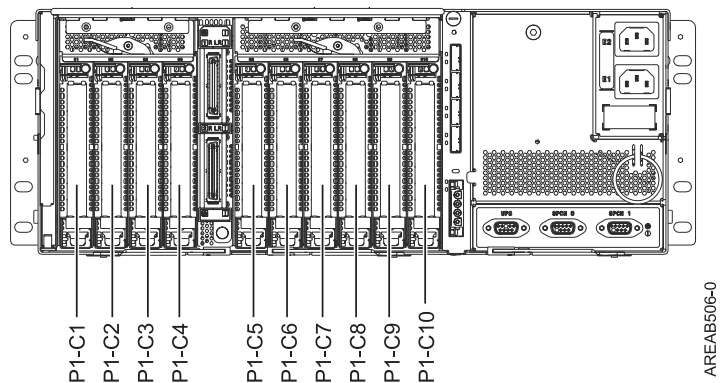
6. ábra: Hátlátnézet. Az ábra a bővítőegység hátlátnézetét mutatja.
