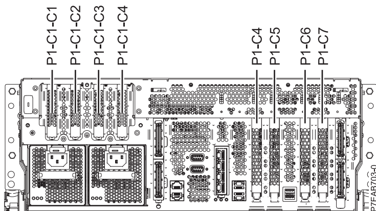
1. ábra: 8202-E4B és 8205-E6B rendszerek hátulnézete a PCI bővítőhelyek elhelyezési kódjaival
