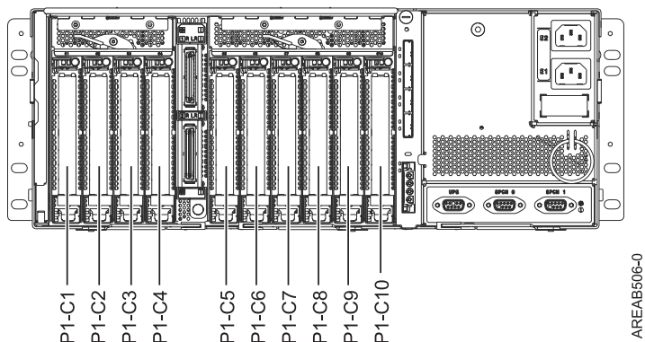
3. ábra: Hátlátnézet. Az ábra a bővítőegység hátlátnézetét mutatja.
