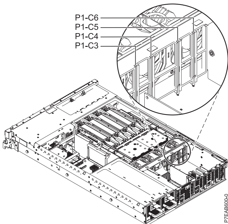
1. ábra: A 8231-E2B hátulnézete a PCI bővítőhelyek helykódjával.
