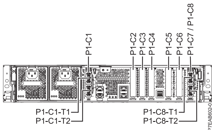
3. ábra: Rendszer hátulnézete az elhelyezési kódokkal
