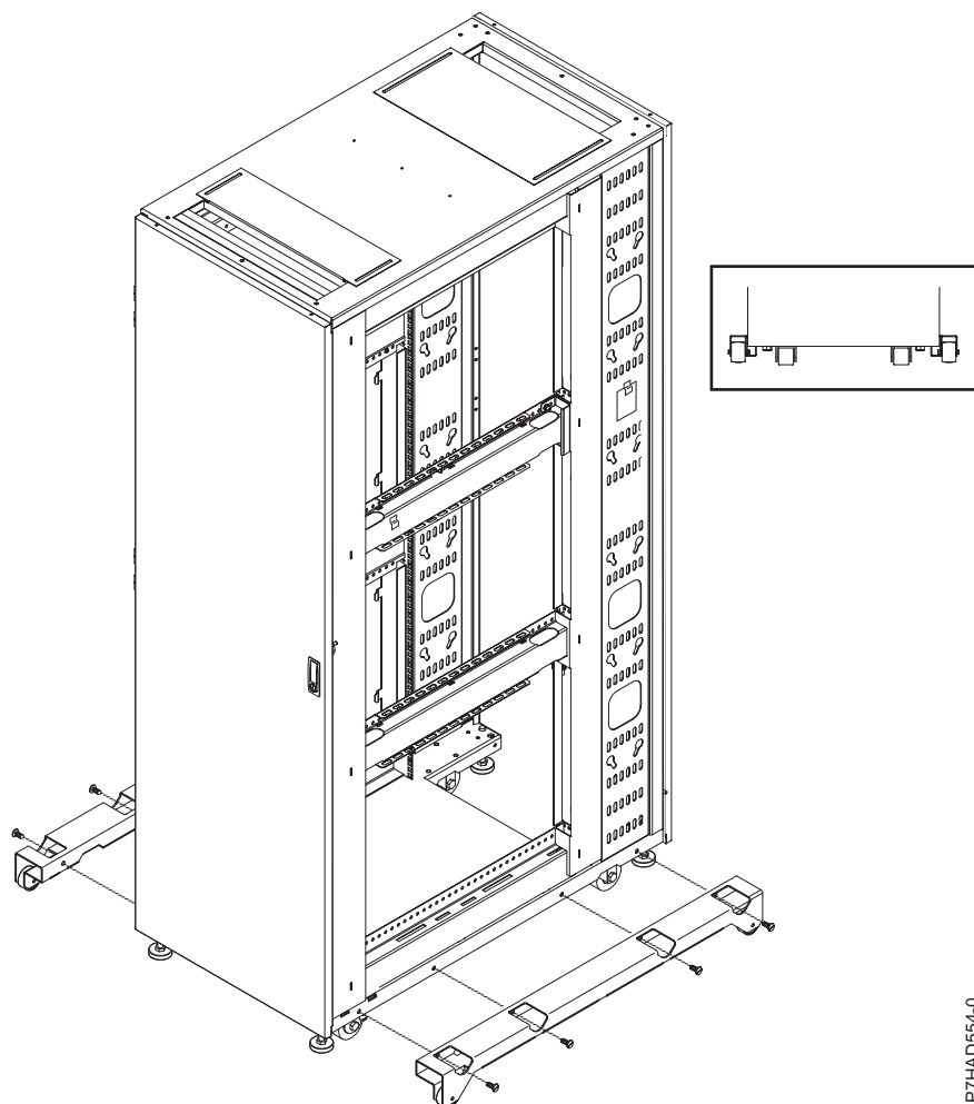
Slika 27. Lokacije držača
