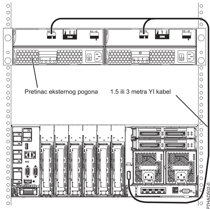
Slika 146. Sistemski eksterni SAS adaptorski port na pretinac disk proširenja (modeli 9117-MMB i 9179-MHB)
