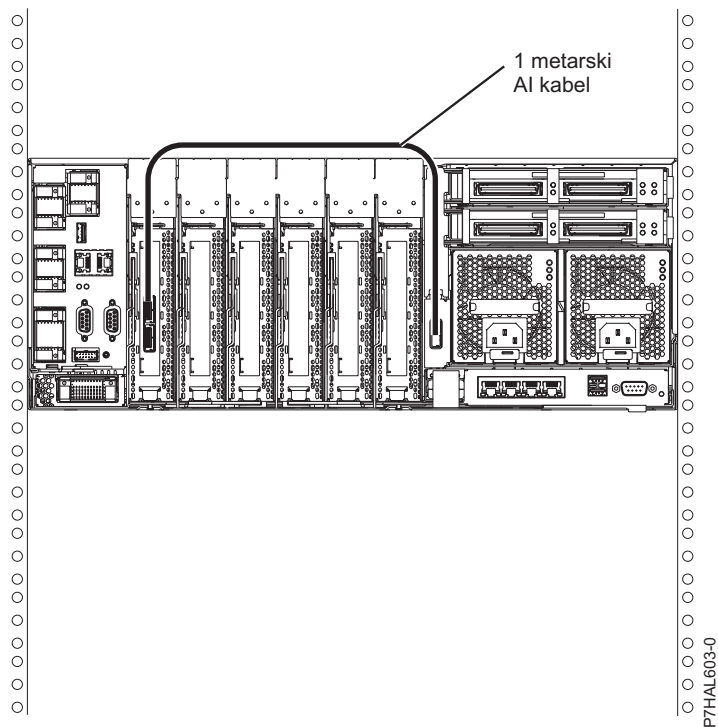
Slika 147. SAS adaptor do internih SAS disk priključnica preko sistemskih eksternih SAS portova
