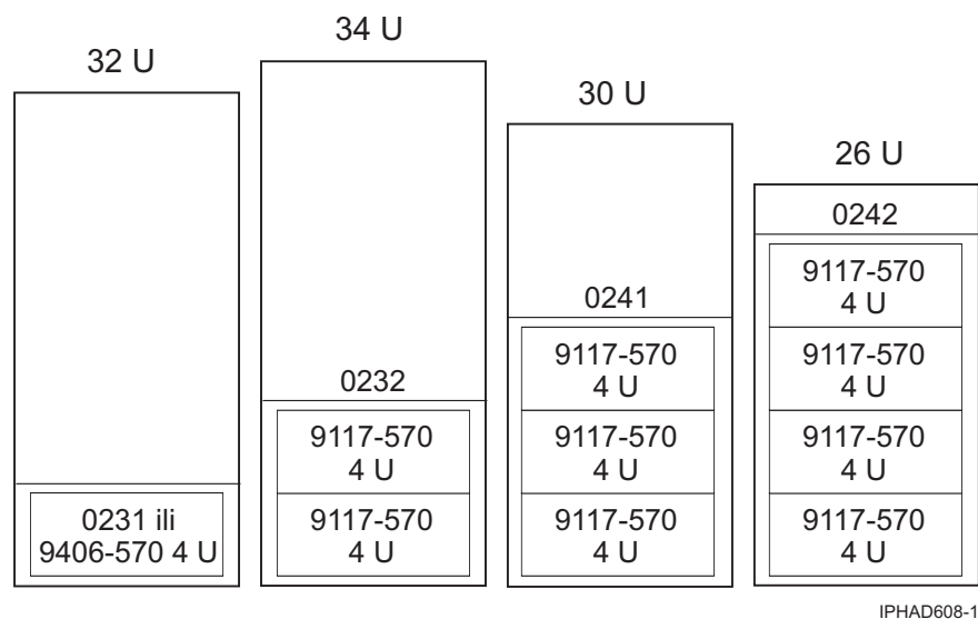
Slika 7. 570 u stalku
