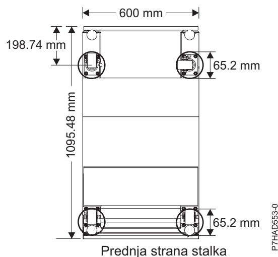
Slika 28. Lokacije kotačića
