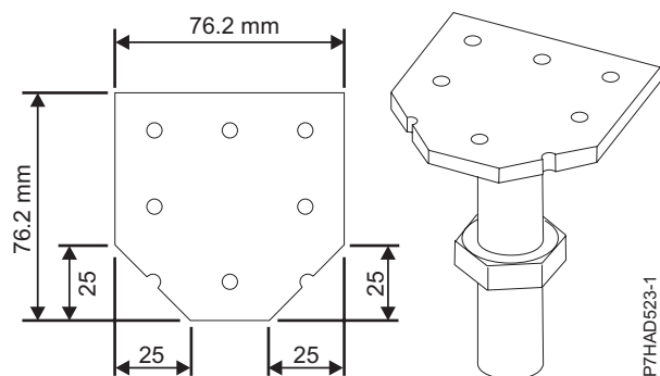
Slika 4. Dimenzije izrezanog postolja
