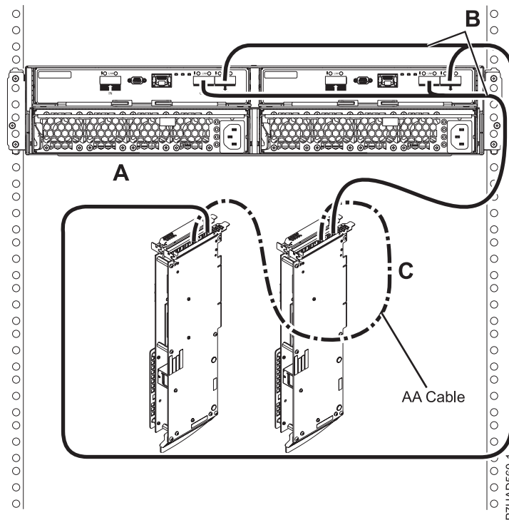
Slika 172. Povezivanje s načinom 1 za 5887 pretinac pomoću YO kablova na dva SAS adaptora
