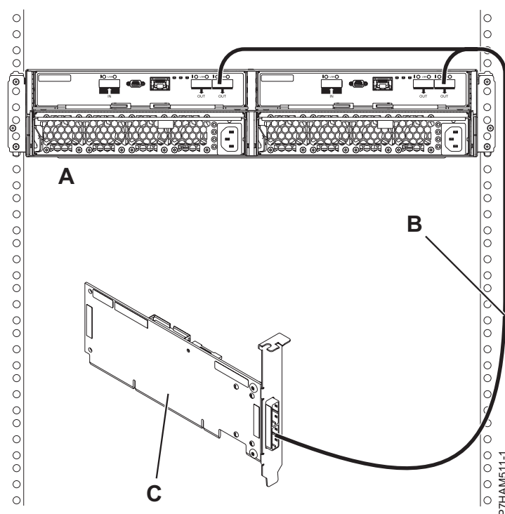
Slika 164. Način 1 povezivanje za 5887 pretinac s YO kablom na jedan SAS adaptor
