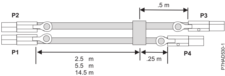
Slika 142. Dužine kablova sklopa SAS eksternih X kablova
