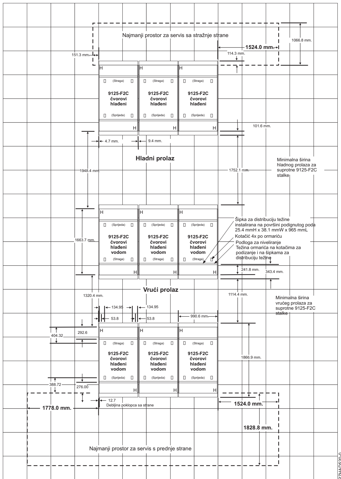
Slika 2. Prostor za servis za više stalaka - Vrući i hladni prolaz
