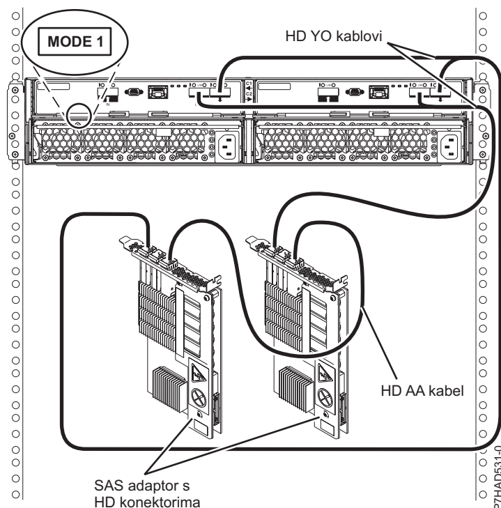
Slika 173. Način 1 povezivanje za 5887 pretinac na dva SAS adaptora s HD konektorima
