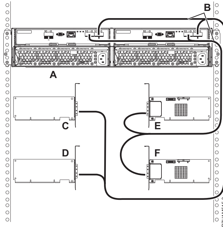
Slika 168. Povezivanje s načinom 4 za 5887 pretinac pomoću X kablova na četiri pojedinačna SAS adaptora
