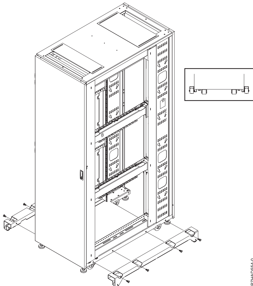
Slika 32. Lokacije držača
