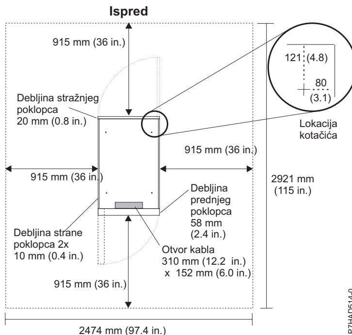
Slika 27. Servisni razmaci i lokacije kotačića za 7014-T00, 7014-T42 i 0553 stalke
