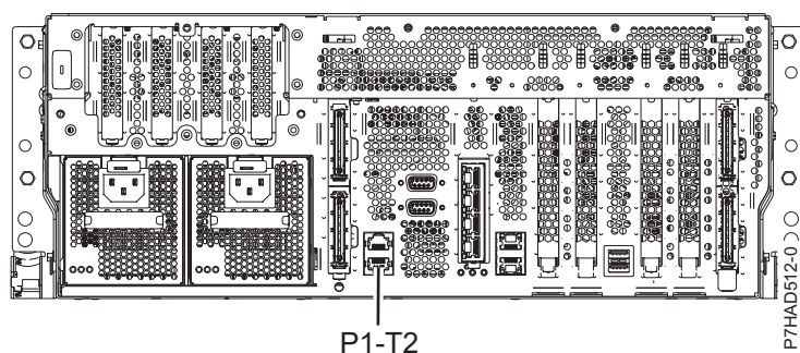
Slika 137. 8202-E4B, 8202-E4C, 8202-E4D, 8205-E6B, 8205-E6C i 8205-E6D pogled straga s lokacijama za instalaciju kablova
