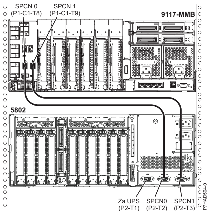
Slika 135. 8412-EAD, 9117-MMB, 9117-MMC, 9117-MMD, 9179-MHB, 9179-MHC, 9179-MHD i 5208 ili 5877 pogled straga na lokaciju instalacije kablova
