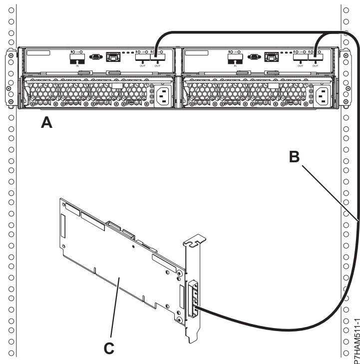
Slika 171. Način 1 povezivanje za 5887 pretinac s YO kablom na jedan SAS adaptor
