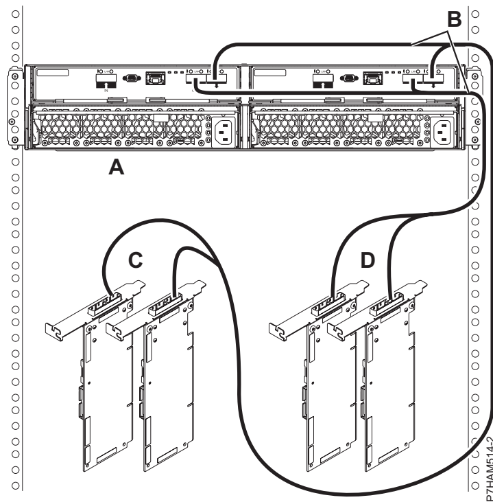
Slika 167. Način 2 povezivanje za 5887 pretinac s X kablovima na dva para SAS adaptora
