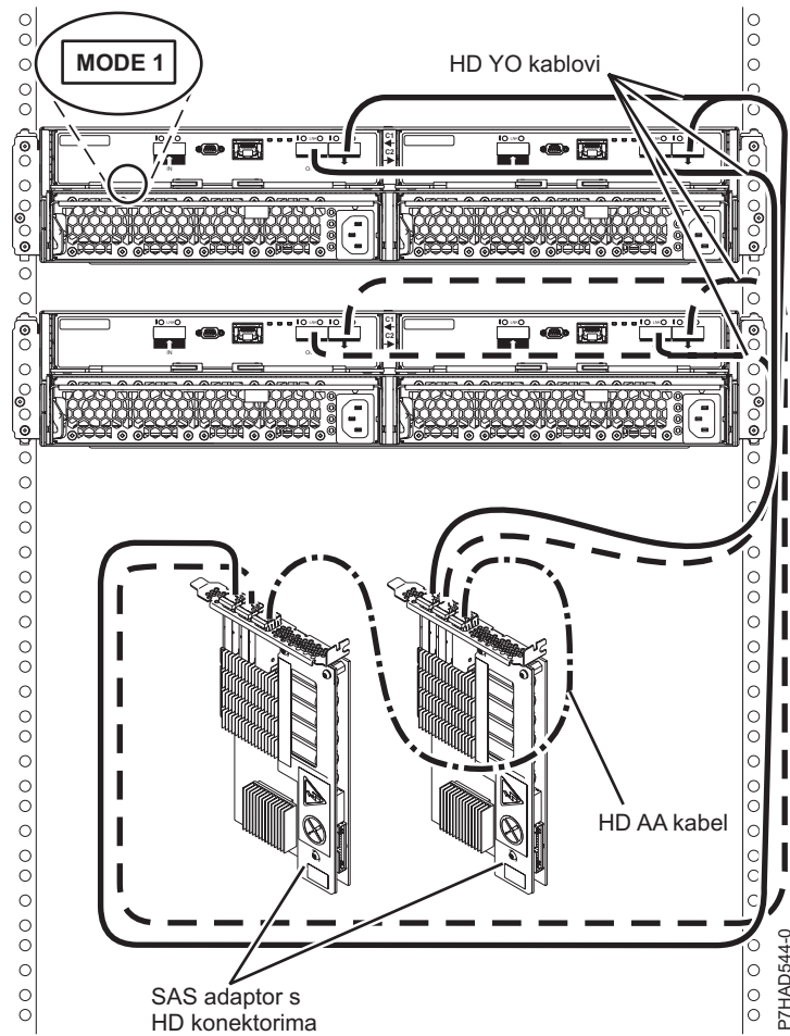
Slika 174. Povezivanje s načinom 1 za dva 5887 pretinca s HD konektorima na dva SAS adaptera
