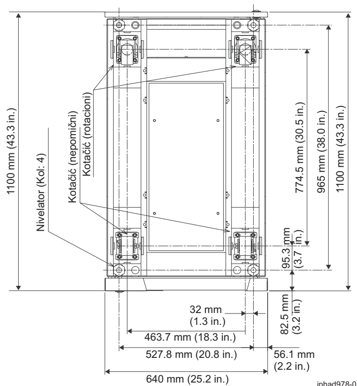
Slika 26. Lokacije kotačića i nivelatora
