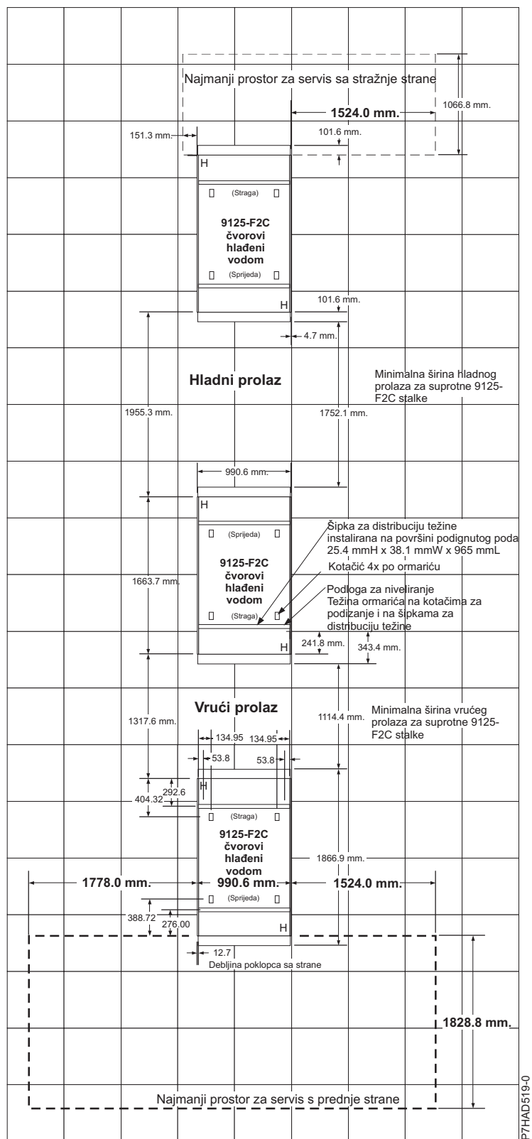
Slika 1. Prostor za servis za jedan stalak - Vrući i hladni prolaz
