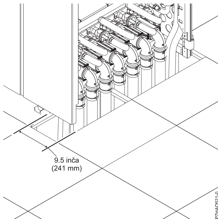
Slika 3. Otvor na podu
