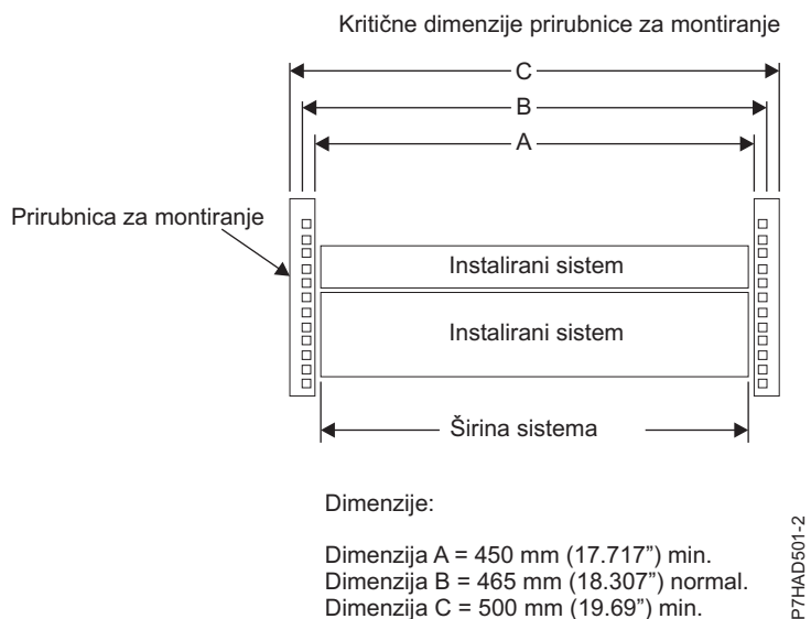
Slika 34. Kritične dimenzije prirubnice za montiranje
