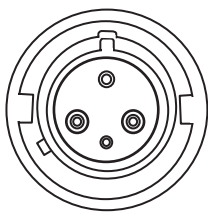
Slika 53. Utičnica tipa IEC 60309 2P+E
