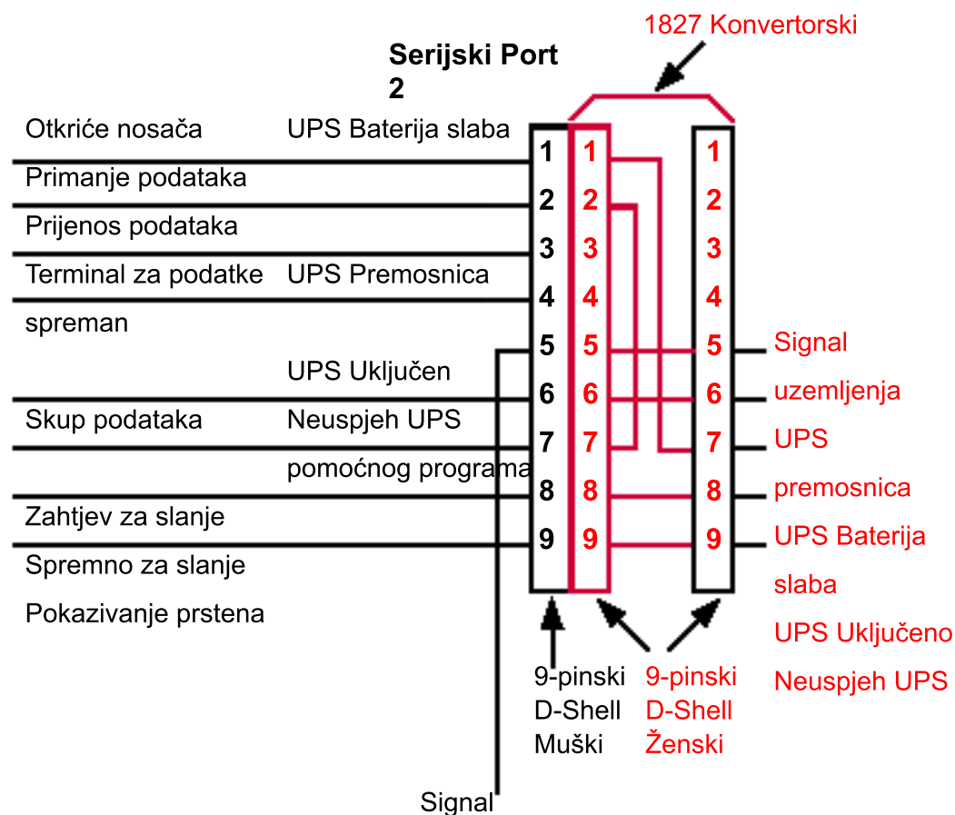
Slika 128. 1827 ožičenje
