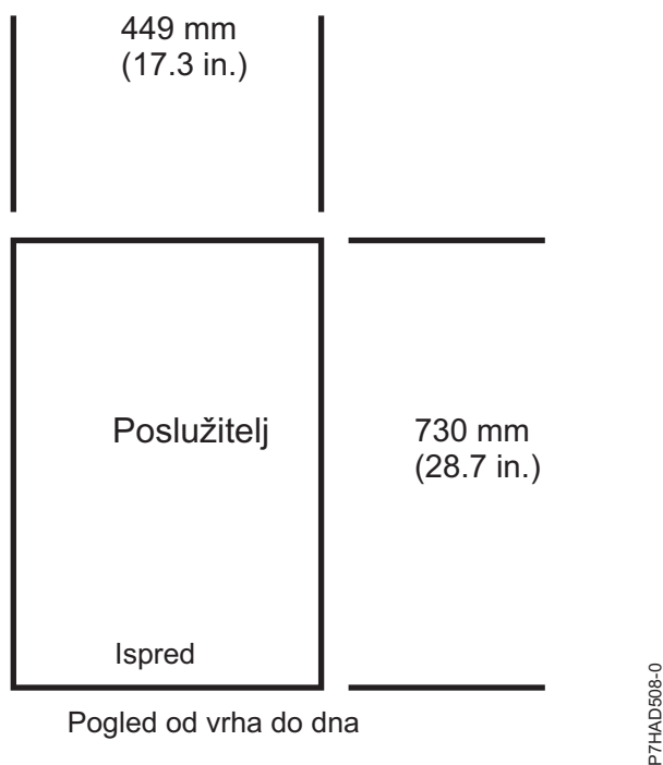
Slika 1. Model 8202-E4B, 8202-E4C, 8202-E4D, 8205-E6B, 8205-E6C i 8205-E6D pogled na plan (poslužitelji montirani u stalak)
