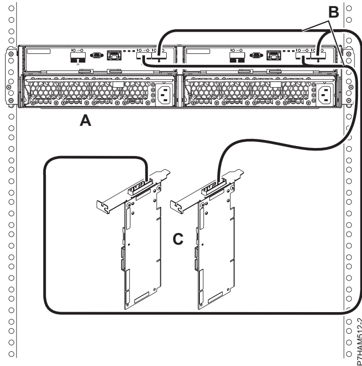
Slika 165. Povezivanje s načinom 1 za 5887 pretinac pomoću YO kablova na dva SAS adaptora
