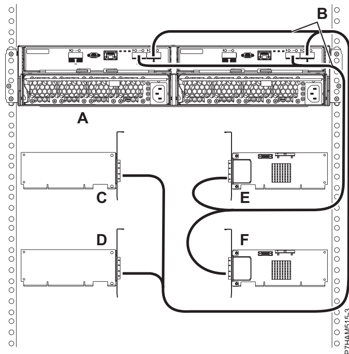
Slika 164. Povezivanje s načinom 4 za 5887 pretinac pomoću X kablova na četiri pojedinačna SAS adaptora
