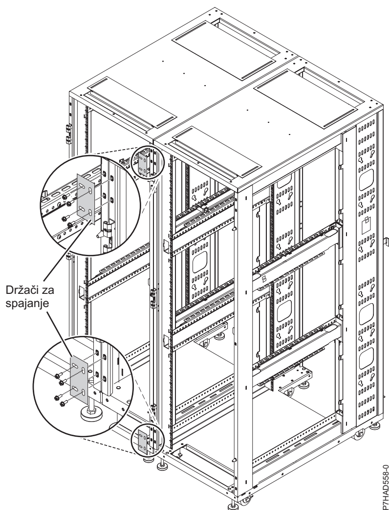
Slika 29. Držači za spajanje
