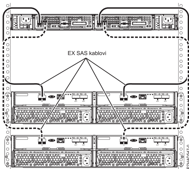
Slika 174. Povezivanje dva 5887 pretinca pomoću HD EX kablova na jedan EDR1
