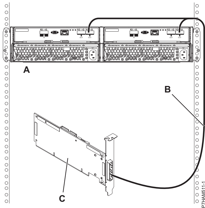
Slika 167. Način 1 povezivanje za 5887 pretinac s YO kablom na jedan SAS adaptor
