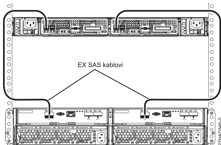
Slika 173. Povezivanje jednog 5887 pretinca pomoću HD EX kablova na jedan EDR1
