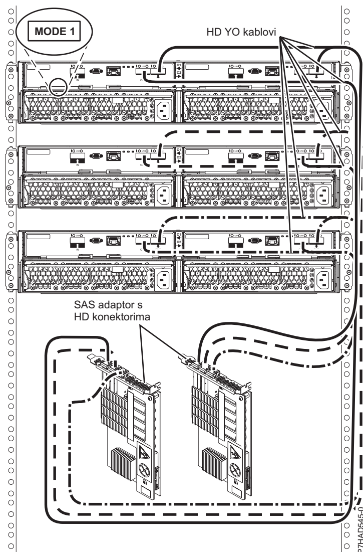
Slika 171. Način 1 povezivanje za tri 5887 pretinca na dva SAS adaptora s HD konektorima
