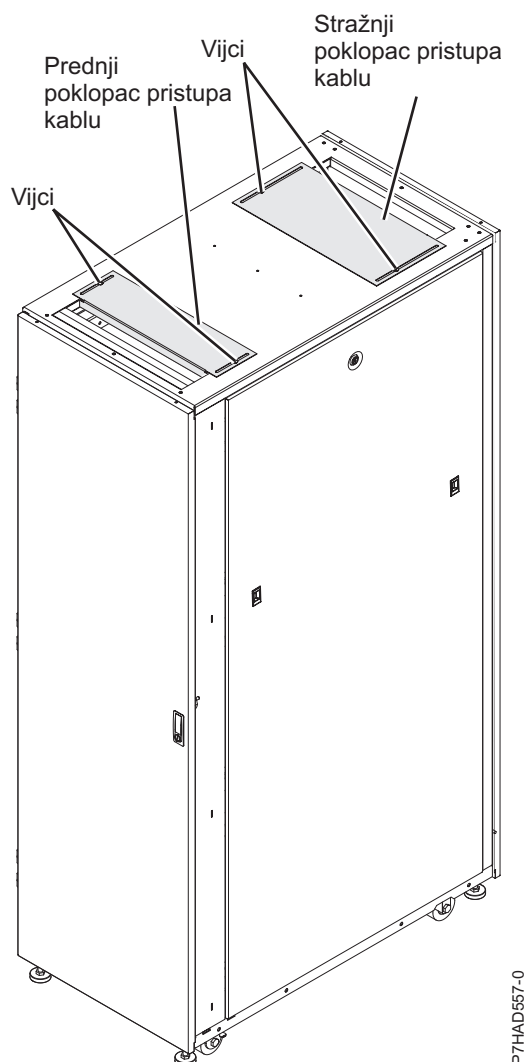
Slika 27. Poklopci pristupa kablovima
