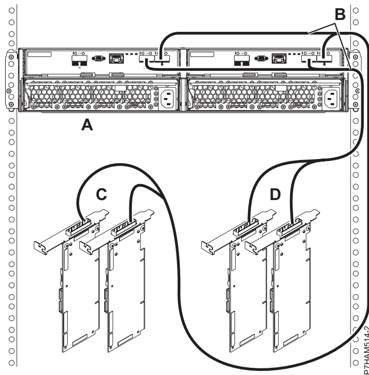
Slika 163. Način 2 povezivanje za 5887 pretinac s X kablovima na dva para SAS adaptora
