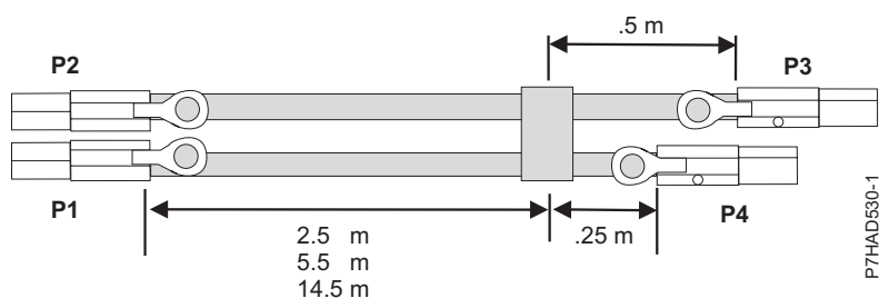
Slika 138. Dužine kablova sklopa SAS eksternih X kablova
