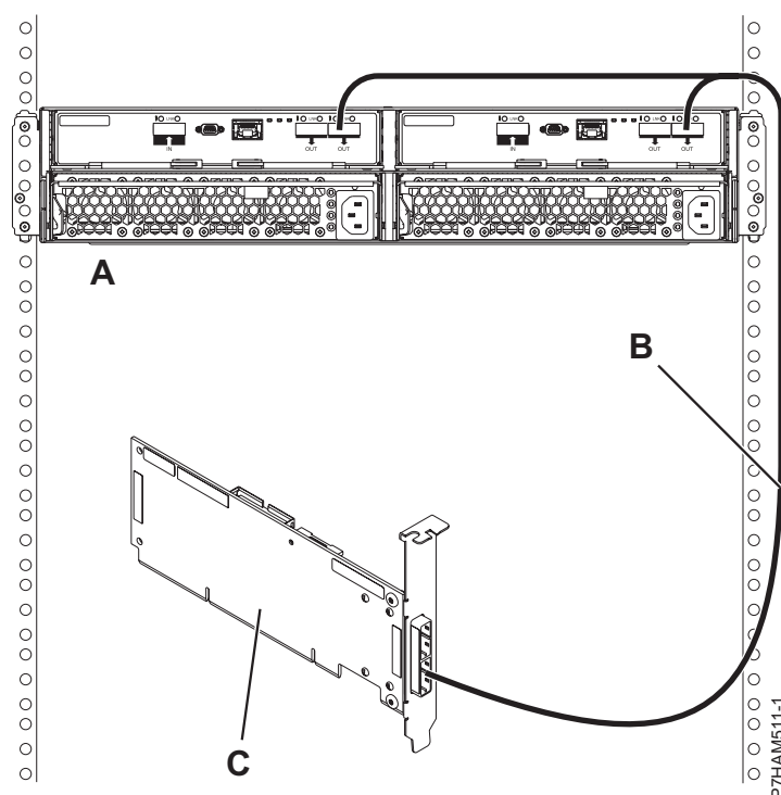
Slika 160. Način 1 povezivanje za 5887 pretinac s YO kablom na jedan SAS adaptor
