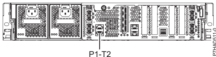
Slika 132. 8231-E2B, 8231-E1C, 8231-E1D, 8231-E2C, 8231-E2D i 8268-E1D pogled straga na lokacije instalacije kablova
