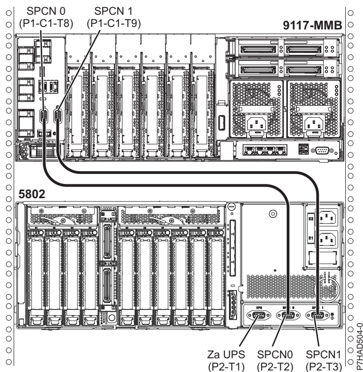
Slika 131. 8412-EAD, 9117-MMB, 9117-MMC, 9117-MMD, 9179-MHB, 9179-MHC, 9179-MHD i 5208 ili 5877 pogled straga na lokaciju instalacije kablova
