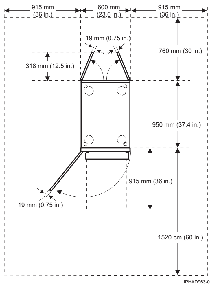
Slika 20. Planski pogled na model 0555 i 7014-S25
