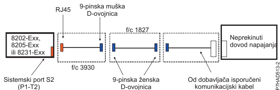
Slika 134. Kabliranje neprekinutog dovoda napajanja za 8202-E4B, 8202-E4C, 8205-E6B, 8205-E6C, 8231-E2B, 8231-E1C, 8231-E1D, 8231-E2C, 8231-E2D i 8268-E1D
