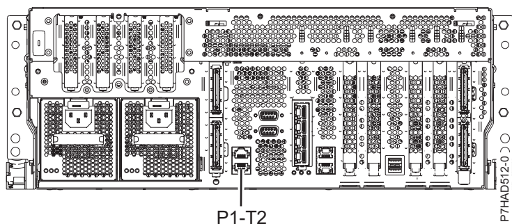
Slika 133. 8202-E4B, 8202-E4C, 8202-E4D, 8205-E6B, 8205-E6C i 8205-E6D pogled straga s lokacijama za instalaciju kablova
