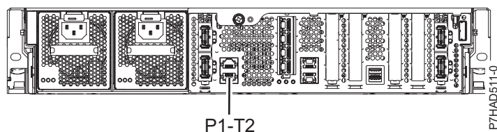
Slika 132. 8231-E2B, 8231-E1C, 8231-E1D, 8231-E2C, 8231-E2D i 8268-E1D pogled straga na lokacije instalacije kablova
