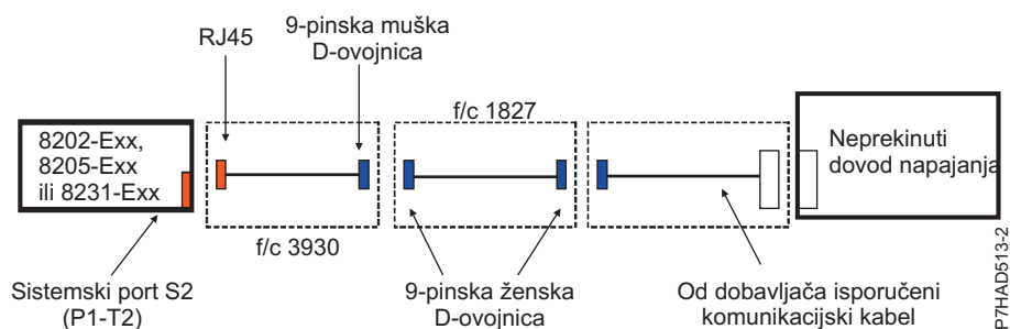
Slika 134. Kabliranje neprekinutog dovoda napajanja za 8202-E4B, 8202-E4C, 8205-E6B, 8205-E6C, 8231-E2B, 8231-E1C, 8231-E1D, 8231-E2C, 8231-E2D i 8268-E1D
