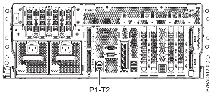
Slika 133. 8202-E4B, 8202-E4C, 8202-E4D, 8205-E6B, 8205-E6C i 8205-E6D pogled straga s lokacijama za instalaciju kablova
