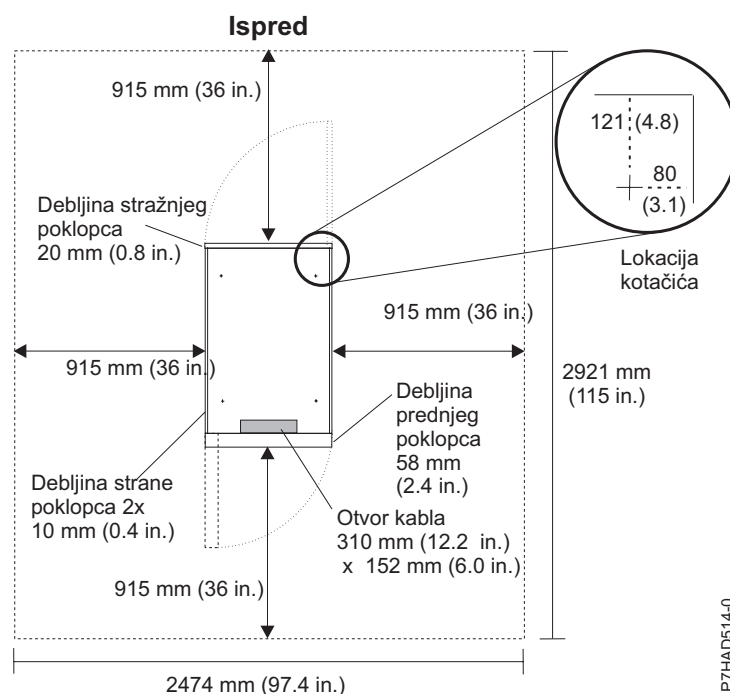
Slika 23. Servisni razmaci i lokacije kotačića za 7014-T00, 7014-T42 i 0553 stalke
