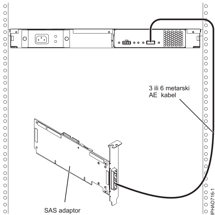
Slika 145. SAS adaptor na pretnac proširenja medija
