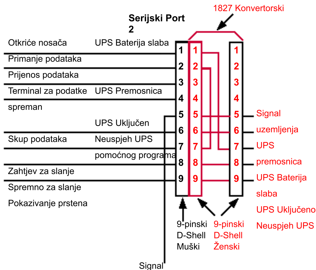
Slika 128. 1827 ožičenje
