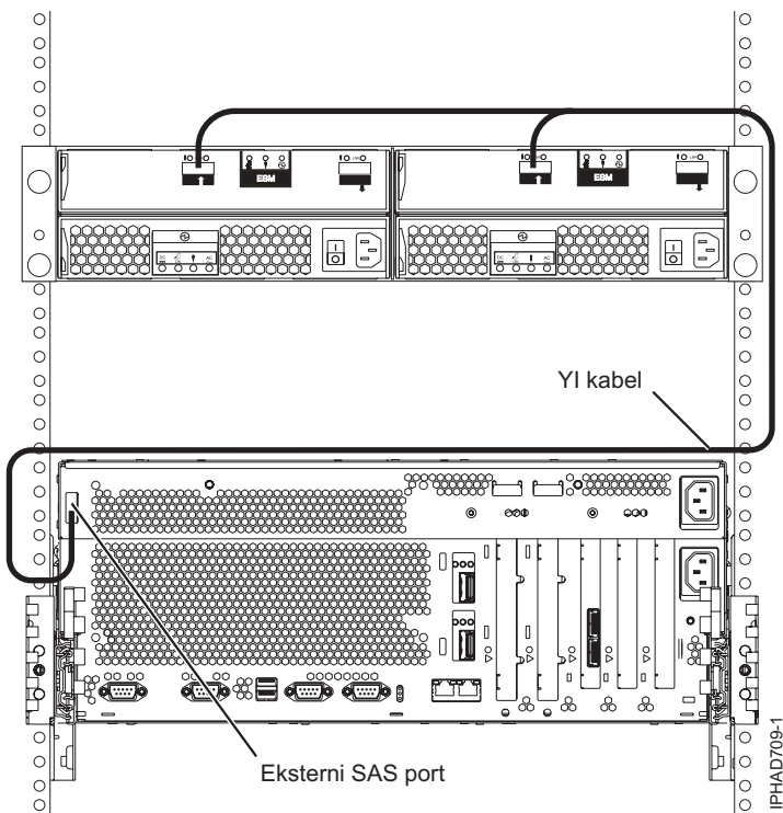
Slika 147. Sistemski eksterni port SAS adaptera na prečinac proširenja diska
