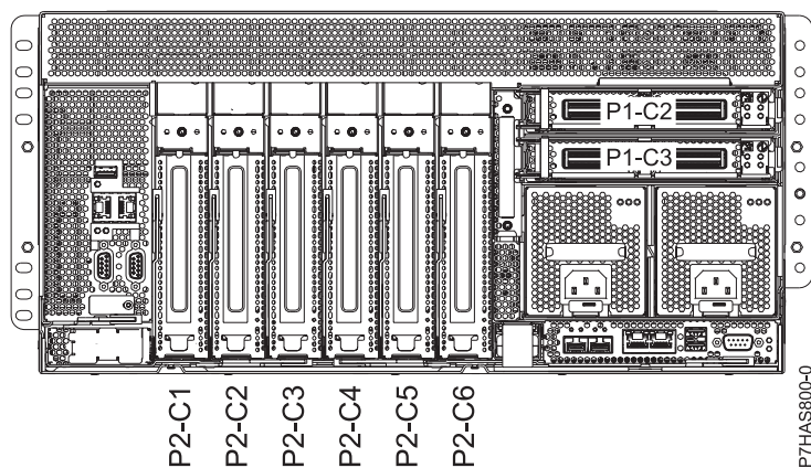
Slika 1. Pogled straga na sistem sa šiframa lokacija
