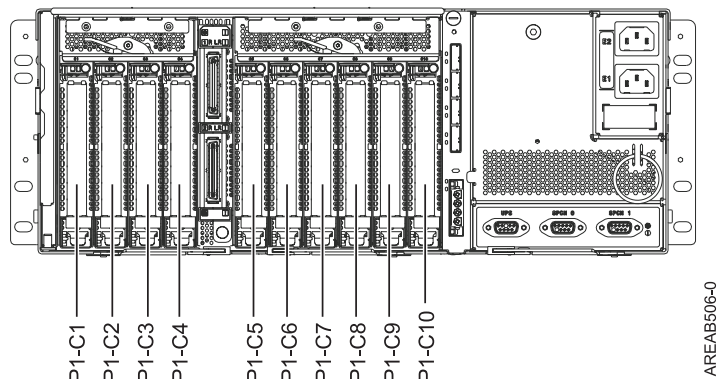
Slika 2. Pogled straga. Ova slika prikazuje stražnji pogled na jedinicu proširenja.
