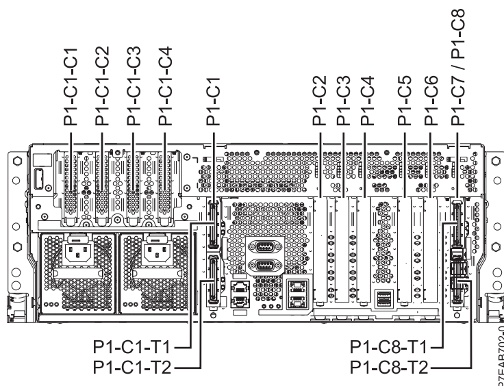
Slika 4. Pogled straga na sistem na kojem se vide PCI priključnice i šifre njihovih lokacija
