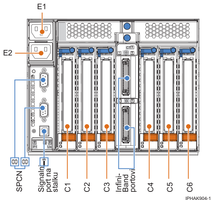
Slika 5. Pogled straga
