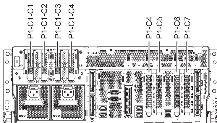
Slika 1. Pogled straga na 8202-E4B i 8205-E6B sisteme sa šiframa lokacija PCI priključnica
