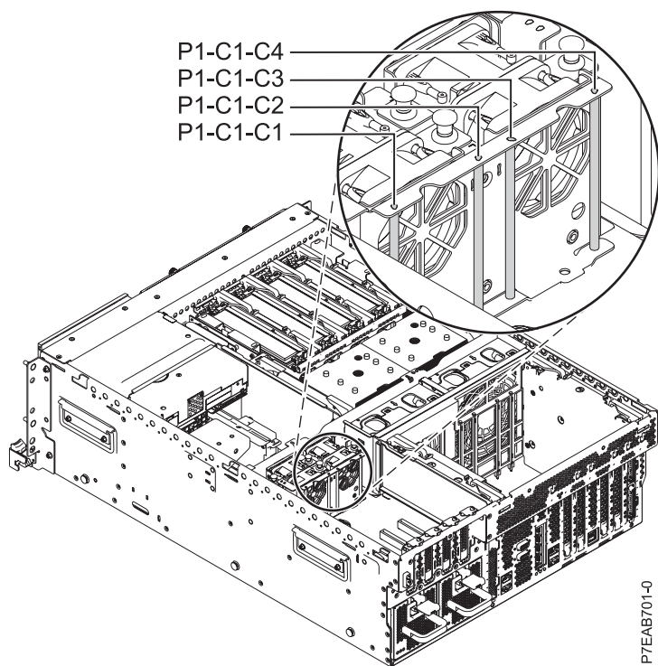
Slika 3. Proširenje PCI podizača sa šiframa lokacija na 8202-E4B i 8205-E6B sistemima
