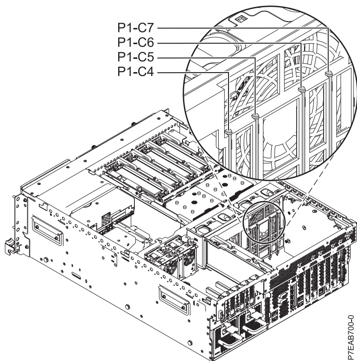
Slika 2. Šifre lokacija PCI priključnica na 8202-E4B i 8205-E6B sistemima
