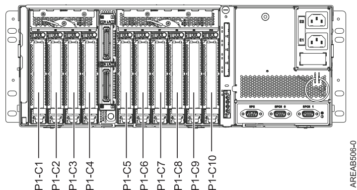
Slika 6. Pogled straga. Ova slika prikazuje stražnji pogled na jedinicu proširenja.
