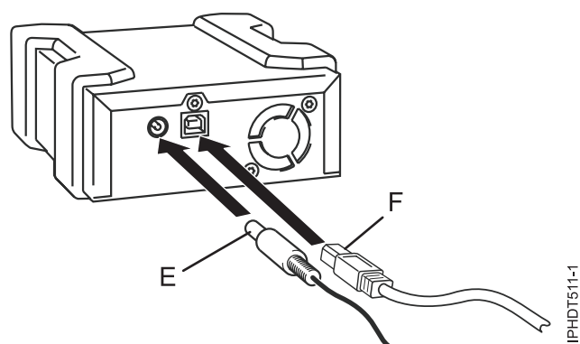
Figure 13. Unité externe, vue arrière et connecteurs
