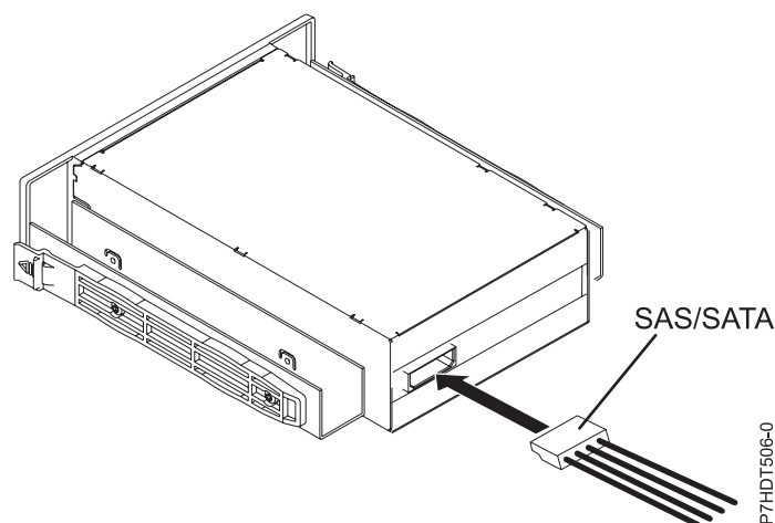
Figure 15. Unité interne, vue arrière et connecteur
