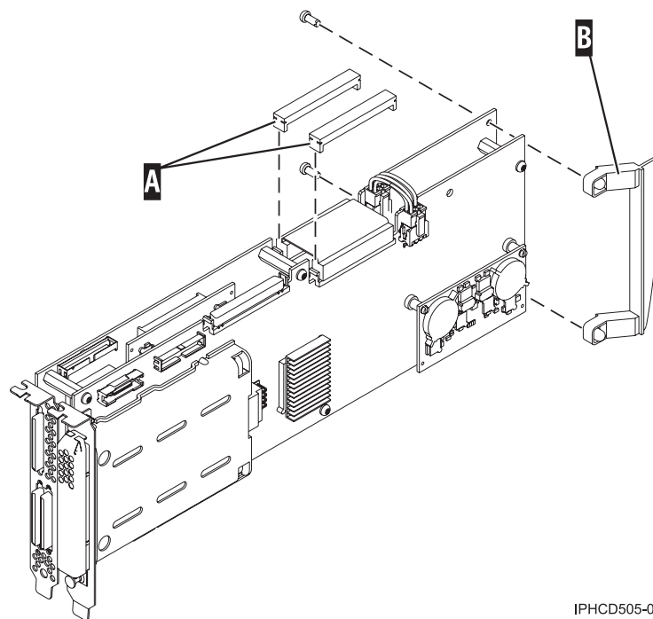
Figure 59. Préparation de la carte pour être placée dans une cassette
