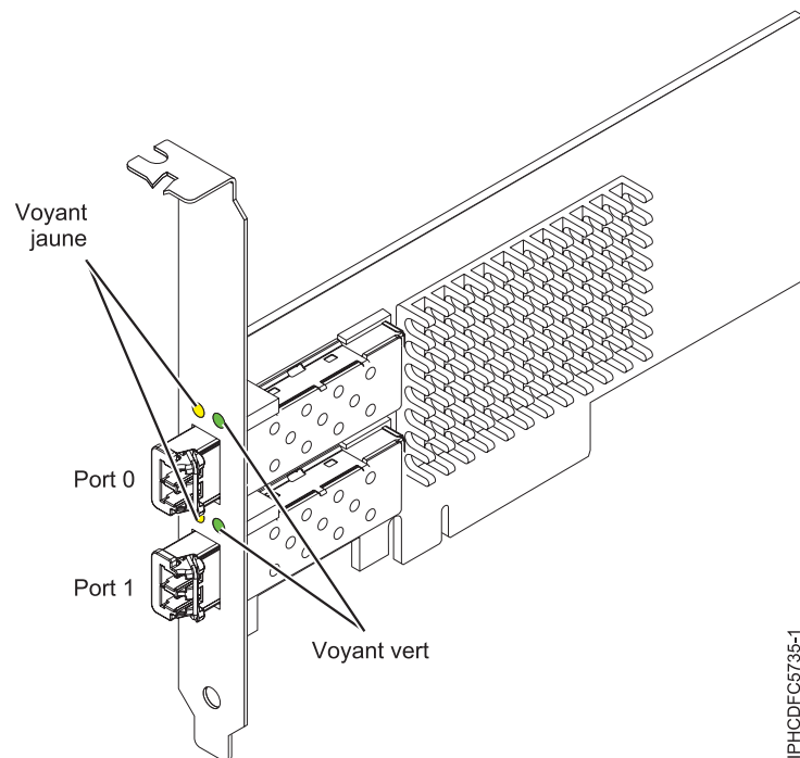
Figure 8. Carte 5735
