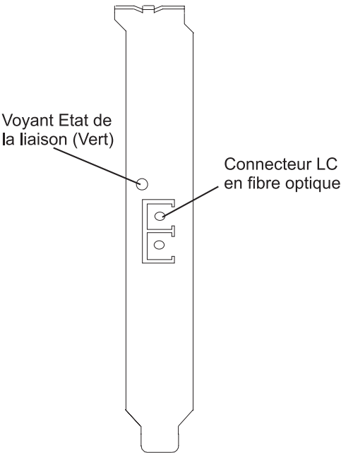
Figure 25. Voyant de la carte PCI-X TOE iSCSI SX 1 Gbit
