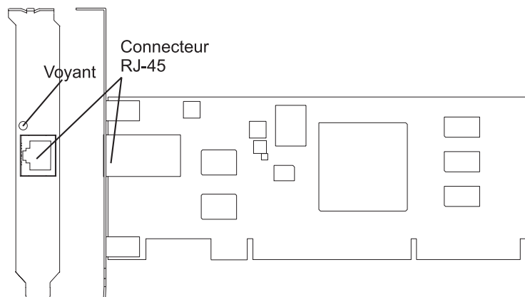
Figure 24. Carte PCI-X TOE iSCSI TX 1 Gbit
