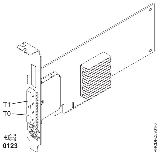
Figure 43. Carte PCIe SAS double accès x4
