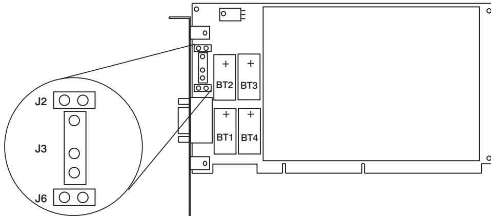
Figure 40. Remplacement des piles du coprocesseur
