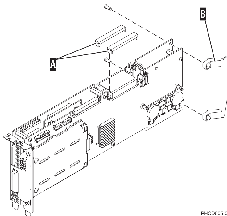
Figure 57. Préparation de la carte pour être placée dans une cassette
