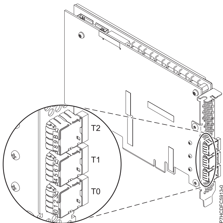
Figure 49. Carte 5913
