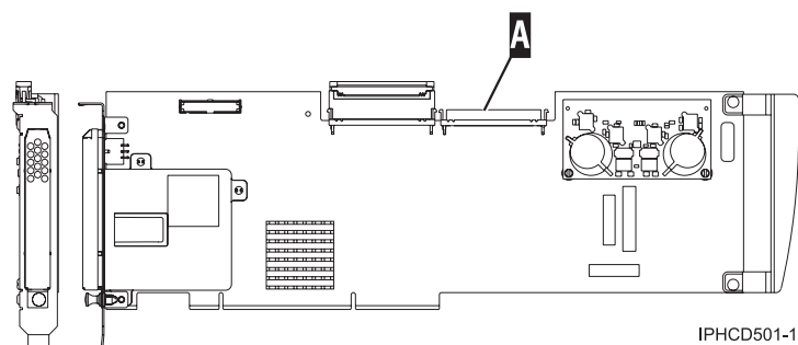
Figure 52. Carte d'entrée-sortie de cache d'écriture auxiliaire
