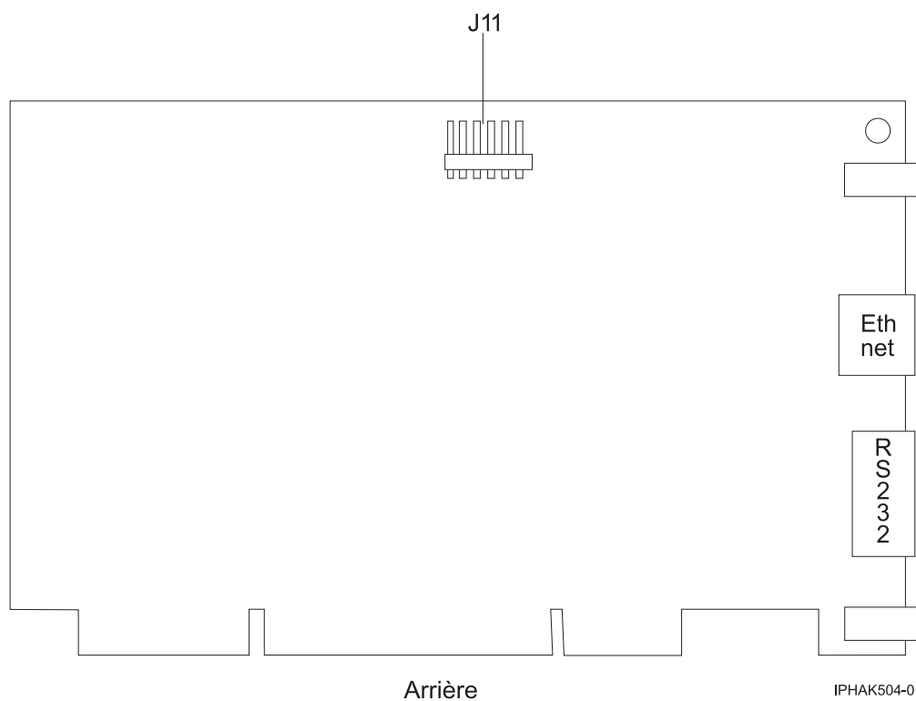
Figure 39. Verso de l'adaptateur
