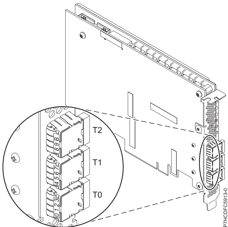
Figure 50. Carte ESA3
