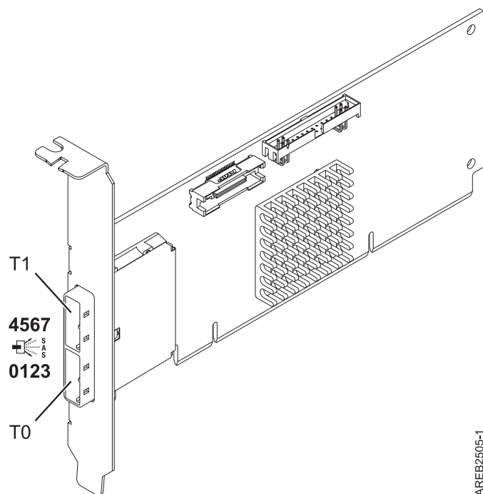
Figure 42. Carte SAS PCI-X DDR externe double accès – x4
