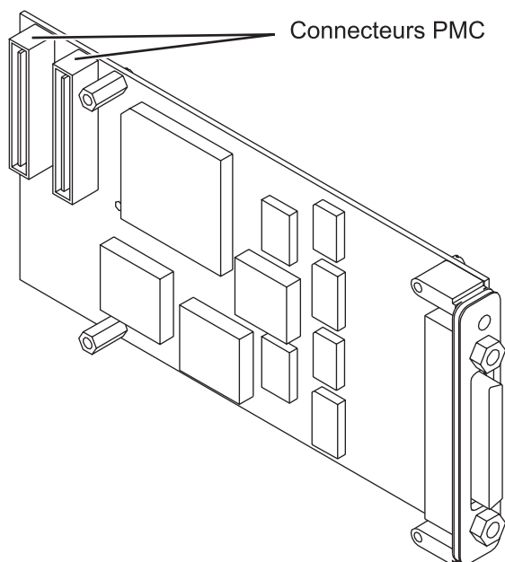
Figure 61. Carte PMC 4 ports sélectionnables
