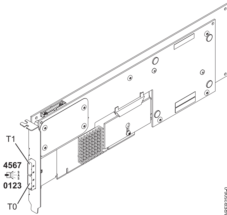
Figure 44. carte SAS RAID PCI-X DDR double accès –x4
