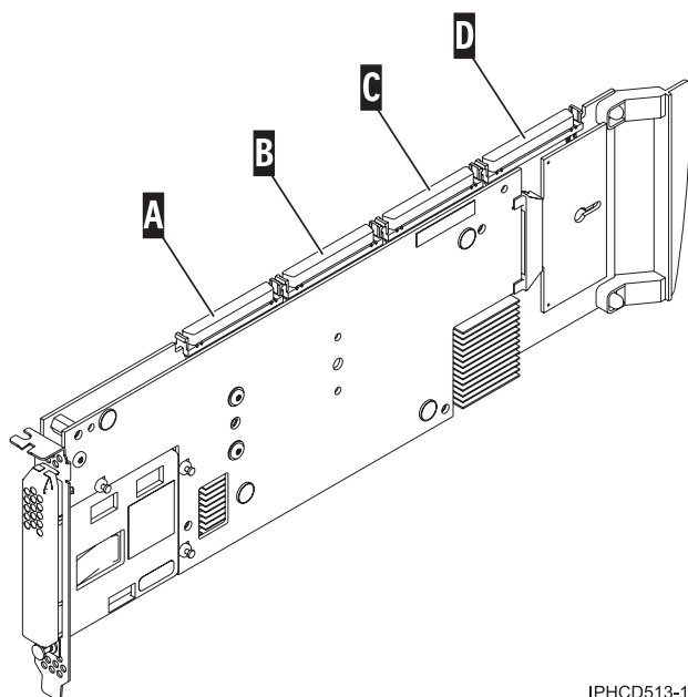
Figure 55. Connecteurs SCSI de la carte
