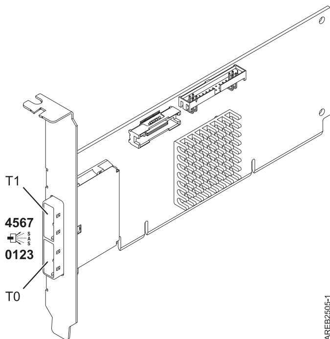
Figure 48. Carte SAS PCI-X DDR externe double accès – x4
