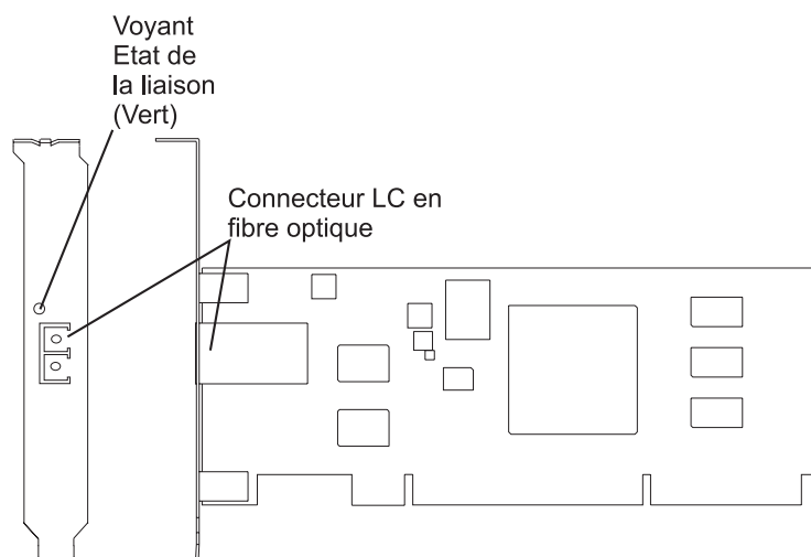
Figure 23. Carte PCI-X TOE iSCSI SX 1 Gbit
