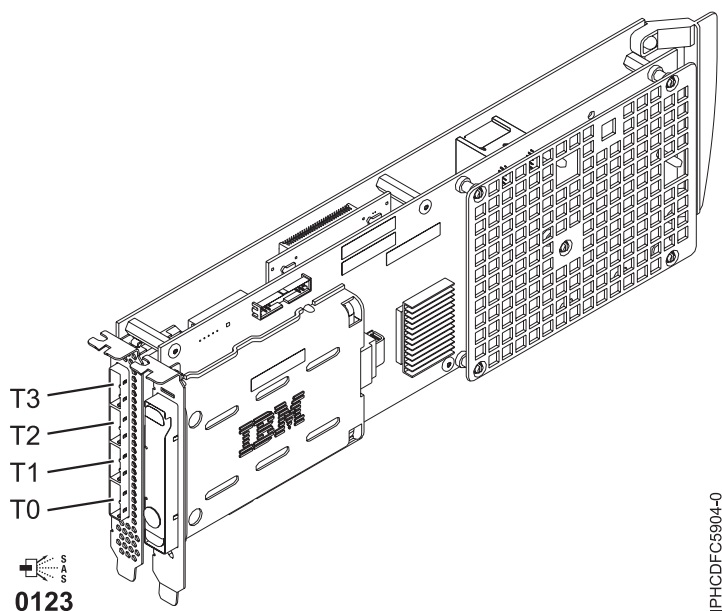
Figure 47. Carte SAS RAID PCI-X DDR 1,5 Go de cache
