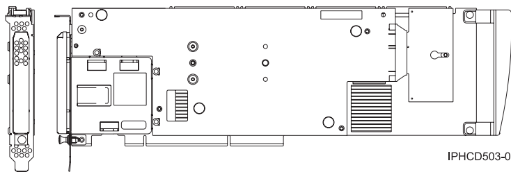
Figure 68. Vue latérale et vue d'extrémité de la carte
