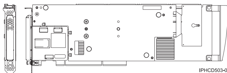
Figure 72. Vue latérale et vue d'extrémité de la carte
