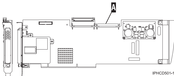
Figure 70. Carte d'entrée-sortie de cache d'écriture auxiliaire
