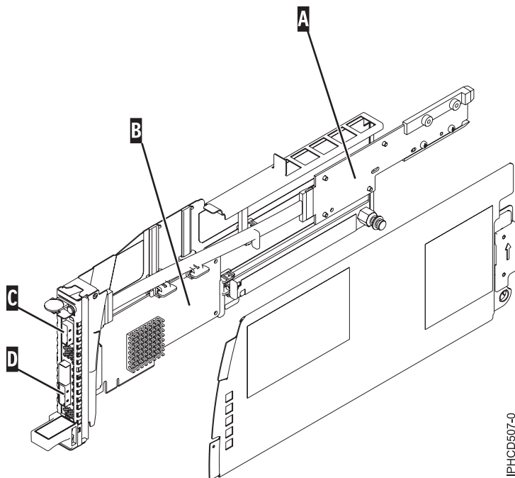
Figure 61. Carte SAS PCI Express x8 externe double accès -x4 3 Go et carte câble dans une cassette
