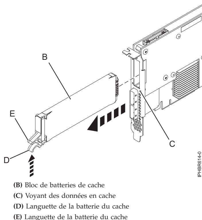
Figure 85. Remplacement de la batterie du cache d'une carte 574E
