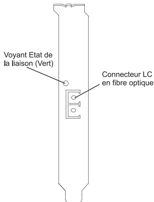
Figure 29. Voyant de la carte PCI-X TOE iSCSI SX 1 Gbit
