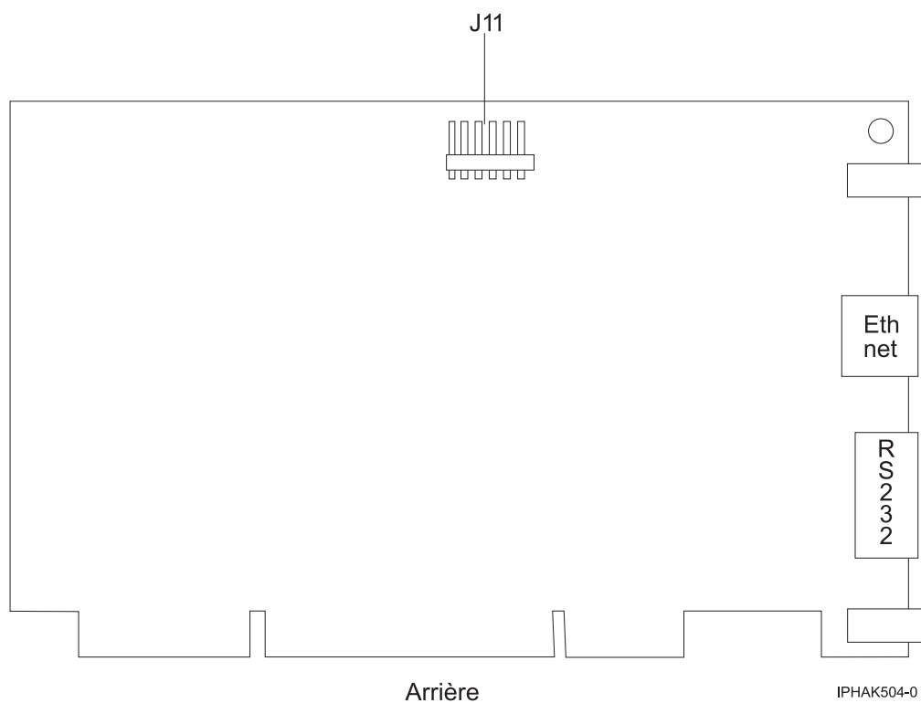
Figure 52. Verso de l'adaptateur
