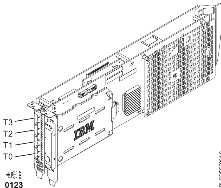
Figure 60. Carte SAS RAID PCI-X DDR 1,5 Go de cache
