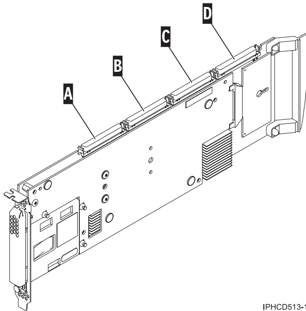
Figure 73. Connecteurs SCSI de la carte
