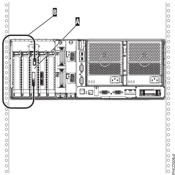
Figure 62. Vue arrière de l'unité centrale sur laquelle le dispositif 5909 est installé et câblé
