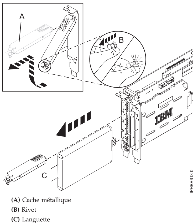
Figure 82. Remplacement de la batterie du cache d'une carte 572F/575C
