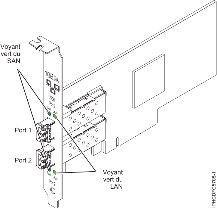
Figure 30. carte double port PCIe FCoE 10 Gb
