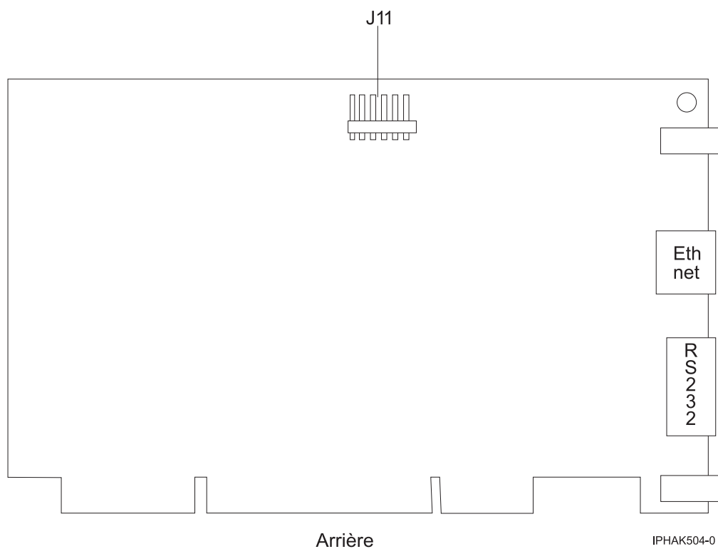
Figure 48. Verso de l'adaptateur
