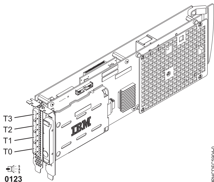
Figure 17. Carte SAS RAID PCI-X DDR 1,5 Go de cache
