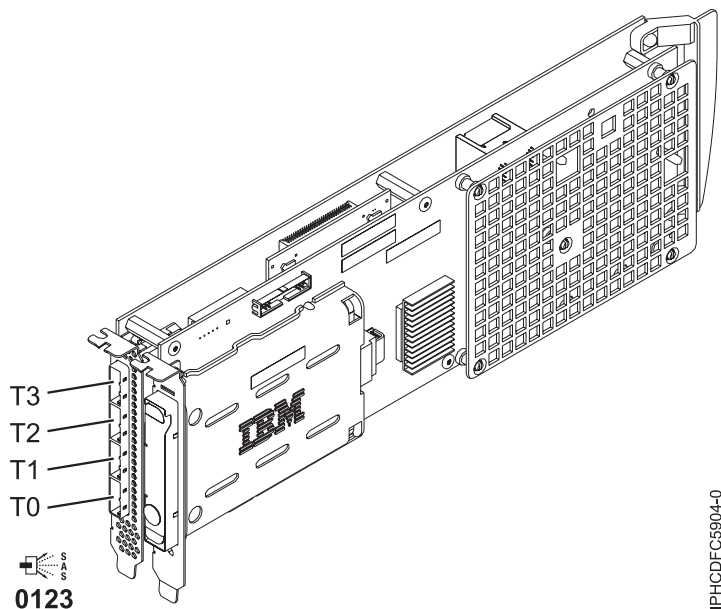
Figure 16. Carte SAS RAID PCI-X DDR 1,5 Go de cache
