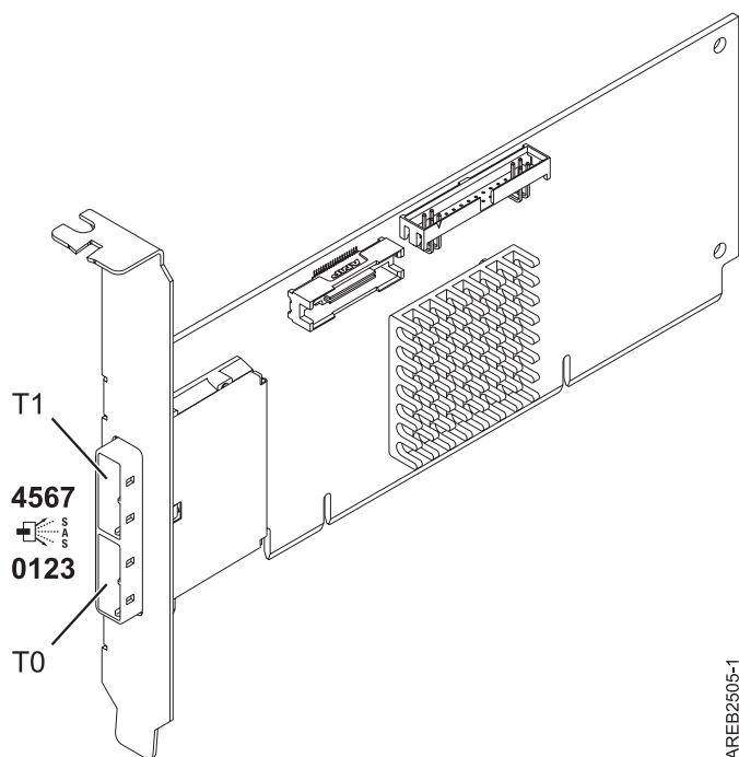
Figure 12. Carte SAS PCI-X DDR externe double accès – x4
