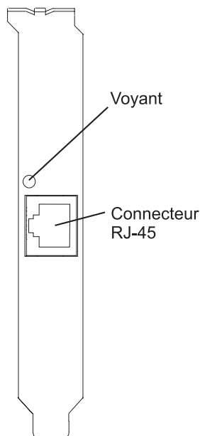
Figure 34. Voyant de la carte PCI-X TOE iSCSI TX 1 Gbit
