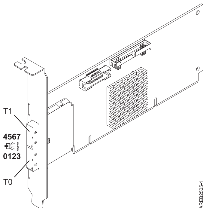
Figure 18. Carte SAS PCI-X DDR externe double accès – x4
