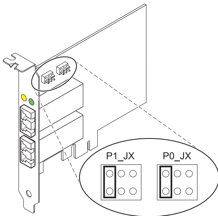
Figure 25. Cavalier ID unité
