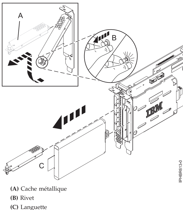
Figure 52. Remplacement de la batterie du cache d'une carte 572F/575C
