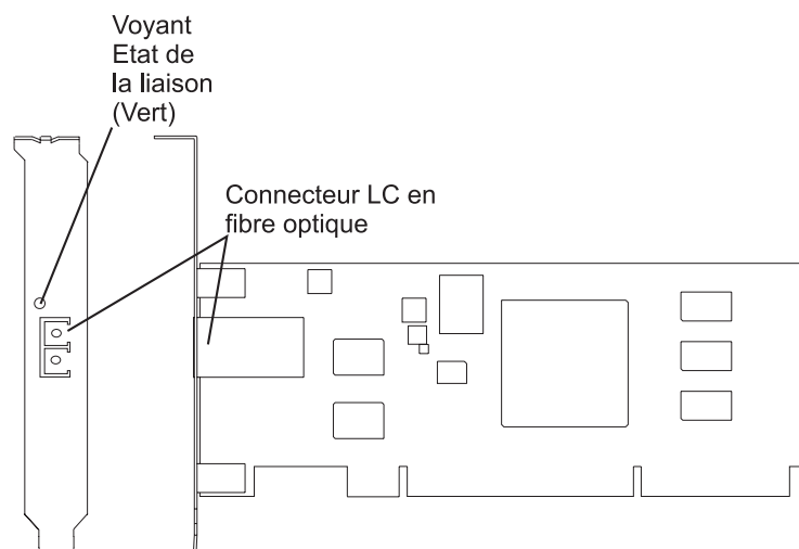
Figure 31. Carte PCI-X TOE iSCSI SX 1 Gbit
