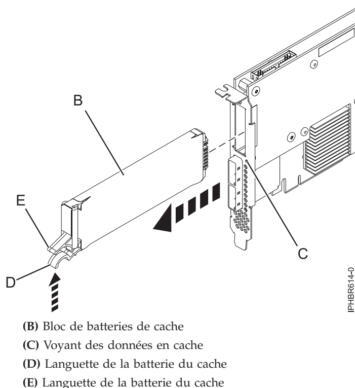
Figure 55. Remplacement de la batterie du cache d'une carte 574E
