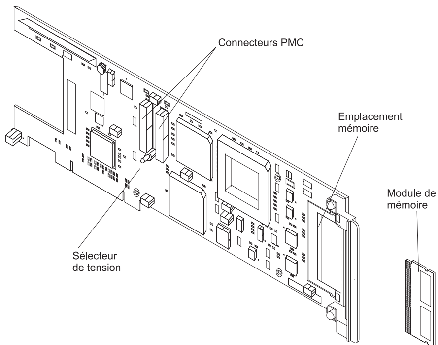
Figure 44. Carte PCI de base IBM ARTIC960Hx
