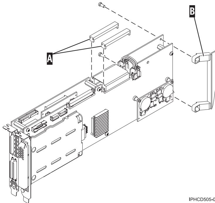
Figure 11. Préparation de la carte pour être placée dans une cassette
