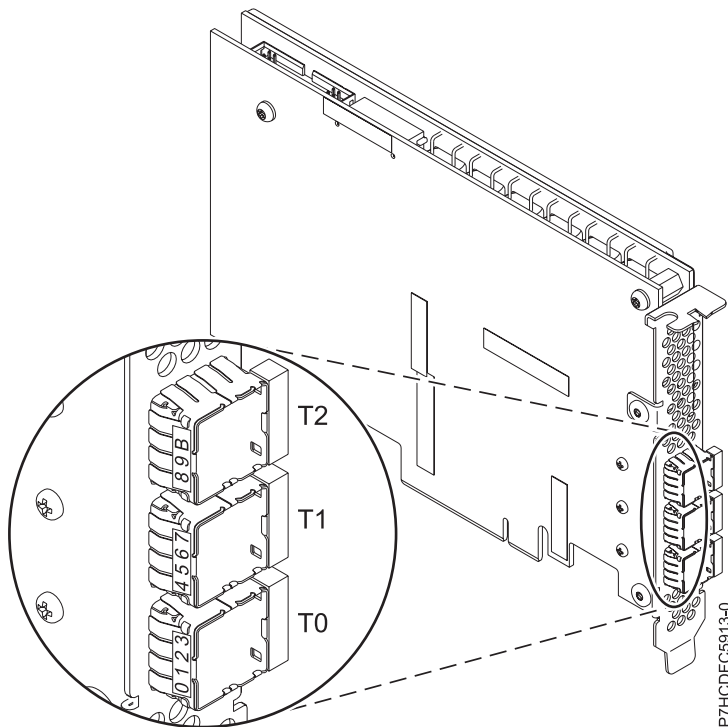
Figure 56. Carte 5913
