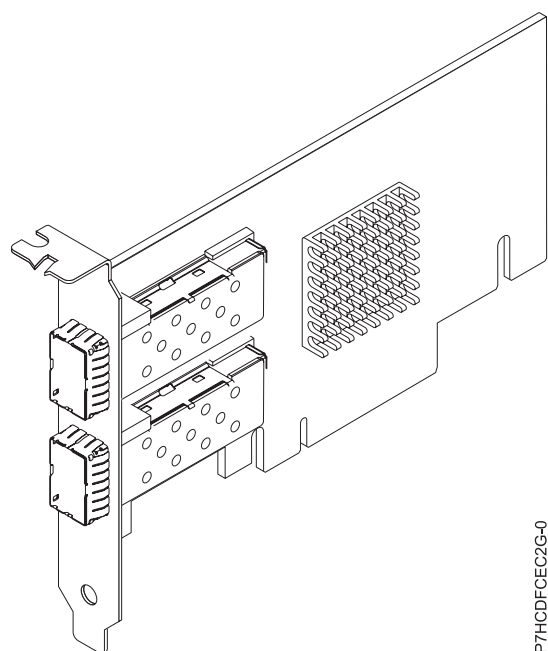
Figure 47. Carte FC EC2G
