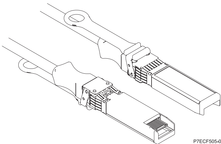
Figure 50. Schéma des extrémités du câble
