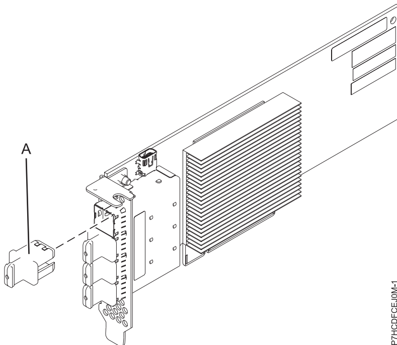
Figure 20. Carte PCIe3 SAS RAID de 6 Go LP à quatre ports
