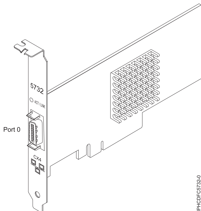
Figure 37. carte PCI Express (PCIe) 10 Gigabit Ethernet-CX4
