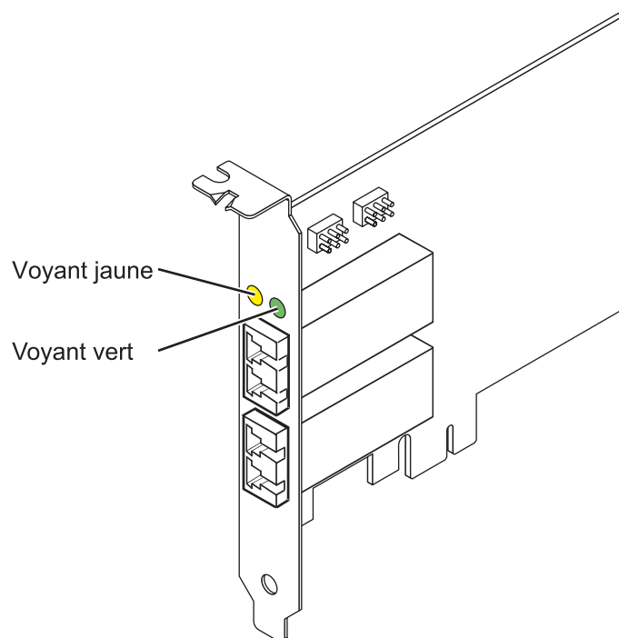
Figure 13. Carte 5774
