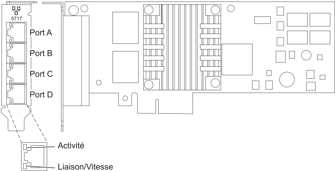
Figure 25. Carte FC 5271
