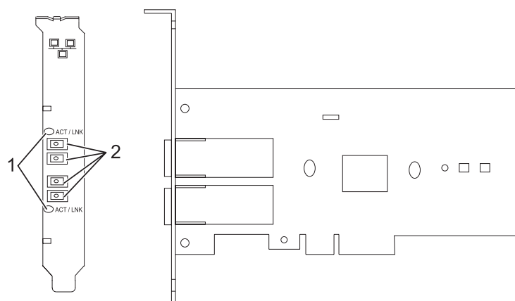
Figure 27. carte PCIe LP 2 ports 1GbE SX
