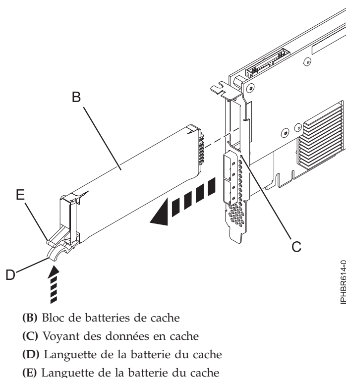
Figure 64. Remplacement de la batterie du cache d'une carte 574E
