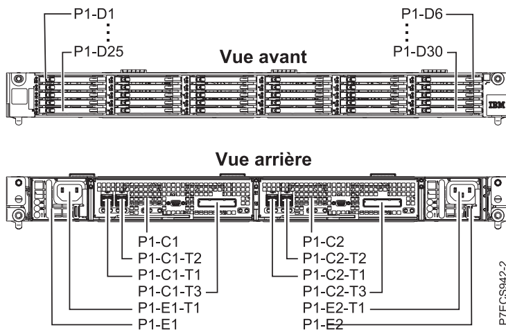
Figure 57. Codes d'emplacement de la carte PCIe2 SAS RAID intégrée avec cache de 3,1 Go
