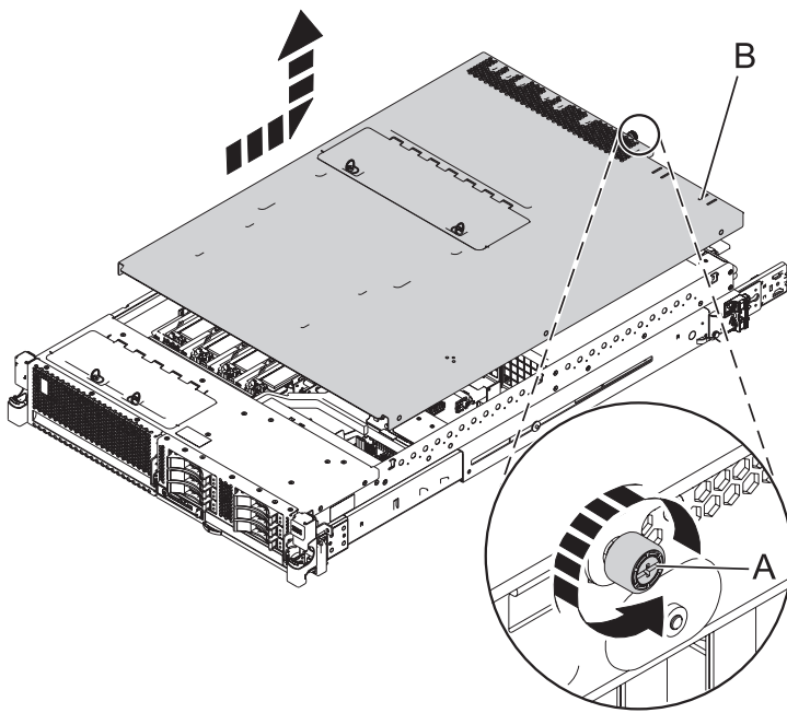
Figure 15. Retrait du capot d'accès
