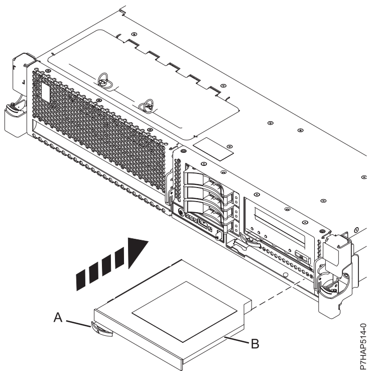
Figure 11. Installation de l'unité de stockage SAS
