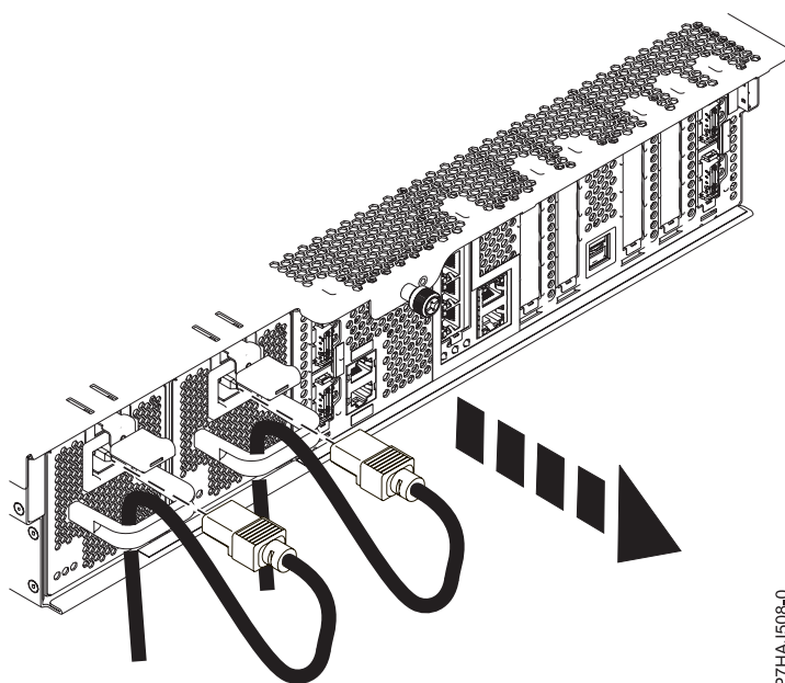
Figure 21. Retrait des cordons d'alimentation
