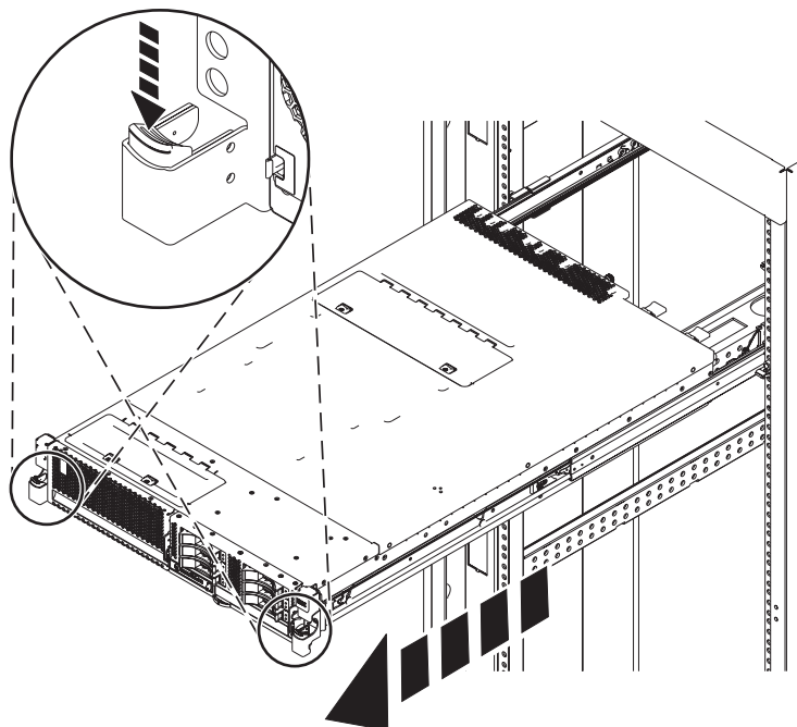
Figure 18. Placement du système en position de maintenance
