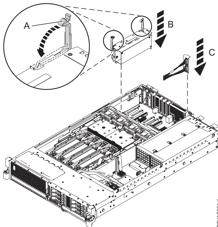
Figure 10. Remise en place de l'adaptateur GX à code dispositif EJ0G dans un système
