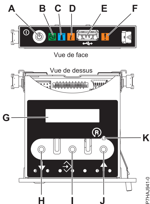
Figure 15. Panneau de commande
