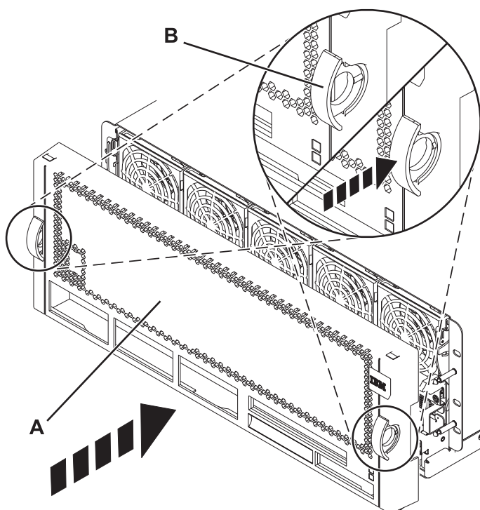
Figure 15. Installation du capot avant
