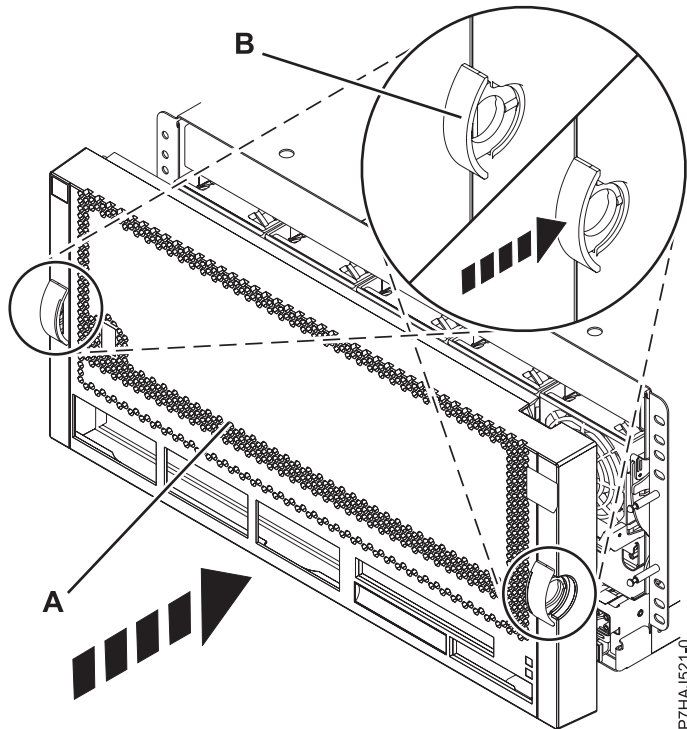
Figure 8. Installation du capot avant
