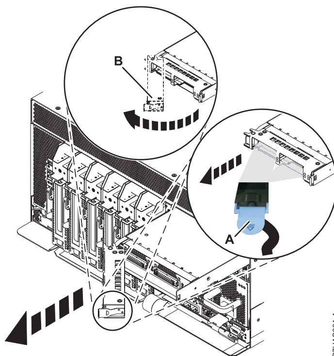
Figure 3. Retrait de l'adaptateur GX du système
