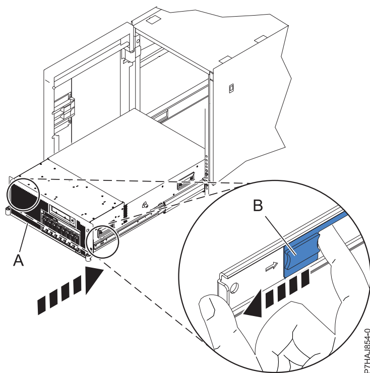
Figure 14. Déblocage des taquets de sécurité de la glissière
