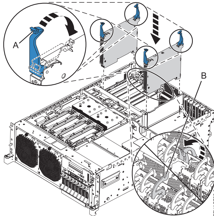
Figure 4. Installation de l'adaptateur GX (code dispositif EJ03) sur un système 8202-E4C, 8202-E4D, 8205-E6C ou 8205-E6D monté en armoire
