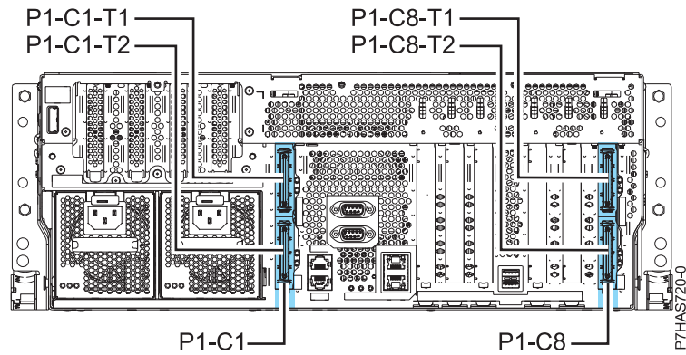
Figure 2. Vue arrière du système 8202-E4C, 8202-E4D, 8205-E6C ou 8205-E6D avec illustration des emplacements d'adaptateur GX++ P1-C2 et P1-C8
