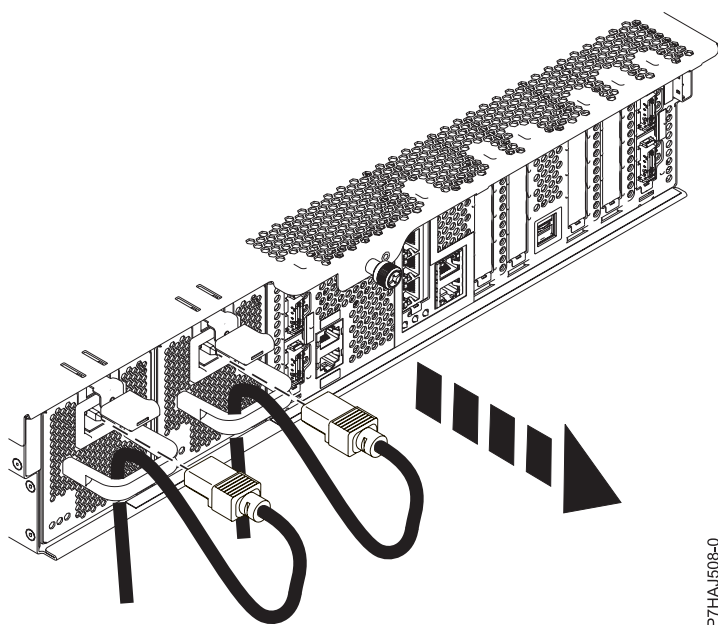
Figure 16. Retrait des cordons d'alimentation
