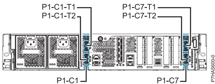
Figure 1. Vue arrière du système 8231-E2B montrant les emplacements pour adaptateur GX et codes d'emplacement
