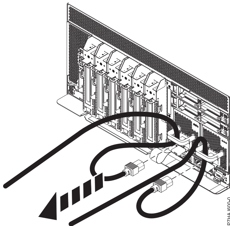
Figure 4. Débranchement des cordons d'alimentation
