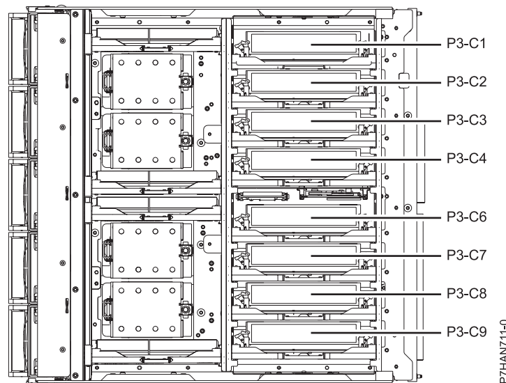
Figure 14. Séquence de branchement des cartes d'extension de mémoire
