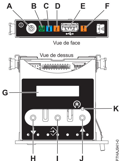
Figure 26. Panneau de commande
