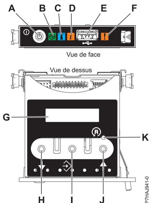
Figure 25. Panneau de commande
