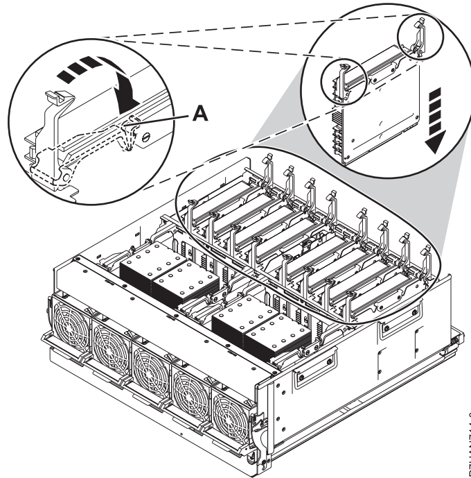
Figure 9. Remplacement d'une carte d'extension de mémoire
