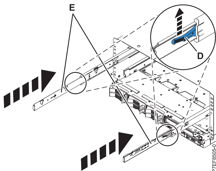
Figure 31. Déverrouillage des taquets de sécurité du rail
