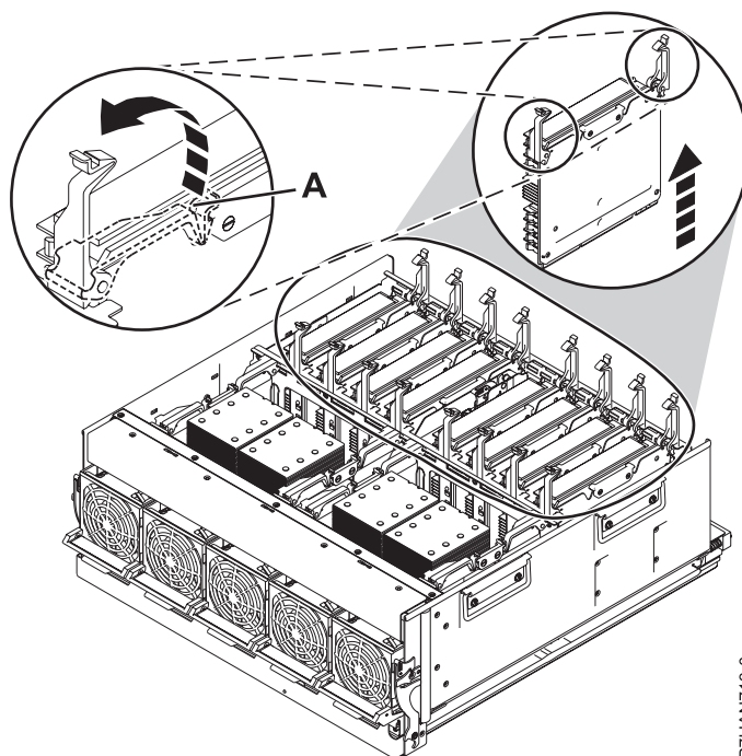
Figure 18. Retrait d'une carte d'extension de mémoire
