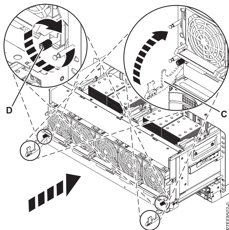
Figure 32. Verrouillage des taquets de l'unité centrale
