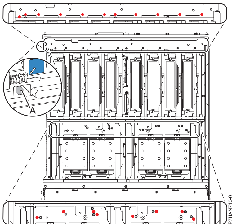
Figure 5. Bouton de commande sur la carte
