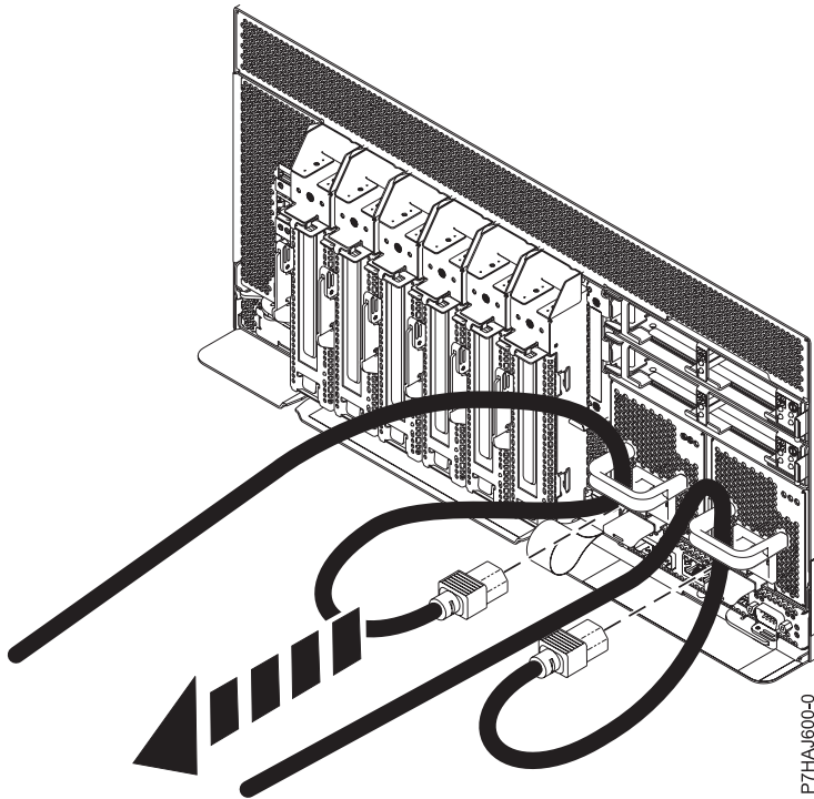
Figure 7. Débranchement des cordons d'alimentation
