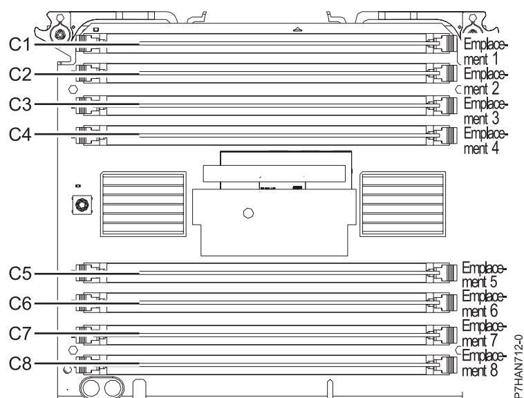
Figure 15. Emplacements des modules de mémoire pour le système 8248-L4T, 8408-E8D ou 9109-RMD
