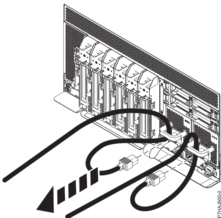
Figure 16. Débranchement des cordons d'alimentation
