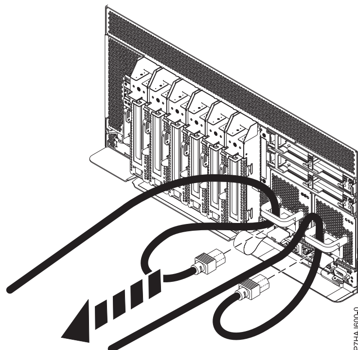
Figure 21. Débranchement des cordons d'alimentation
