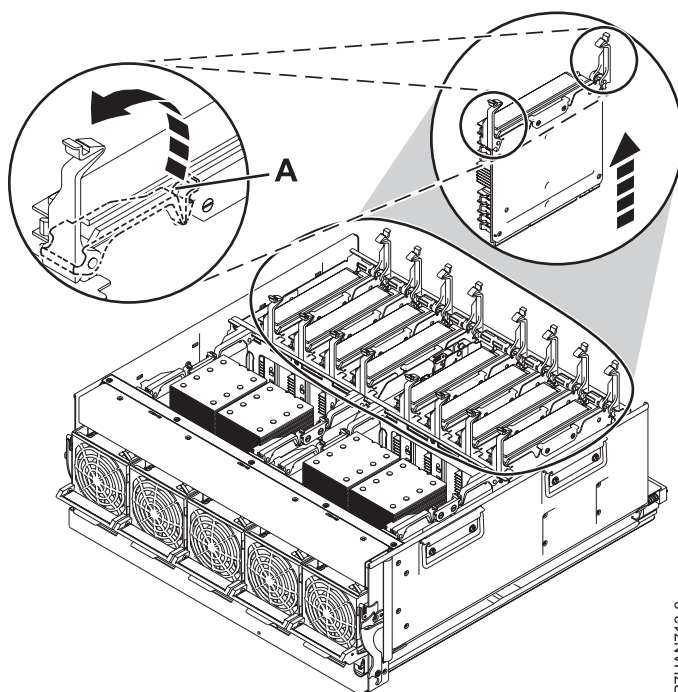
Figure 12. Retrait de la carte d'extension de mémoire
