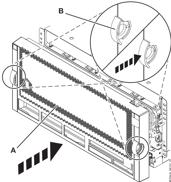
Figure 28. Installation du capot avant
