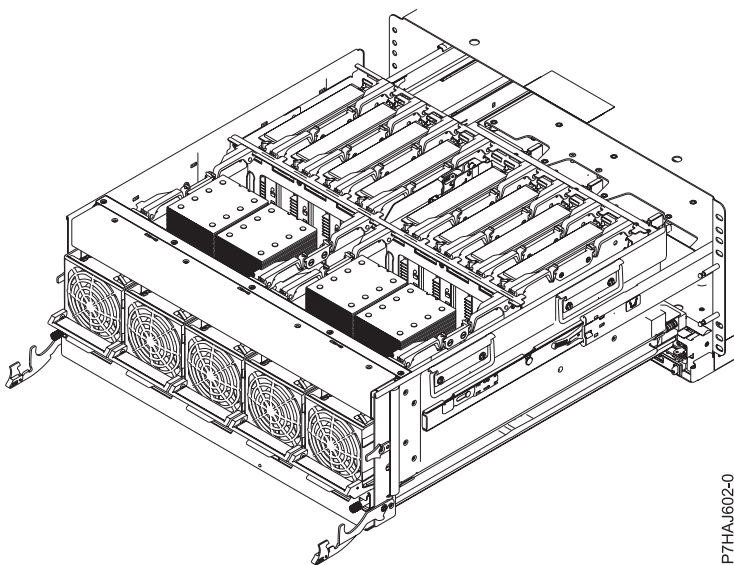
Figure 30. Système en position de maintenance
