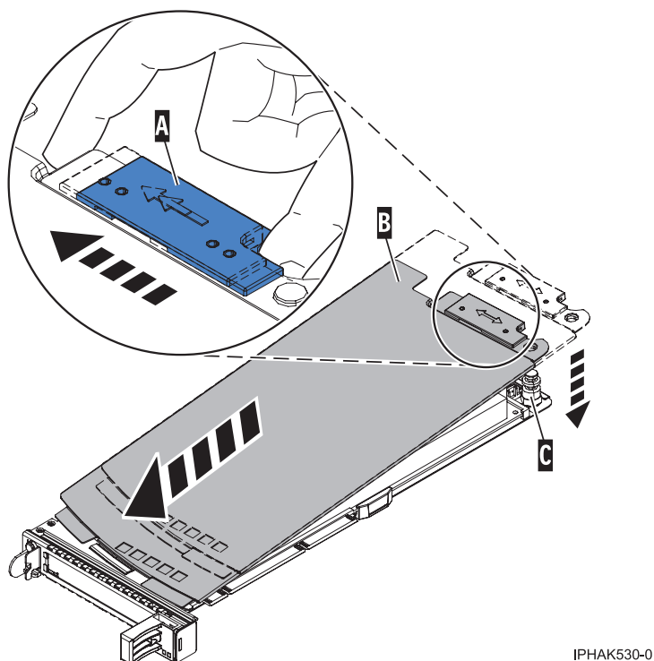
Figure 82. Réinstallation du couvercle de la cassette de cartes PCI
