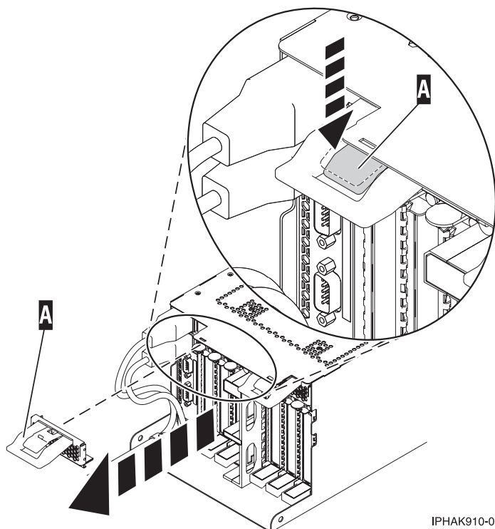
Figure 63. Retrait du blindage électromagnétique
