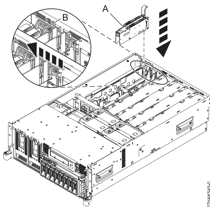
Figure 32. Remplacement de la carte PCI RAID et SSD SAS d'une unité centrale montée en armoire
