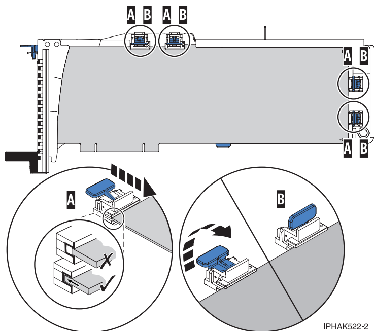
Figure 109. Installation d'une carte longue dans la cassette de cartes PCI (crochets de retenue et stabilisateur en place)
