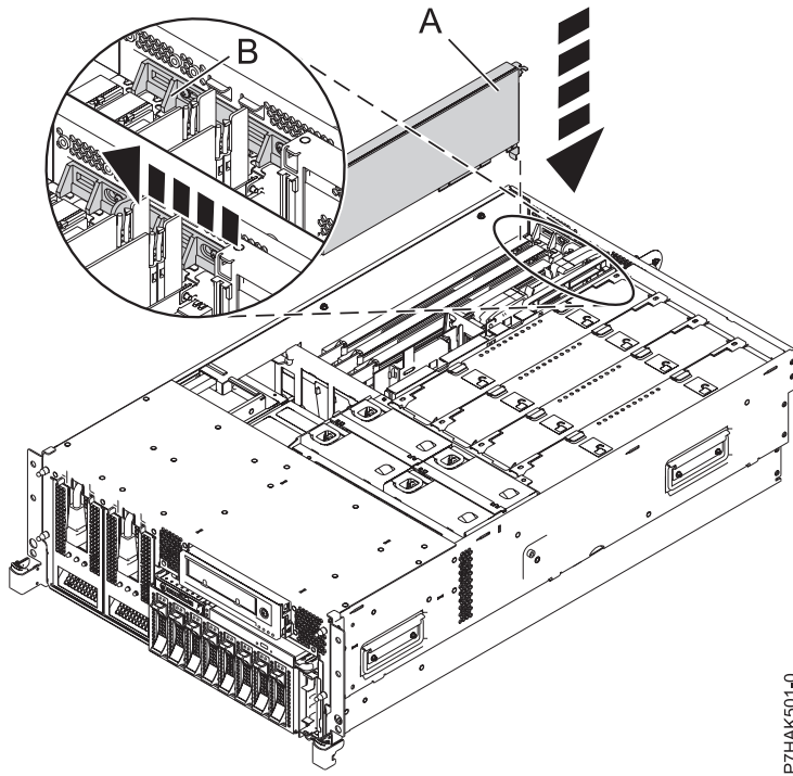
Figure 17. Remplacement de la carte PCI d'une unité centrale montée en armoire
