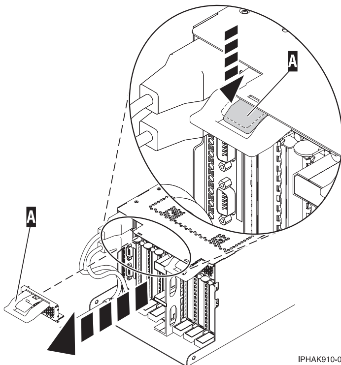
Figure 61. Retrait du blindage électromagnétique
