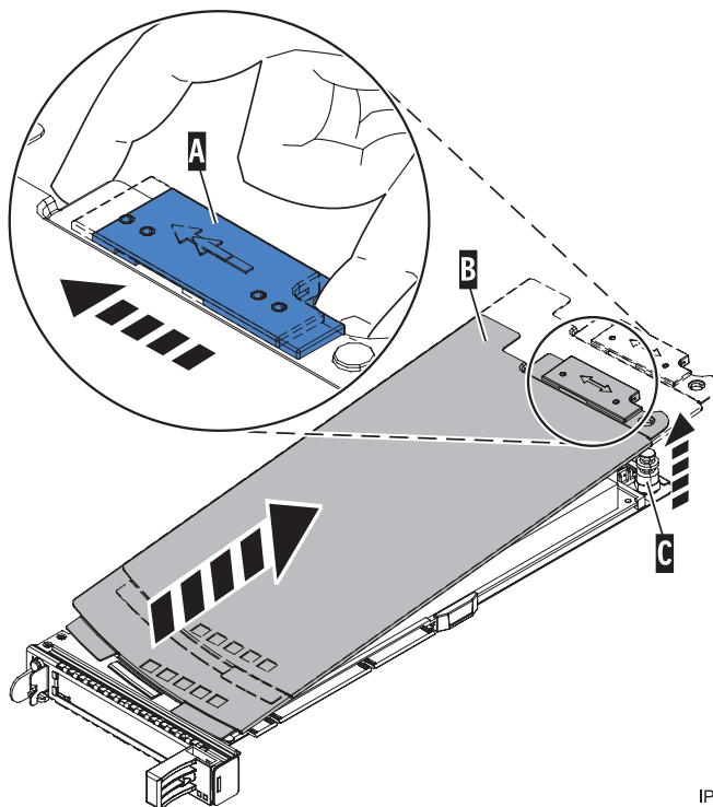
Figure 75. Retrait du couvercle de la cassette de cartes PCI simple largeur
