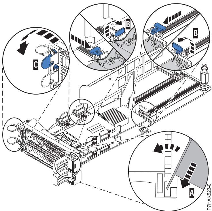
Figure 120. Remplacement d'une carte PCIe RAID et SSD SAS dans la cassette de la carte PCI
