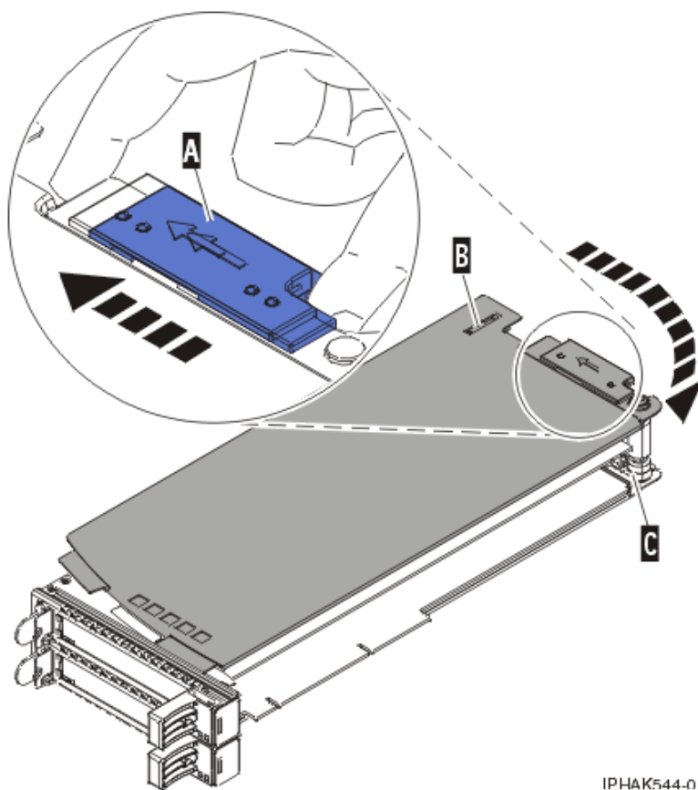
Figure 117. Retrait du couvercle de la cassette de cartes PCI
