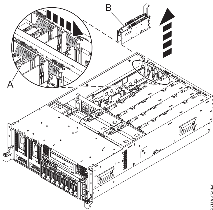
Figure 27. Retrait d'une carte PCI RAID et SSD SAS d'une unité centrale montée en armoire
