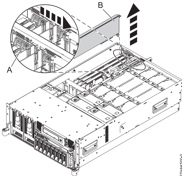
Figure 14. Retrait du panneau obturateur ou de la carte PCI d'une unité centrale montée en armoire
