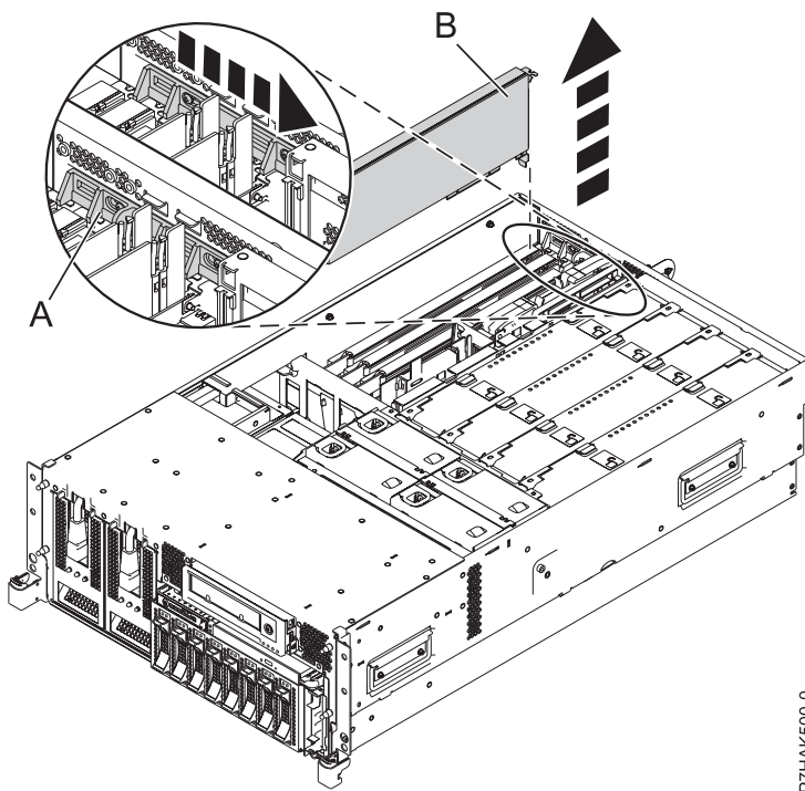
Figure 31. Retrait du panneau obturateur ou de la carte PCI d'une unité centrale montée en armoire
