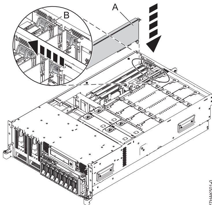
Figure 16. Remplacement de la carte PCI d'une unité centrale montée en armoire
