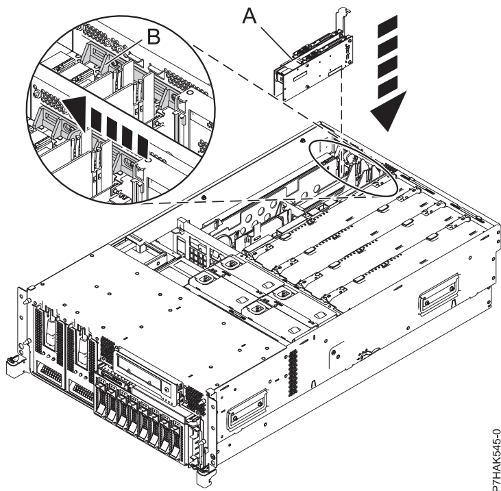
Figure 33. Remplacement de la carte PCI RAID et SSD SAS d'une unité centrale montée en armoire
