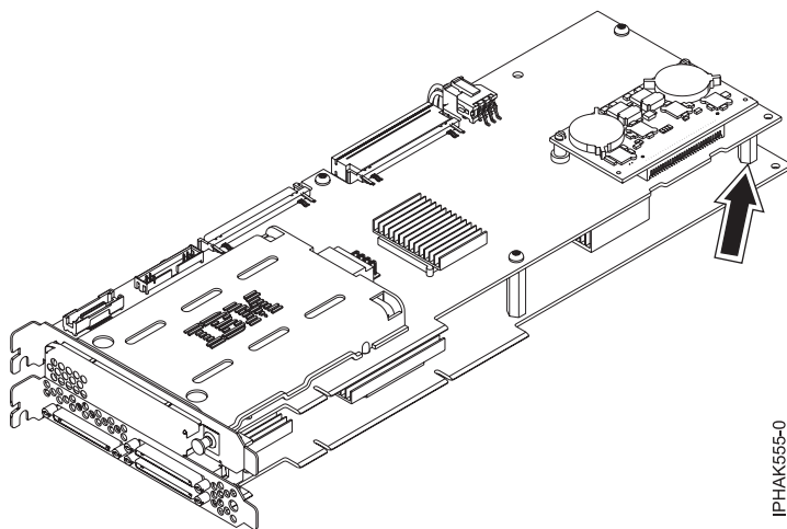
Figure 125. Retrait de la vis de butée
