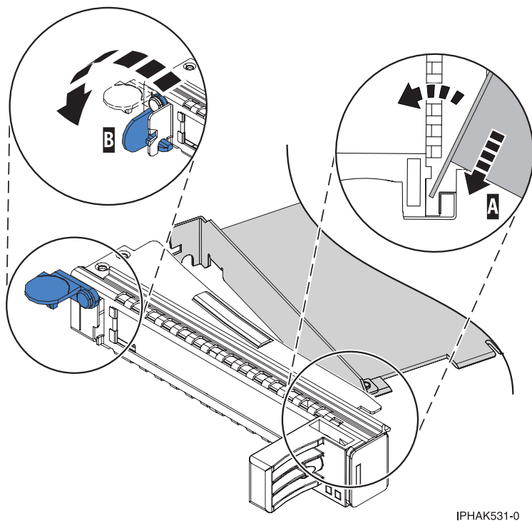
Figure 84. Installation d'une cassette d'adaptateurs (cartes) PCI simple largeur
