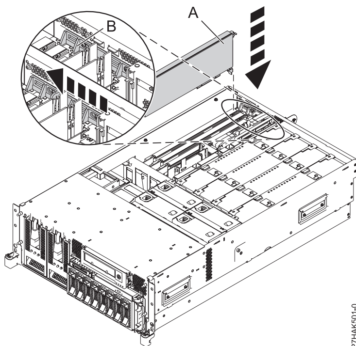
Figure 15. Remplacement de la carte PCI d'une unité centrale montée en armoire
