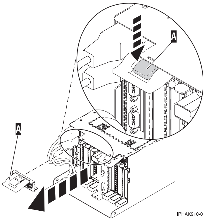
Figure 59. Retrait du blindage électromagnétique
