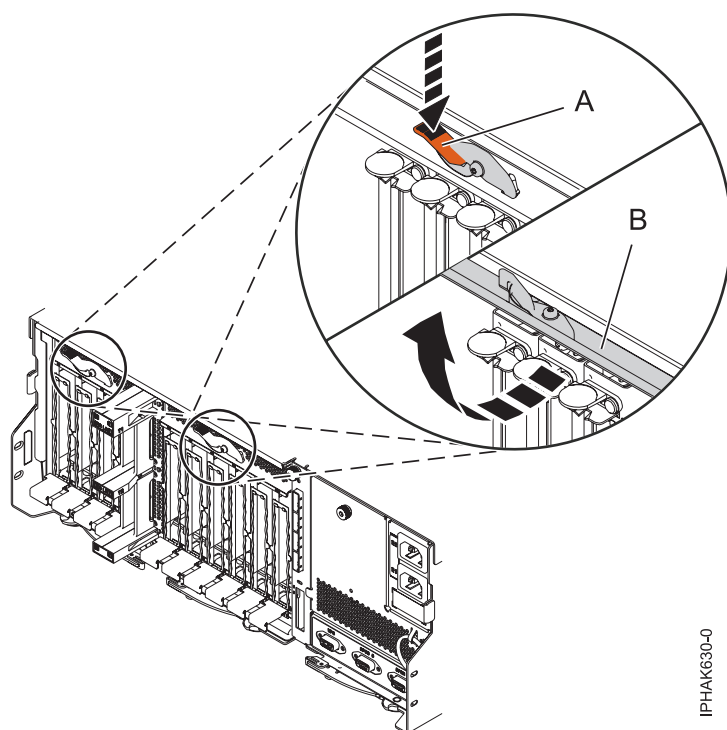
Figure 100. Ouverture du capot d'accès
