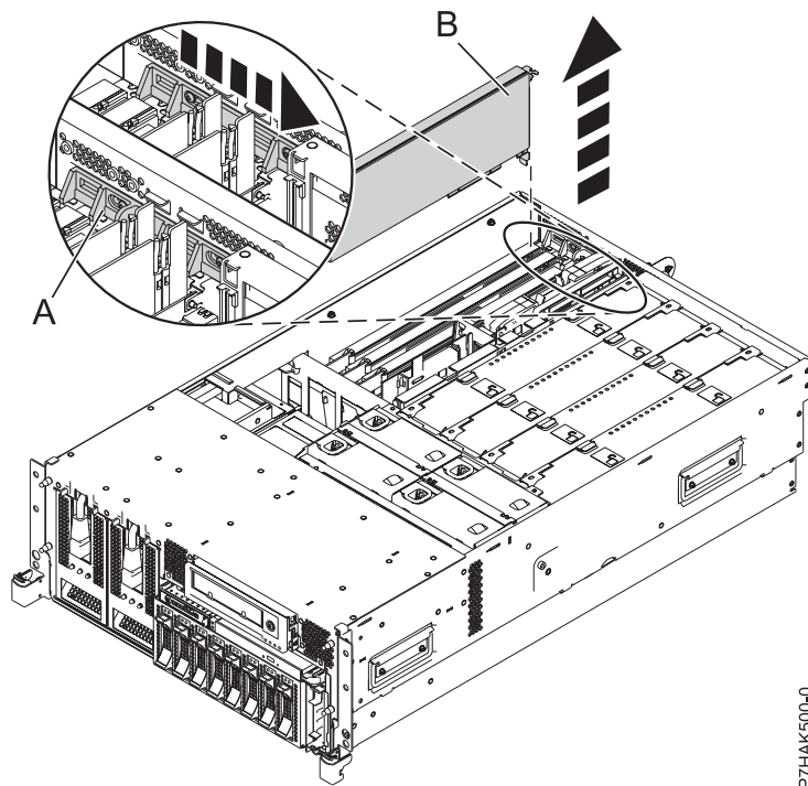
Figure 35. Retrait du panneau obturateur ou de la carte PCI d'une unité centrale montée en armoire
