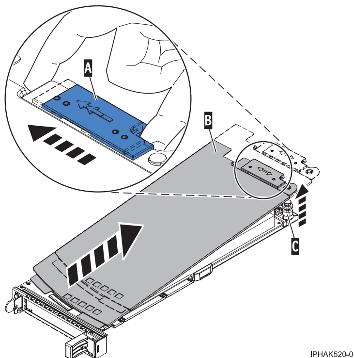
Figure 88. Retrait du couvercle de la cassette de cartes PCI
