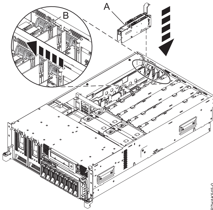
Figure 19. Remplacement de la carte PCIe RAID et SSD SAS d'une unité centrale montée en armoire
