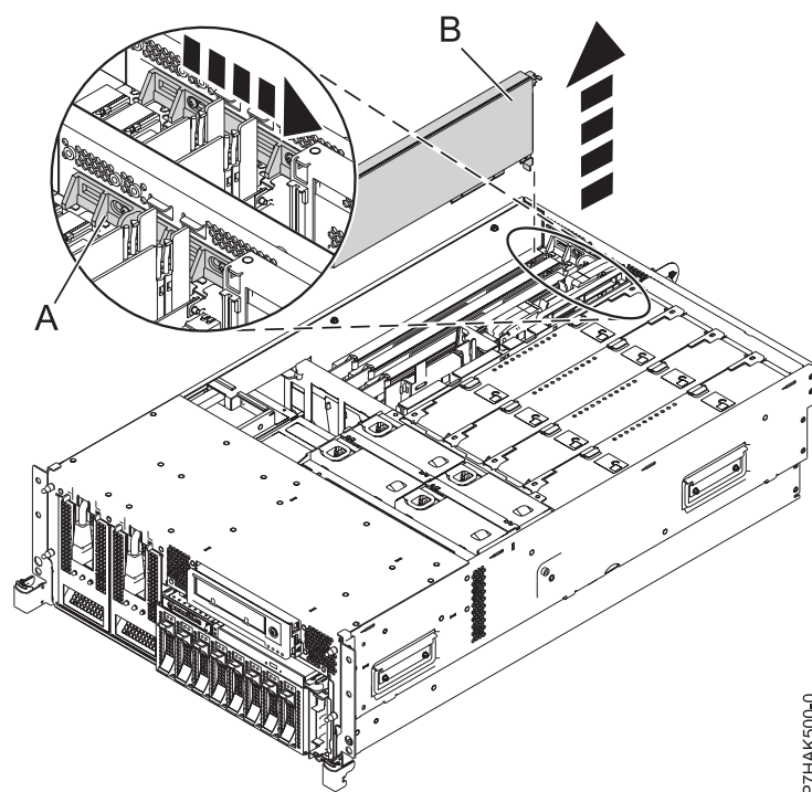
Figure 10. Retrait du panneau obturateur ou de la carte PCI d'une unité centrale montée en armoire
