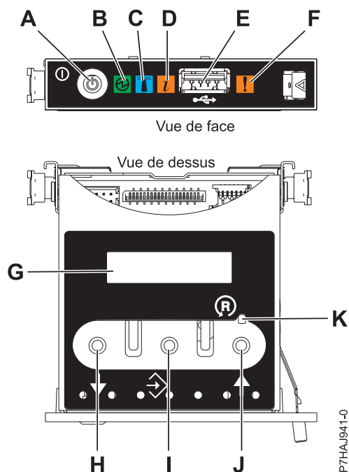
Figure 127. Panneau de commande
