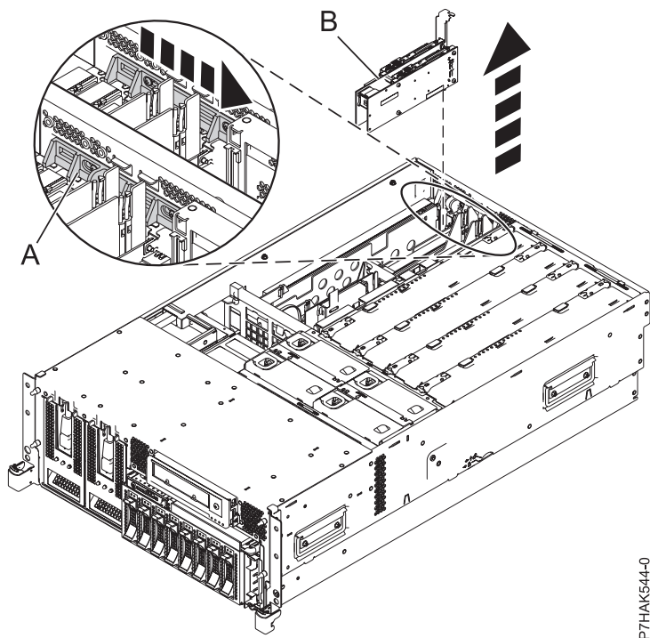
Figure 29. Retrait d'une carte PCI RAID et SSD SAS d'une unité centrale montée en armoire
