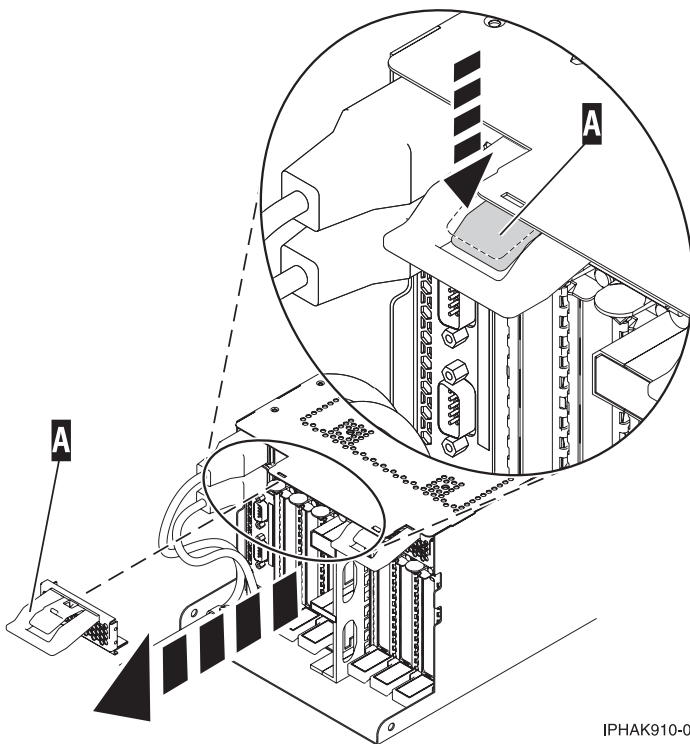
Figure 68. Retrait du blindage électromagnétique
