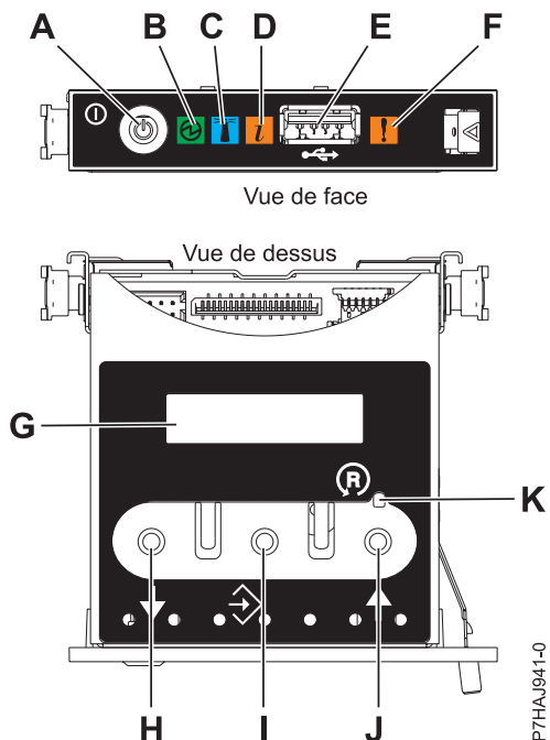
Figure 128. Panneau de commande
