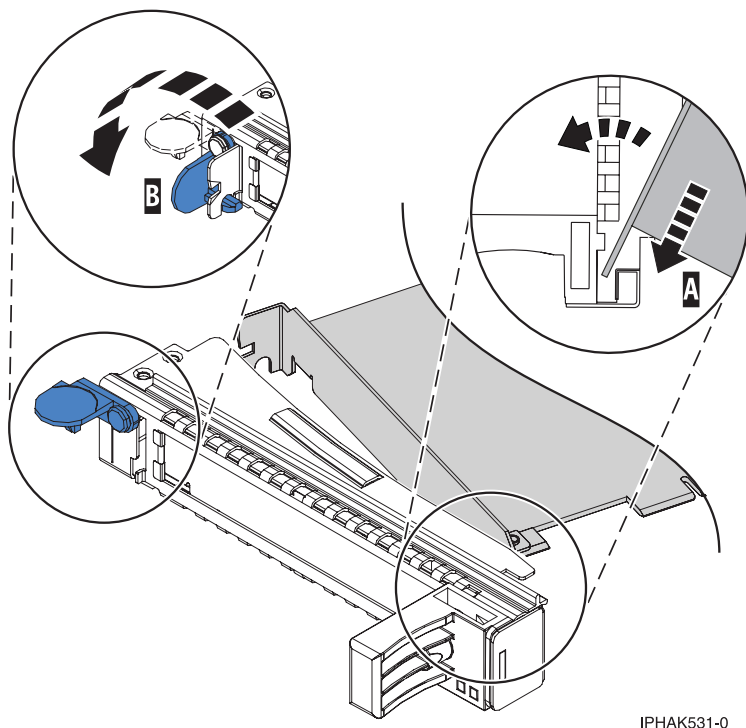
Figure 78. Retrait de la carte de la cassette de cartes PCI simple largeur
