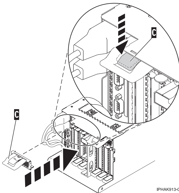
Figure 56. Blindage électromagnétique de la carte PCI en position fermée
