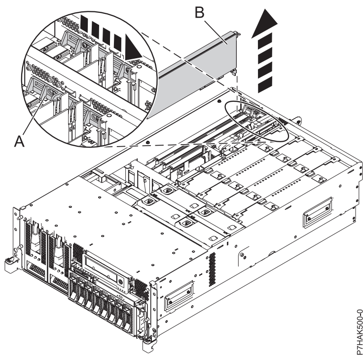
Figure 38. Retrait du panneau obturateur ou de la carte PCI d'une unité centrale montée en armoire
