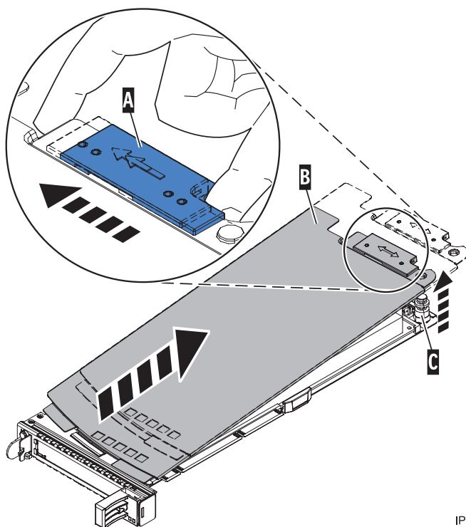
Figure 105. Retrait du couvercle de la cassette de cartes PCI simple largeur
