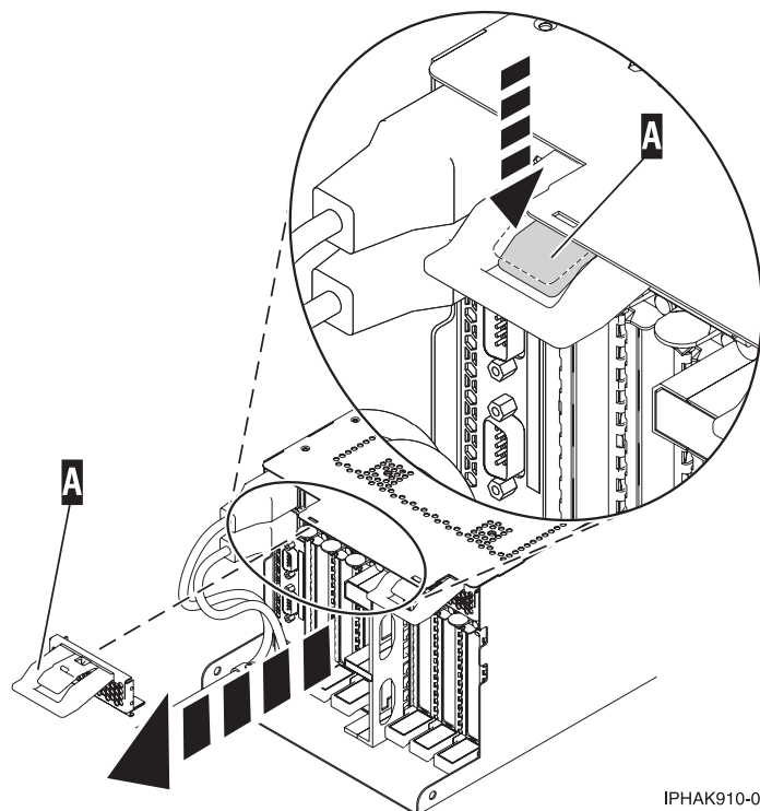
Figure 65. Retrait du blindage électromagnétique
