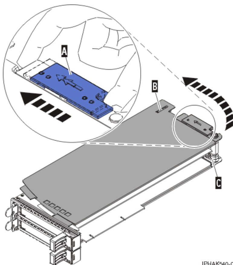
Figure 116. Réinstallation du couvercle de la cassette de cartes PCI
