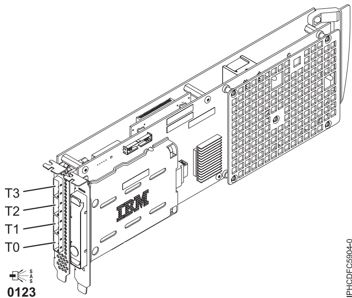
Figure 126. Carte SAS RAID PCI-X DDR 1,5 Go de cache
