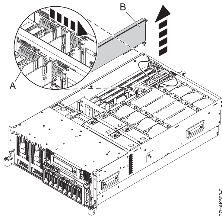
Figure 22. Retrait du panneau obturateur ou de la carte PCI d'une unité centrale montée en armoire
