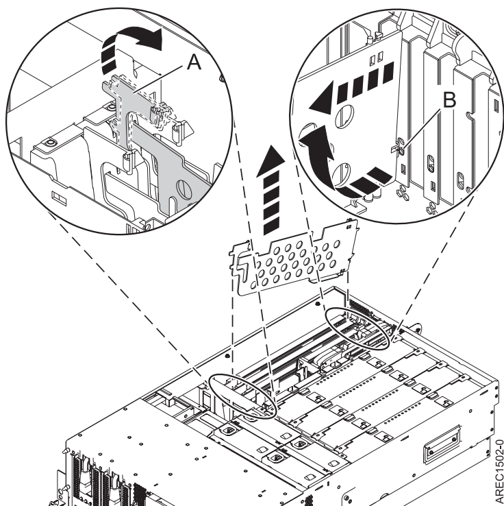
Figure 36. Retrait du diviseur de carte PCI d'une unité centrale
