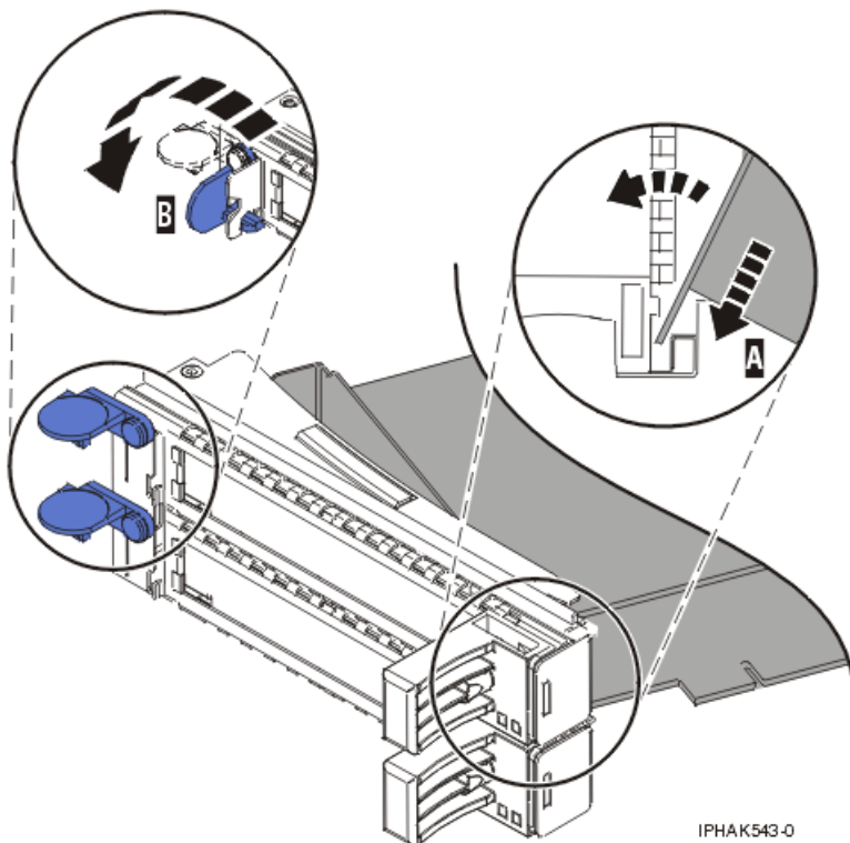
Figure 95. Remplacement de la carte de la cassette de cartes PCI
