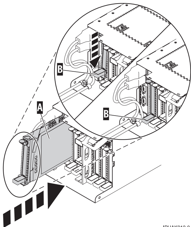
Figure 55. Installation de la cassette de cartes PCI dans l'unité centrale
