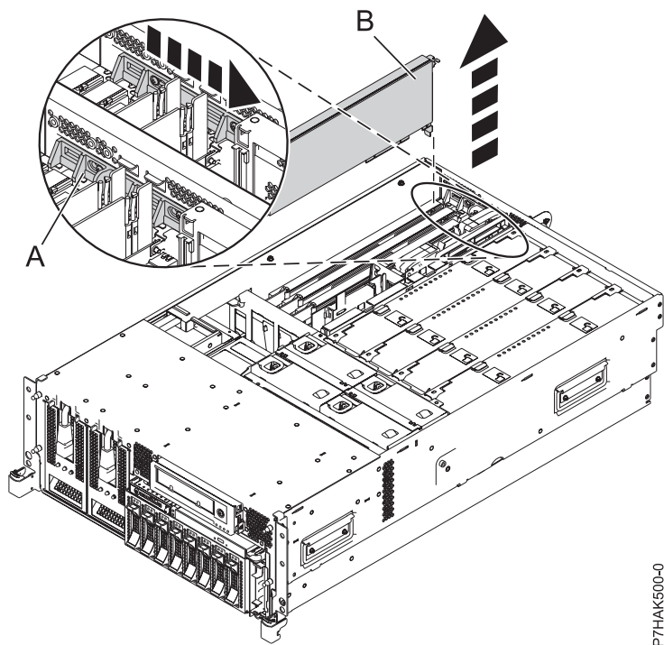
Figure 12. Retrait du panneau obturateur ou de la carte PCI d'une unité centrale montée en armoire
