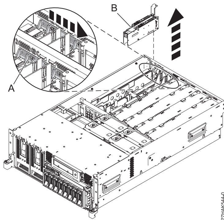
Figure 26. Retrait d'une carte PCI RAID et SSD SAS d'une unité centrale montée en armoire
