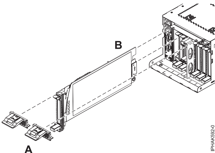
Figure 87. Remplacement de la cassette et installation de la protection électromagnétique
