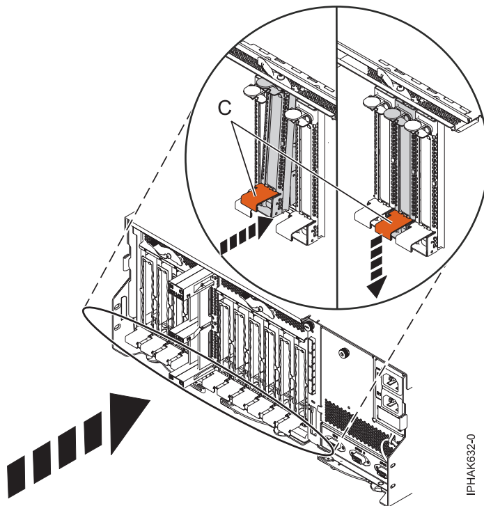
Figure 98. Installation de la cassette de cartes PCI
