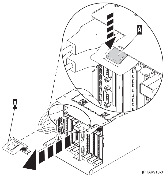
Figure 72. Retrait du blindage électromagnétique
