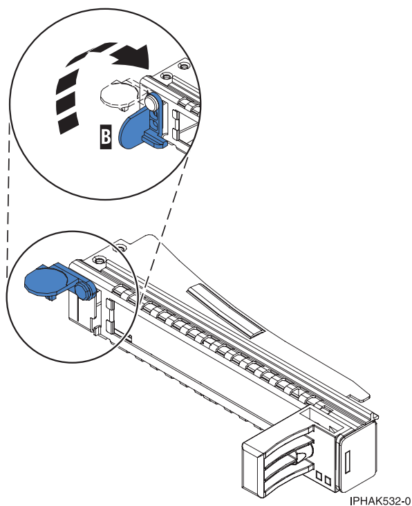
Figure 77. Levier de blocage de la poupée en position ouverte
