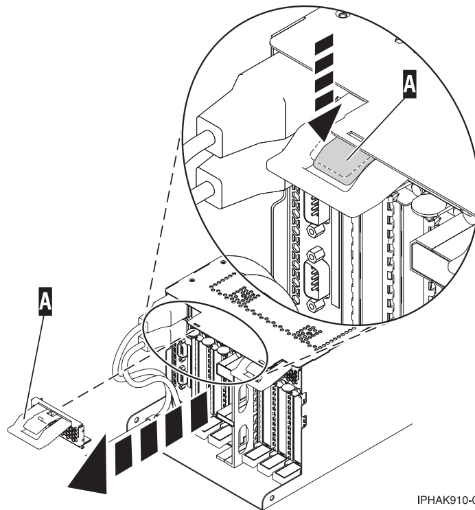
Figure 53. Retrait du blindage électromagnétique
