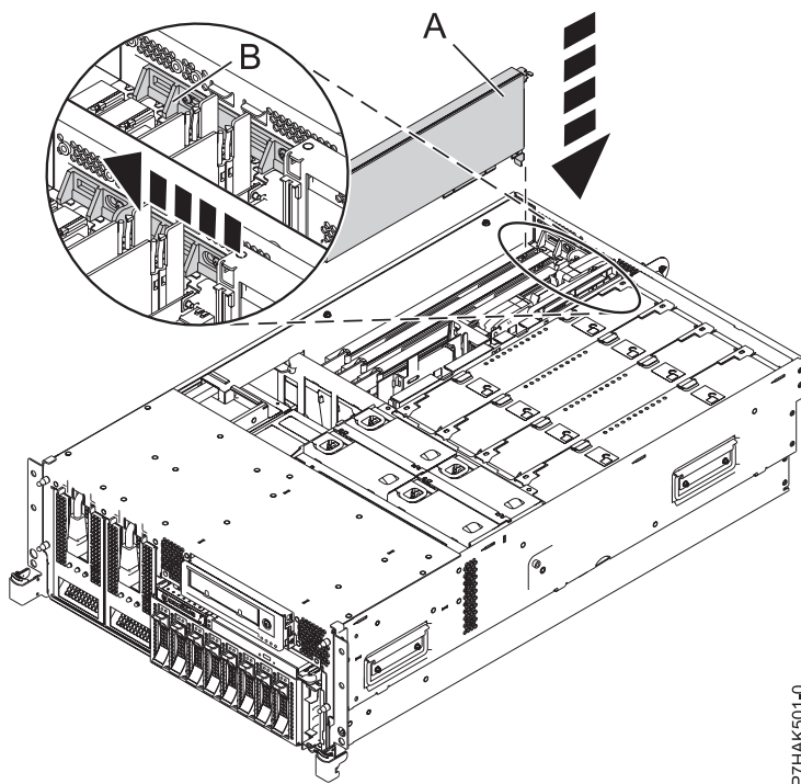
Figure 40. Remplacement de la carte PCI d'une unité centrale montée en armoire
