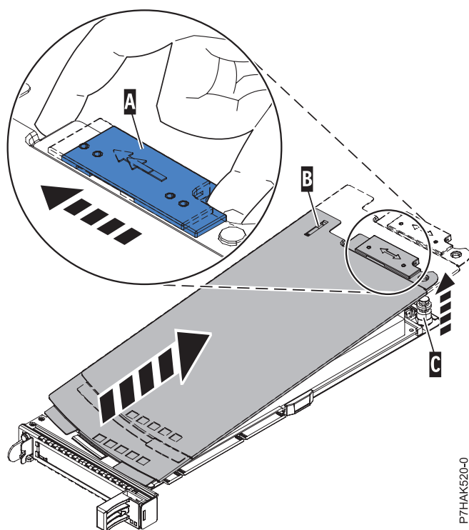
Figure 102. Retrait du couvercle de la cassette de cartes PCI
