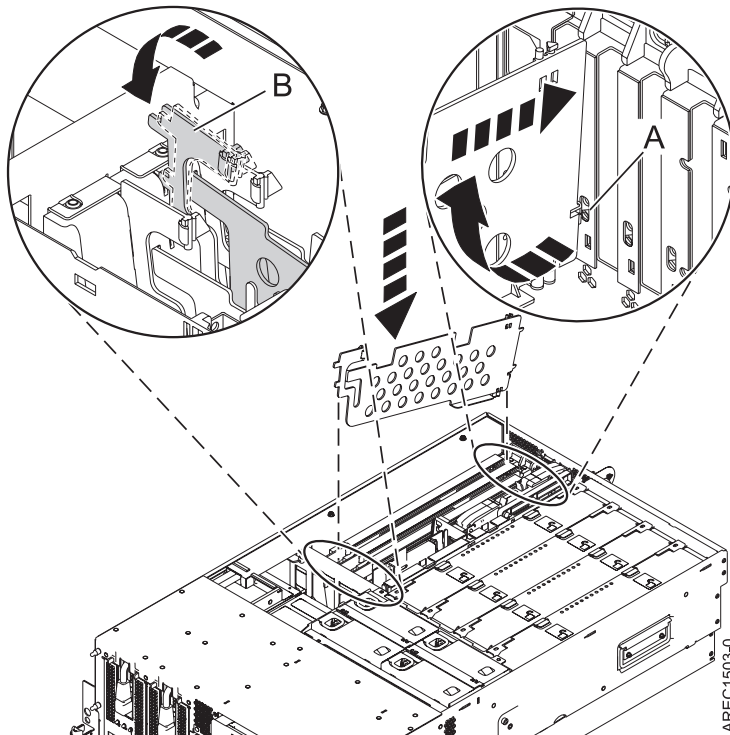
Figure 39. Remplacement du diviseur de carte PCI sur une unité centrale
