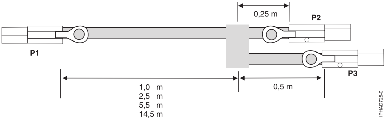
Figure 138. Longueurs de câble d'assemblage de câble YO externe SAS
