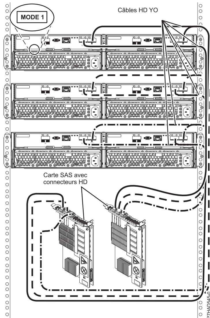
Figure 170. Connexion de mode 1 de trois tiroirs 5887 à deux cartes SAS avec connecteurs HD
