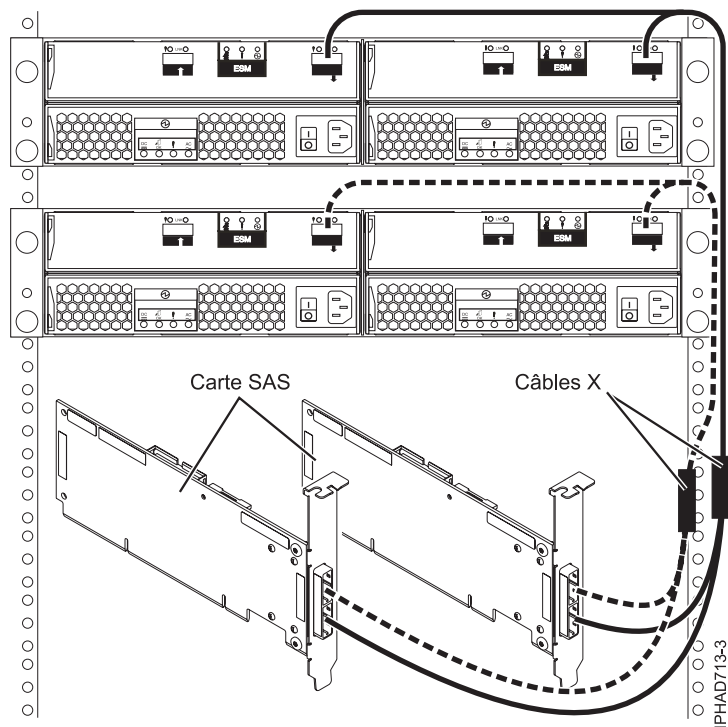
Figure 150. Connexion de deux cartes SAS RAID à deux tiroirs d'extension de disque dans une configuration RAID haute disponibilité multi-initiateur
