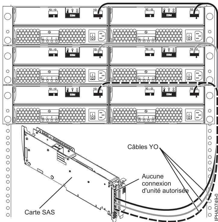
Figure 143. Connexion d'une carte SAS trois ports à des tiroirs d'extension de disque
