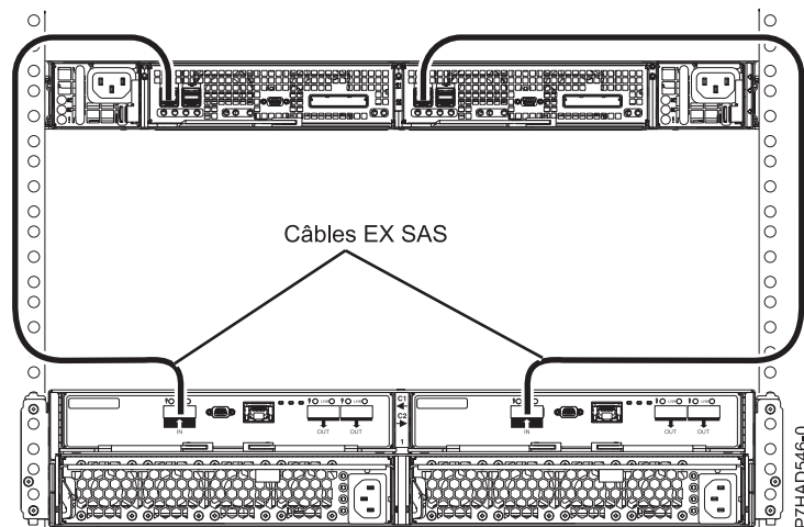
Figure 172. Connexion d'un tiroir 5887 à l'aide de câbles HD EX vers une armoire EDR1
