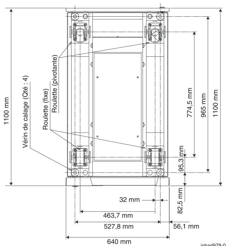
Figure 4. Emplacement des roulettes et des vérins de calage
