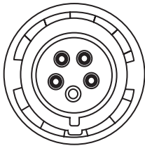
Figure 31. Brochage de fiche
