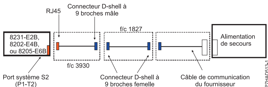
Figure 133. Câblage de l'alimentation de secours pour les modèles 8202-E4B, 8202-E4C, 8205-E6B, 8205-E6C, 8231-E2B, 8231-E1C, 8231-E1D, 8231-E2C, 8231-E2D et 8268-E1D
