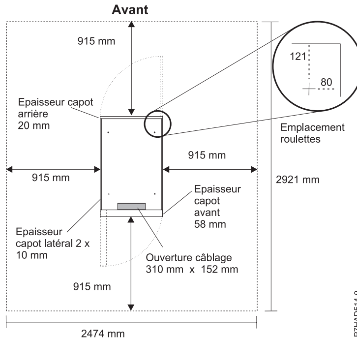
Figure 22. Dégagements et emplacement des roulettes pour les armoires modèles 7014-T00, 7014-T42 et 0553
