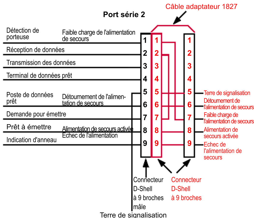
Figure 127. Câblage du câble 1827
