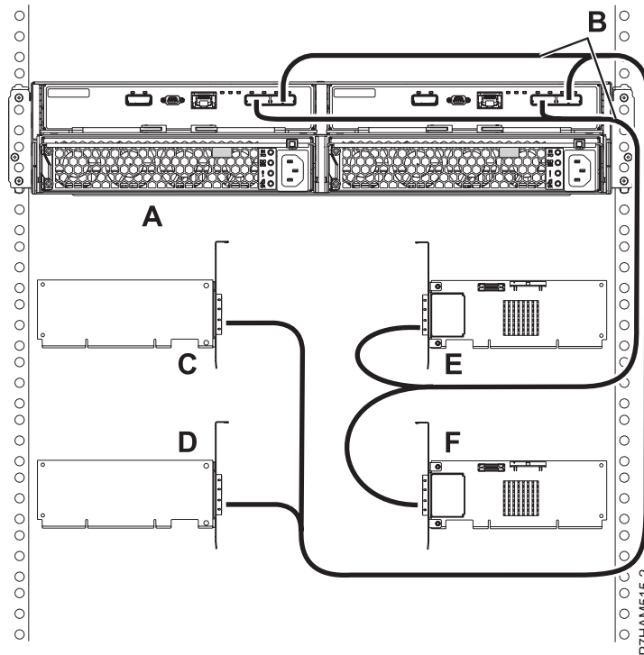
Figure 163. Connexion de mode 4 d'un tiroir 5887 à quatre cartes SAS via des câbles X
