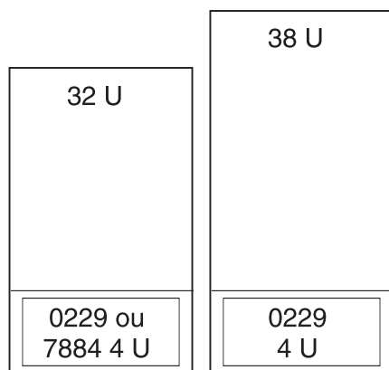
Figure 5. Code dispositif 7884 : 9406-520 et 9111-520 en armoire
