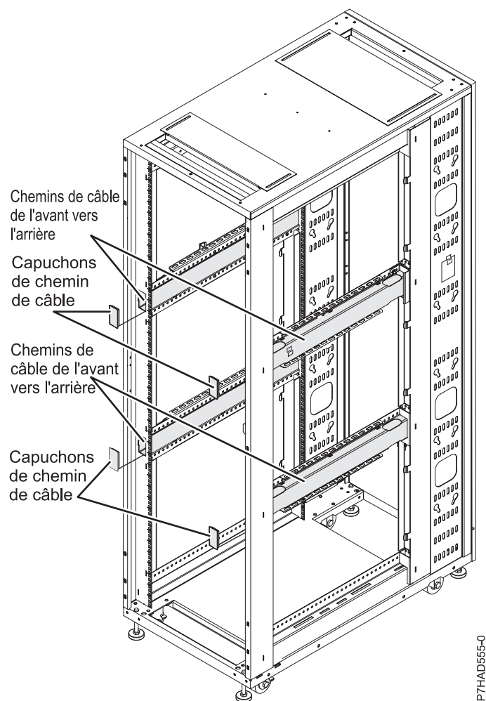
Figure 24. Câblage dans l'armoire
