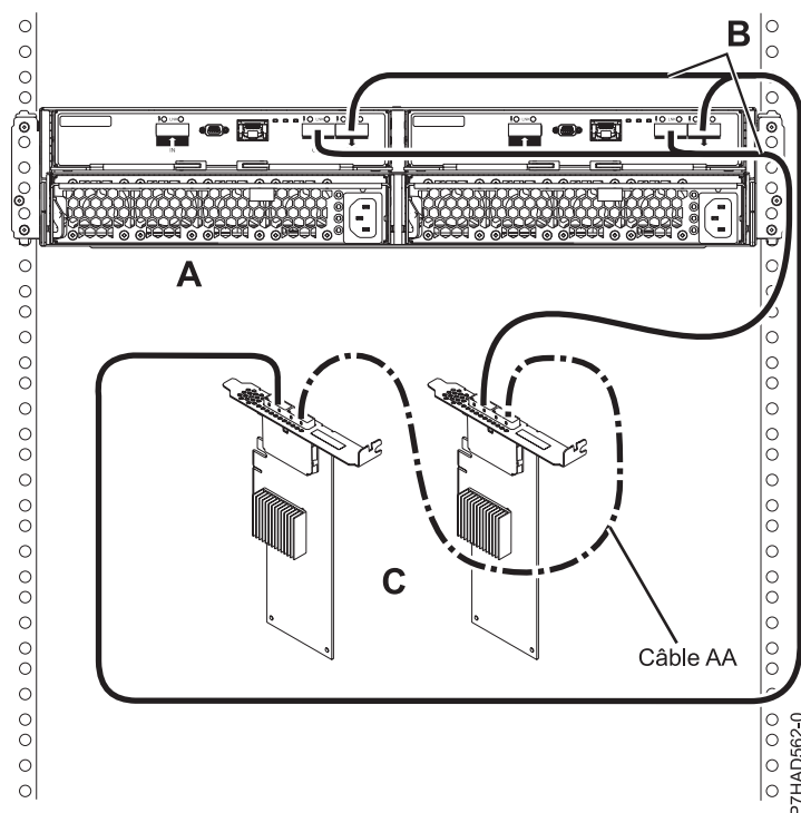
Figure 160. Connexion de mode 1 d'un tiroir 5887 à deux cartes SAS via des câbles YO
