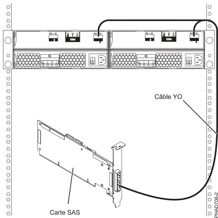
Figure 140. Connexion d'une carte SAS à un tiroir d'extension de disque
