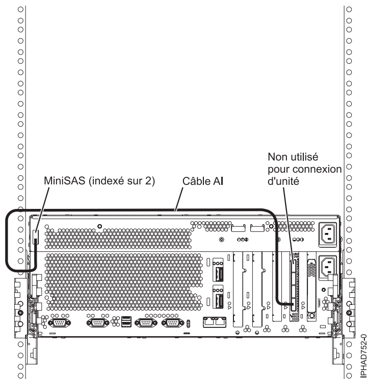
Figure 148. Adaptateur FC 5904 ou FC 5908 connecté à des tiroirs d'extension de disque
