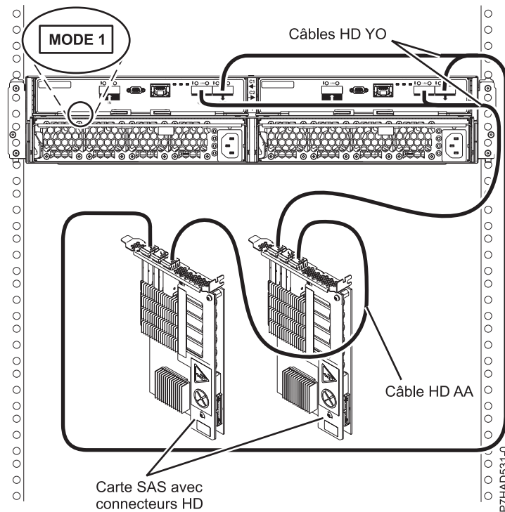
Figure 168. Connexion de mode d'un tiroir 5887 à deux cartes SAS avec connecteurs HD
