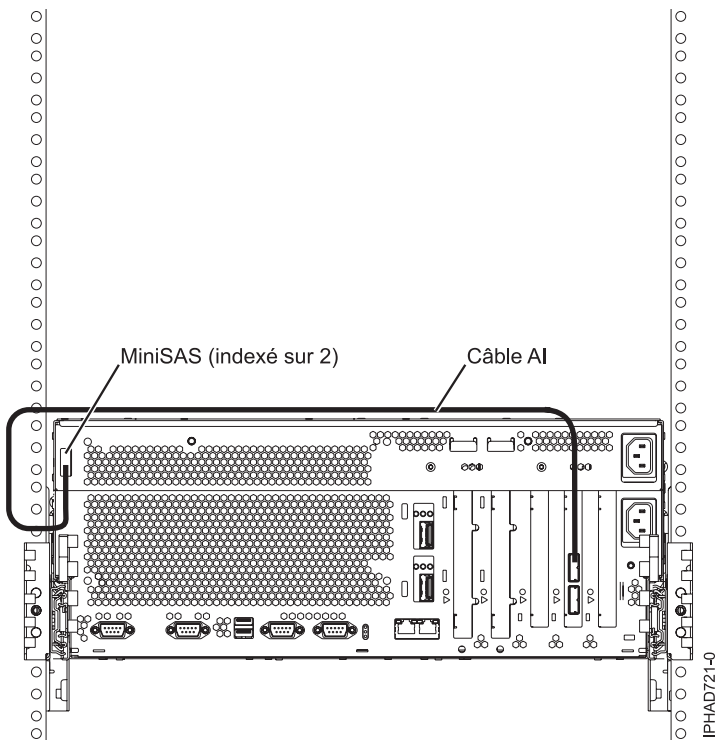
Figure 147. Raccordement de l'adaptateur SAS aux emplacements de disques SAS internes via le port SAS système externe
