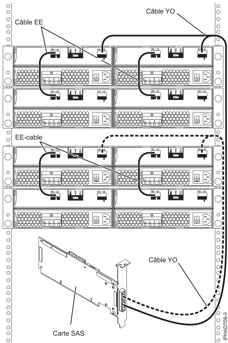
Figure 142. Connexion d'une carte SAS à quatre tiroirs d'extension de disque
