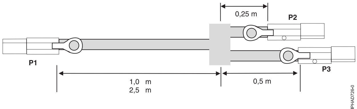
Figure 139. Longueurs de câble d'assemblage de câble YI externe SAS
