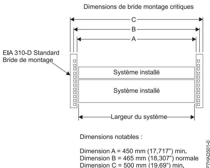
Figure 29. Dimensions critiques des cornières de montage
