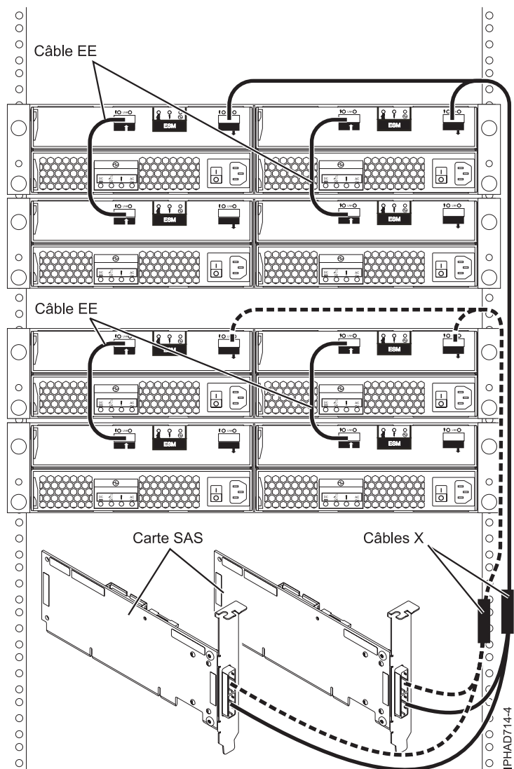
Figure 151. Connexion de deux cartes SAS RAID à quatre tiroirs d'extension de disque dans une configuration RAID haute disponibilité multi-initiateur
