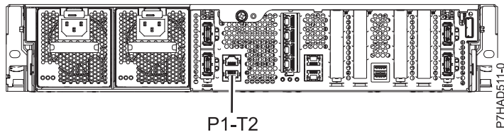
Figure 131. Vue arrière des modèles 8231-E2B, 8231-E1C, 8231-E1D, 8231-E2C, 8231-E2D et 8268-E1D avec l'emplacement d'installation du câble
