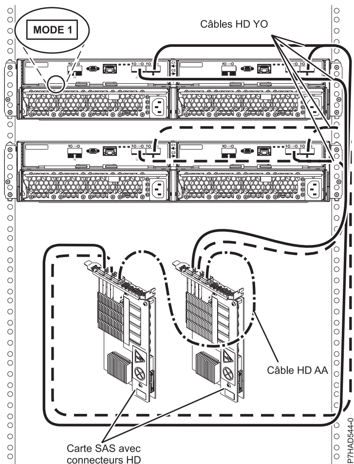
Figure 169. Connexion de mode 1 de deux tiroirs 5887 à deux cartes SAS via des connecteurs HD.
