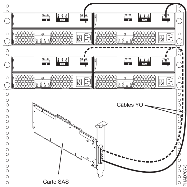
Figure 141. Connexion d'une carte SAS à deux tiroirs d'extension de disque
