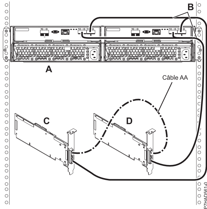
Figure 161. Connexion de mode 2 d'un tiroir 5887 à deux adaptateurs SAS distincts via des câbles YO
