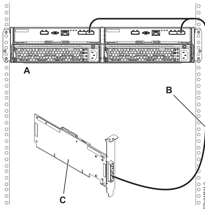
Figure 159. Connexion de mode 1 d'un tiroir 5887 à une carte SAS unique via un câble YO
