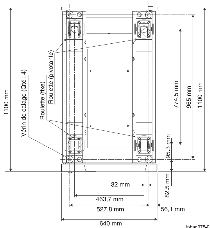
Figure 21. Emplacement des roulettes et des vérins de calage
