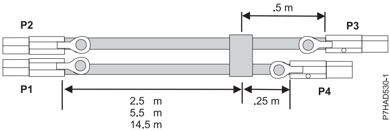
Figure 137. Longueurs de câble d'assemblage de câble X externe SAS
