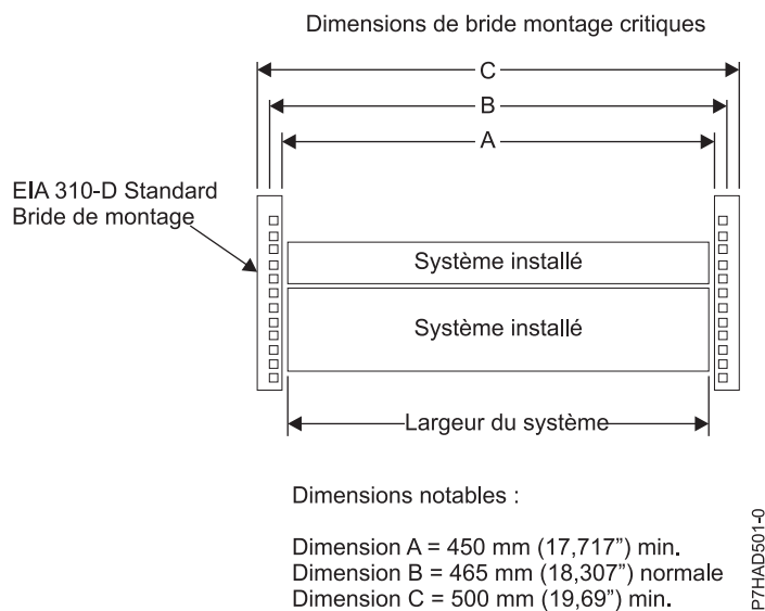
Figure 174. Dimensions critiques des cornières de montage
