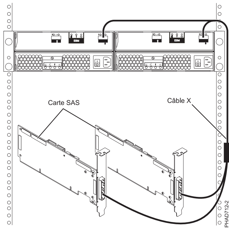
Figure 149. Connexion de deux cartes SAS RAID à un tiroir d'extension de disque dans une configuration RAID haute disponibilité multi-initiateur
