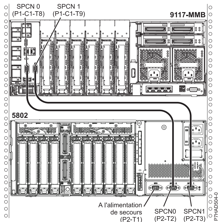
Figure 130. Vue arrière des modèles 8412-EAD, 9117-MMB, 9117-MMC, 9117-MMD, 9179-MHB, 9179-MHC, 9179-MHD et 5208 ou 5877 avec l'emplacement d'installation des câbles
