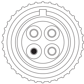
Figure 113. Fiche de type RS 7328DP
