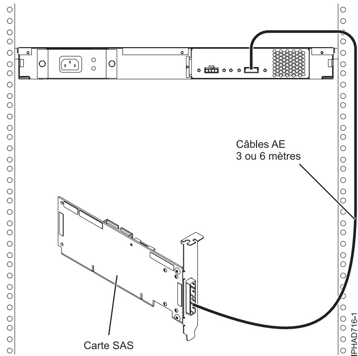
Figure 144. Connexion d'une carte SAS à un tiroir d'extension de stockage
