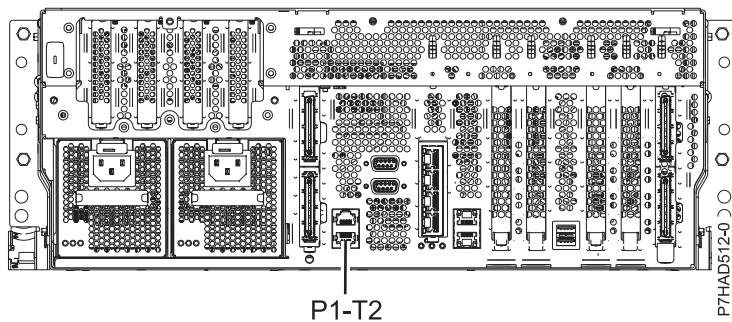
Figure 132. Vue arrière des modèles 8202-E4B, 8202-E4C, 8202-E4D, 8205-E6B, 8205-E6C et 8205-E6D avec l'emplacement d'installation du câble
