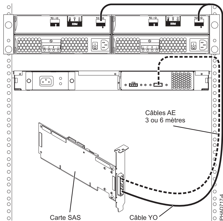
Figure 145. Connexion d'une carte SAS à un tiroir d'extension de disque et un tiroir d'extension de stockage
