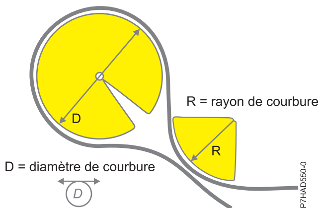
Figure 135. Rayon de courbure du câble
