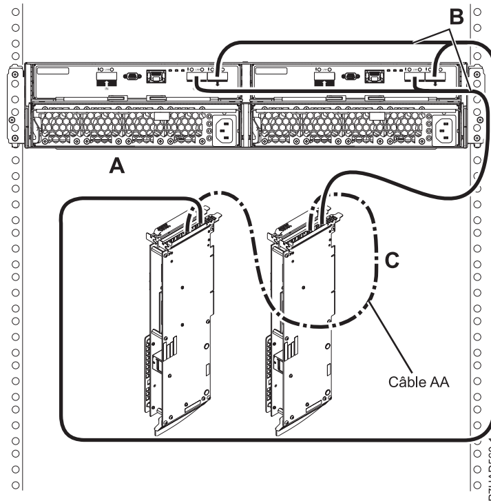
Figure 167. Connexion de mode 1 d'un tiroir 5887 à deux cartes SAS via des câbles YO
