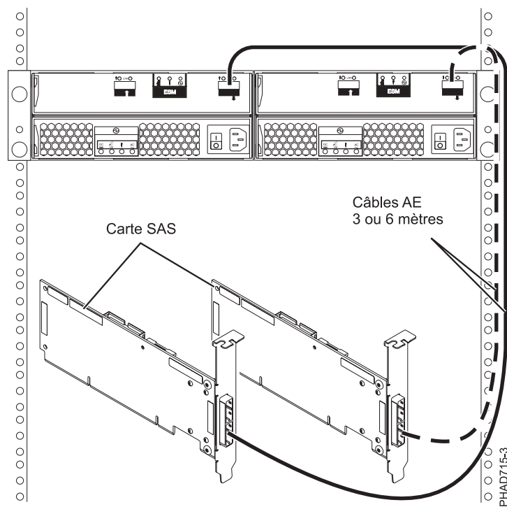
Figure 157. Connexion de deux cartes SAS RAID à un tiroir d'extension de disque dans une configuration JBOD haute disponibilité multi-initiateur
