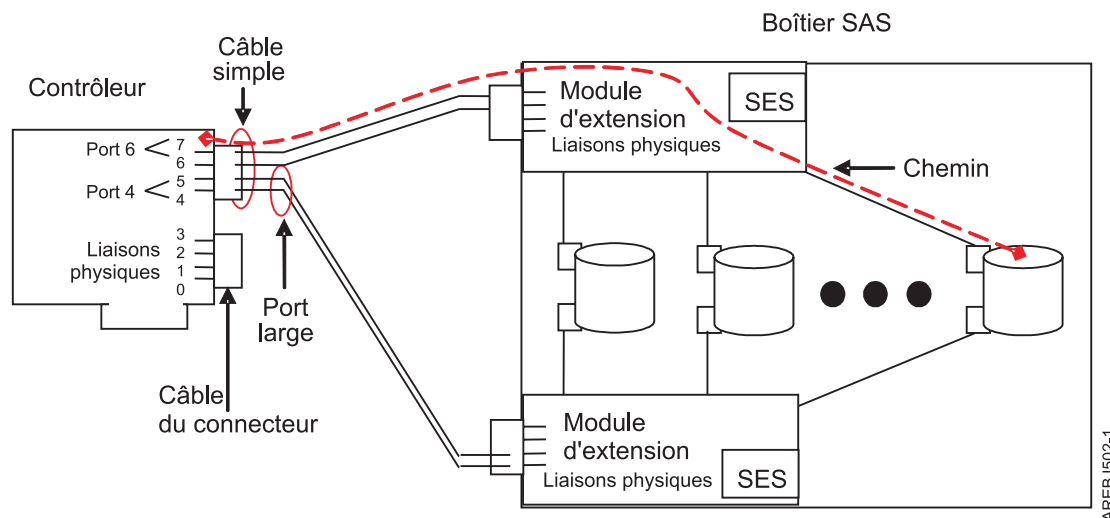
Figure 16. Exemple de sous-système SAS
