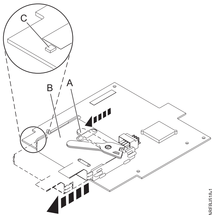
Figure 24. Retrait de la batterie de cache
