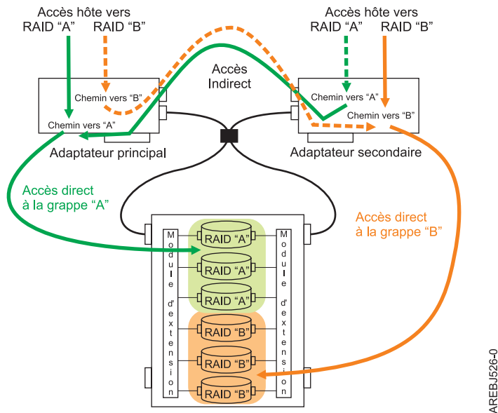
Figure 23. Optimisation des accès à haute disponibilité
