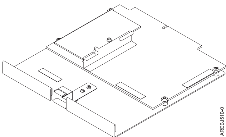
Figure 3. CCIN 57B8 : carte d'activation Planar RAID
