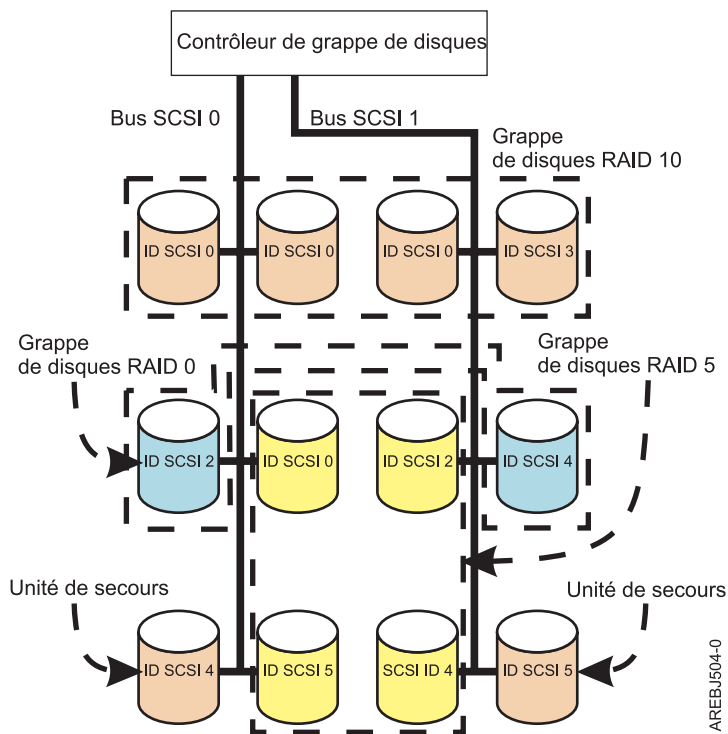
Figure 17. Configuration de grappes de disques
