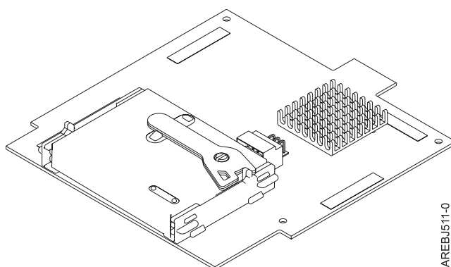
Figure 5. CCIN 57B7 : cache auxiliaire sur carte
