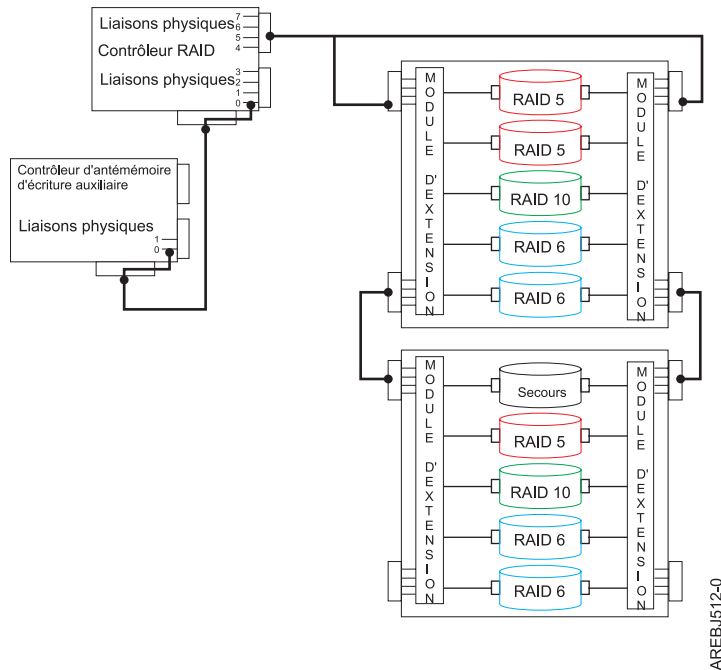
Figure 22. Exemple de configuration des contrôleurs RAID et de cache d'écriture auxiliaire
