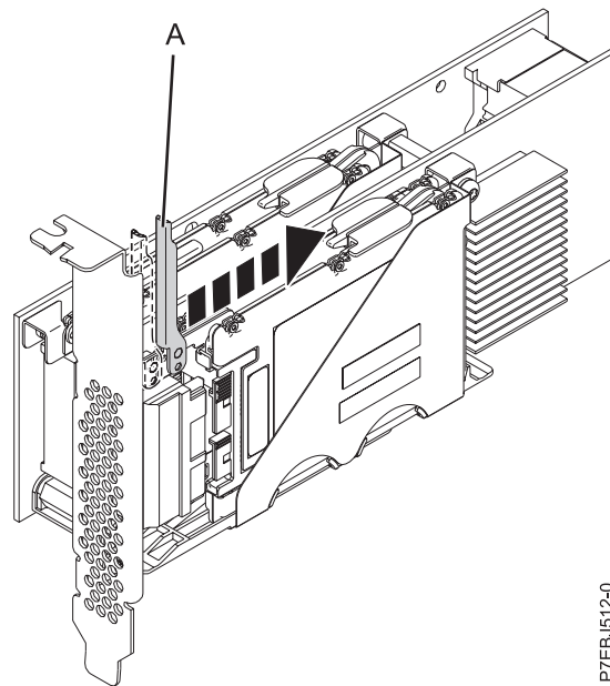
Figure 29. Pousser le levier pour l'écarter de la contre-poupée de la carte
