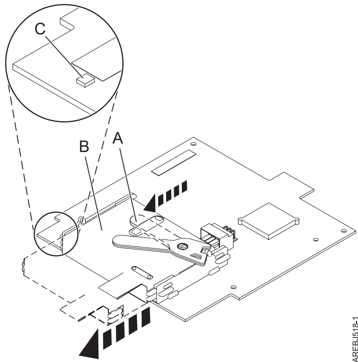
Figure 26. Retrait de la batterie de cache
