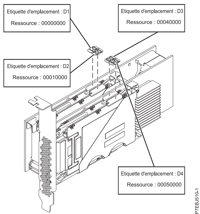
Figure 11. CCIN 57CD - Carte PCIe SAS RAID et SSD 3 Go x8
