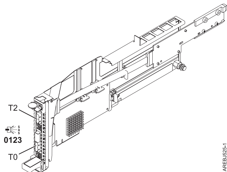
Figure 6. CCIN 57B9 : carte SAS PCI Express x8 Ext Dual-x4 3 Go et carte câble
