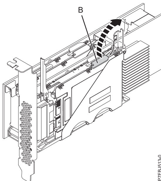
Figure 30. Soulever le taquet de retenue d'unité
