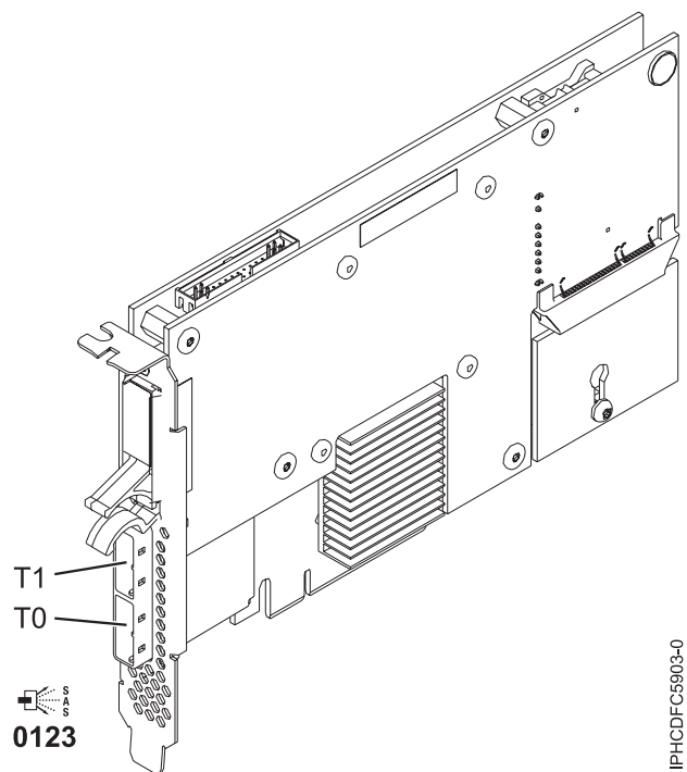
Figure 10. CCIN 574E : carte SAS RAID PCI Express x8 Ext Dual-x4 3 Go
