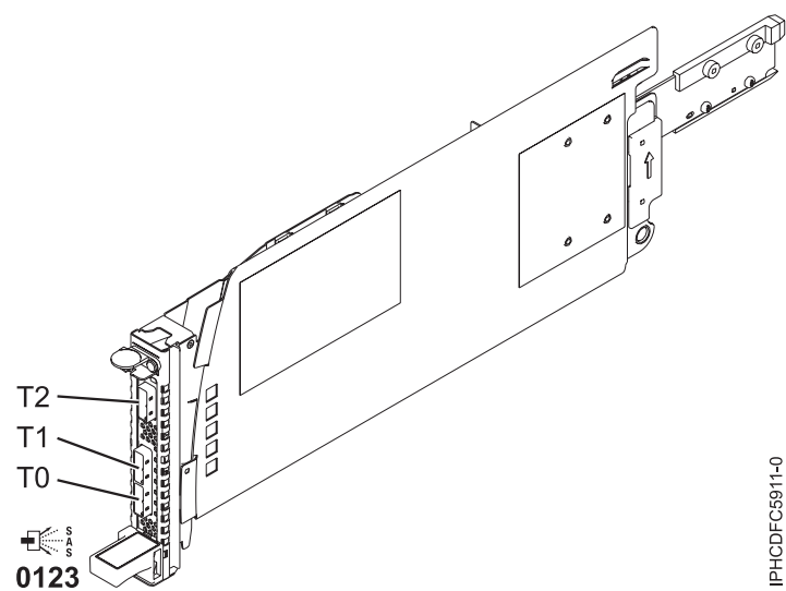
Figure 7. CCIN 57BA : carte SAS PCI Express x8 Ext Dual-x4 3 Go et carte câble
