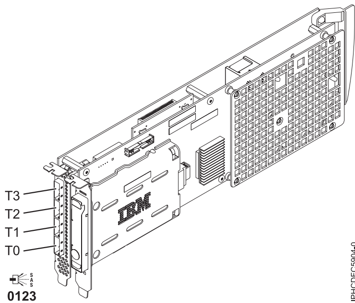
Figure 4. CCIN 572F : carte SAS RAID PCI-X266 Ext Tri-x4 3 Go et CCIN 575C : carte cache auxiliaire PCI-X 266
