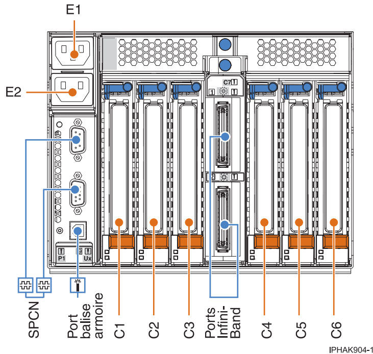
Figure 5. Vue arrière
