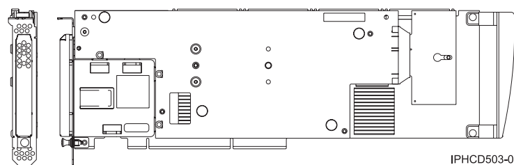
Figura 54. Vista lateral y vista posterior del adaptador
