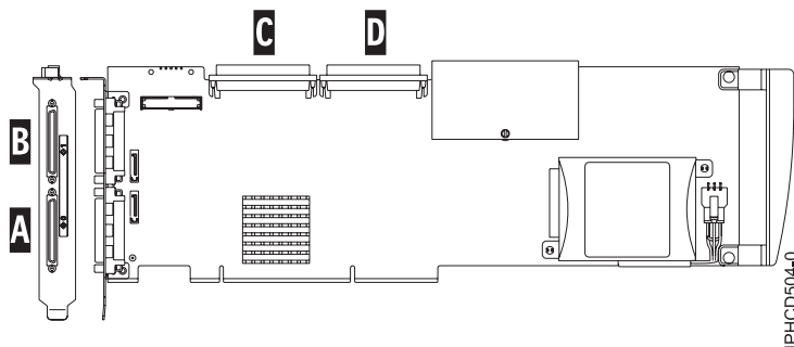
Figura 53. Adaptador PCI-X DDR de canal dual Ultra320 SCSI RAID
