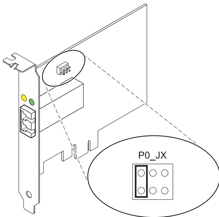
Figura 10. Puente de ID de dispositivo
