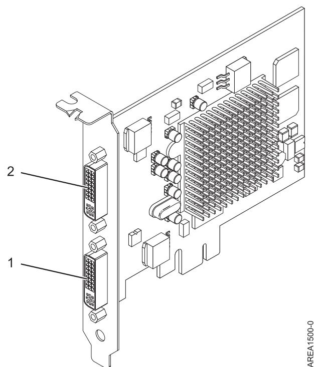
Figura 14. adaptador Acelerador de gráficos PCI Express POWER GXT145
