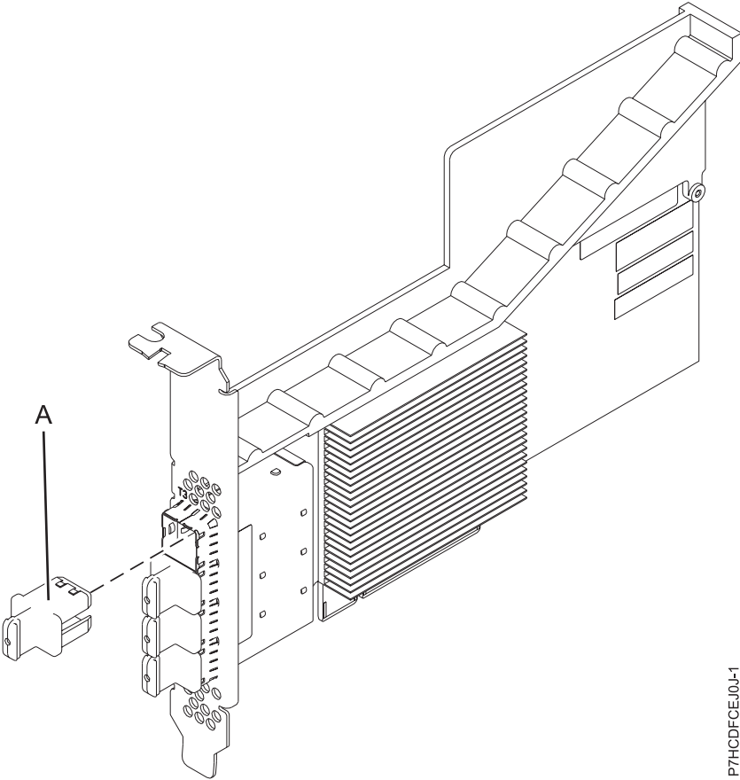
Figura 18. Adaptador de puerto SAS PCIe3 4 x8
