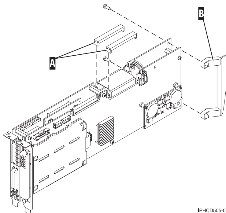
Figura 59. Preparar el adaptador para colocarlo en una casete
