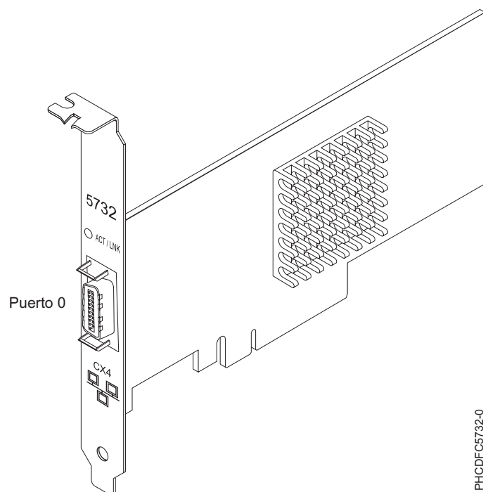
Figura 28. adaptador PCI Express (PCIe) Ethernet-CX4 de 10 gigabits
