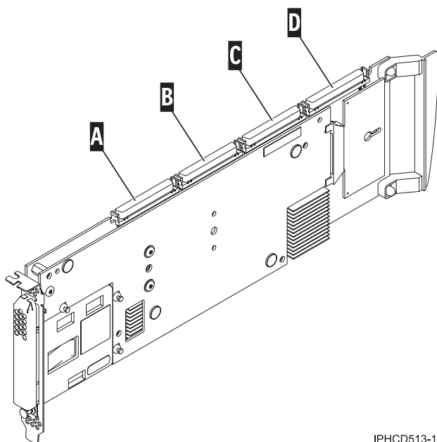
Figura 55. Conectores SCSI del adaptador
