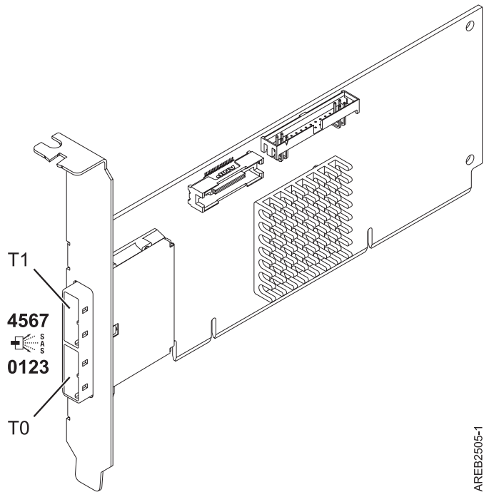
Figura 42. Adaptador SAS PCI-X DDR de puerto dual externo x4
