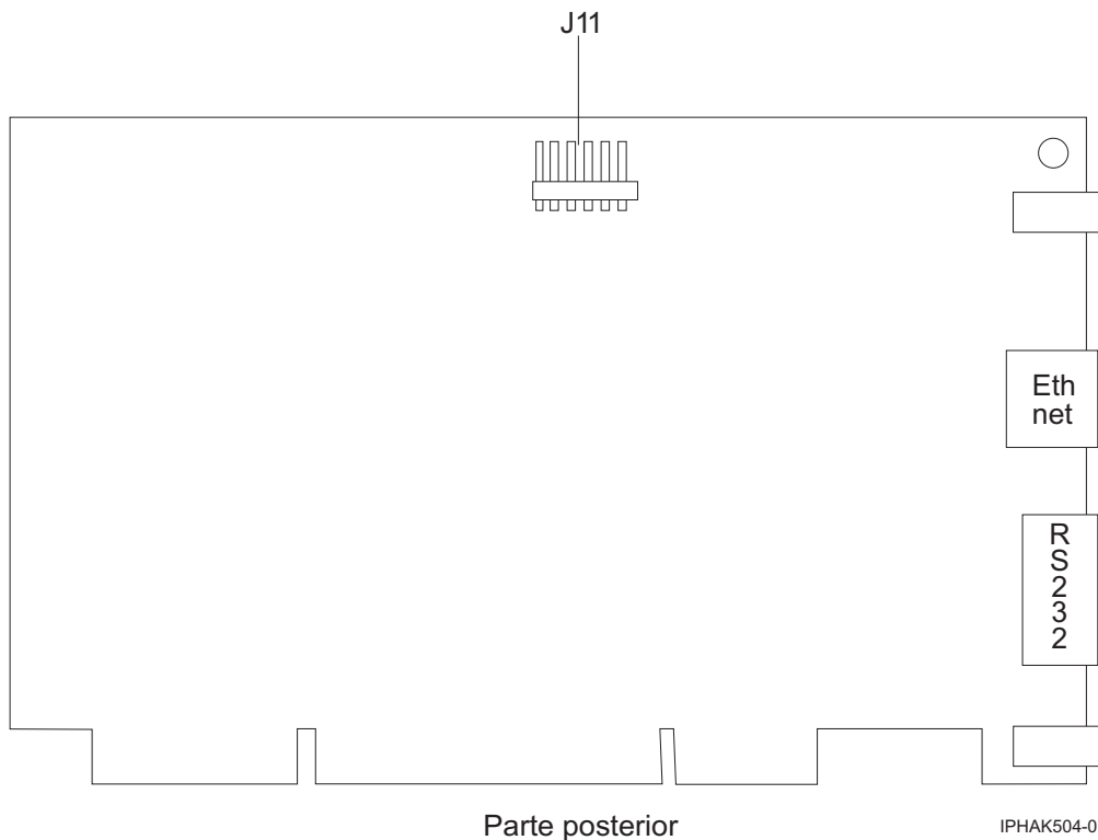
Figura 39. Parte posterior del adaptador
