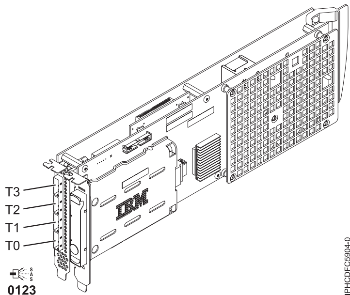
Figura 47. Adaptador RAID SAS PCI-X DDR de memoria caché de 1,5 GB
