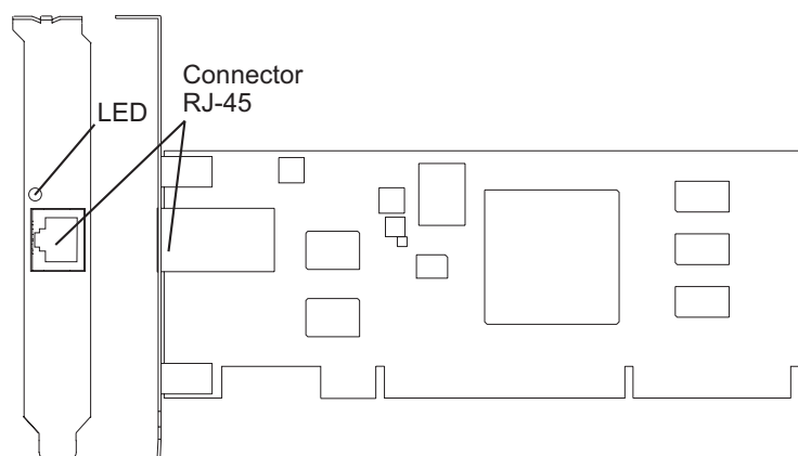
Figura 24. Adaptador PCI-X 1 Gigabit-TX iSCSI TOE
