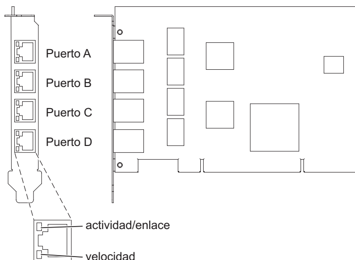
Figura 30. Adaptador PCI-X 4 Puertos 10/100/1000 Base-TX
