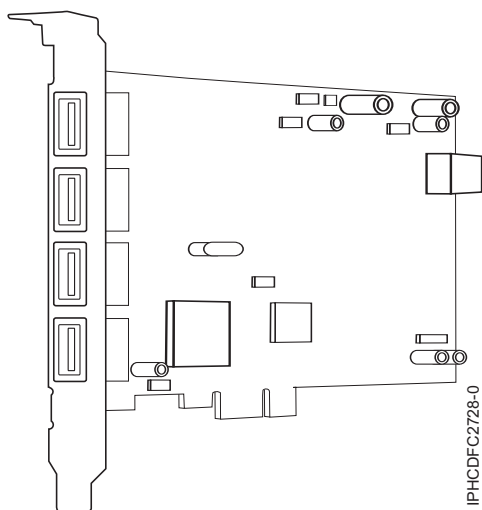
Figura 37. Adaptador PCIe USB de 4 puertos
