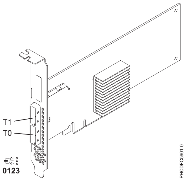
Figura 43. Adaptador PCIe Dual - x4 SAS
