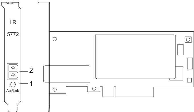
Figura 34. Adaptador PCI Express Ethernet-LR de 10 gigabits
