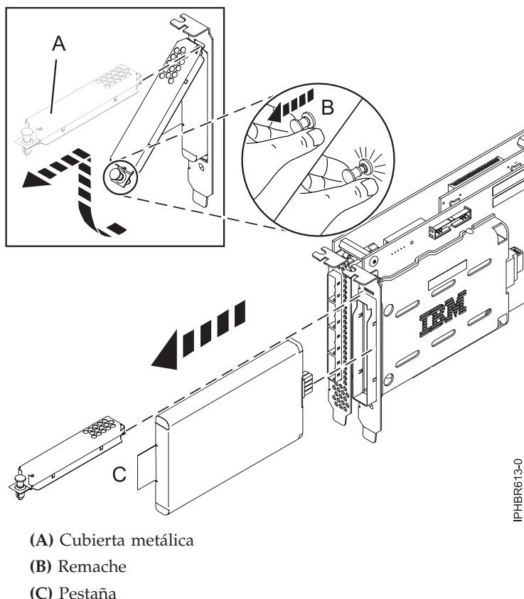
Figura 63. Sustitución de la batería de memoria caché 572F/575C
