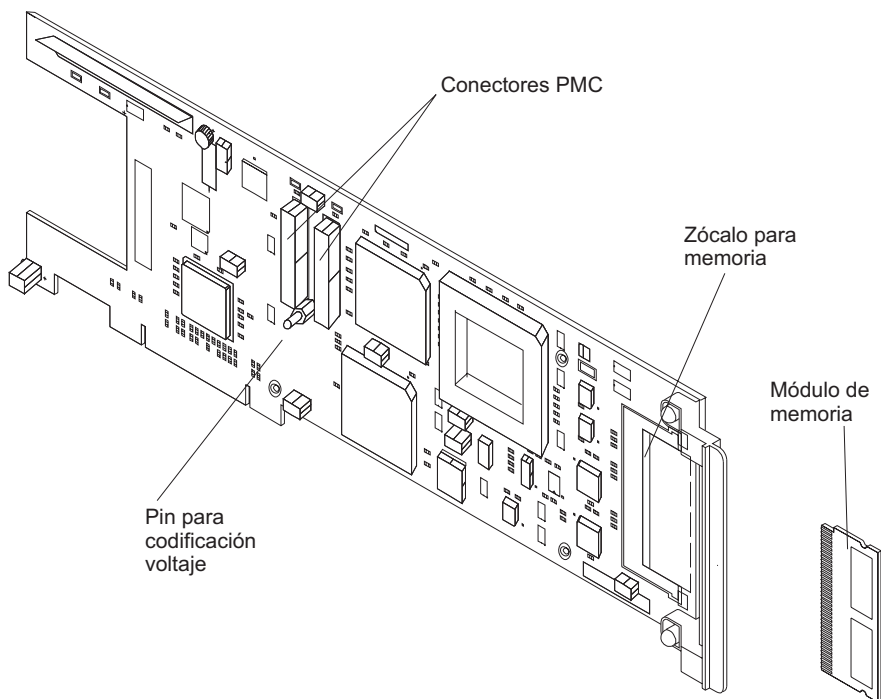
Figura 60. Adaptador PCI base ARTIC960Hx de IBM
