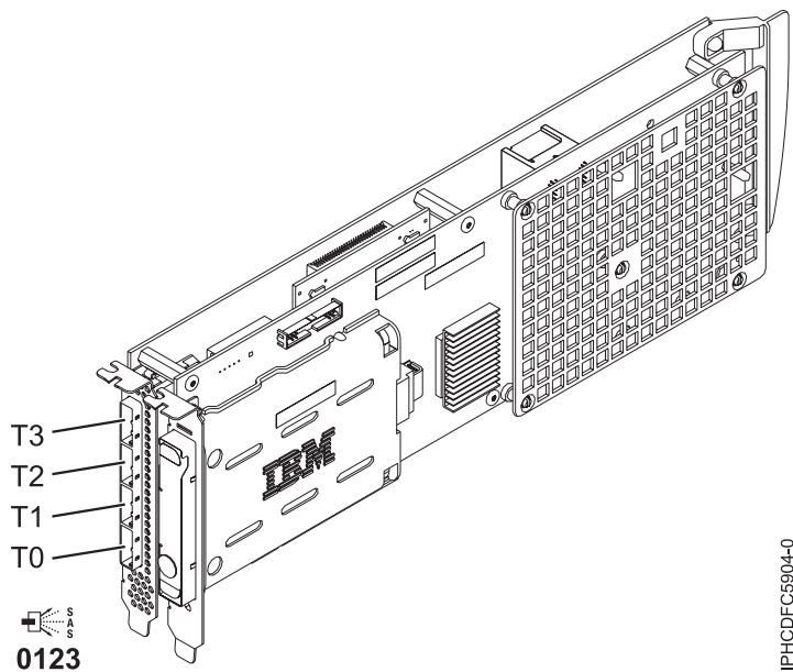
Figura 46. Adaptador SAS RAID PCI-X DDR de memoria caché de 1,5 GB
