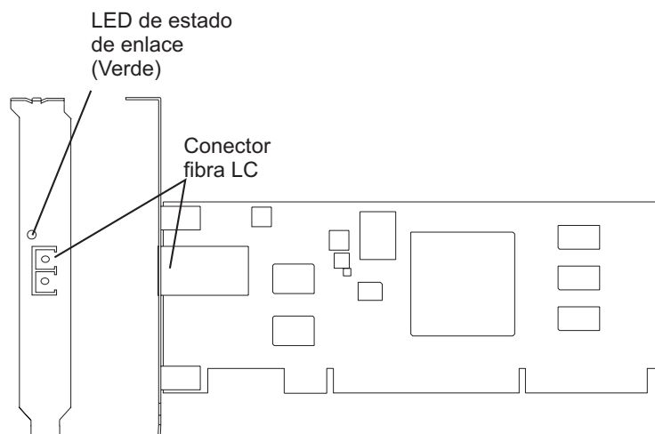
Figura 23. Adaptador PCI-X 1 Gigabit-SX iSCSI TOE
