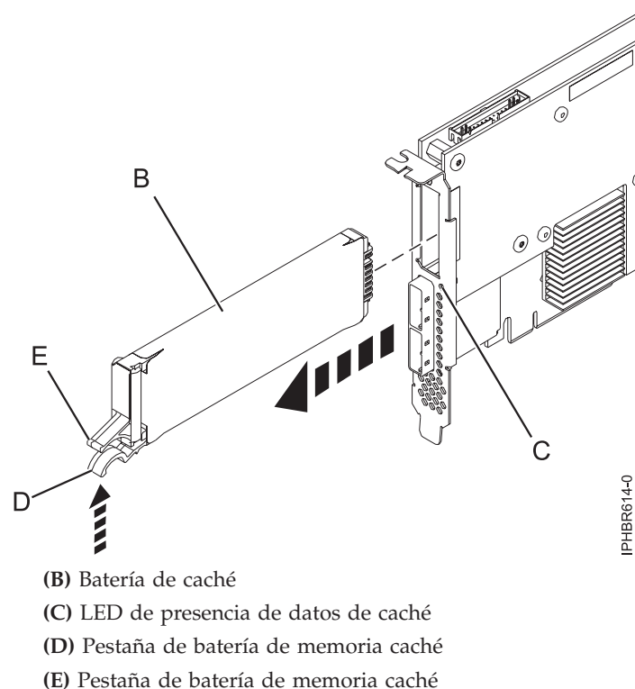
Figura 66. Sustitución de la batería de memoria caché 574E
