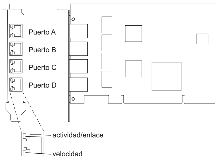
Figura 29. Adaptador PCI-X 4 Puertos 10/100/1000 Base-TX
