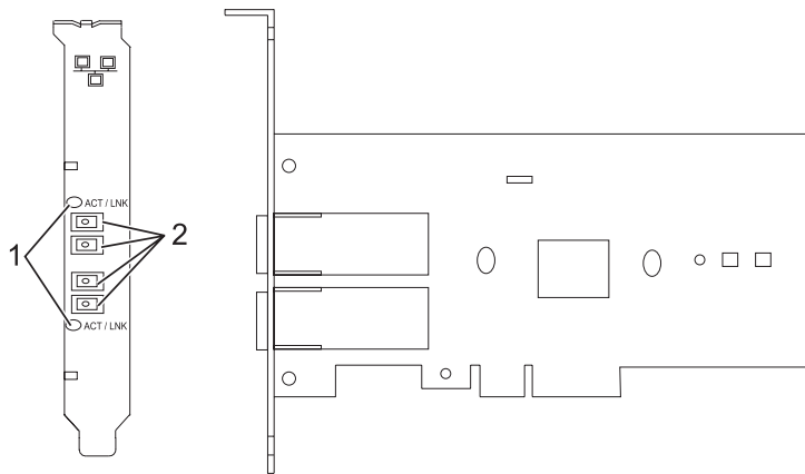
Figura 32. Adaptador PCI Express Gigabit Ethernet-SX de 2 puertos
