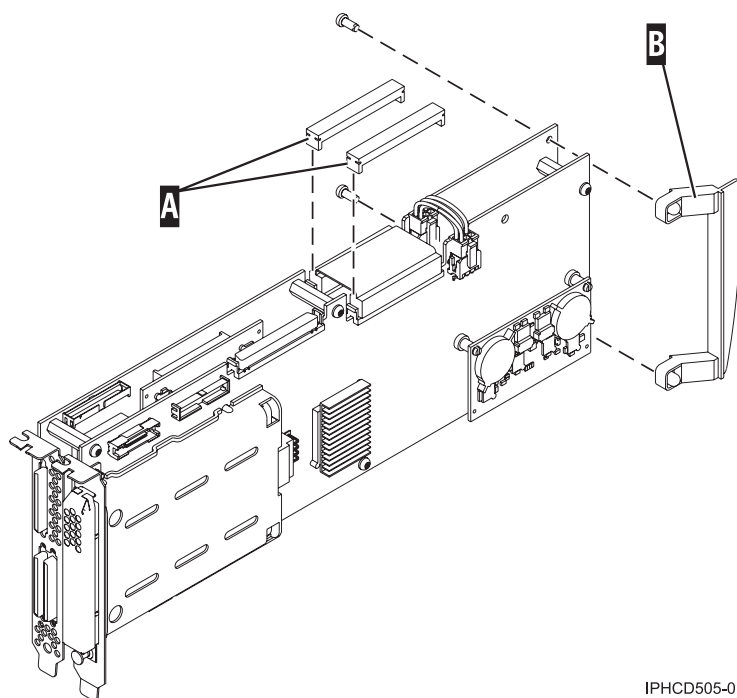
Figura 57. Preparar el adaptador para colocarlo en una casete
