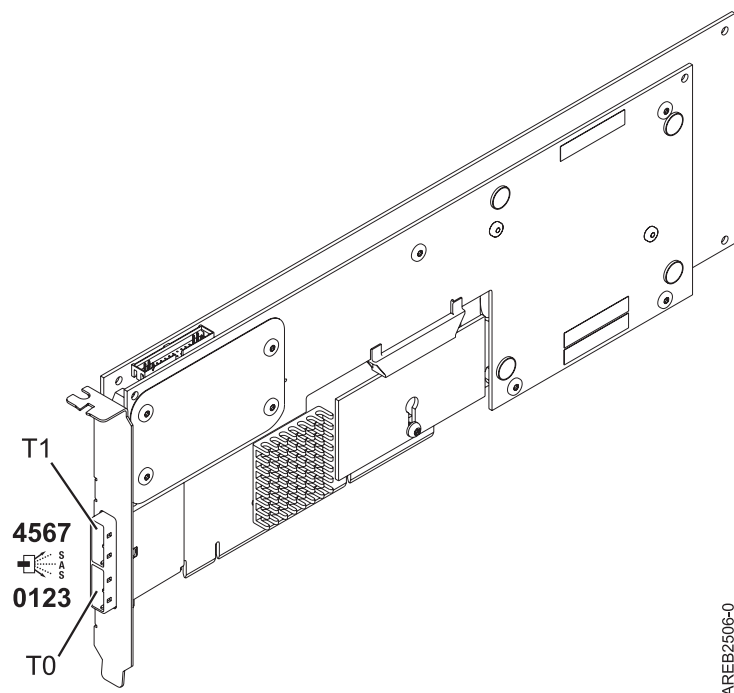
Figura 44. adaptador RAID SAS PCI-X DDR de puerto dual x4
