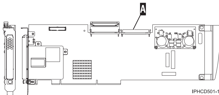
Figura 52. IOA de caché de escritura auxiliar
