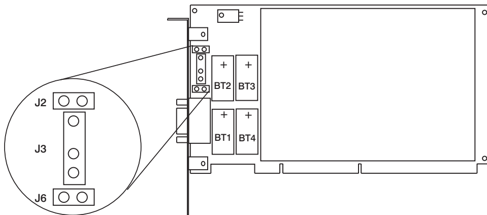
Figura 40. Sustituir las baterías del coprocesador
