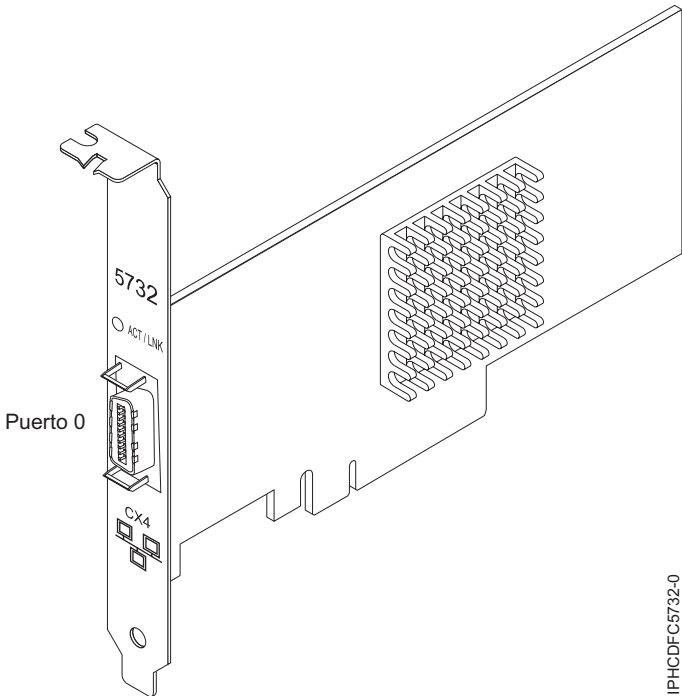
Figura 52. adaptador PCI Express (PCIe) Ethernet-CX4 de 10 gigabits
