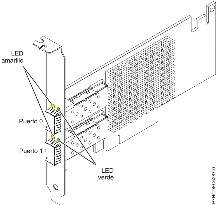
Figura 40. adaptador PCIe2 LP de 2 puertos 10GbE SR
