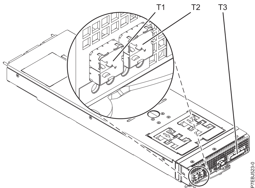
Figura 106. Alojamiento PCIe2 SAS RAID de memoria caché de 3,1GB 6Gb x8
