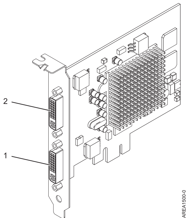
Figura 23. adaptador de Acelerador de gráficos PCIe LP POWER GXT145
