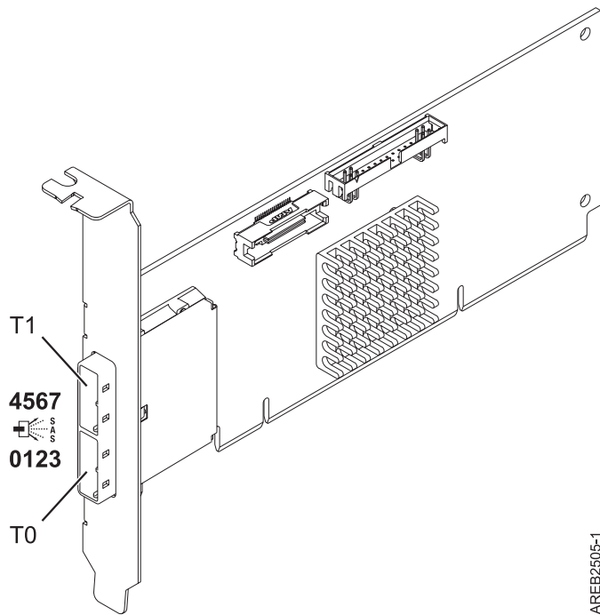
Figura 90. Adaptador SAS PCI-X DDR de puerto dual externo x4
