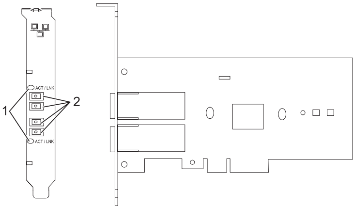
Figura 34. Adaptador PCIe LP de 2 puertos 1GbE SX
