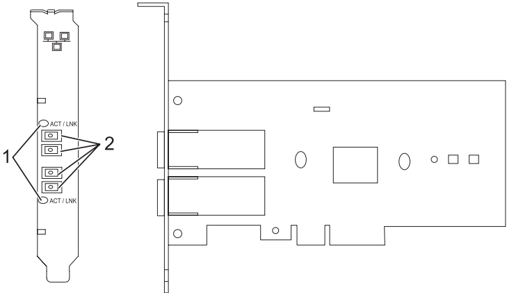
Figura 59. Adaptador PCI Express Gigabit Ethernet-SX de 2 puertos
