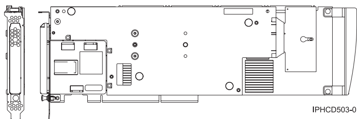
Figura 94. Vista lateral y vista posterior del adaptador
