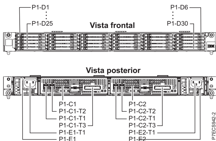
Figura 105. Códigos de ubicación de Adaptador PCIe2 RAID SAS integrado con memoria caché de 3,1GB
