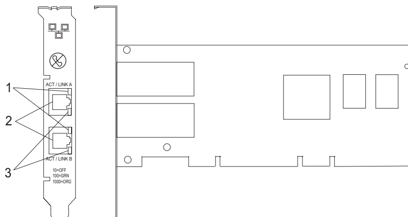
Figura 45. Adaptador PCI-X 10/100/1000 Base-TX Ethernet de 2 puertos
