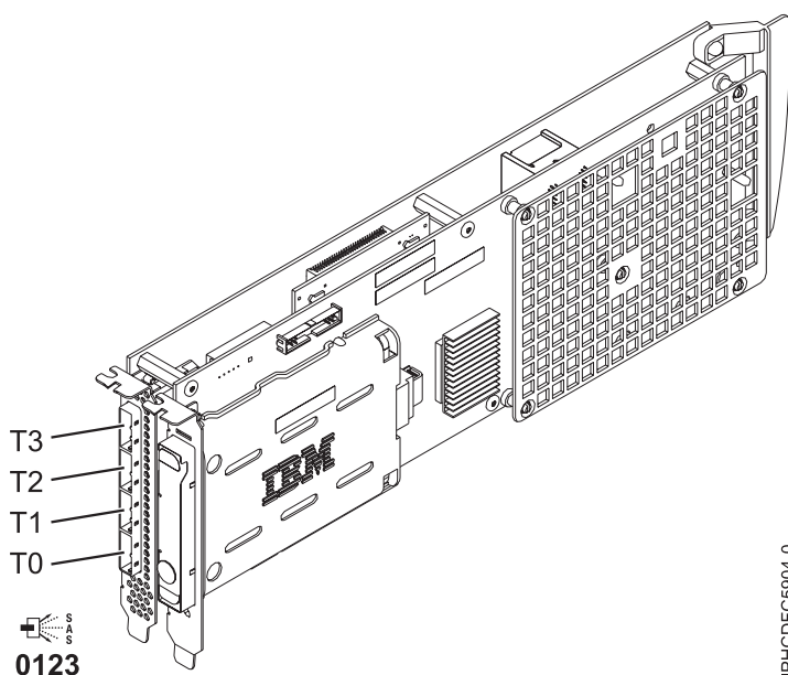
Figura 89. Adaptador RAID SAS PCI-X DDR de memoria caché de 1,5 GB
