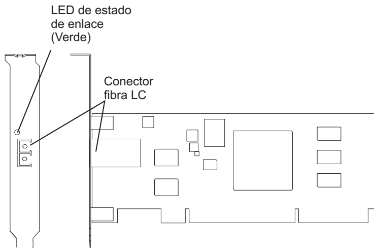
Figura 47. Adaptador PCI-X 1 Gigabit-SX iSCSI TOE
