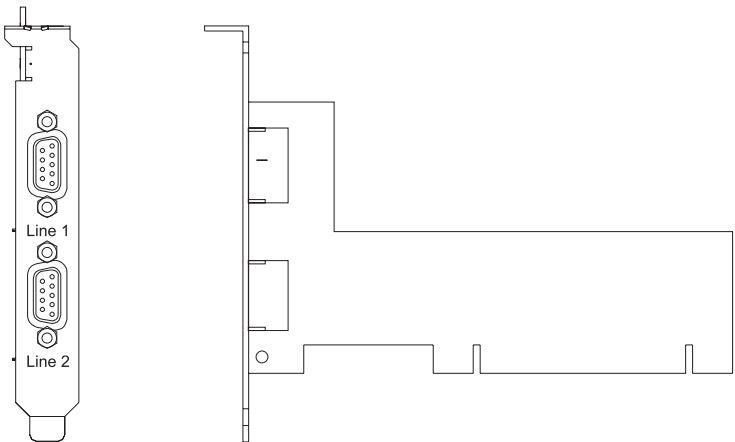
Figura 7. Adaptador PCI asíncrono EIA-232 de 2 puertos
