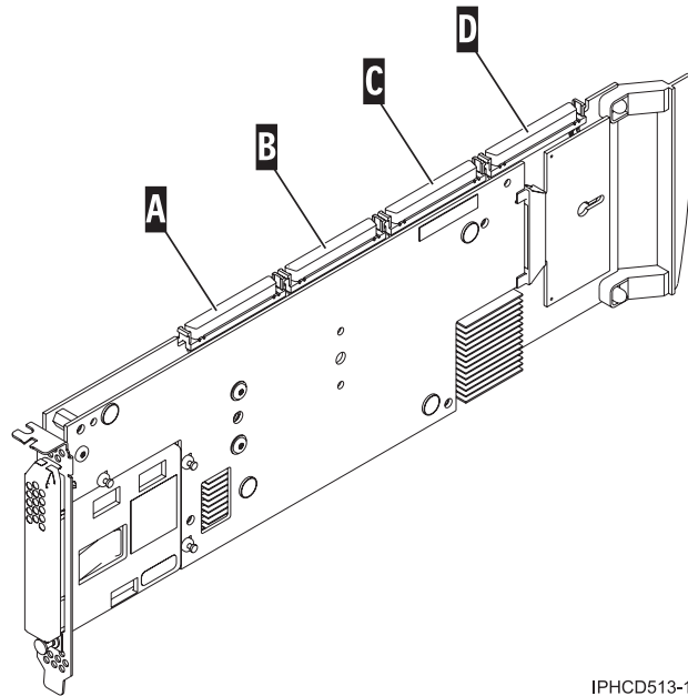
Figura 98. Conectores SCSI del adaptador
