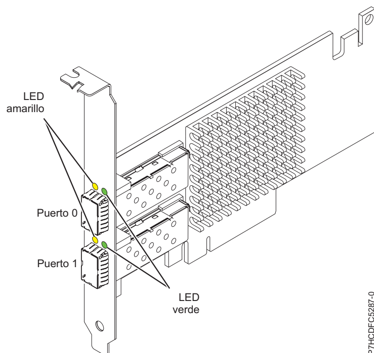
Figura 42. adaptador PCIe2 de 2 puertos 10GbE SR
