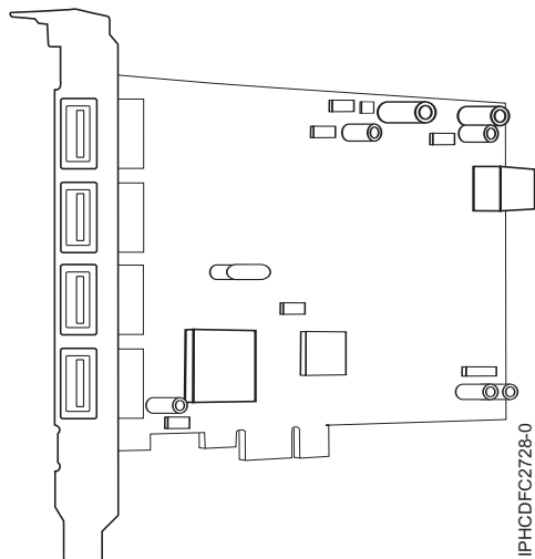
Figura 77. Adaptador PCIe USB de 4 puertos
