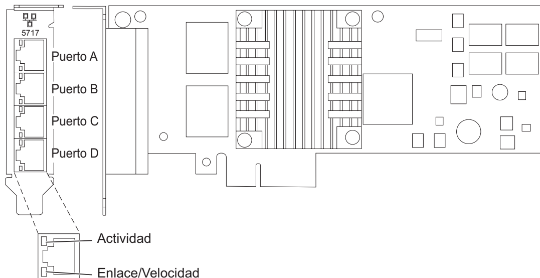
Figura 51. Adaptador PCIe 4 Puertos 10/100/1000 Base-TX
