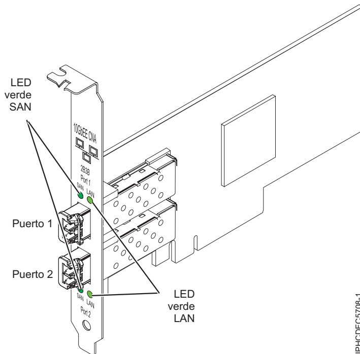
Figura 31. adaptador PCIe LP 10-Gb FCoE de 2 puertos
