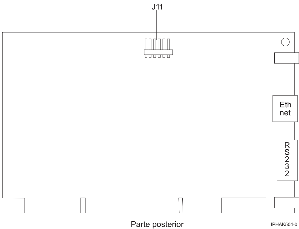
Figura 79. Parte posterior del adaptador
