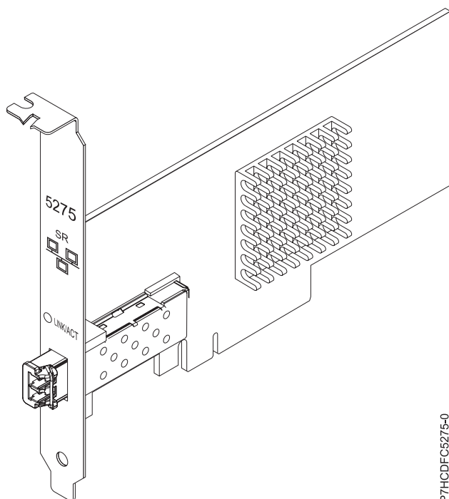
Figura 35. adaptador PCIe LP 10GbE SR de 1 puerto
