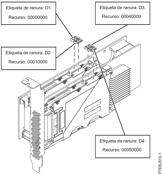
Figura 82. Adaptador RAID SAS PCIe Dual - x4 de 3 Gb
