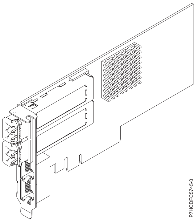
Figura 36. Adaptador PCIe2 LP 2x10GbE SFP+ de cobre y cable de par trenzado no apantallado
