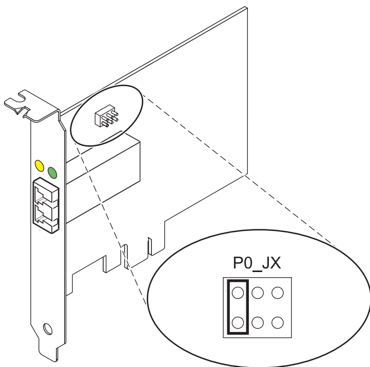
Figura 16. Puente de ID de dispositivo
