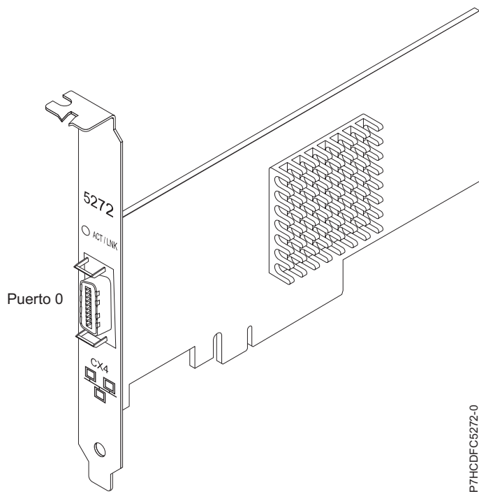
Figura 33. adaptador PCIe LP 10GbE CX4 de 1 puerto
