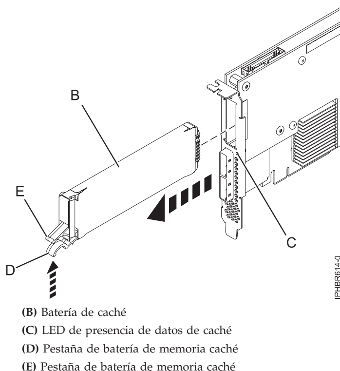
Figura 112. Sustitución de la batería de memoria caché 574E
