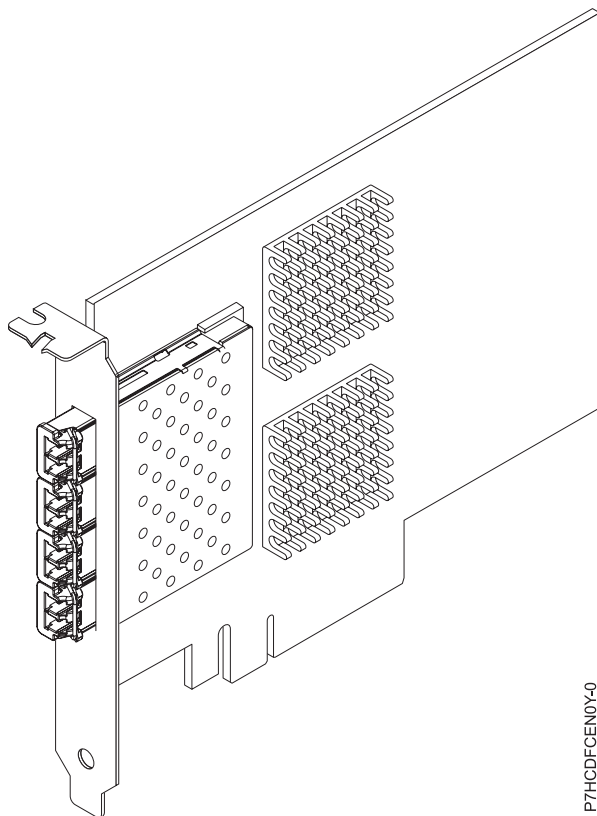
Figura 21. adaptador de canal de fibra PCIe2 LP 8 gigabits de 4 puertos
