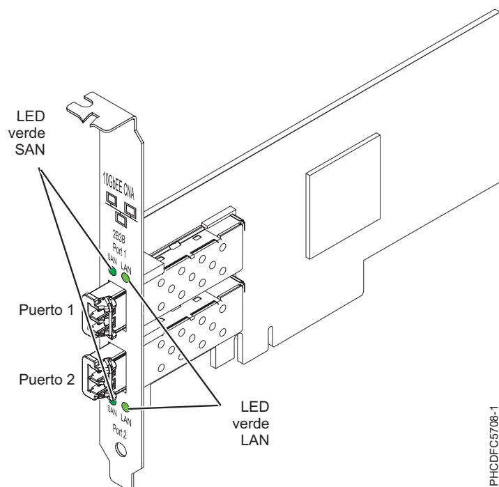
Figura 46. adaptador PCIe de puerto dual FCoE de 10 Gb
