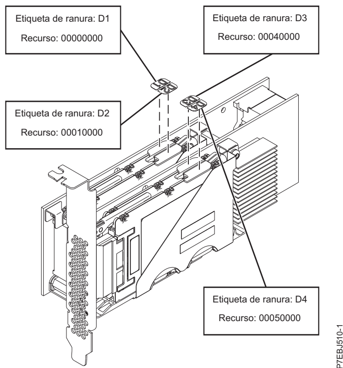
Figura 81. Adaptador RAID SAS PCIe Dual - x4 de 3 Gb
