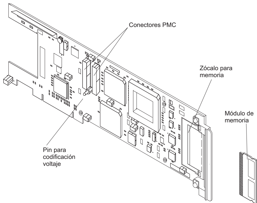
Figura 103. Adaptador PCI base ARTIC960Hx de IBM
