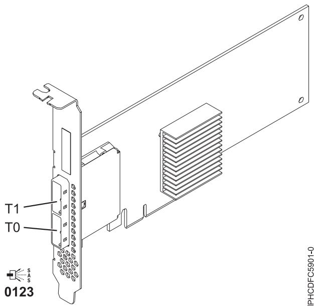
Figura 83. Adaptador PCIe Dual - x4 SAS
