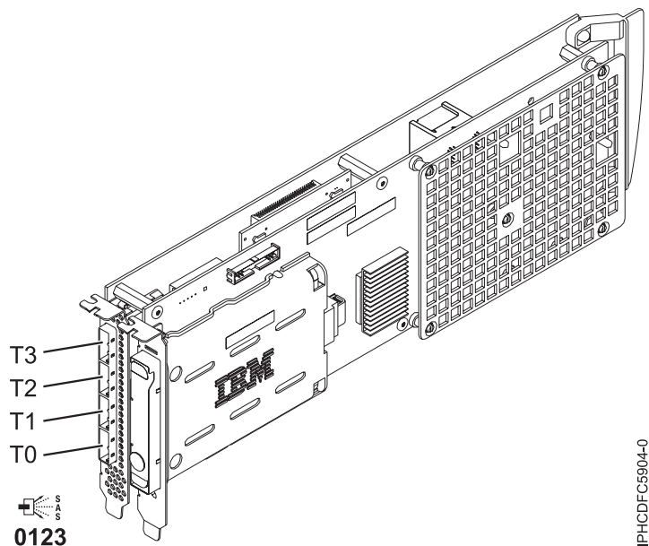
Figura 88. Adaptador SAS RAID PCI-X DDR de memoria caché de 1,5 GB
