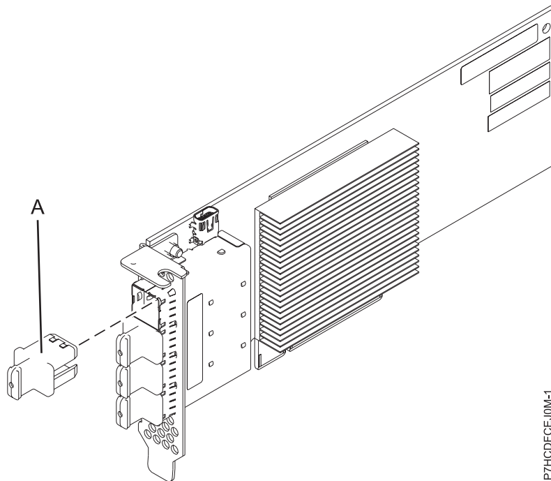
Figura 27. Adaptador PCIe3 SAS RAID de altura reducida y cuatro puertos de 6 Gb
