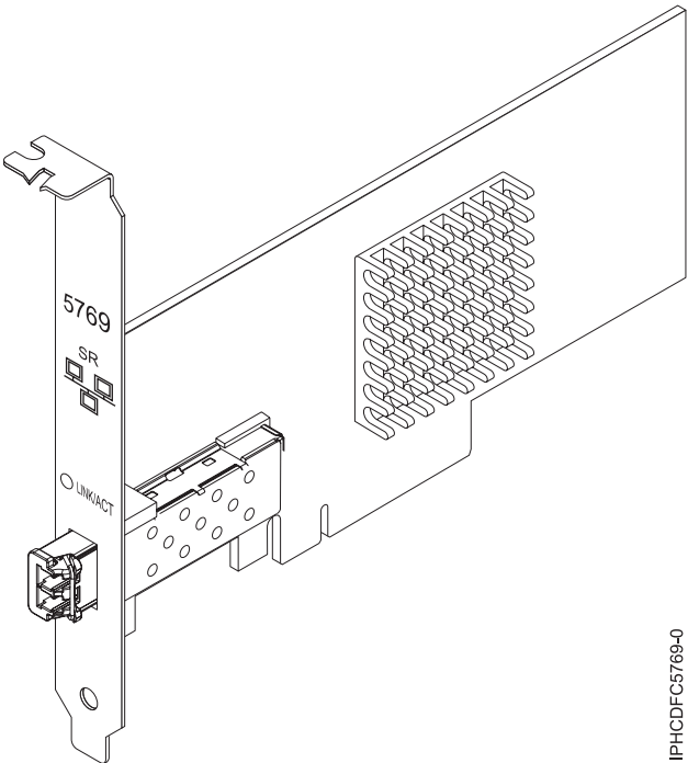
Figura 60. adaptador PCIe Ethernet-SR 10 Gigabit
