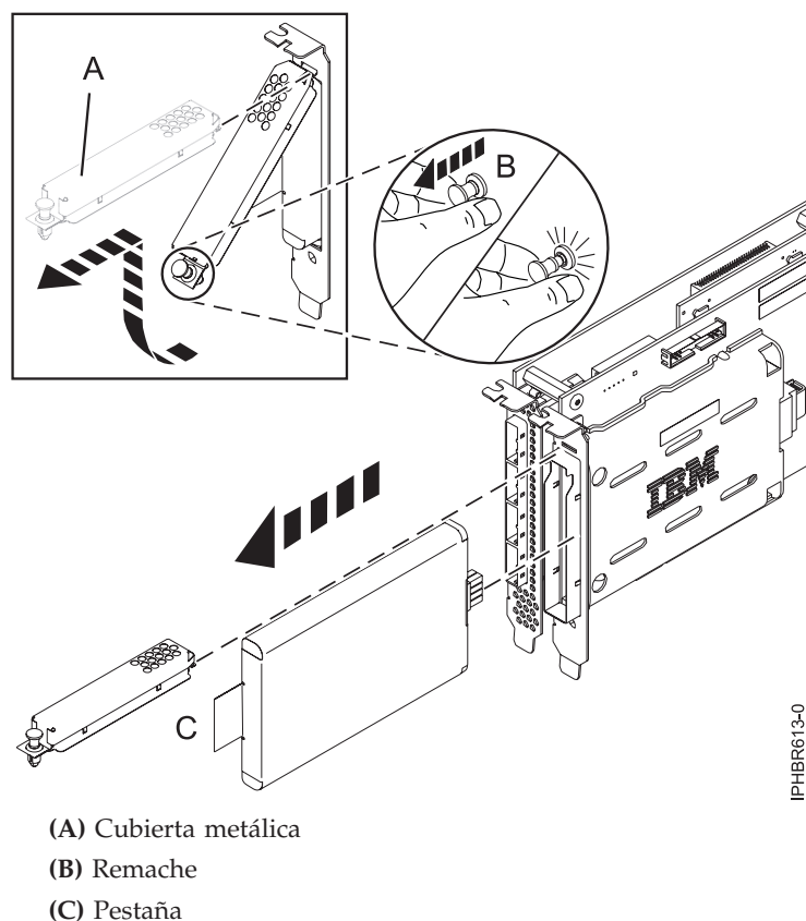
Figura 109. Sustitución de la batería de memoria caché 572F/575C
