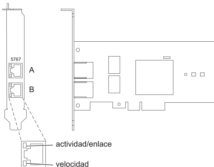
Figura 63. adaptador PCIe de 2 puertos 1GbE TX
