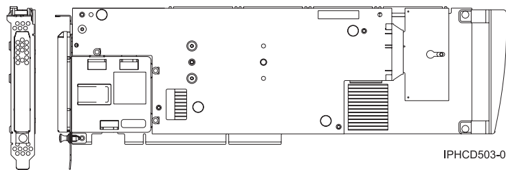
Figura 97. Vista lateral y vista posterior del adaptador
