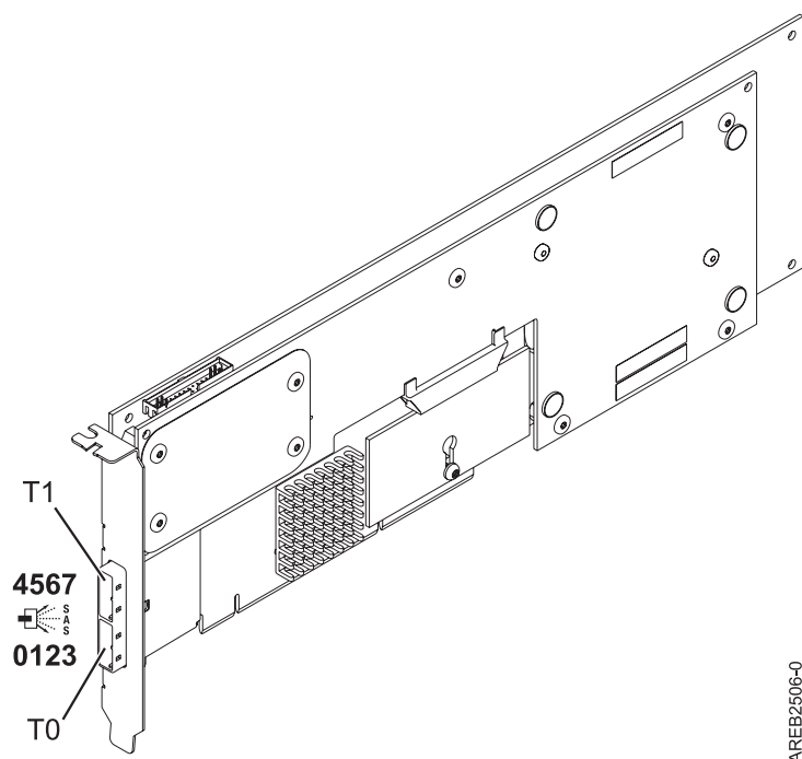
Figura 86. adaptador RAID SAS PCI-X DDR de puerto dual x4
