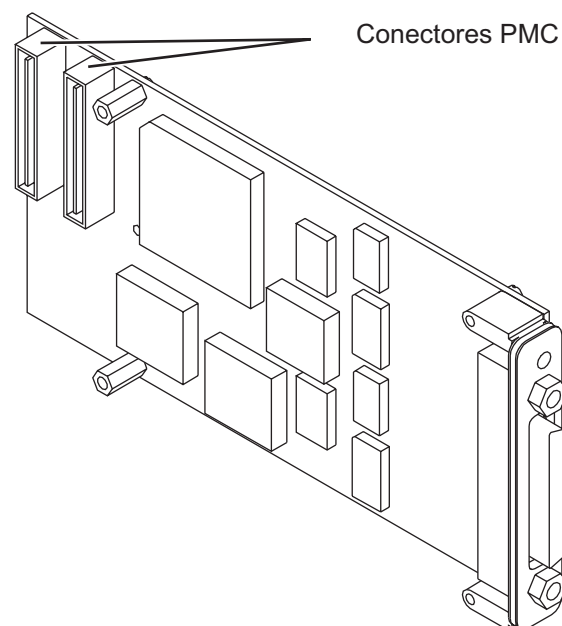
Figura 104. PMC de 4 puertos seleccionables
