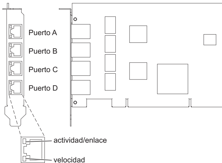
Figura 53. Adaptador PCI-X 4 Puertos 10/100/1000 Base-TX
