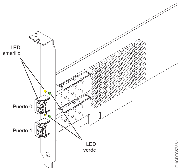
Figura 6. Adaptador 5273
