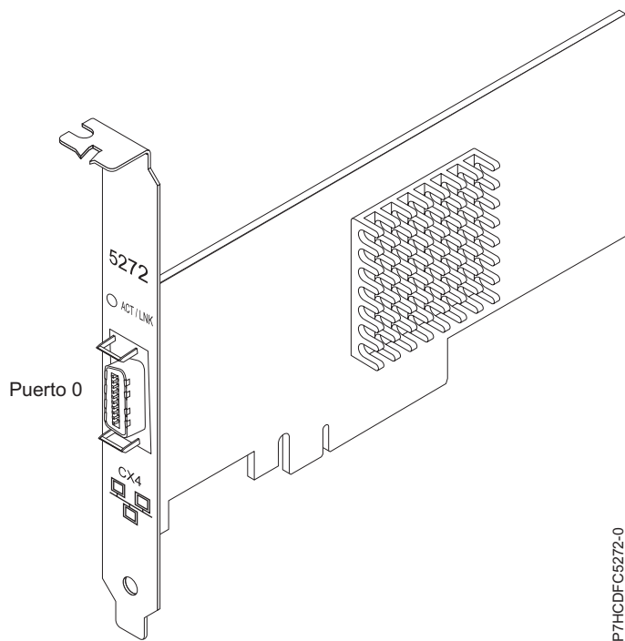
Figura 26. adaptador PCIe LP 10GbE CX4 de 1 puerto
