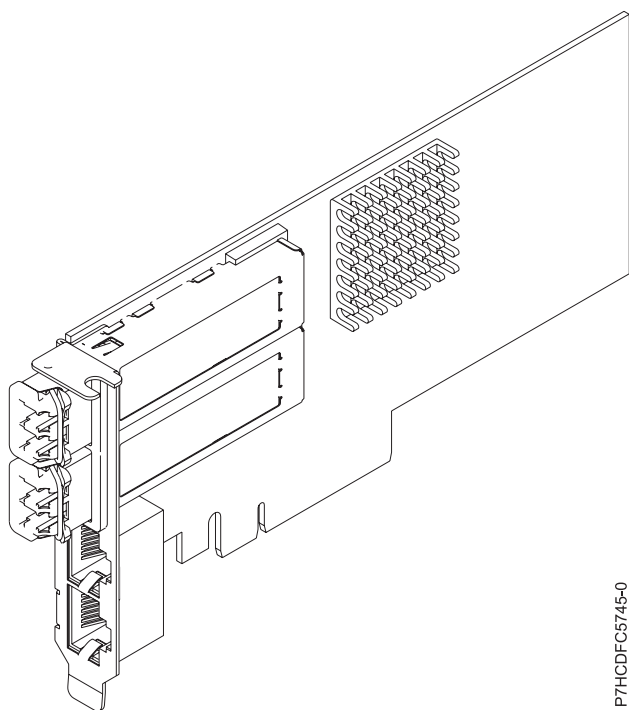
Figura 46. Adaptador EN0L
