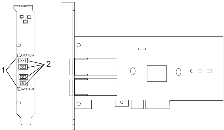
Figura 27. Adaptador PCIe LP de 2 puertos 1GbE SX
