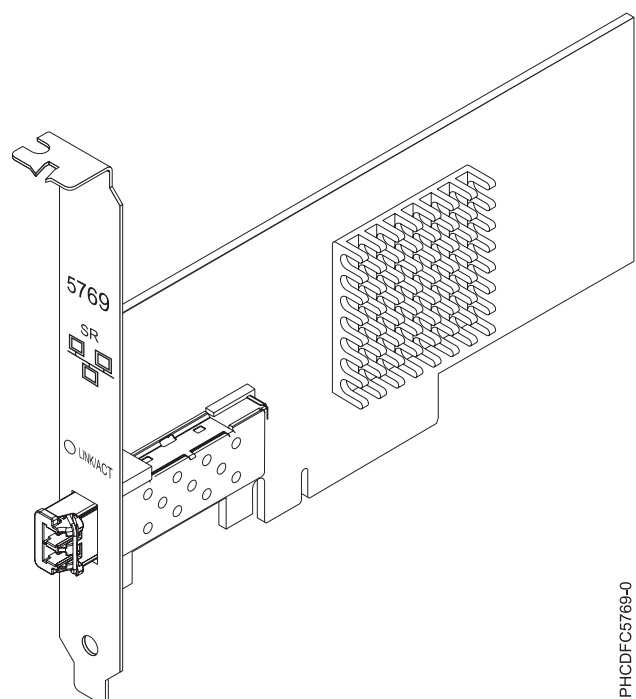
Figura 40. adaptador PCIe Ethernet-SR 10 Gigabit
