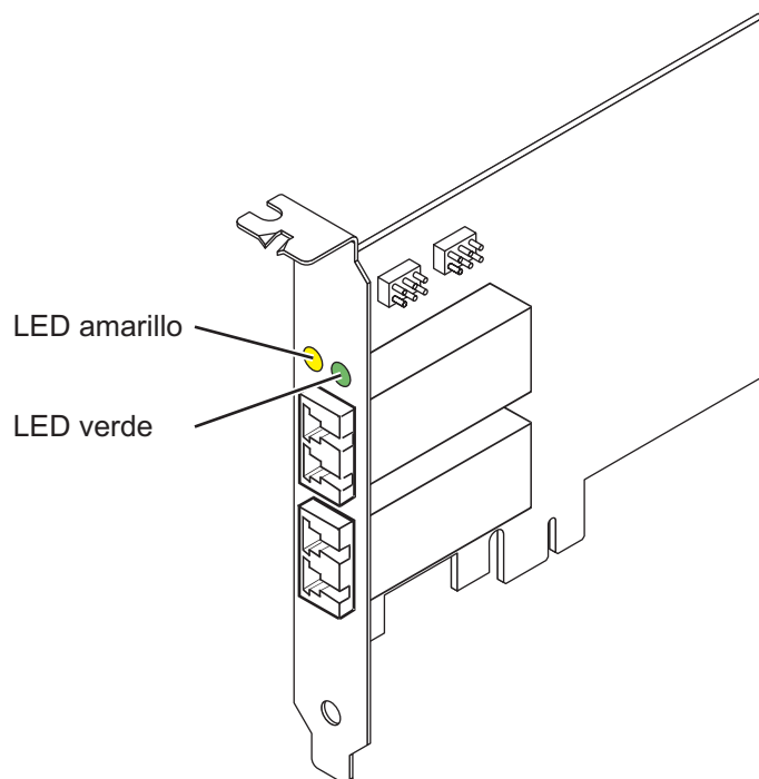
Figura 7. Adaptador 5276
