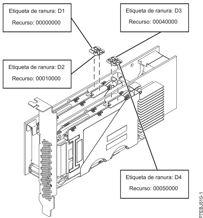
Figura 52. Adaptador RAID SAS PCIe Dual - x4 de 3 Gb
