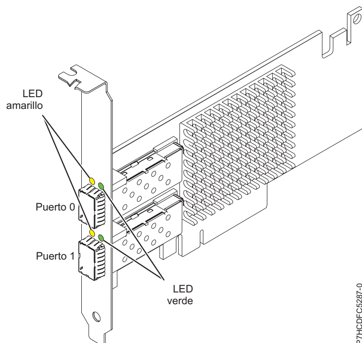
Figura 33. adaptador PCIe2 LP de 2 puertos 10GbE SR
