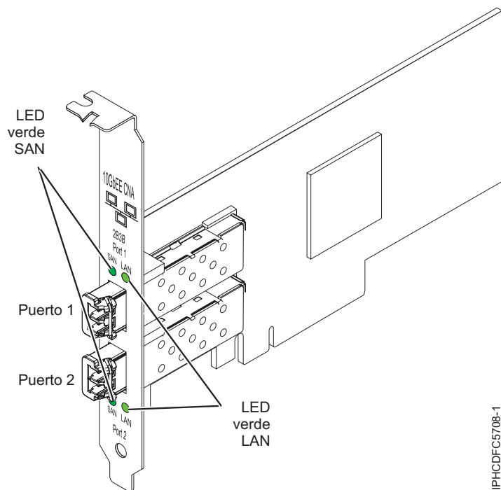
Figura 24. adaptador PCIe LP 10-Gb FCoE de 2 puertos
