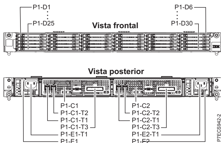
Figura 57. Códigos de ubicación de Adaptador PCIe2 RAID SAS integrado con memoria caché de 3,1GB
