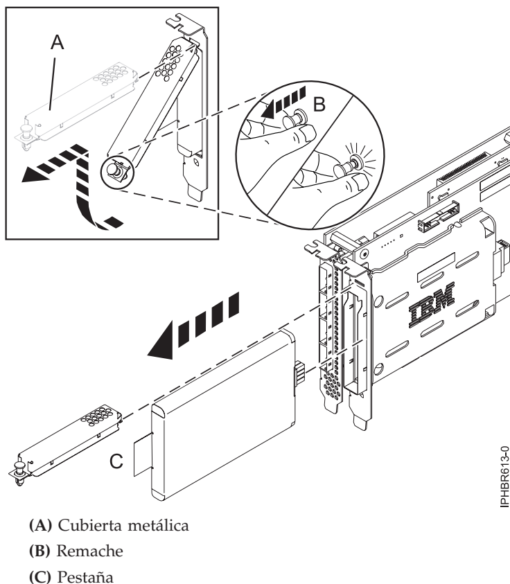
Figura 61. Sustitución de la batería de memoria caché 572F/575C
