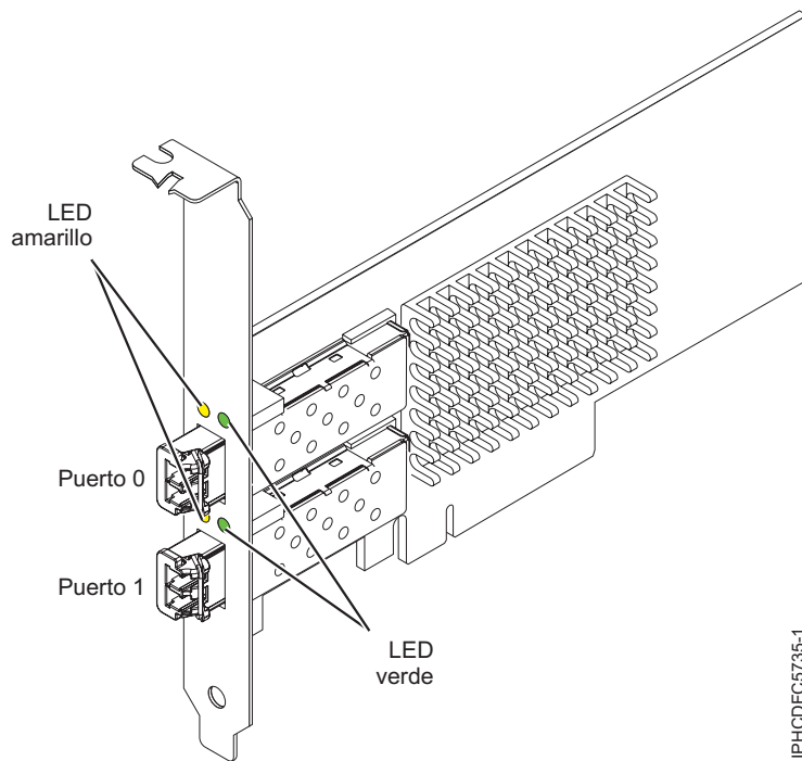
Figura 9. Adaptador EN0B
