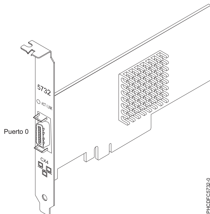
Figura 37. adaptador PCI Express (PCIe) Ethernet-CX4 de 10 gigabits
