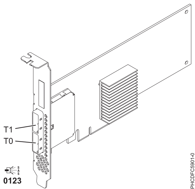
Figura 53. Adaptador PCIe Dual - x4 SAS
