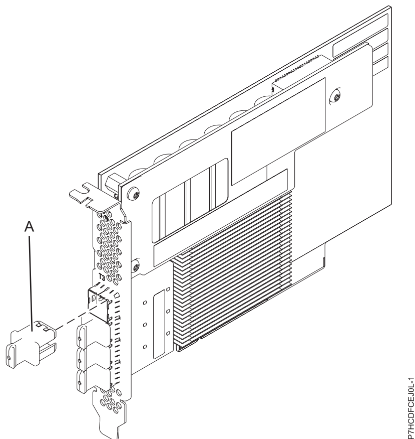
Figura 19. Adaptador PCIe3 12 GB Caché RAID SAS 6 Gb
