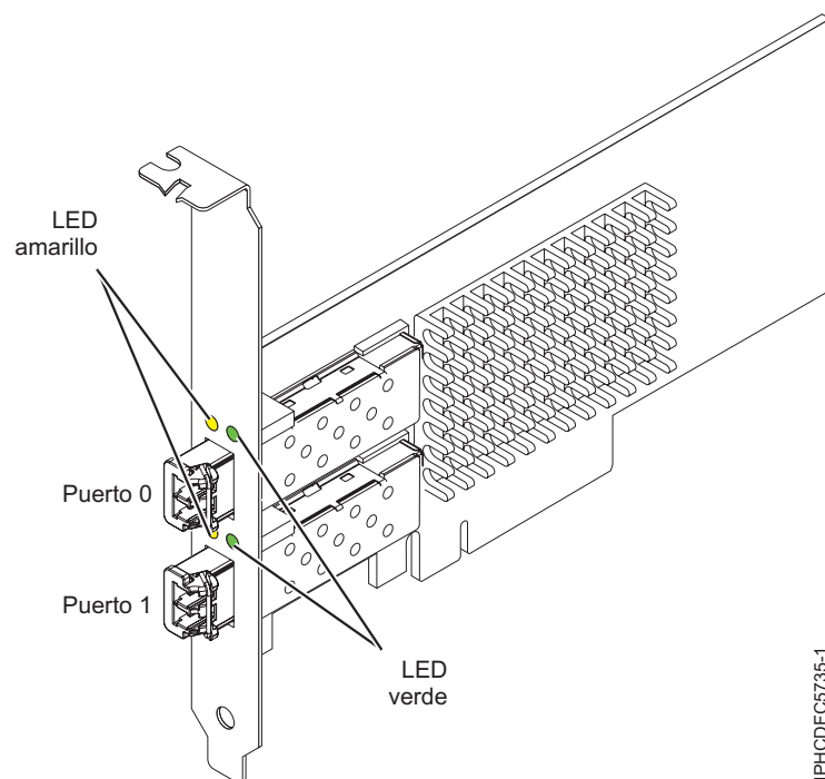
Figura 10. Adaptador 5735
