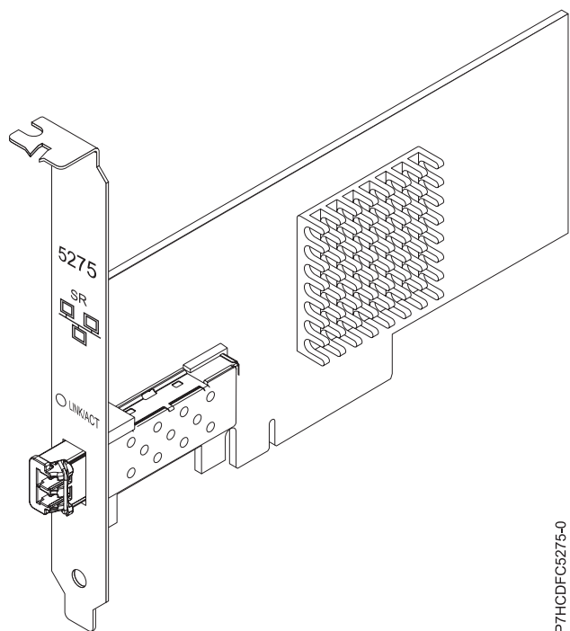
Figura 28. adaptador PCIe LP 10GbE SR de 1 puerto
