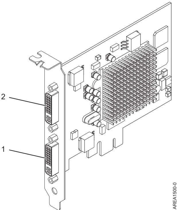
Figura 17. adaptador Acelerador de gráficos PCI Express POWER GXT145
