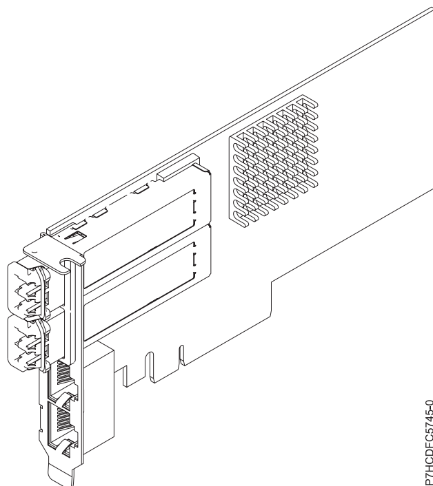
Figura 29. Adaptador PCIe2 LP 2x10GbE SFP+ de cobre y cable de par trenzado no apantallado
