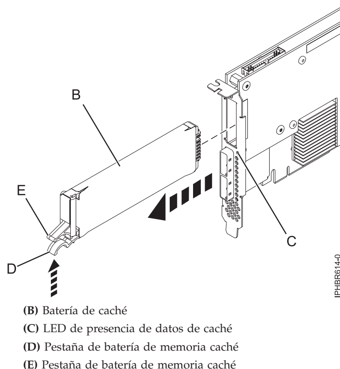
Figura 64. Sustitución de la batería de memoria caché 574E
