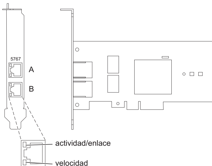
Figura 43. adaptador PCIe LP de 2 puertos 1GbE TX
