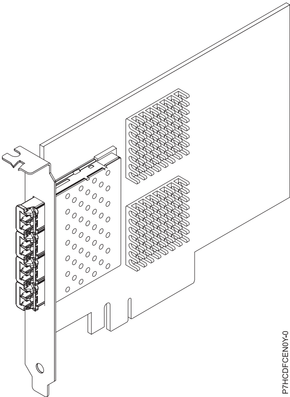
Figura 15. adaptador de canal de fibra PCIe2 LP 8 gigabits de 4 puertos
