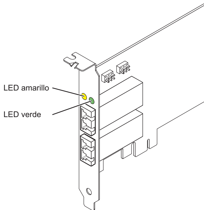
Figura 13. Adaptador 5774
