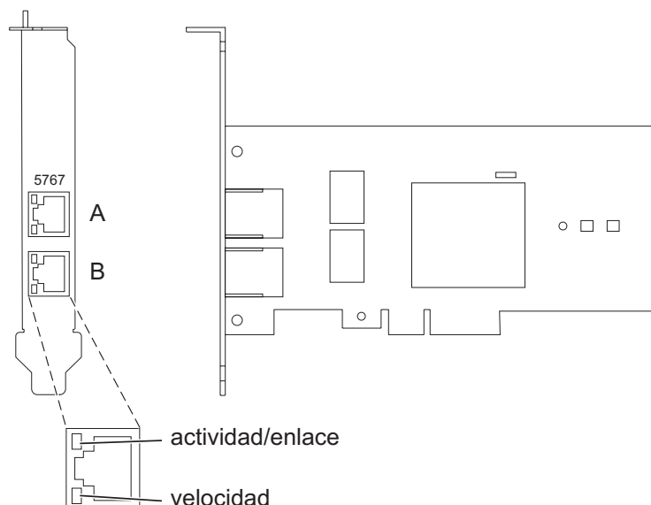
Figura 32. Adaptador PCI Express Ethernet Base-TX 10/100/1000 de 2 puertos
