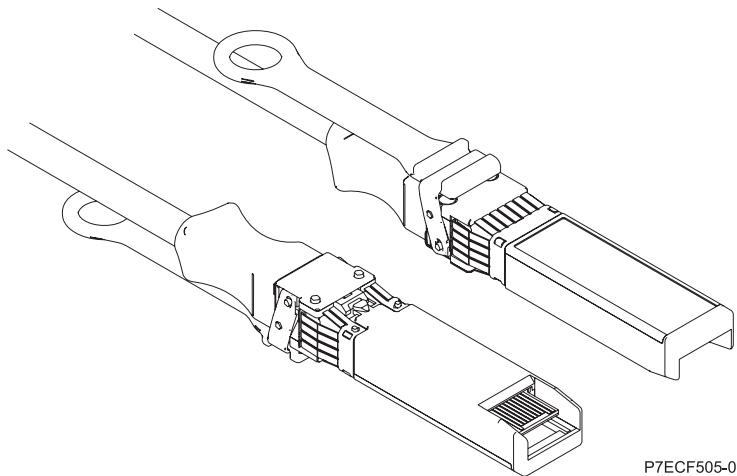
Figura 48. Vistas superior e inferior del cable
