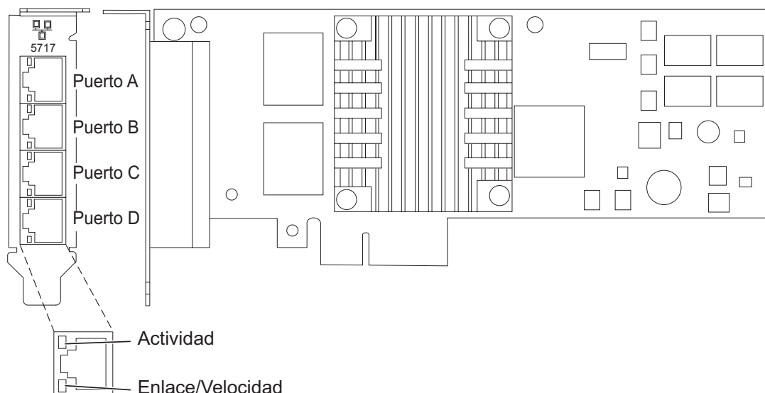
Figura 36. Adaptador PCIe 4 Puertos 10/100/1000 Base-TX
