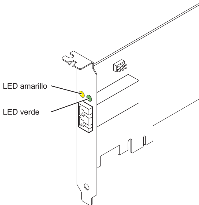
Figura 11. Adaptador 5773
