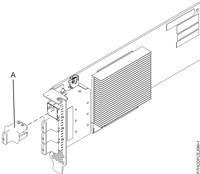
Figura 20. Adaptador PCIe3 SAS RAID de altura reducida y cuatro puertos de 6 Gb
