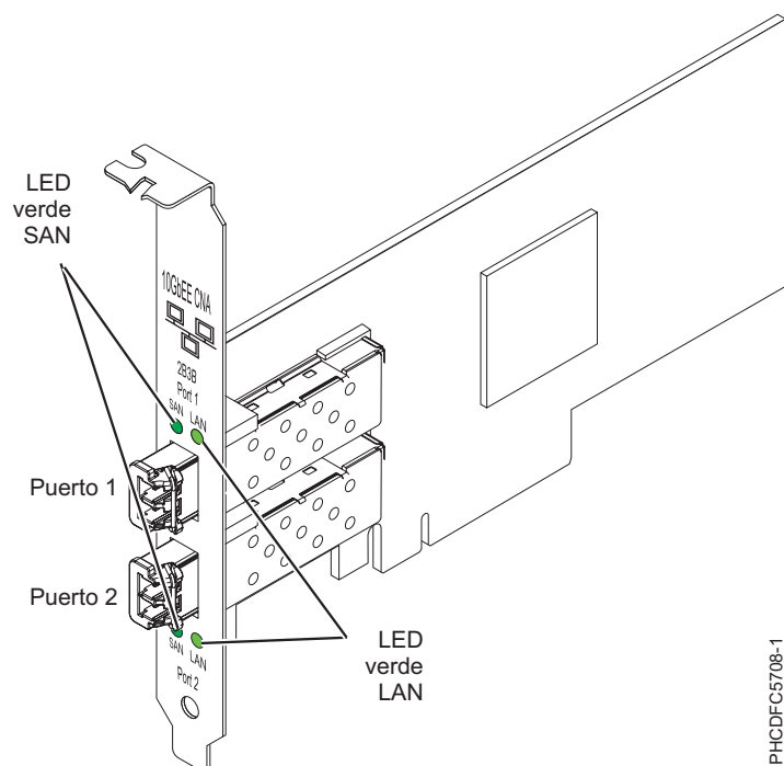
Figura 35. adaptador PCIe de puerto dual FCoE de 10 Gb
