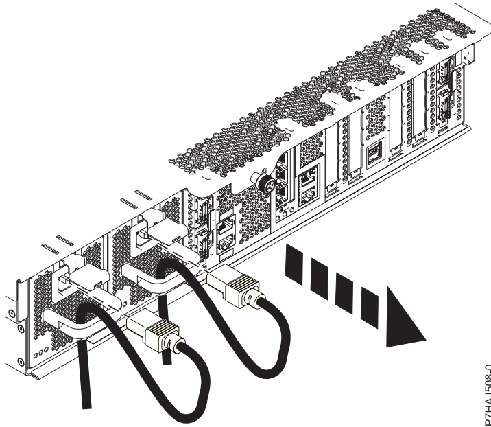
Figura 9. Quitar los cables de alimentación
