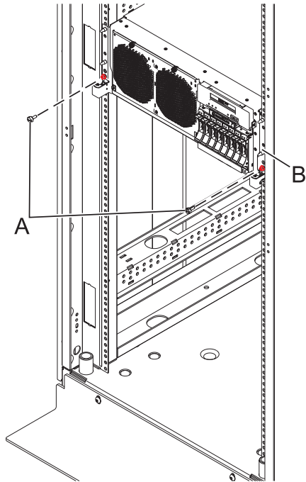
Figura 15. Colocar la unidad del sistema en la posición de servicio
