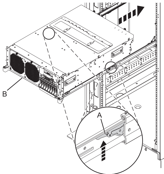
Figura 17. Colocar el sistema en la posición operativa
