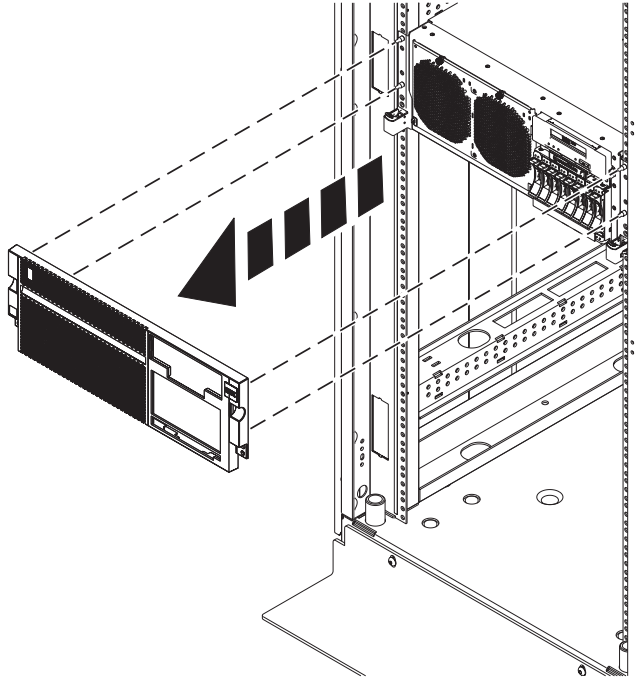
Figura 4. Extracción de la cubierta frontal
