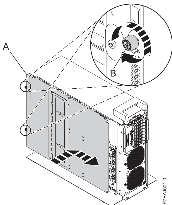
Figura 13. Instalar la cubierta de acceso de servicio interior
