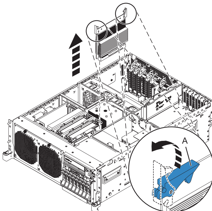
Figura 1. Módulos reguladores de voltaje
