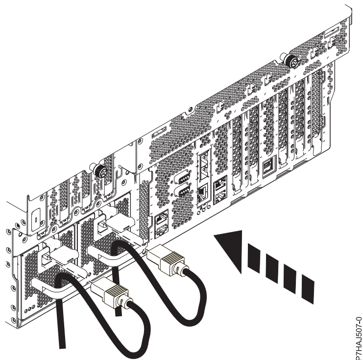
Figura 21. Conectar los cables de alimentación
