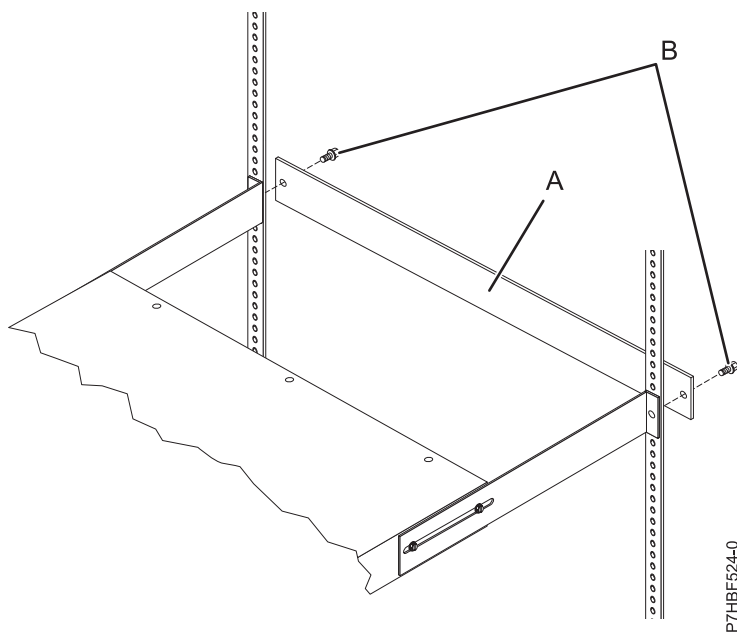
Figura 45. Fijación de las piezas de sujeción y del panel de relleno al bastidor
