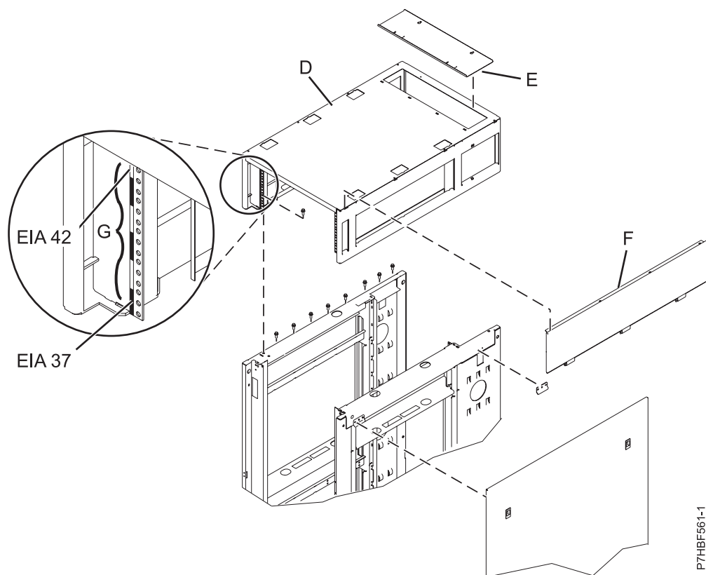
Figura 36. Extracción de la cubierta superior
