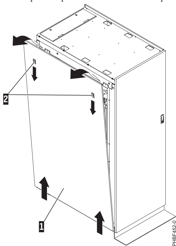
Figura 19. Extracción del panel lateral
