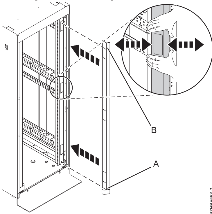
Figura 22. Instalar el panel de acabado en el bastidor
