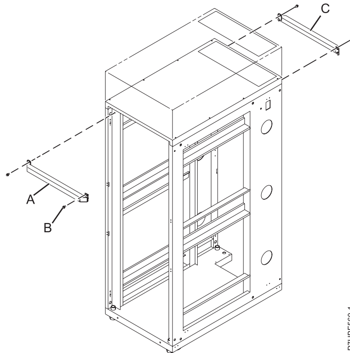
Figura 34. Fijación de la escuadra del bastidor
