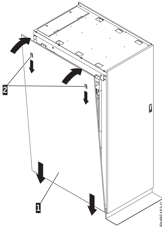
Figura 20. Sustituir el panel lateral
