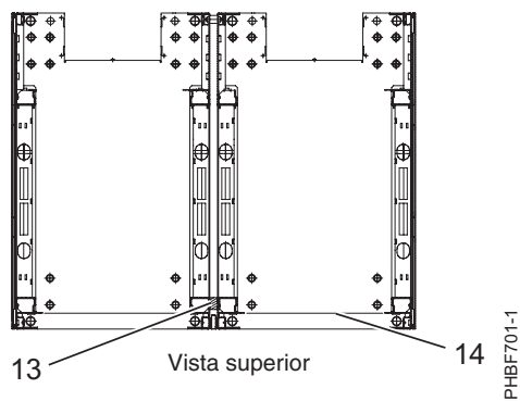
Figura 33. Ubicación de las tiras de espuma (vista superior)
