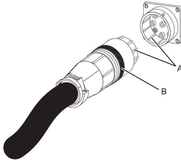
Figura 41. Alineación del conector del cable de alimentación con el modelo PDU
