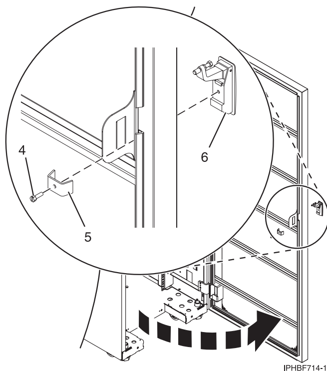
Figura 26. Quitar el pestillo existente en la puerta
