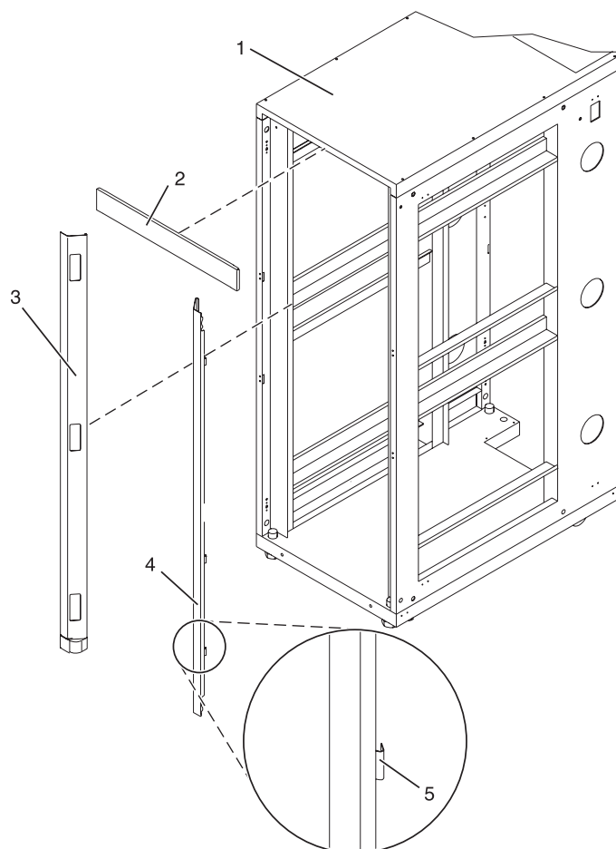
Figura 24. Quitar los paneles de acabado
