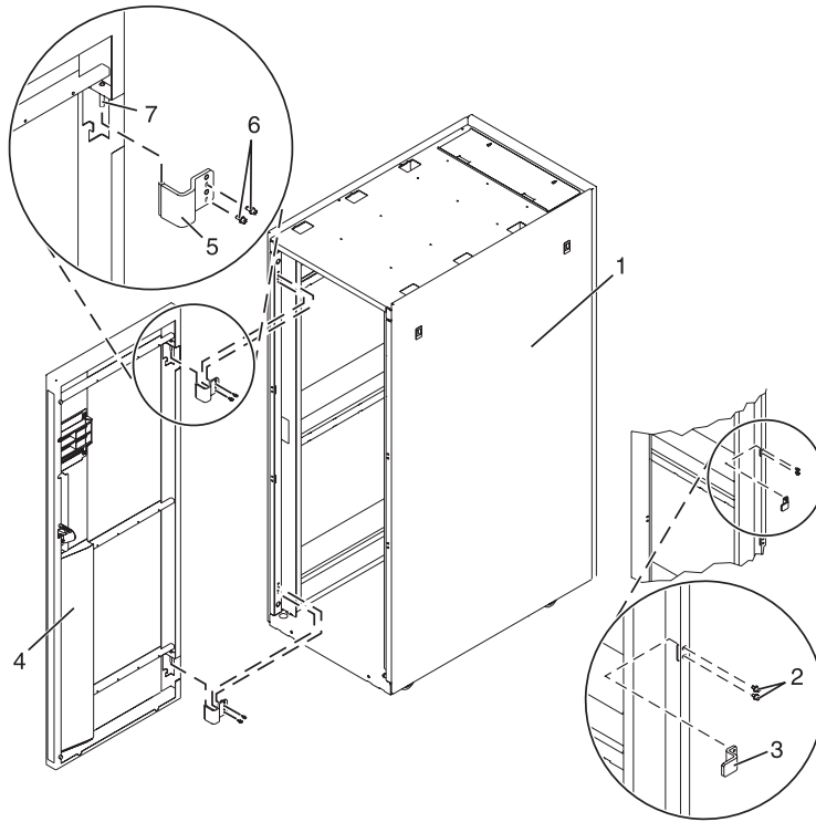
Figura 23. Colocar la puerta del bastidor
