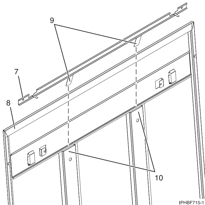
Figura 27. Instalar una barra corredera de seguridad
