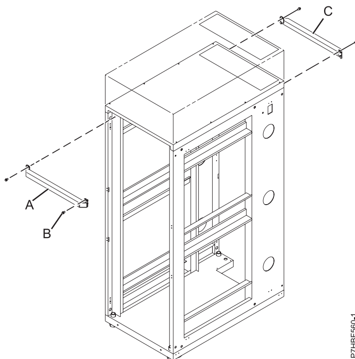
Figura 37. Extracción de la cubierta superior
