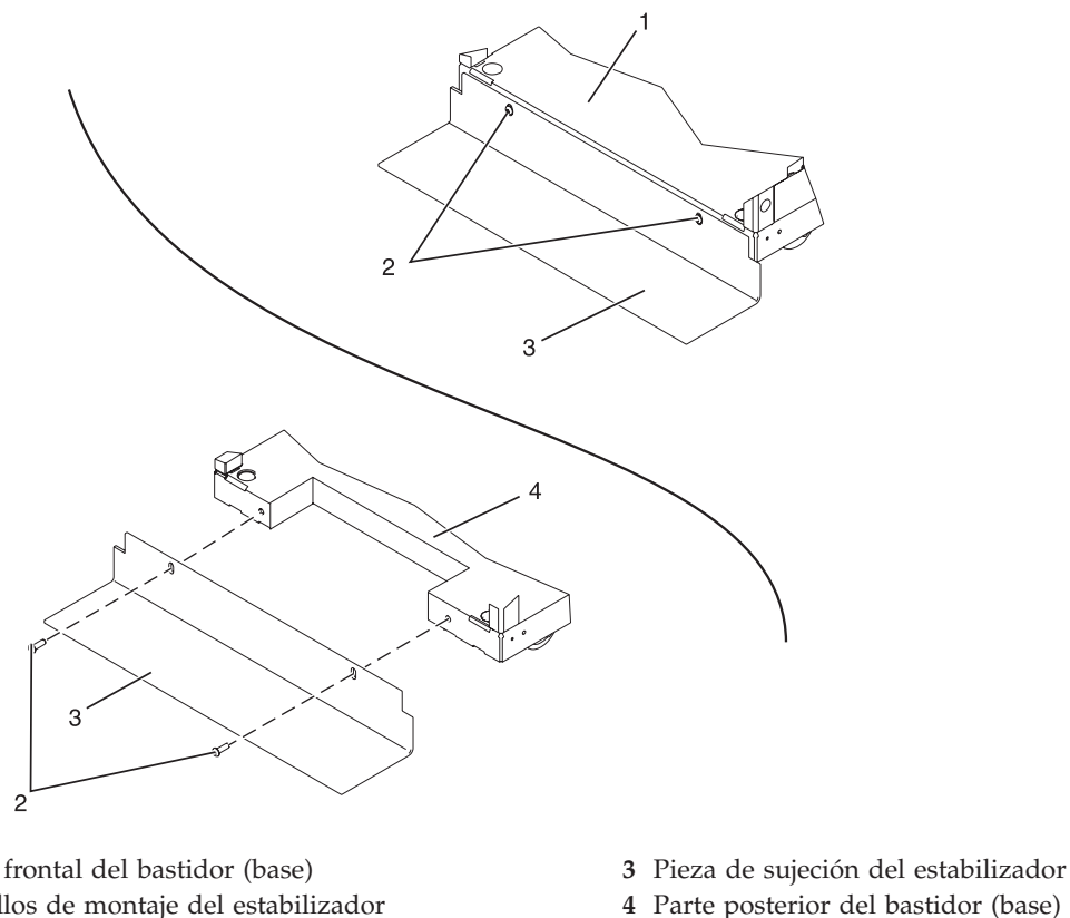
Figura 3. Fijar las piezas de sujeción del estabilizador
