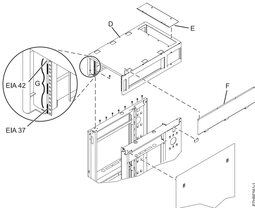
Figura 35. Extracción de la cubierta superior
