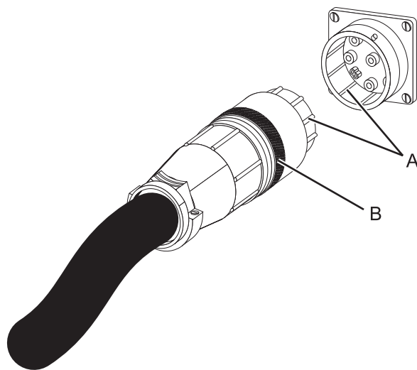
Figura 46. Alineación del conector del cable de alimentación con el modelo PDU
