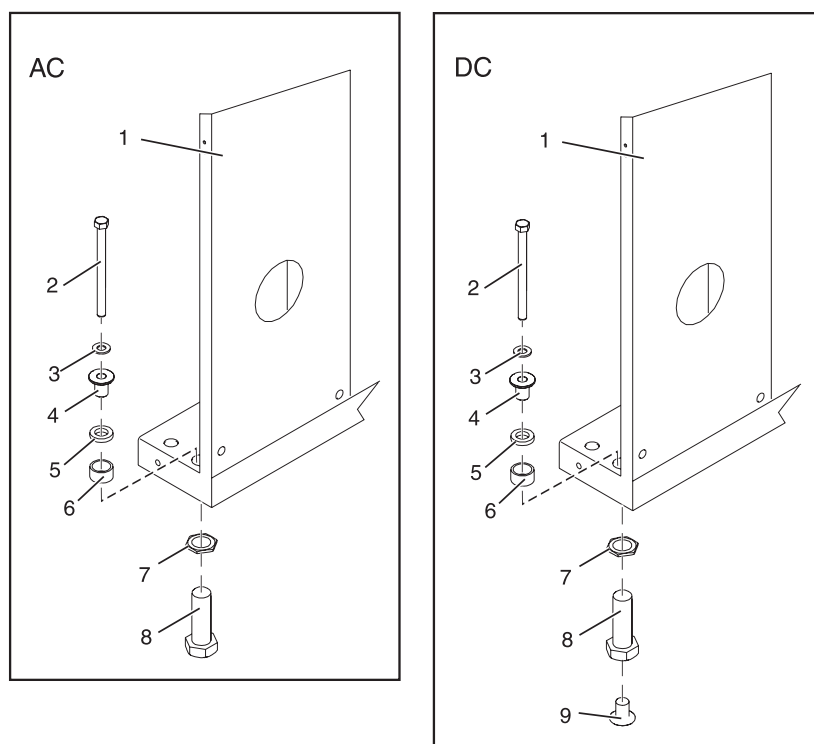
Figura 5. Instalación de las placas de montaje de alimentación CA
