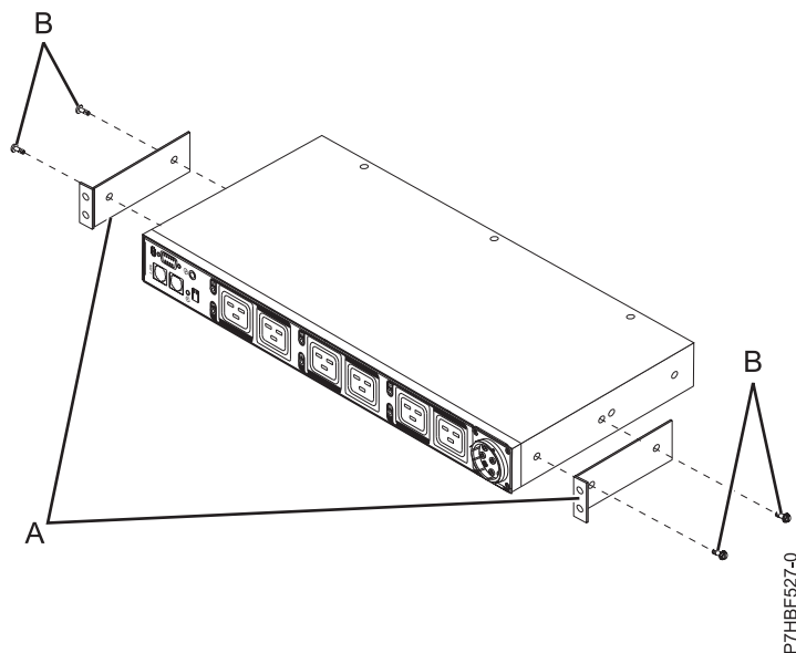
Figura 38. Alinear las piezas de soporte de montaje en vertical con la parte frontal de la PDU+
