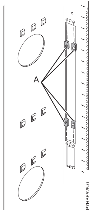
Figura 39. Sujeción de los clips de tuerca a los rebordes de montaje en bastidor
