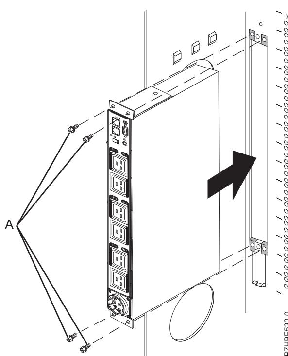
Figura 40. Alinear la PDU+ con la abertura del lateral del bastidor
