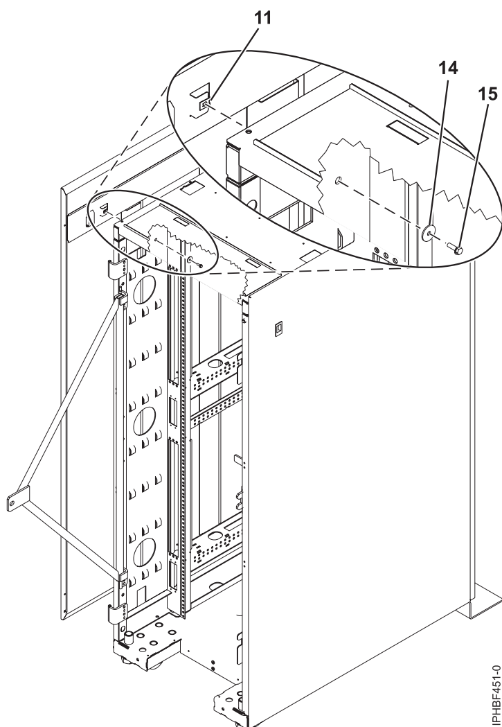
Figura 31. Quitar los tornillos de fijación del panel lateral
