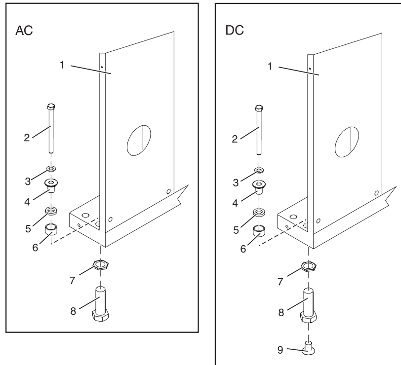
Figura 9. Instalar las placas de montaje de la fuente de alimentación
