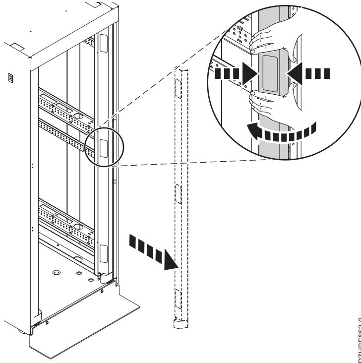
Figura 21. Quitar el panel de acabado del bastidor
