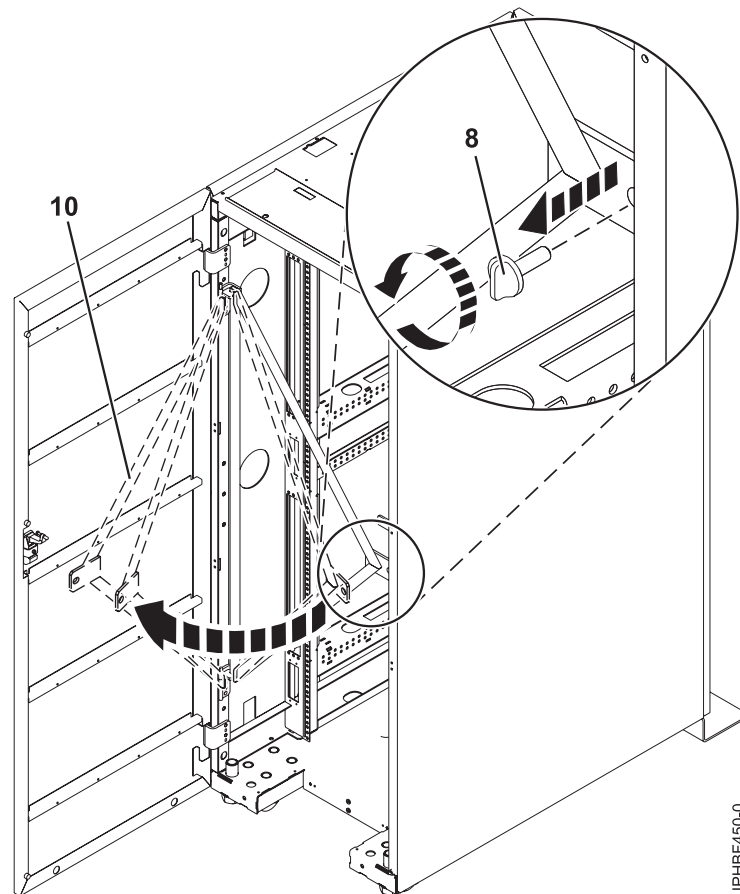
Figura 30. Soltar la escuadra para acceder a los sistemas
