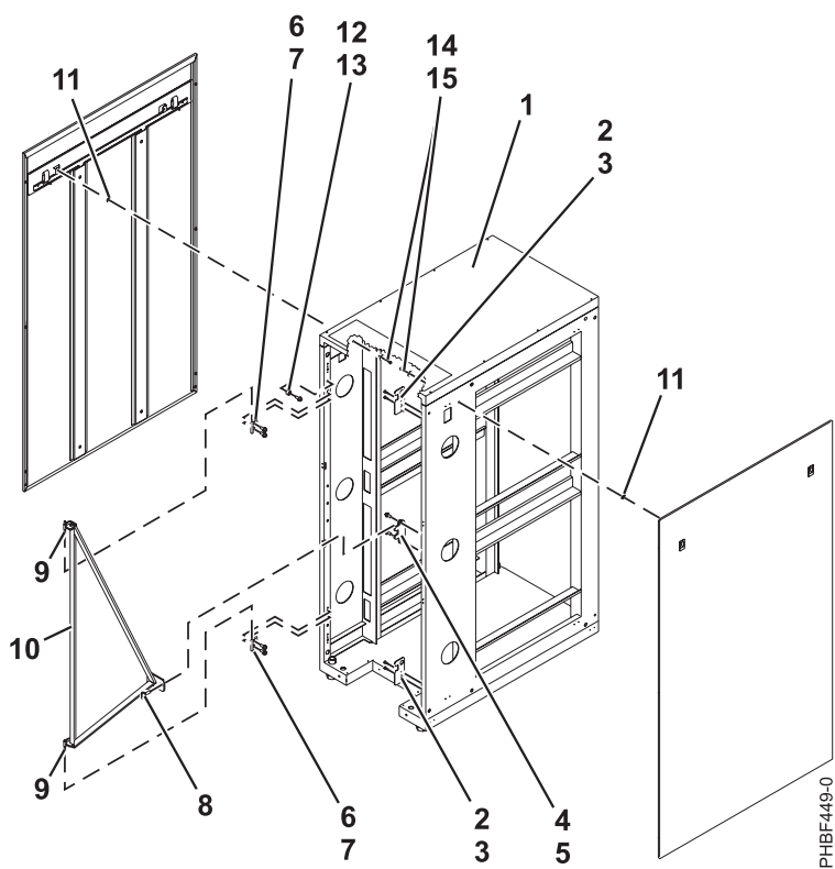
Figura 29. Piezas del kit de alta protección
