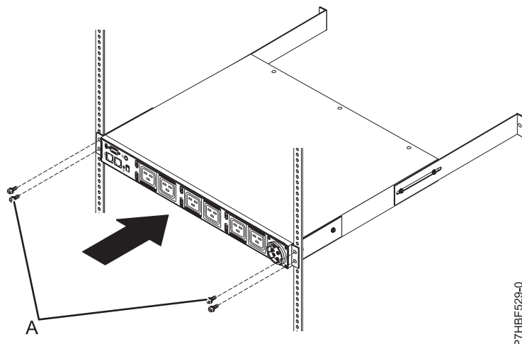
Figura 44. Fijación de la parte frontal de PDU+ al bastidor
