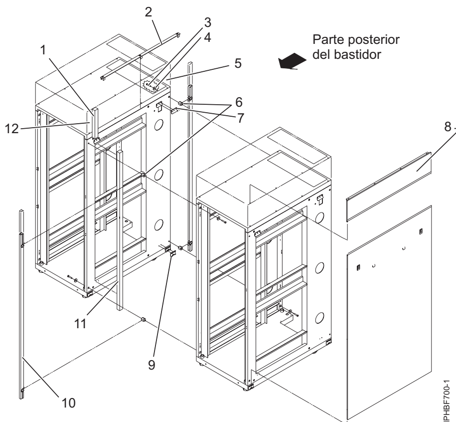
Figura 32. Quitar los paneles laterales y las piezas de sujeción en forma de Z y de J e instalar empalmes y tiras de espuma largas para conectar varios bastidores
