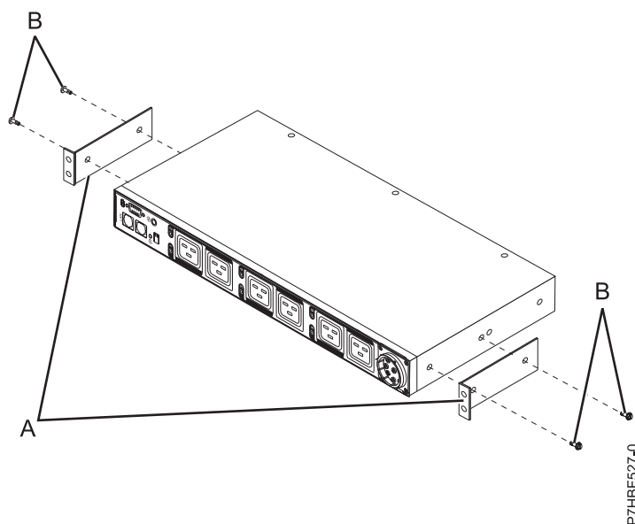
Figura 42. Alinear las piezas de soporte de montaje en vertical con la parte frontal de la PDU+
