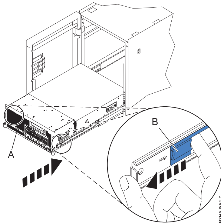
Figura 8. Liberación de los pestillos de seguridad de los rieles
