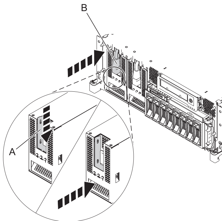
Figura 3. Sustitución de una fuente de alimentación
