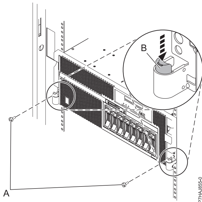
Figura 7. Soltar los pestillos del bastidor
