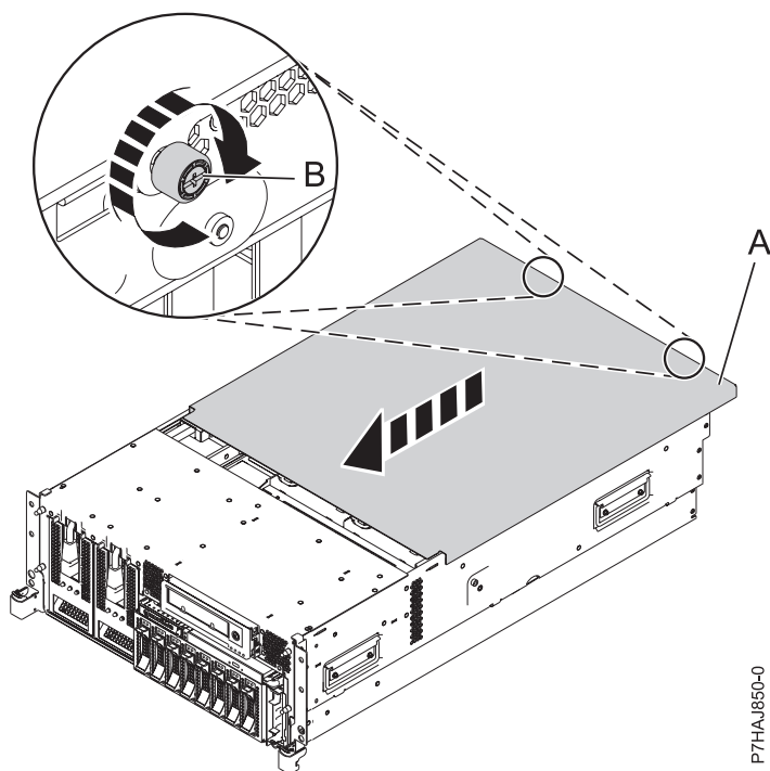
Figura 13. Instalación de la cubierta de acceso de servicio
