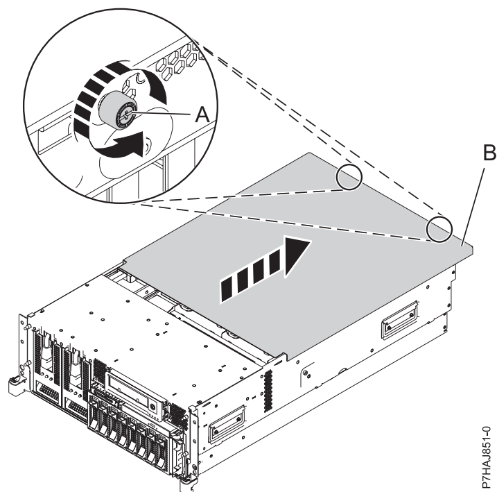
Figura 12. Extracción de la cubierta de acceso de servicio
