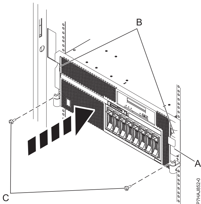
Figura 9. Volver a poner los tornillos de mano
