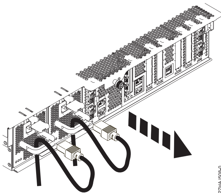
Figura 16. Extracción de los cables de alimentación
