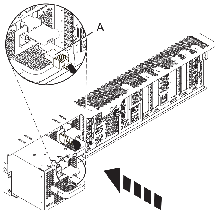
Figura 7. Sustitución de una fuente de alimentación
