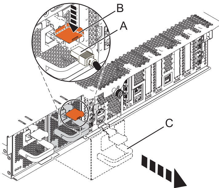
Figura 6. Extracción de la fuente de alimentación
