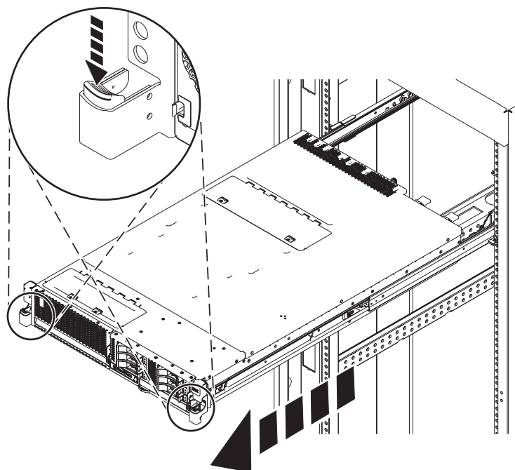
Figura 13. Colocación del sistema en posición de servicio
