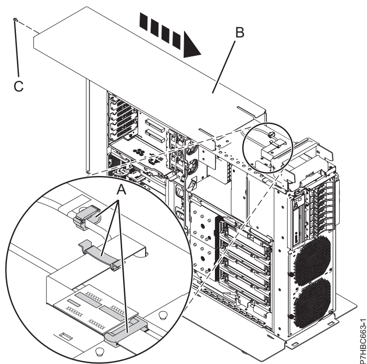
Figura 16. Fijación de un cable de señal en un sistema autónomo
