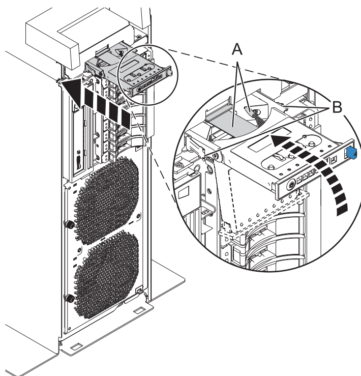
Figura 4. Sustitución de un panel de control en un sistema autónomo
