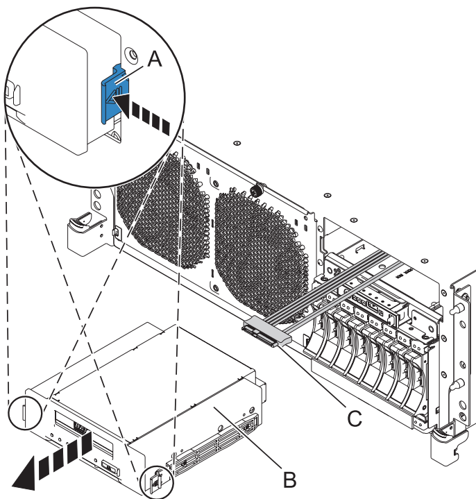
Figura 5. Extracción de un dispositivo de soporte SAS
