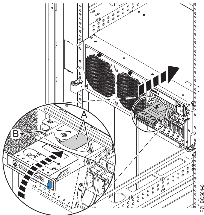
Figura 3. Sustitución de un panel de control en un sistema montado en bastidor
