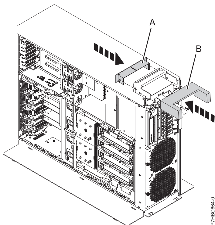
Figura 17. Recolocación de las tapas de tirador en un sistema autónomo
