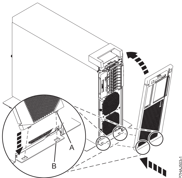
Figura 23. Instalación de la cubierta frontal
