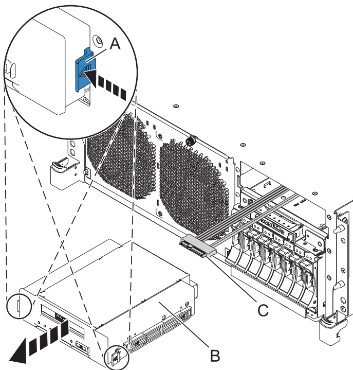
Figura 12. Extracción de un dispositivo de soporte SAS
