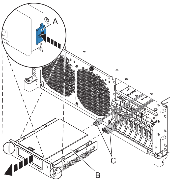
Figura 6. Extracción de un dispositivo de soporte USB
