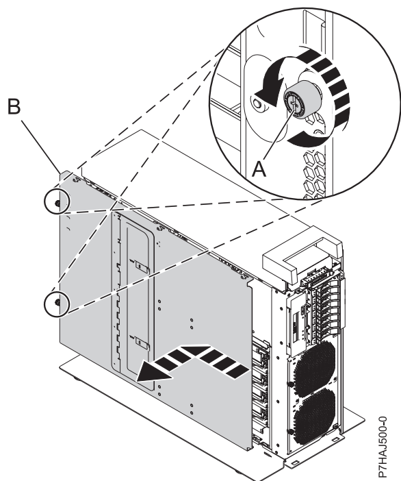
Figura 27. Extracción de la cubierta interior de acceso de servicio
