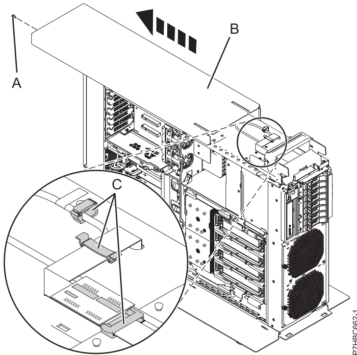
Figura 11. Extracción de la cubierta lateral y del cable de señal de un sistema autónomo
