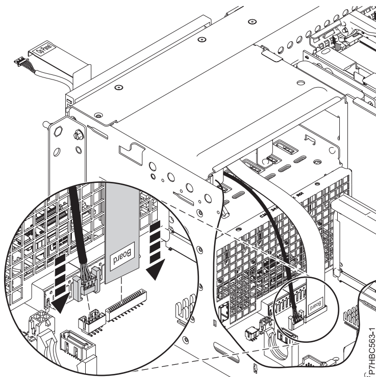
Figura 15. Conexión de un cable de señal en un sistema montado en bastidor
