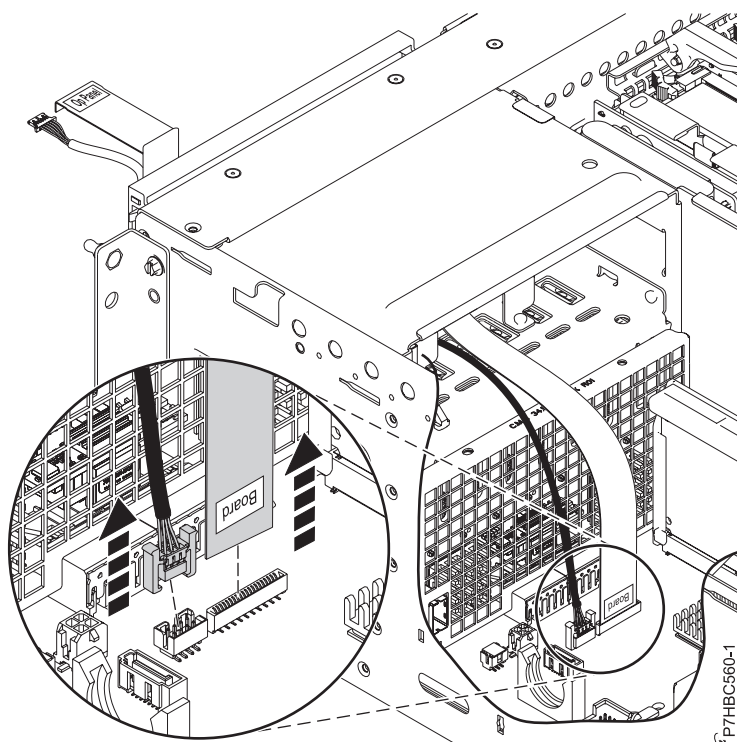
Figura 7. Desconexión de un cable de señal de un sistema montado en bastidor
