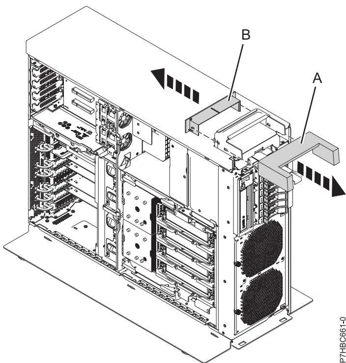
Figura 10. Extracción de las tapas de tirador de un sistema autónomo
