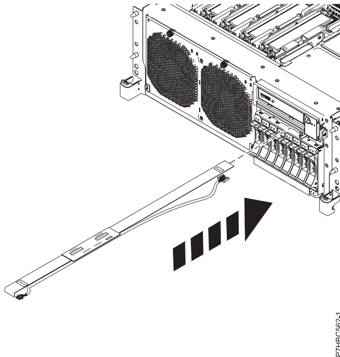
Figura 14. Paso de un cable de señal en un sistema montado en bastidor
