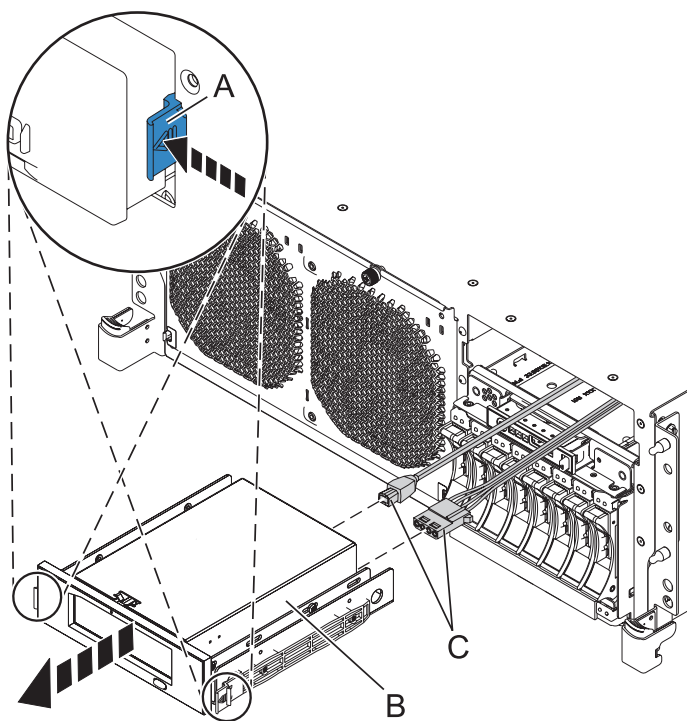
Figura 13. Extracción de un dispositivo de soporte USB
