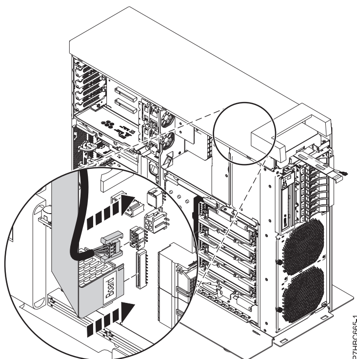
Figura 18. Reconexión del cable de señal en un sistema autónomo
