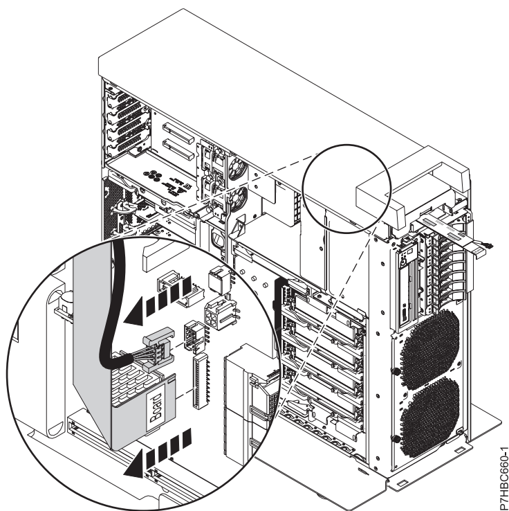
Figura 9. Desconexión de un cable de señal en un sistema autónomo
