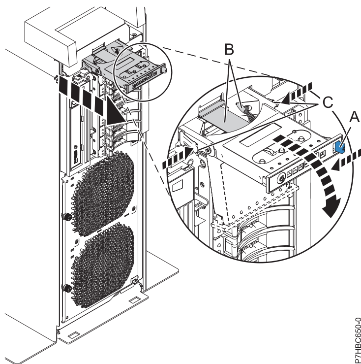
Figura 2. Extracción de un panel de control de un sistema autónomo
