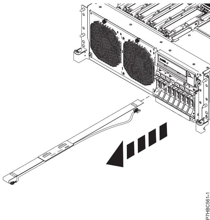
Figura 8. Extracción de un cable de señal de un sistema montado en bastidor
