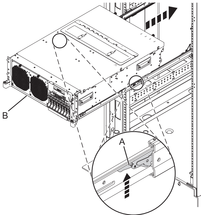
Figura 33. Colocar la unidad del sistema en posición operativa
