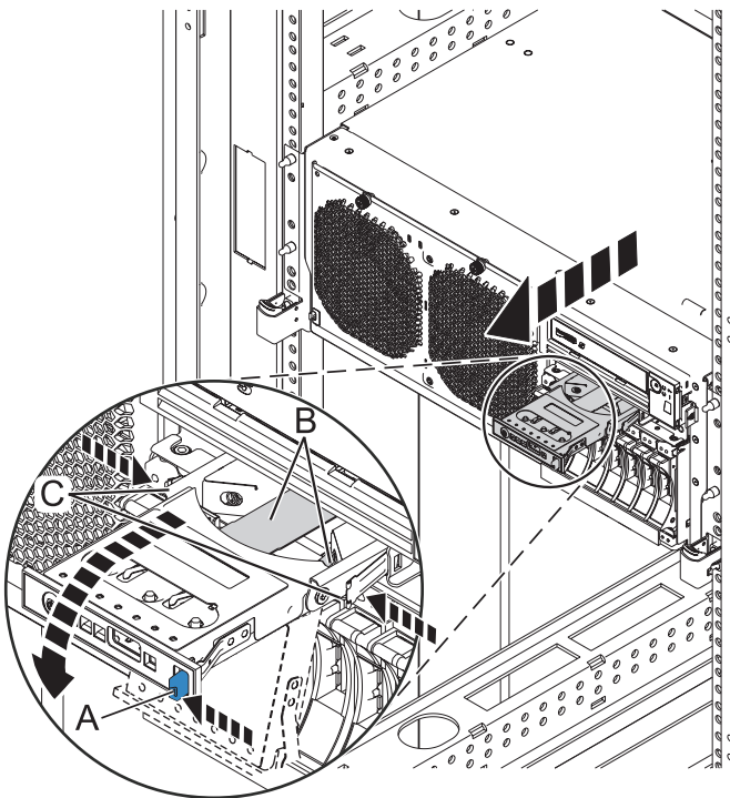
Figura 1. Extracción de un panel de control de un sistema montado en bastidor
