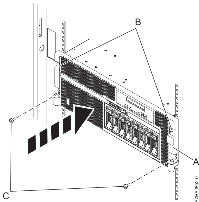
Figura 21. Instalación de la cubierta frontal
