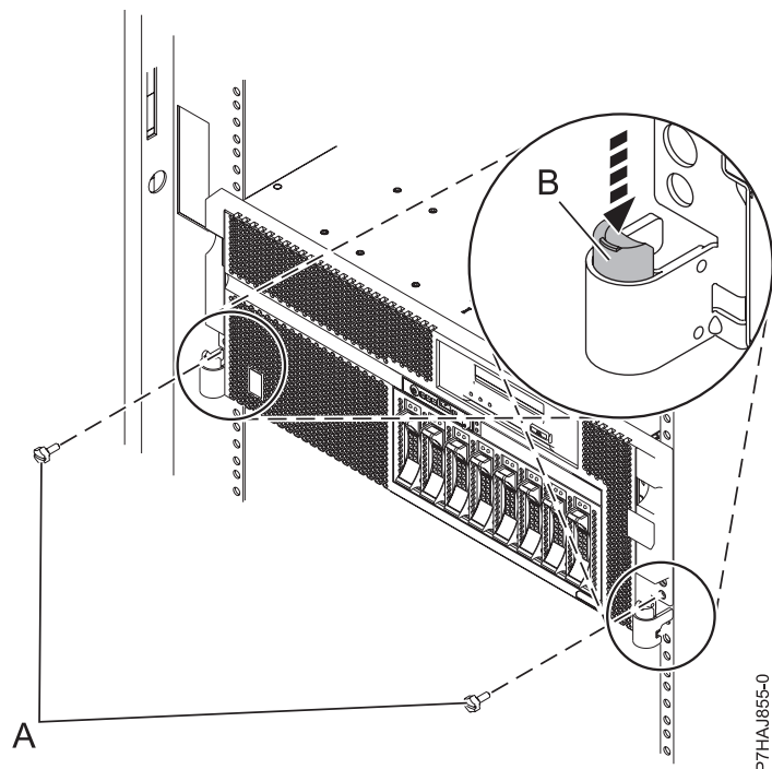
Figura 24. Soltar los pestillos del bastidor
