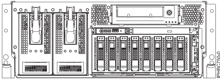
Figura 1. Placa posterior de la unidad de disco
