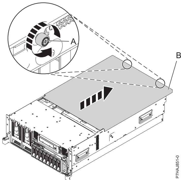
Figura 22. Extraer la cubierta de acceso de servicio
