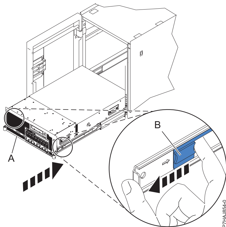
Figura 25. Liberación de los pestillos de seguridad de los rieles
