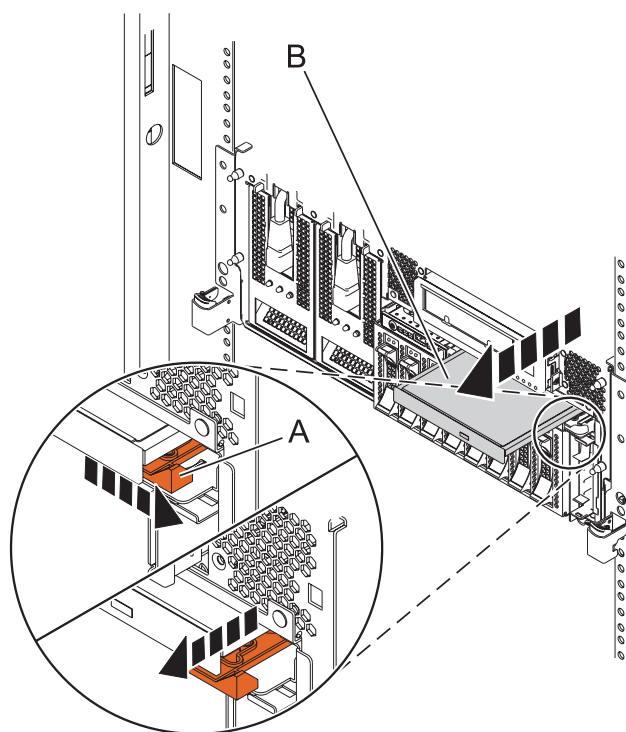
Figura 7. Extraer el dispositivo de soporte de la placa posterior de la unidad de disco
