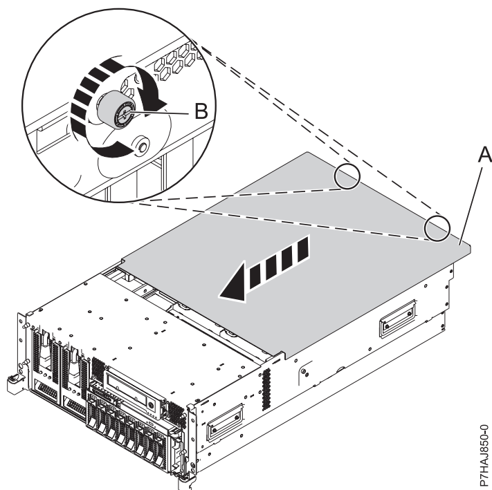
Figura 23. Instalar la cubierta de acceso de servicio
