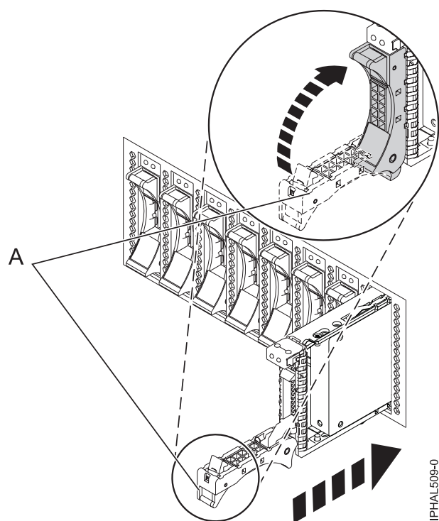
Figura 14. Instalar las unidades de disco de la placa posterior
