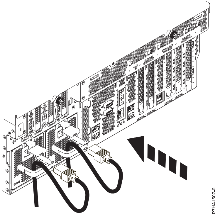
Figura 30. Conexión de los cables de alimentación
