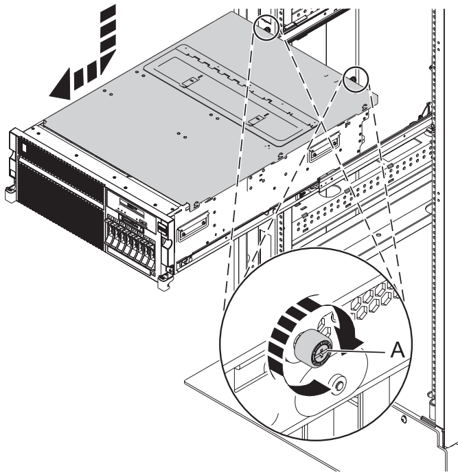
Figura 21. Instalar la cubierta de acceso de servicio
