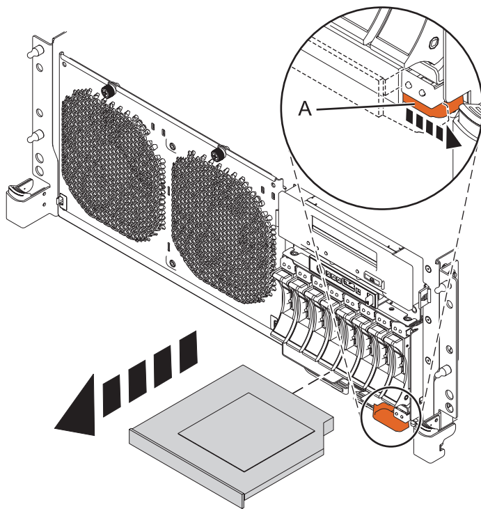
Figura 4. Extraer el dispositivo de soporte de la placa posterior de la unidad de disco
