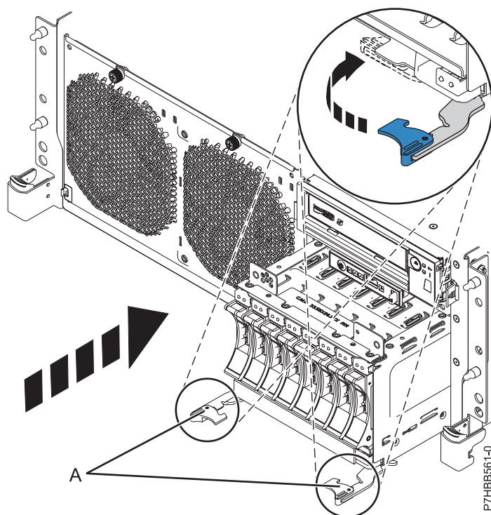
Figura 8. Instalación de la placa posterior llena de unidades de disco en un modelo montado en bastidor
