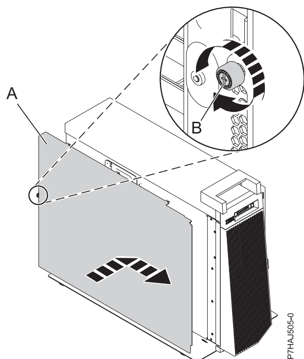
Figura 23. Instalar la cubierta de acceso de servicio exterior
