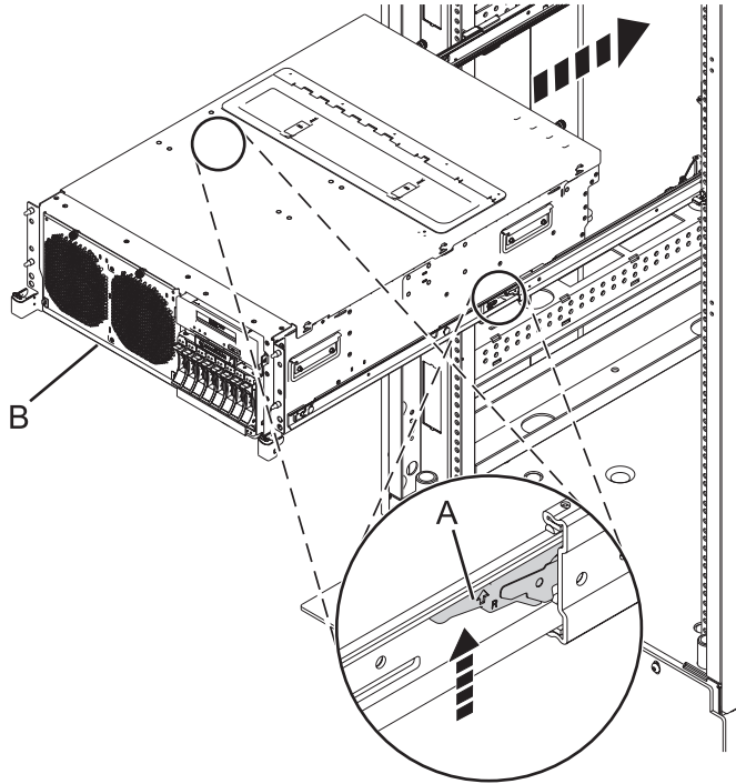
Figura 26. Colocación de la unidad del sistema en la posición operativa
