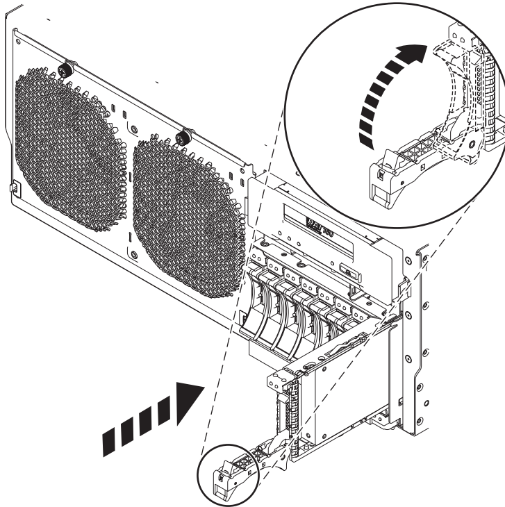
Figura 9. Instalar las unidades de disco de la placa posterior
