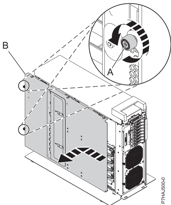
Figura 20. Quitar la cubierta de acceso de servicio interior
