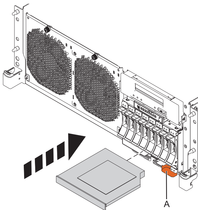
Figura 10. Instalación del dispositivo de soporte
