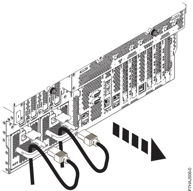
Figura 28. Extracción de los cables de alimentación de un sistema montado en bastidor
