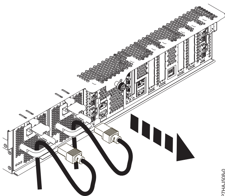
Figura 20. Extracción de los cables de alimentación
