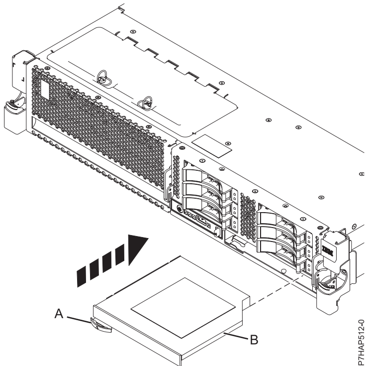
Figura 12. Instalación del dispositivo de soporte extraplano
