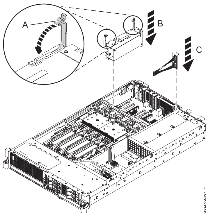
Figura 10. Sustitución del adaptador GX FC EJ0G de un sistema
