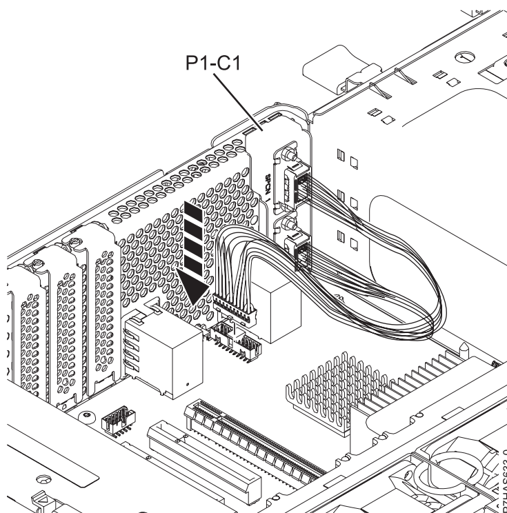
Figura 4. Instalación del cable de SPCN
