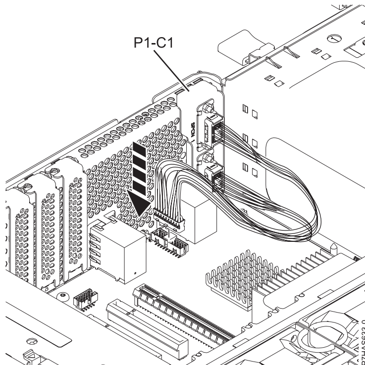
Figura 12. Sustitución del cable SPCN
