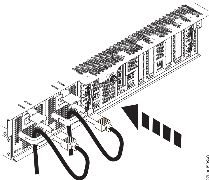
Figura 22. Conectar los cables de alimentación
