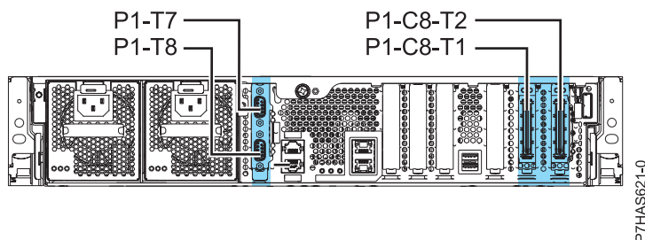
Figura 1. Ranuras del adaptador GX y códigos de ubicación
