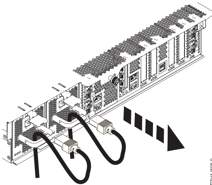
Figura 21. Extracción de los cables de alimentación
