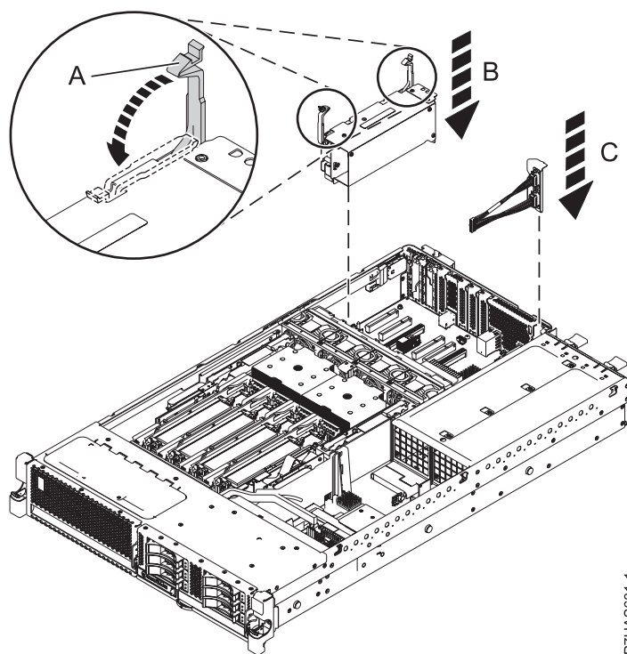
Figura 10. Sustitución del adaptador GX FC EJ0G del sistema
