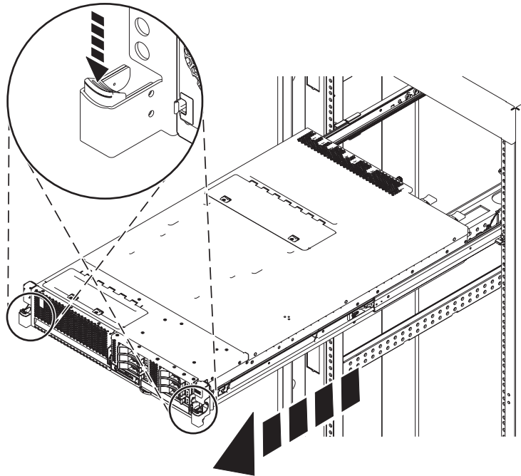
Figura 18. Colocar el sistema en la posición de servicio
