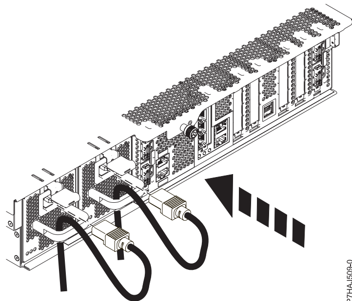
Figura 17. Conectar los cables de alimentación
