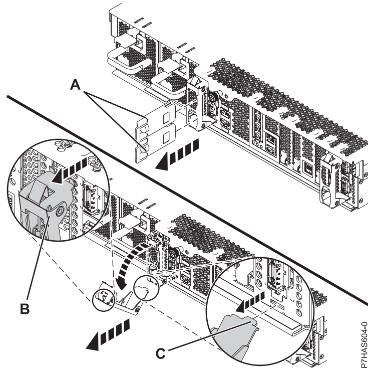
Figura 5. Extracción de la abrazadera de cables
