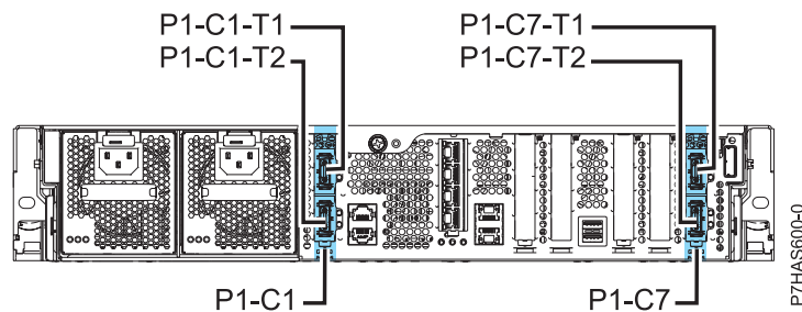
Figura 1. Vista posterior del sistema 8231-E2B que muestra las ranuras y códigos de ubicación de los adaptadores GX.
