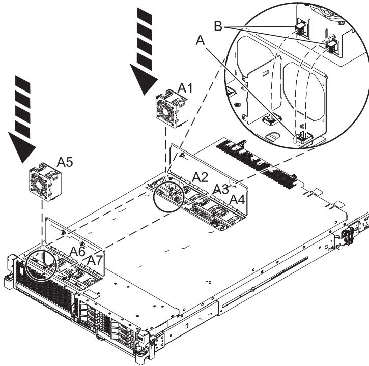
Figura 2. Sustitución del ventilador en un modelo montado en bastidor para 8246-L1C, 8246-L1D, 8246-L1S, 8246-L1T, 8246-L2C, 8246-L2D, 8246-L2S o 8246-L2T
