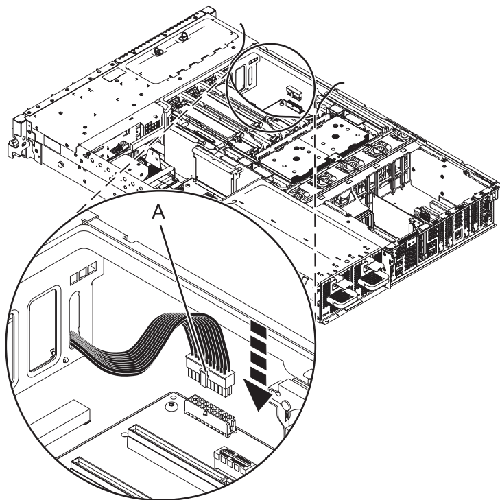
Figura 6. Conectar el cable del ventilador
