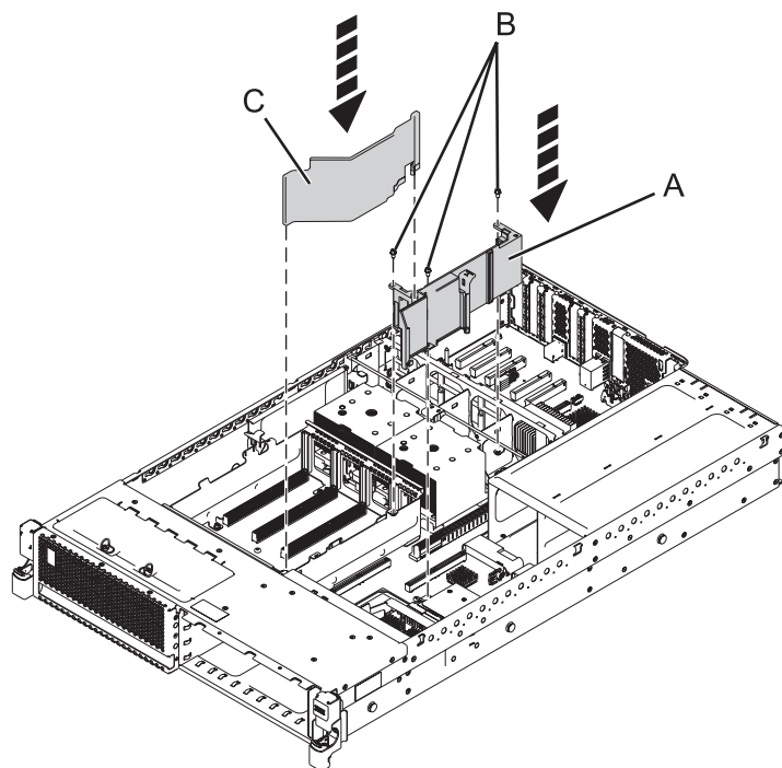
Figura 10. Sustitución de la guía de regulador de voltaje y el separador de aire (8246-L1C, 8246-L1D, 8246-L1S, 8246-L1T, 8246-L2C, 8246-L2D, 8246-L2S o 8246-L2T)
