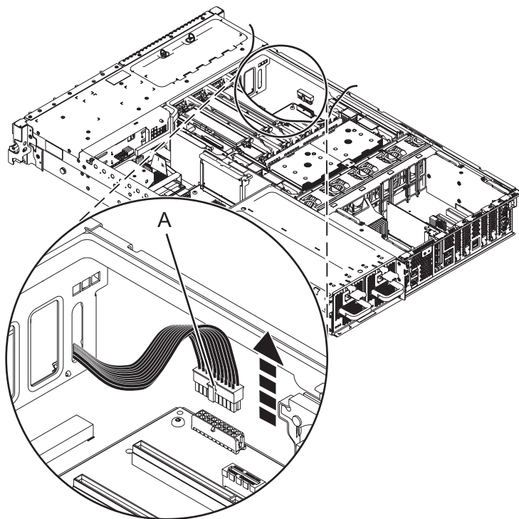
Figura 3. Extracción del cable del ventilador
