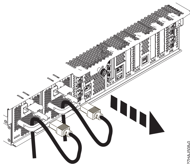
Figura 18. Extracción de los cables de alimentación
