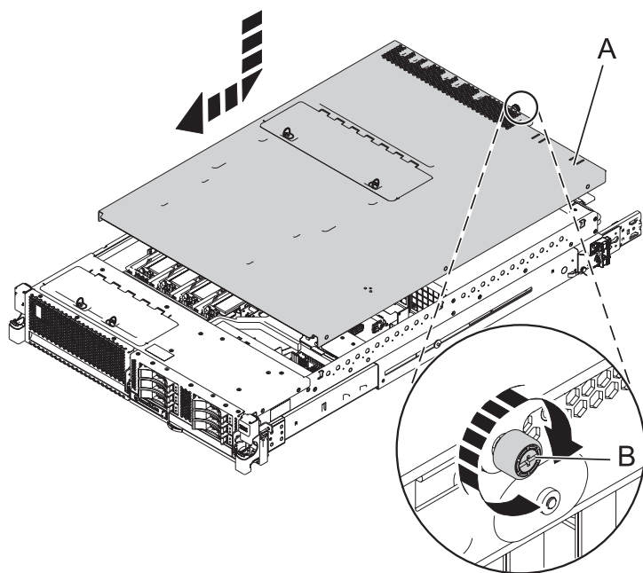
Figura 14. Instalación de la cubierta de acceso de servicio
