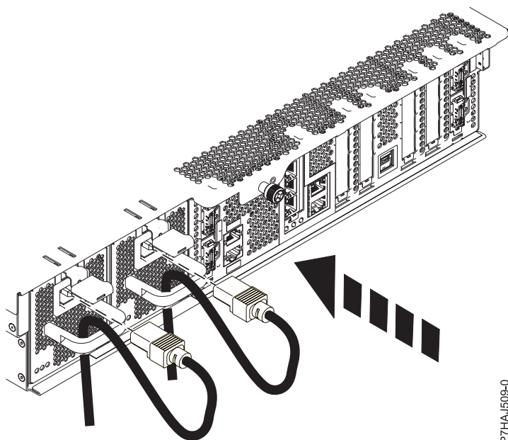
Figura 19. Conectar los cables de alimentación
