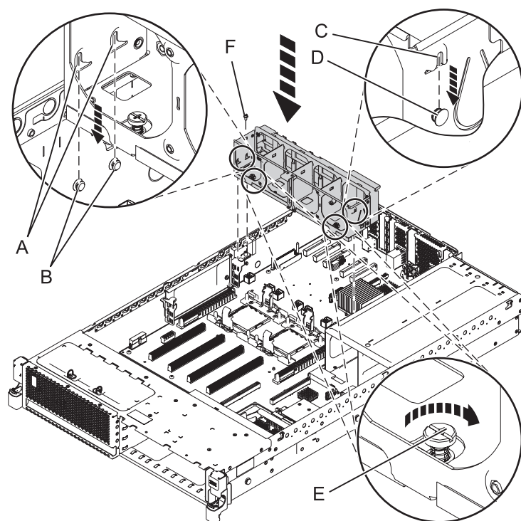
Figura 9. Sustitución del chasis del ventilador central de 8246-L1C, 8246-L1D, 8246-L1S, 8246-L1T, 8246-L2C, 8246-L2D, 8246-L2S o 8246-L2T
