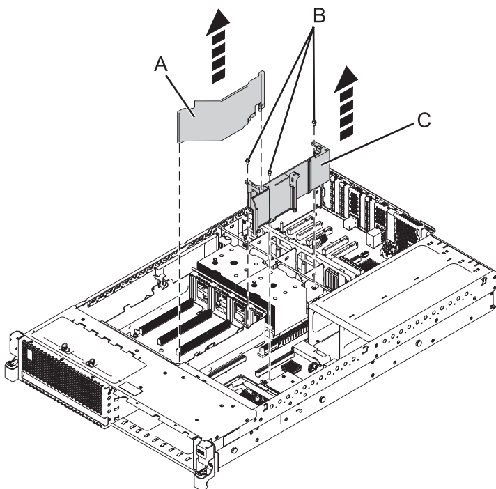
Figura 7. Extracción de la guía de regulador de voltaje y el separador de aire (8246-L1C, 8246-L1D, 8246-L1S, 8246-L1T, 8246-L2C, 8246-L2D, 8246-L2S o 8246-L2T)
