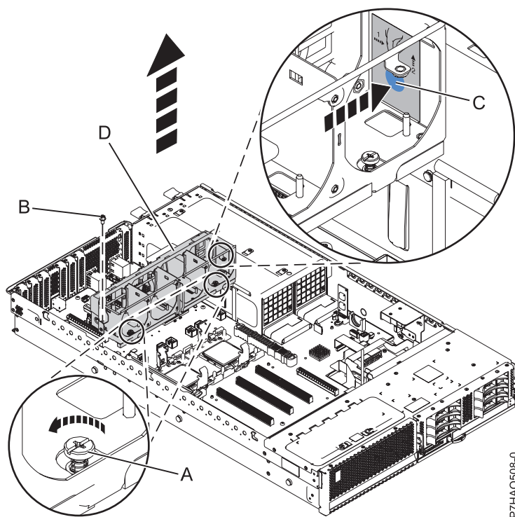
Figura 8. Extracción del chasis de ventilador
