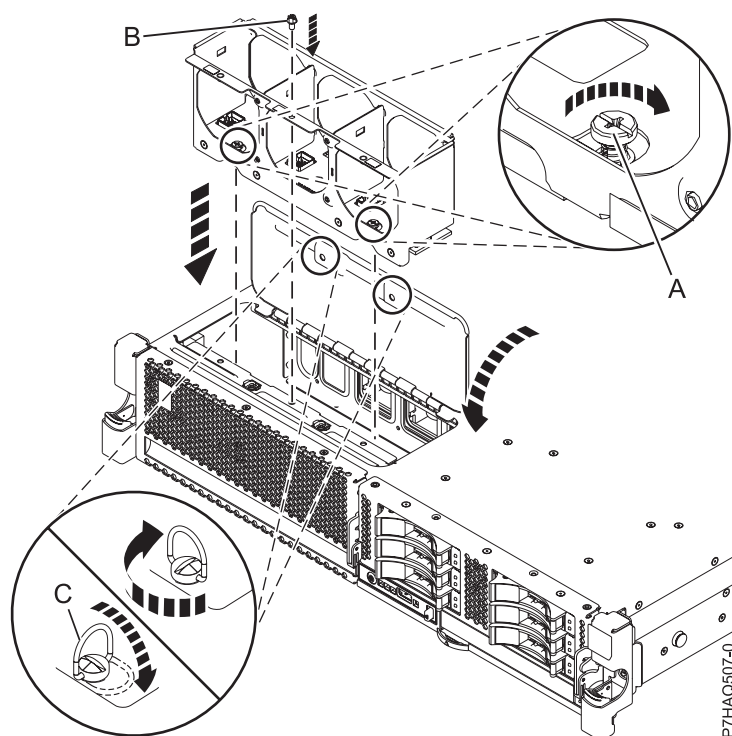
Figura 5. Sustitución del chasis del ventilador frontal para el sistema 8246-L1C, 8246-L1D, 8246-L1S, 8246-L1T, 8246-L2C, 8246-L2D, 8246-L2S o 8246-L2T
