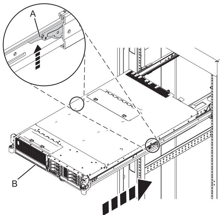
Figura 16. Desbloqueo los pestillos de seguridad de los rieles
