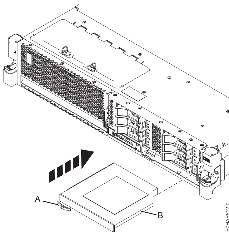
Figura 8. Instalación de un dispositivo multimedia extraplano
