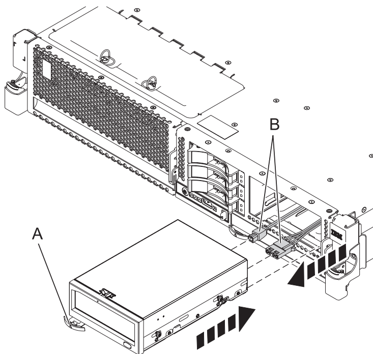
Figura 21. Instalación de una unidad de disco USB
