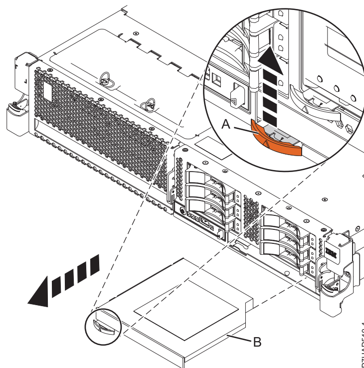
Figura 11. Extracción de un dispositivo de soporte extraplano
