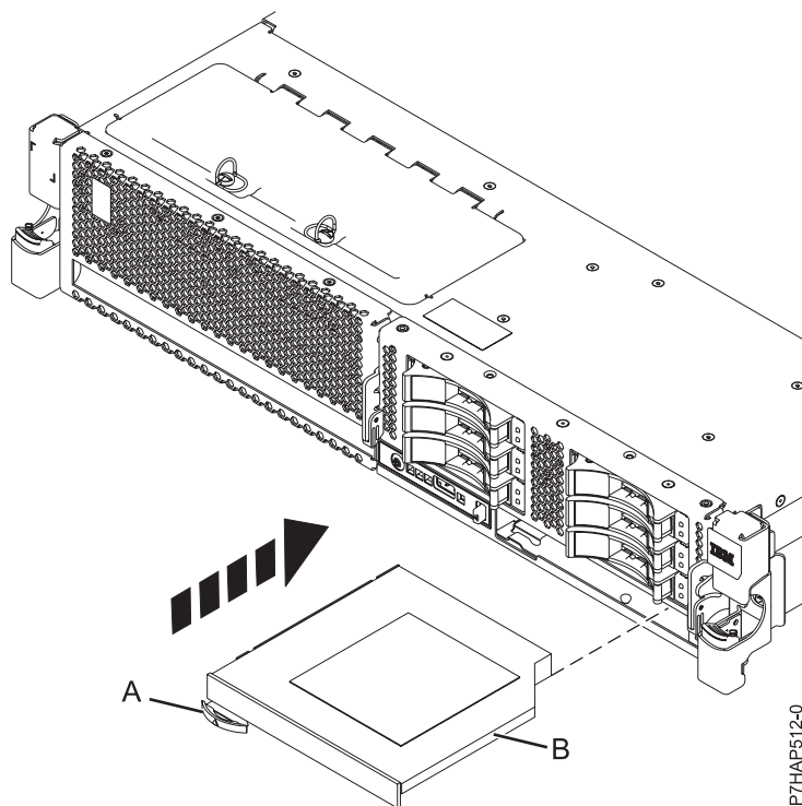
Figura 18. Instalar un dispositivo de soporte extraplano
