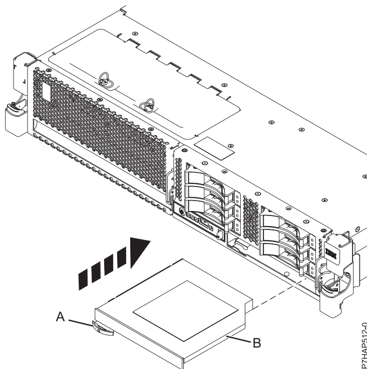
Figura 7. Instalar un dispositivo de soporte extraplano
