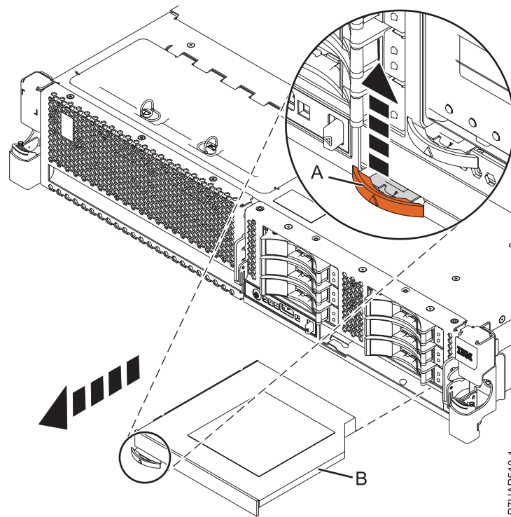
Figura 16. Extracción de un dispositivo de soporte extraplano
