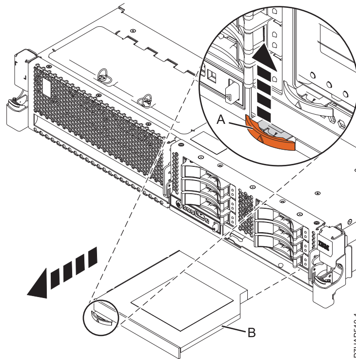
Figura 6. Extracción de un dispositivo de soporte extraplano
