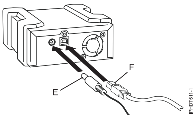
Figura 23. Conexión de USB y cables de la fuente de alimentación
