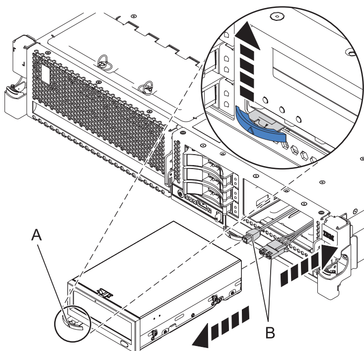
Figura 19. Extracción del dispositivo de soporte
