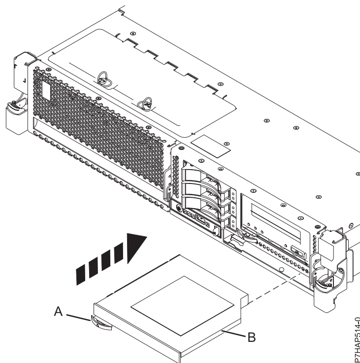
Figura 5. Instalar un dispositivo de soporte extraplano
