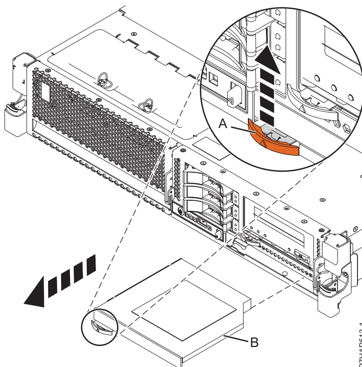
Figura 4. Extracción de un dispositivo de soporte extraplano
