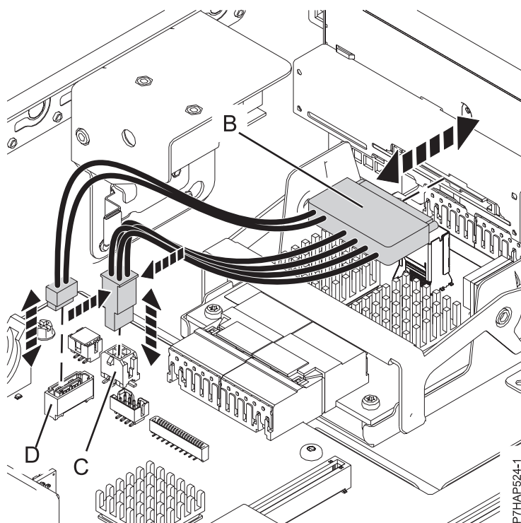
Figura 3. Conexiones de cable de soporte
