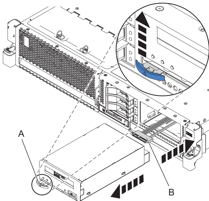
Figura 1. Extracción de un dispositivo de soporte SAS
