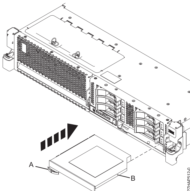
Figura 12. Instalar un dispositivo de soporte extraplano
