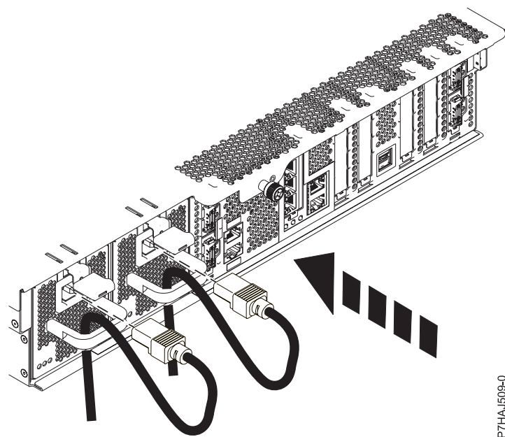
Figura 32. Conectar los cables de alimentación
