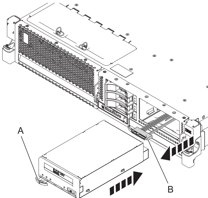
Figura 2. Instalación de un dispositivo de soporte SAS
