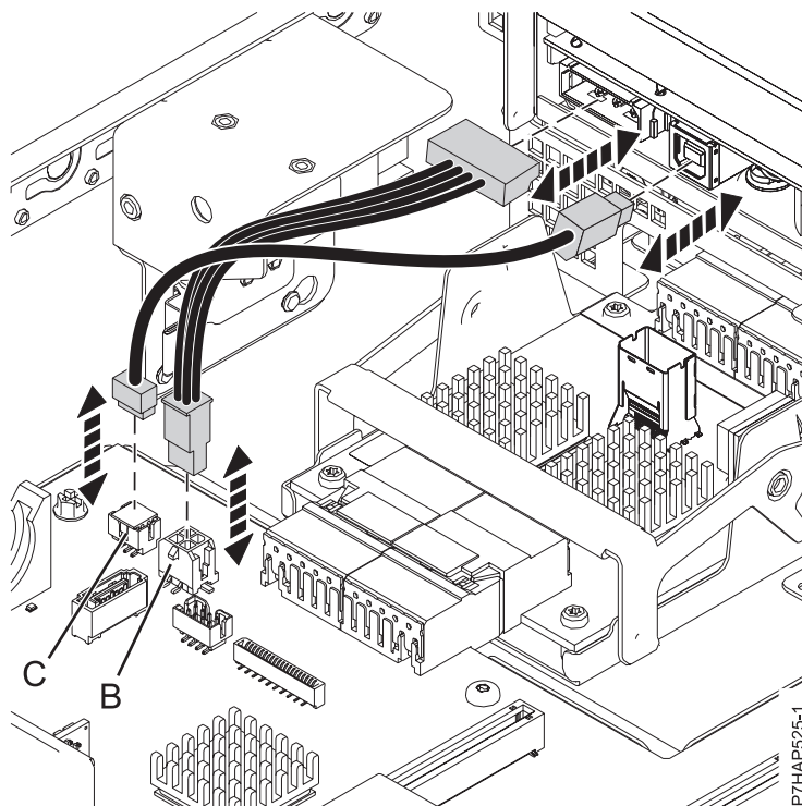
Figura 22. Conexiones de cable de soporte
