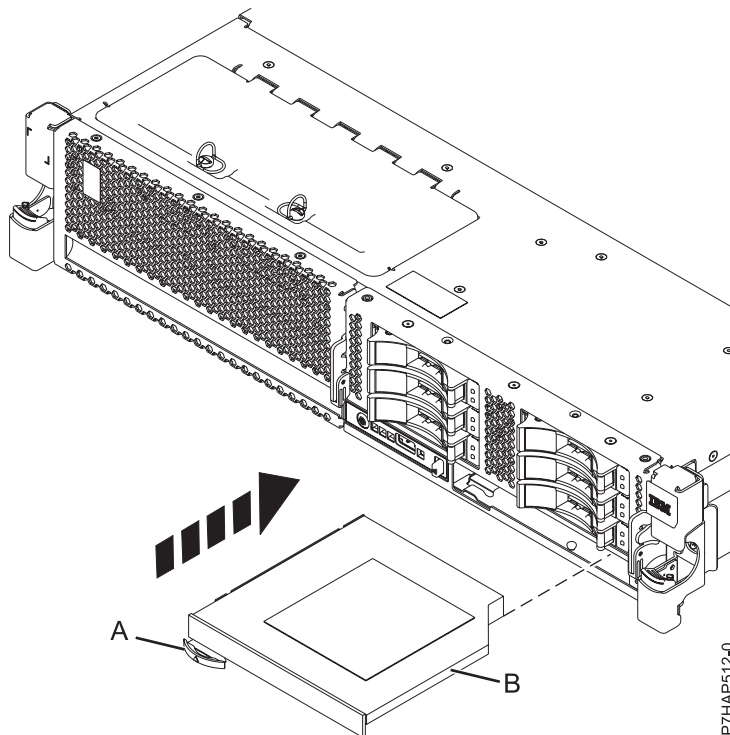
Figura 15. Instalar un dispositivo de soporte extraplano
