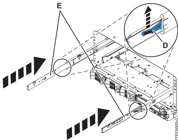
Figura 31. Desbloqueo los pestillos de seguridad de los rieles
