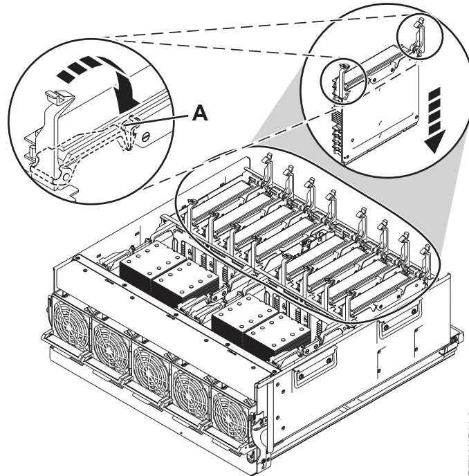
Figura 24. Sustitución de una tarjeta de memoria
