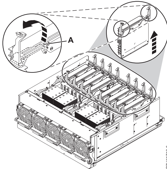
Figura 12. Extracción de la tarjeta de expansión de memoria
