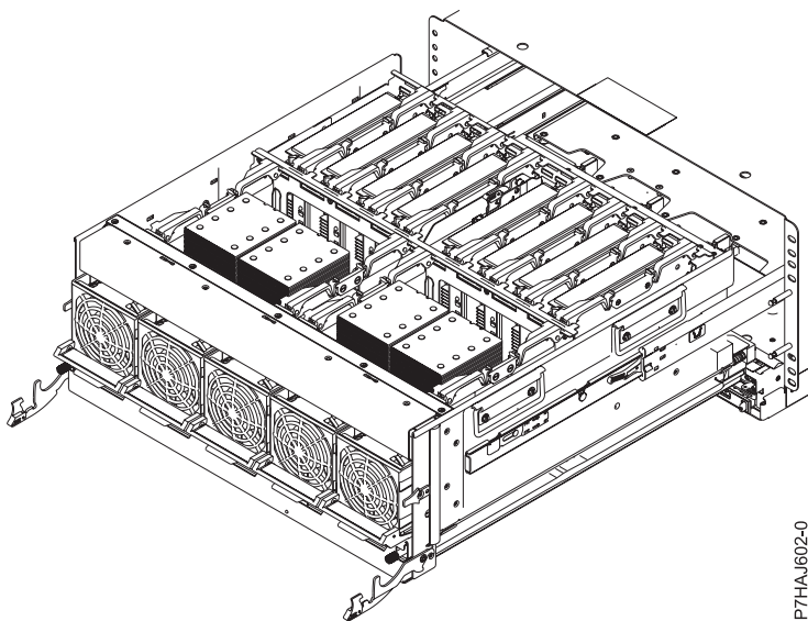
Figura 30. Sistema en la posición de servicio
