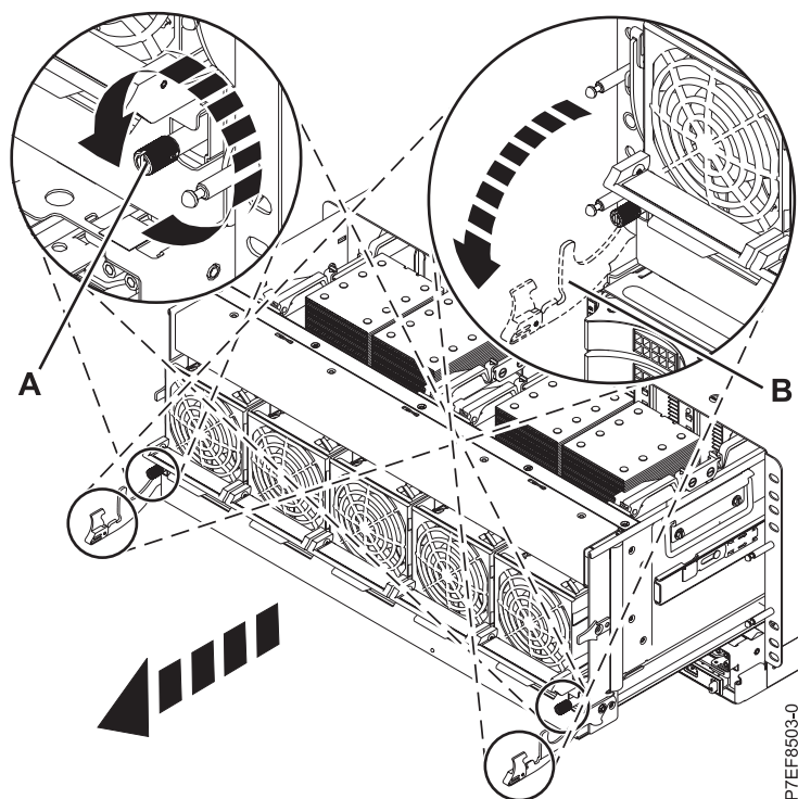
Figura 29. Soltar los pestillos laterales
