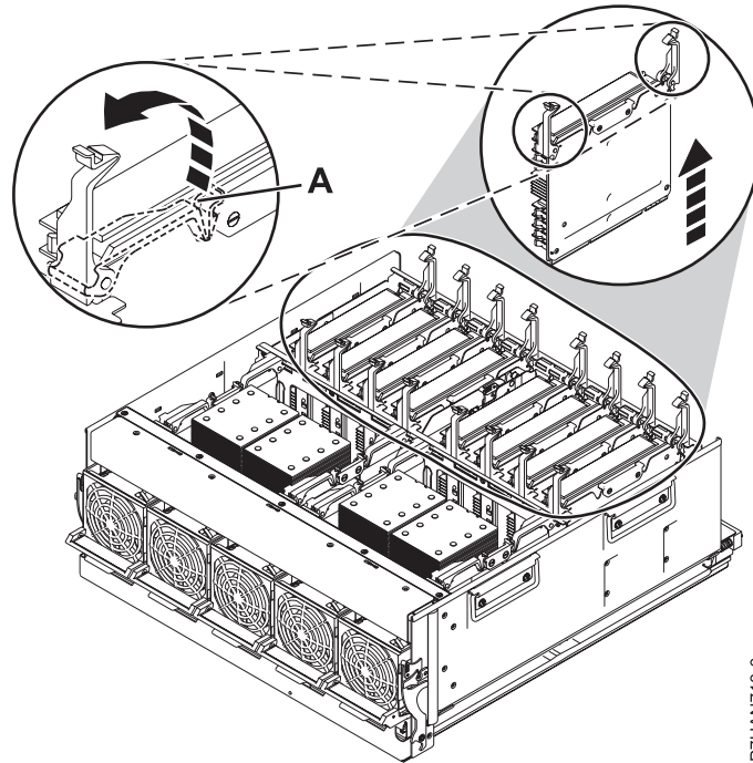
Figura 18. Extracción de una tarjeta de expansión de memoria
