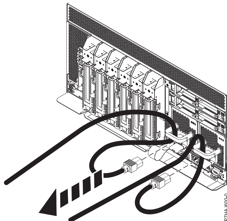
Figura 4. Desconectar los cables de alimentación
