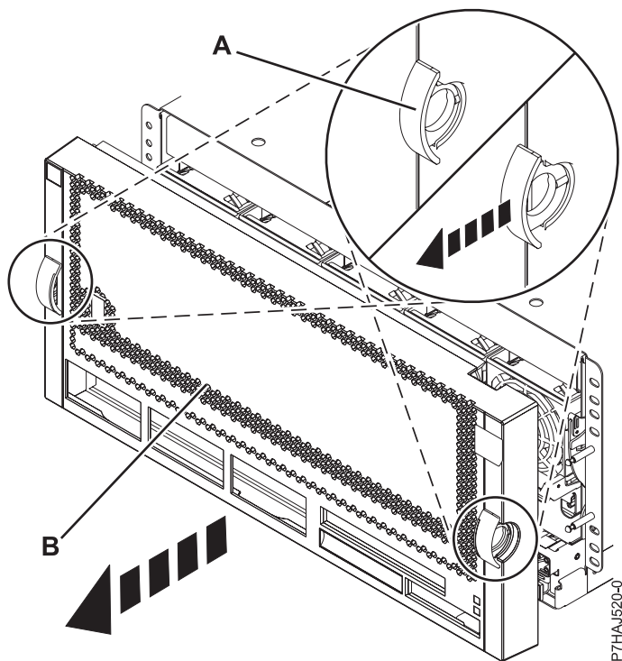
Figura 27. Quitar la cubierta frontal
