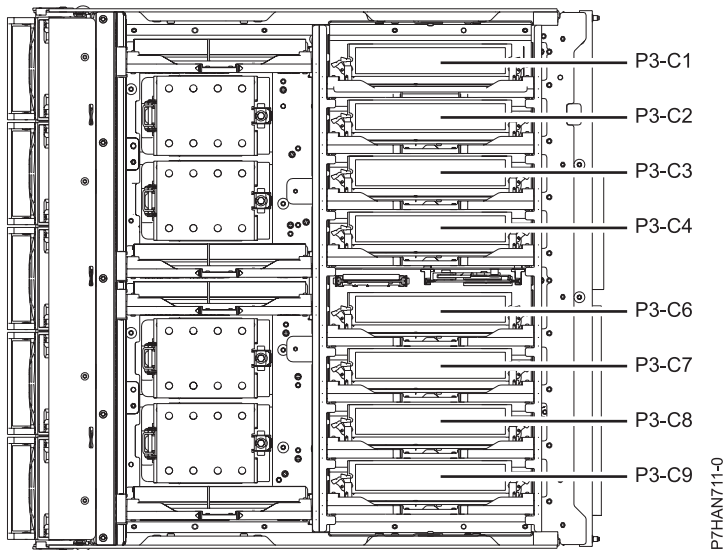
Figura 14. Secuencia de conexión de la tarjeta de expansión de memoria
