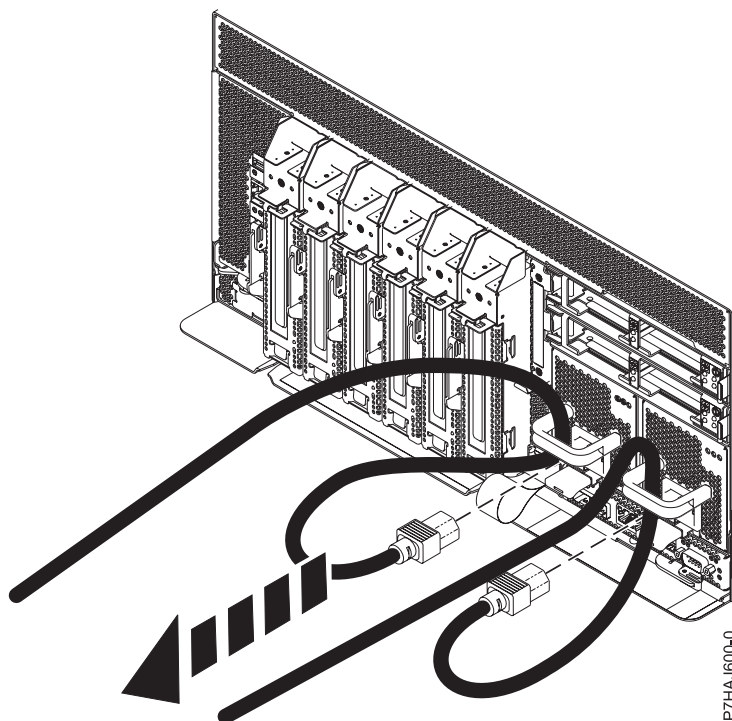
Figura 16. Desconectar los cables de alimentación
