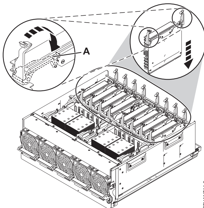
Figura 3. Instalación de una tarjeta de memoria
