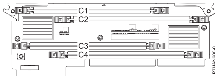
Figura 7. Ubicaciones de las ranuras de módulos de memoria
