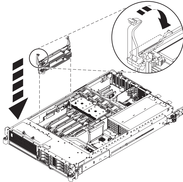
Figura 1. Instalación de una tarjeta de memoria
