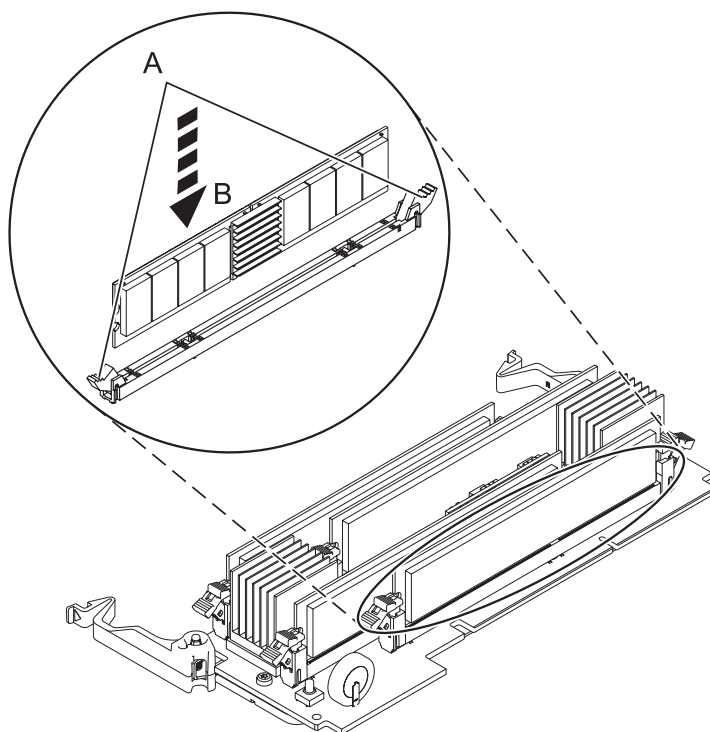
Figura 5. Instalación de un módulo de memoria
