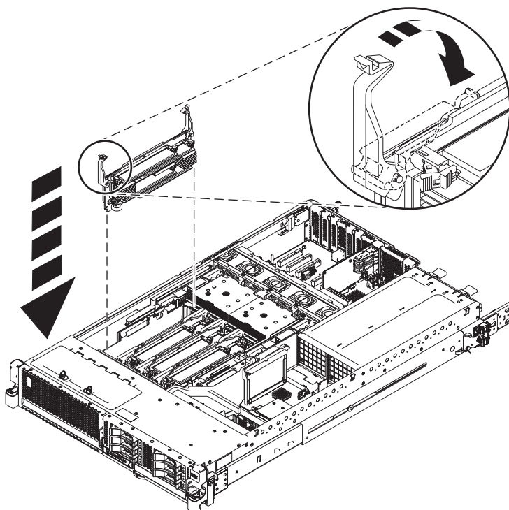
Figura 3. Sustitución de una tarjeta de memoria
