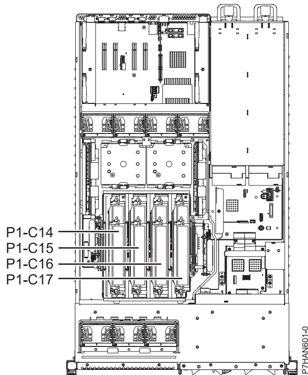
Figura 6. Secuencia de conexión de la tarjeta de expansión de memoria
