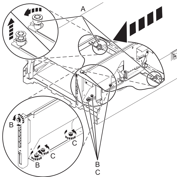
Figura 89. Extraer la tarjeta de conducto SAS y la pieza central
