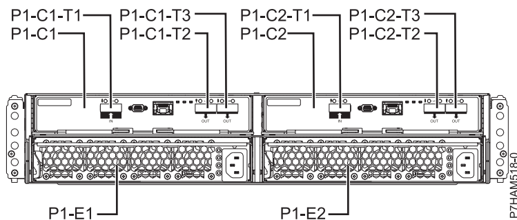
Figura 58. Vista posterior de Alojamiento de unidad de disco 5887
