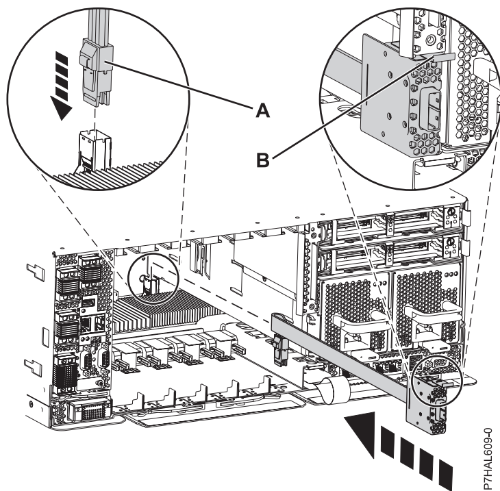
Figura 52. Instalación del puerto SAS externo
