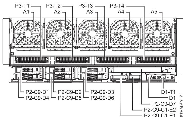
Figura 54. Ubicaciones de las unidades de disco
