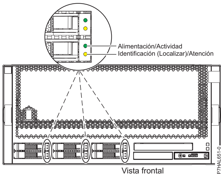
Figura 56. Indicadores de servicio de la unidad de disco para el sistema
