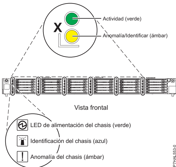
Figura 68. Vista frontal de Alojamiento de almacenamiento PCIe de EDR1 que muestra los indicadores de servicio
