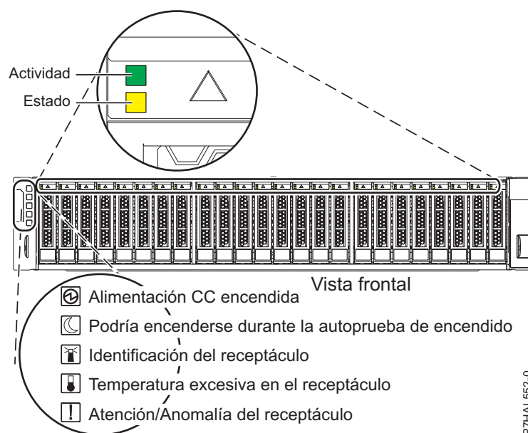
Figura 59. Vista frontal de Alojamiento de unidad de disco 5887 que muestra los indicadores de servicio
