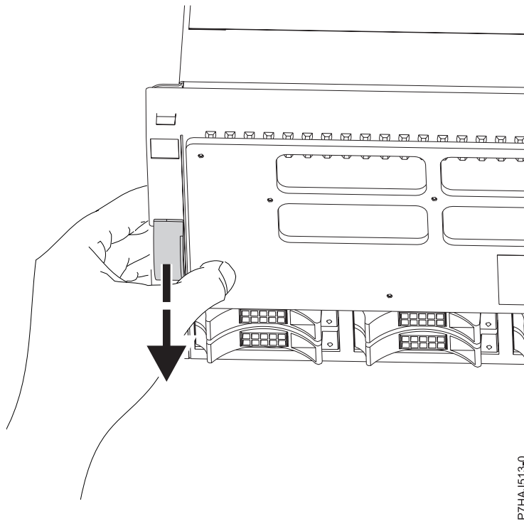
Figura 100. Soltar los pestillos de la cubierta
