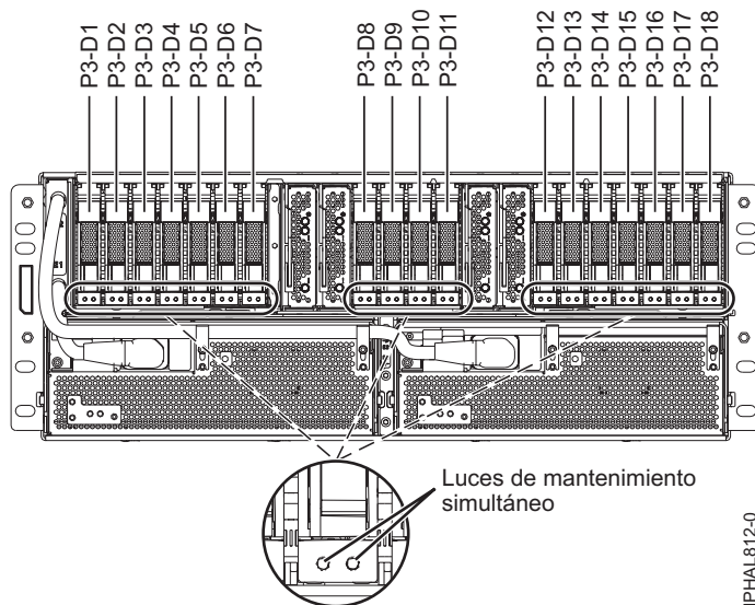
Figura 66. Ubicaciones de las unidades de disco
