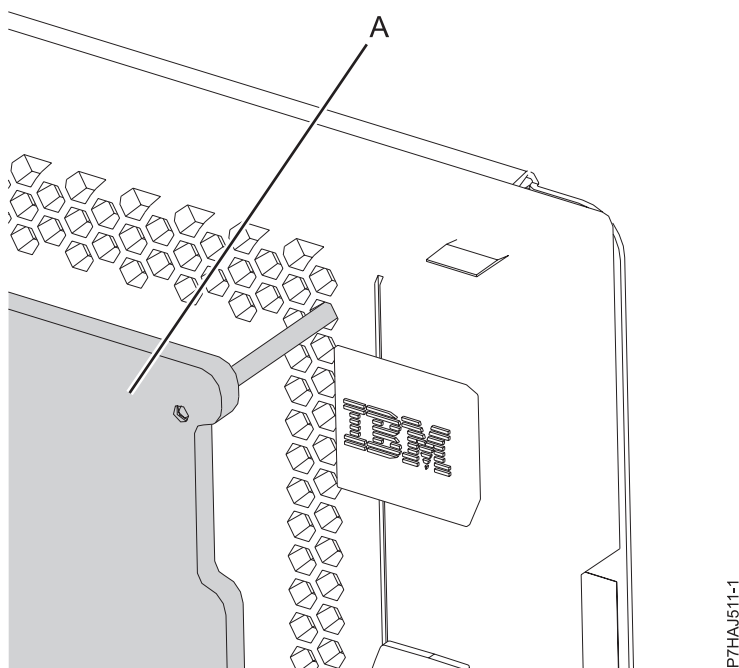
Figura 98. Alineación de la herramienta de extracción de la cubierta
