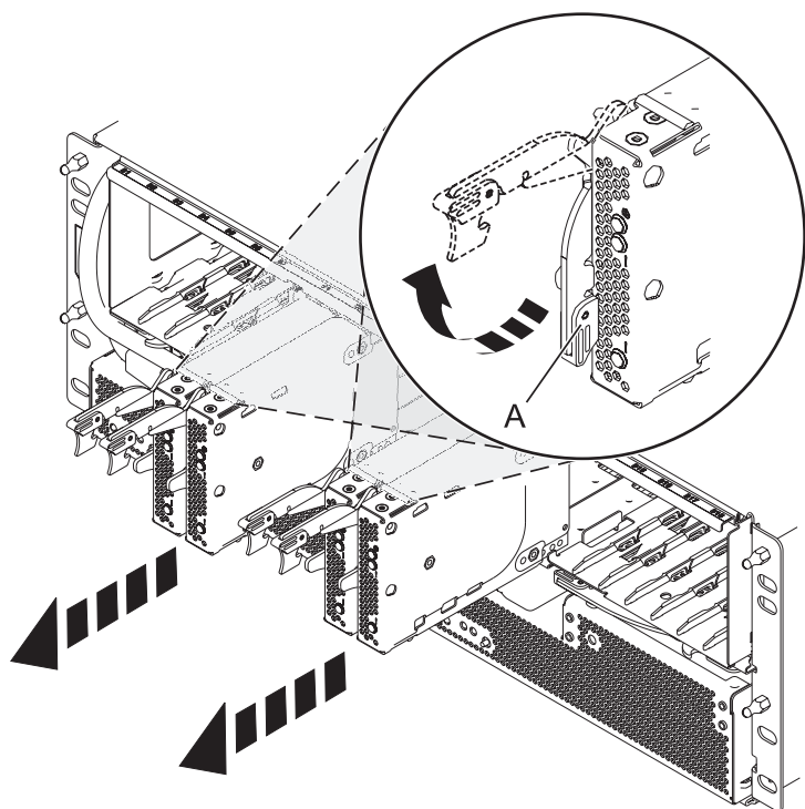
Figura 92. Quitar la tarjeta de expansión SAS.
