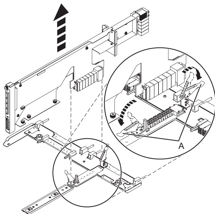
Figura 90. Extraer la tarjeta de conducto SAS de la pieza central
