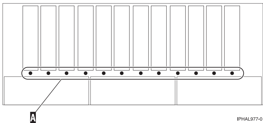
Figura 64. Vista frontal de los indicadores de servicio para 5786, 5787, 7031-D24 y 7031-T24
