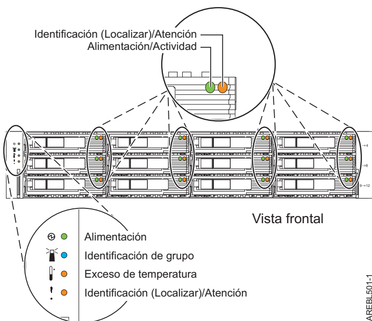
Figura 61. Vista frontal de los indicadores de servicio del alojamiento de unidades de disco para 5886
