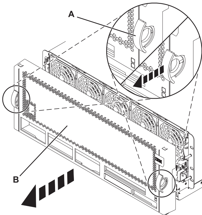
Figura 96. Extracción de la cubierta frontal
