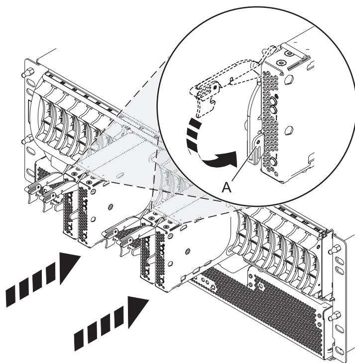
Figura 91. Instalación de la tarjeta de expansión de SAS
