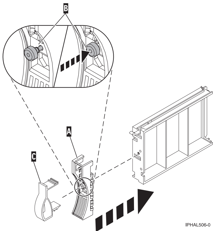
Figura 47. Instalación de una placa frontal en el panel de relleno de una unidad de disco
