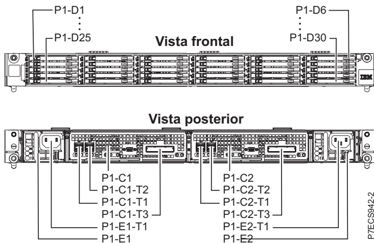
Figura 67. Vistas frontal y posterior de Alojamiento de almacenamiento PCIe de EDR1 que muestran las ubicaciones de las unidades de estado sólido
