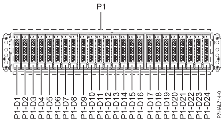
Figura 57. Vista frontal de Alojamiento de unidad de disco 5887 que muestra las ubicaciones de las unidades de disco.
