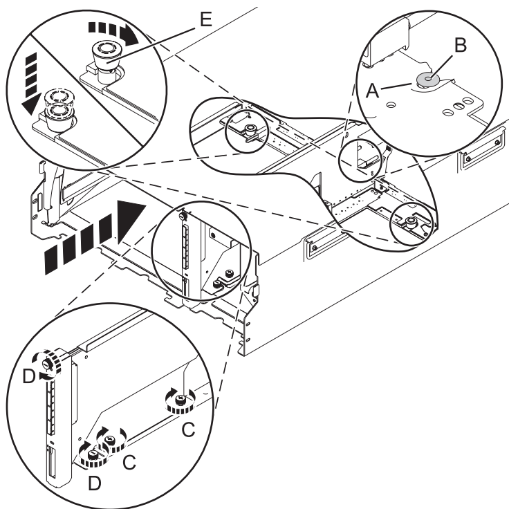
Figura 75. Instalar la tarjeta de conducto SAS y la placa central
