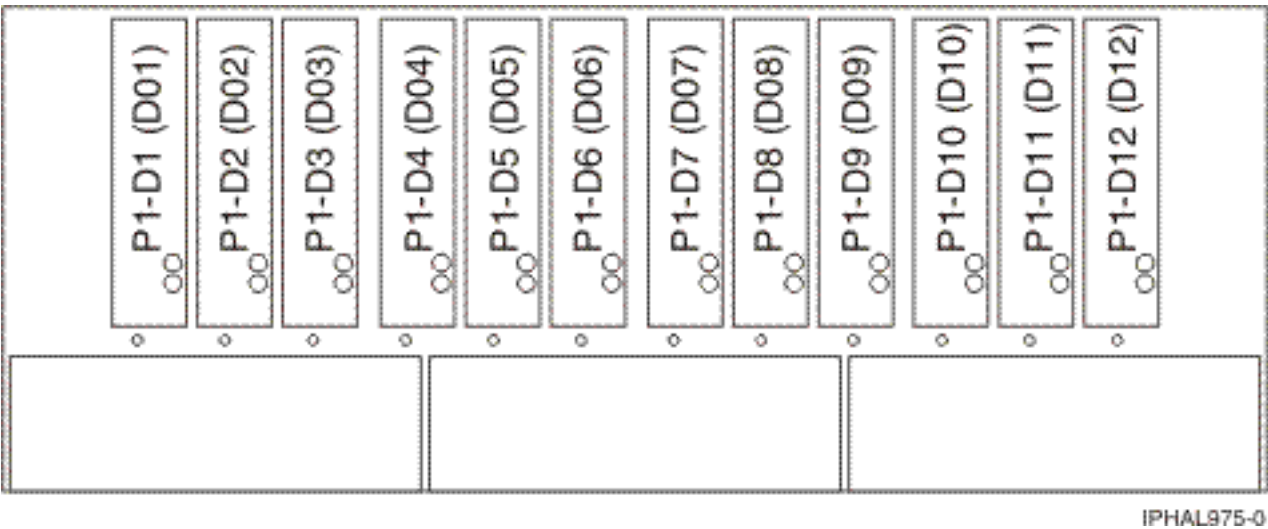
Figura 62. Vista frontal de los alojamientos de las unidades de discos SCSI 5786, 5787, 7031-D24 y 7031-T24
