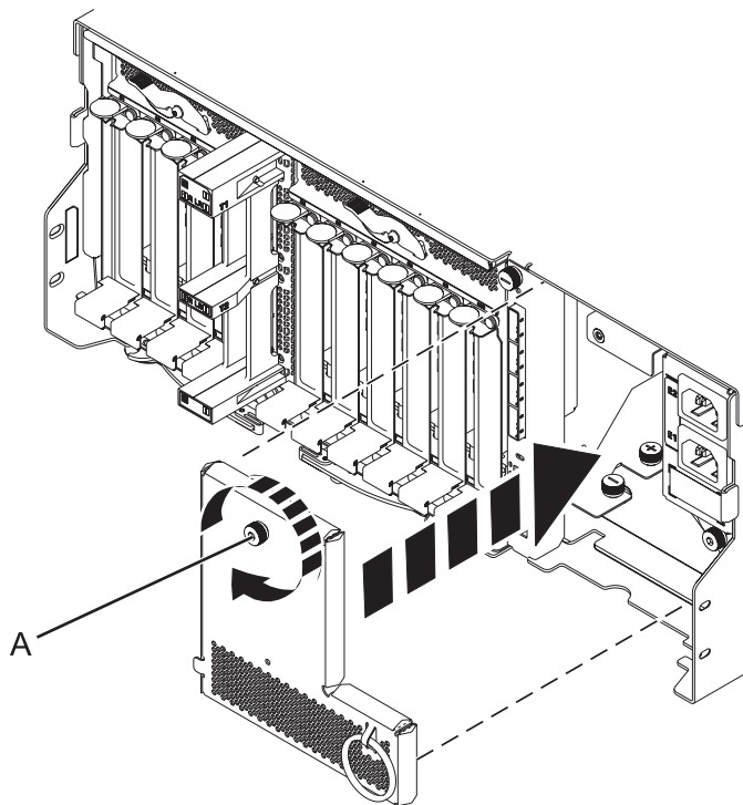
Figura 76. Instalación de la placa del cable de corriente
