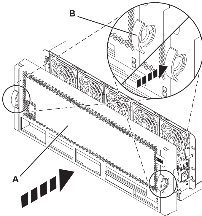
Figura 103. Instalación de la cubierta frontal
