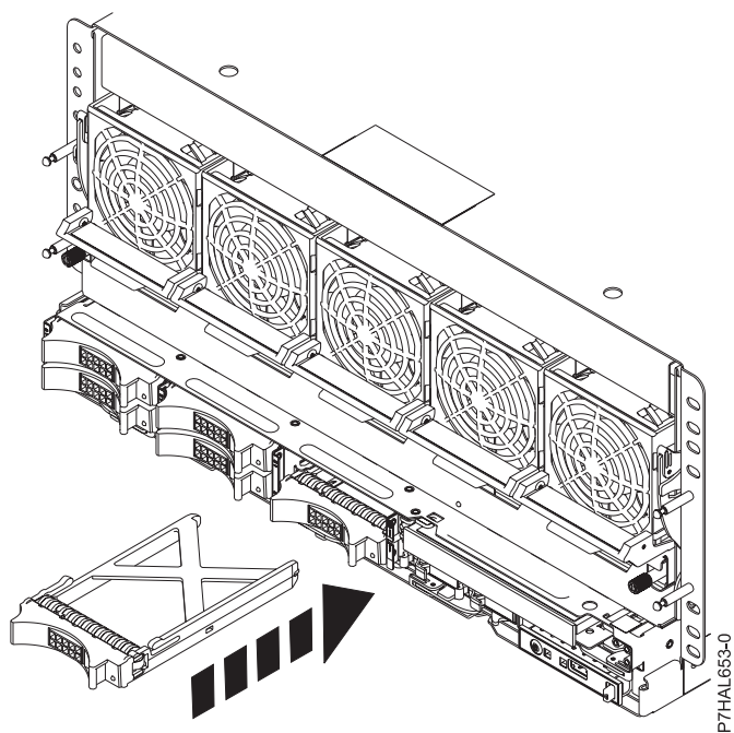
Figura 48. Instalación de un panel de relleno de unidad de disco
