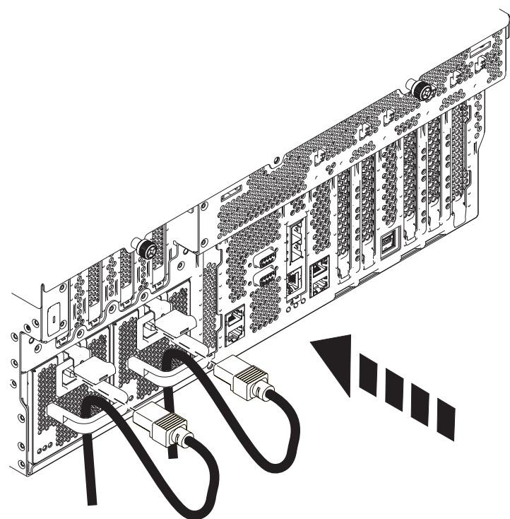
Figura 127. Conectar los cables de alimentación
