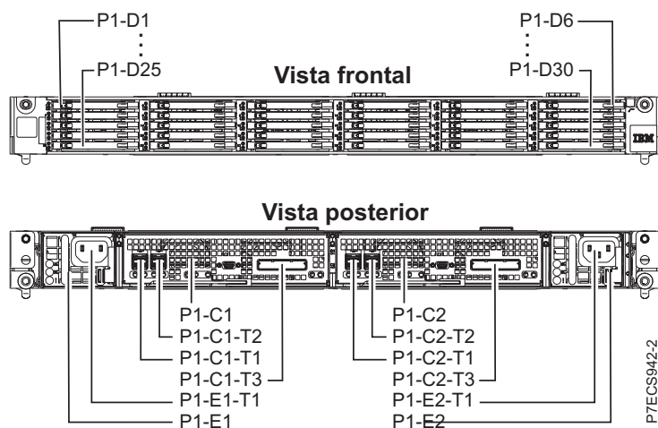
Figura 78. Vistas frontal y posterior de Alojamiento de almacenamiento 5888 PCIe que muestran las ubicaciones de las unidades de estado sólido
