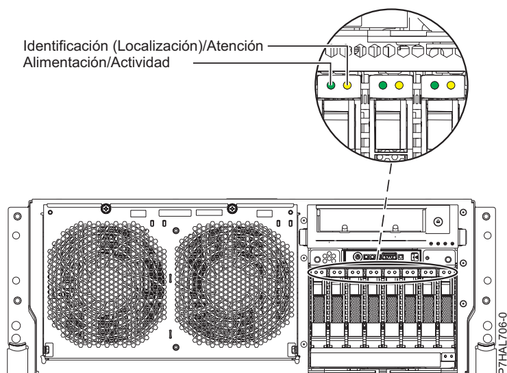
Figura 66. Ubicaciones de los indicadores de servicio para los sistemas montados en un bastidor
