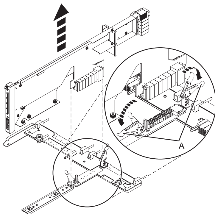
Figura 103. Extraer la tarjeta de conducto SAS de la pieza central
