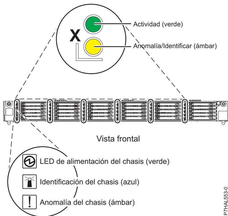
Figura 81. Vista frontal de Alojamiento de almacenamiento PCIe de EDR1 que muestra los indicadores de servicio
