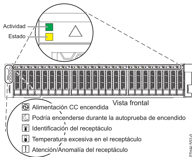
Figura 77. Vista frontal de Alojamiento de unidad de disco 5887 que muestra los indicadores de servicio
