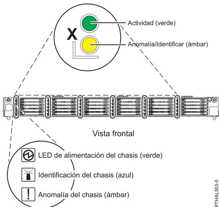
Figura 79. Vista frontal de Alojamiento de almacenamiento 5888 PCIe que muestra los indicadores de servicio
