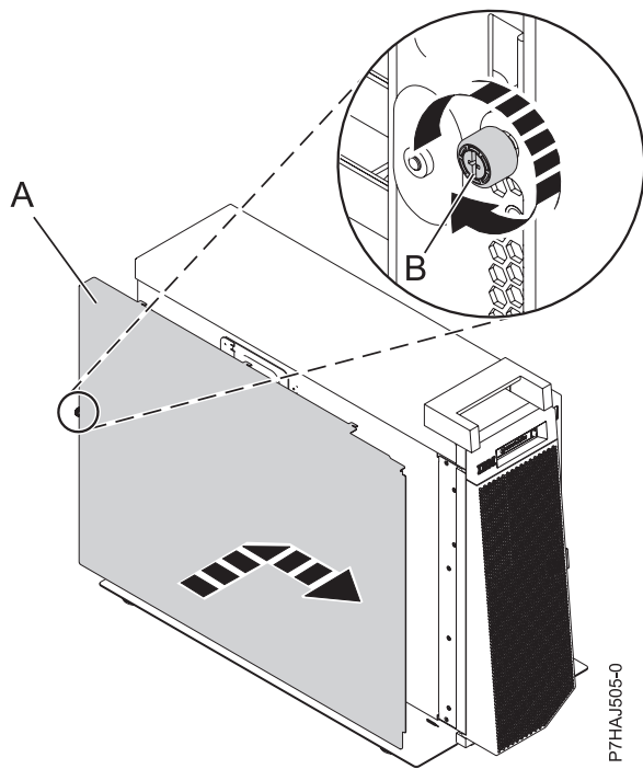
Figura 120. Instalar la cubierta de acceso de servicio exterior
