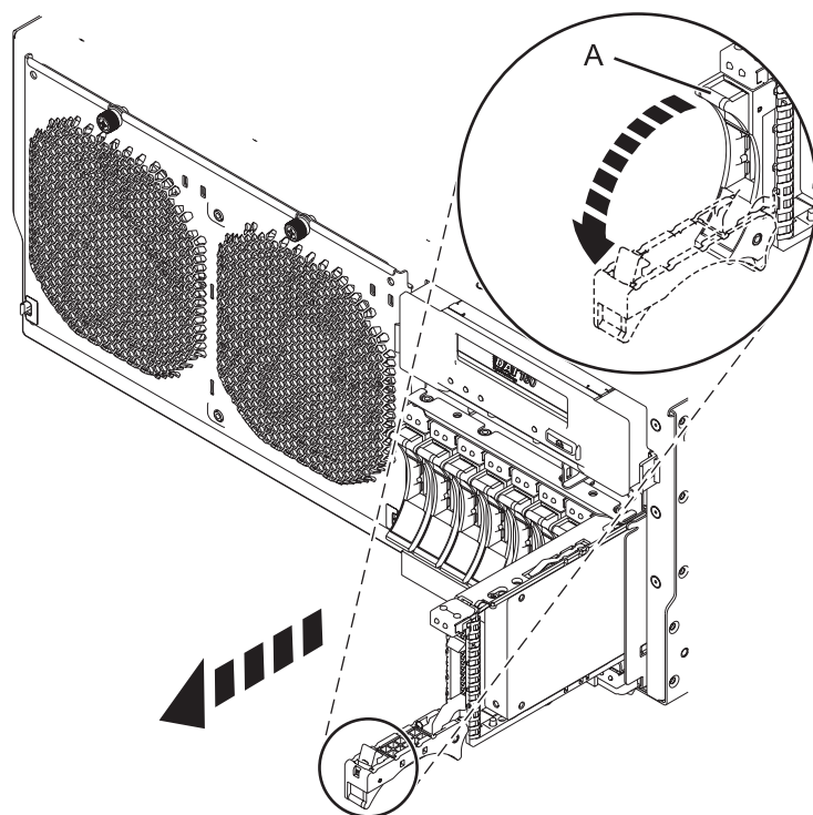
Figura 20. Extracción de una unidad de disco del sistema
