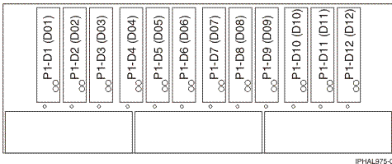
Figura 69. Vista frontal de los alojamientos de las unidades de discos SCSI 5786, 5787, 7031-D24 y 7031-T24
