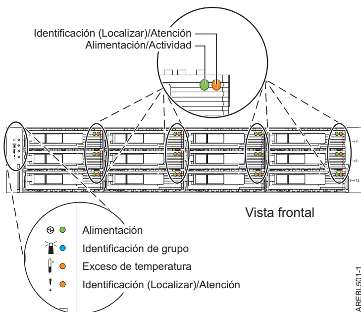
Figura 74. Vista frontal de los indicadores de servicio del alojamiento de unidades de disco para 5886
