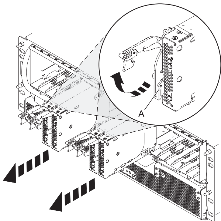
Figura 105. Quitar la tarjeta de expansión SAS.
