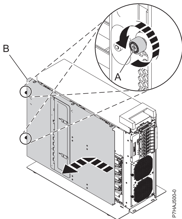
Figura 117. Extracción de la cubierta de acceso de servicio interior
