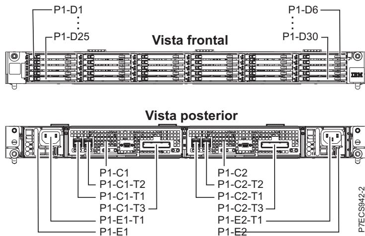
Figura 80. Vistas frontal y posterior de Alojamiento de almacenamiento PCIe de EDR1 que muestran las ubicaciones de las unidades de estado sólido
