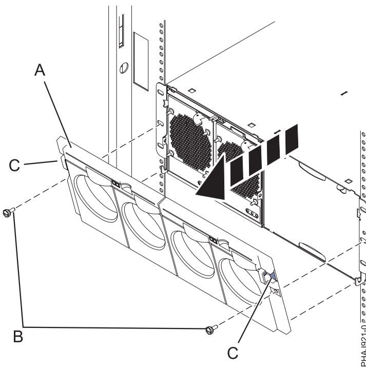
Figura 108. Extracción de la cubierta frontal para el modelo 7314-G30 o 5796
