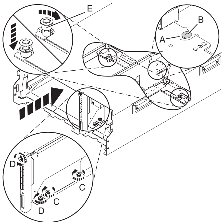
Figura 88. Instalar la tarjeta de conducto SAS y la placa central
