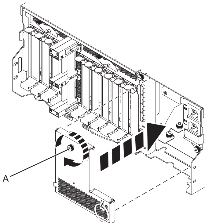
Figura 89. Instalación de la placa del cable de corriente
