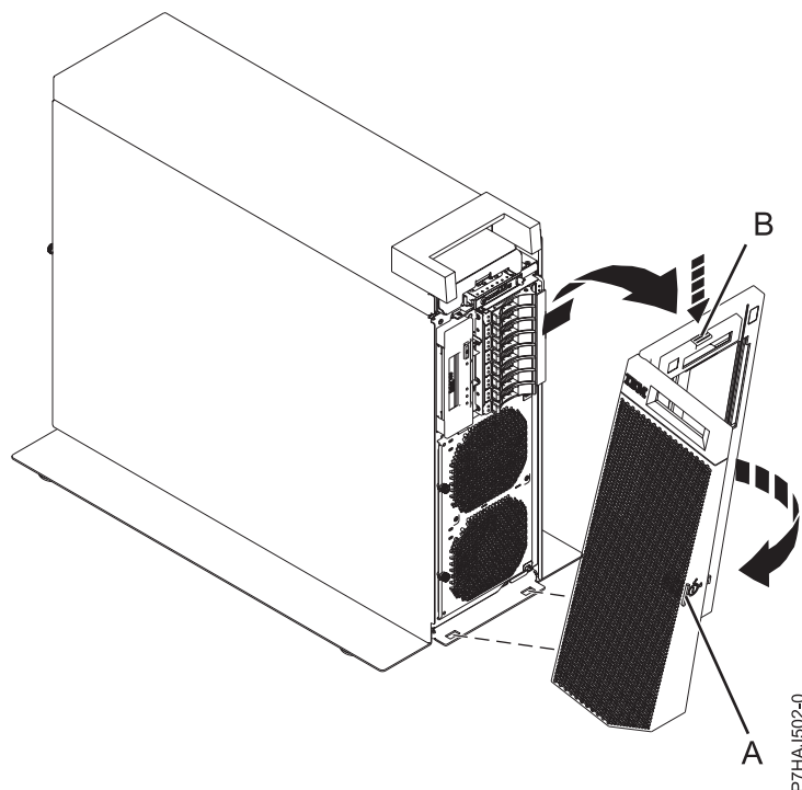
Figura 111. Extracción de la cubierta frontal
