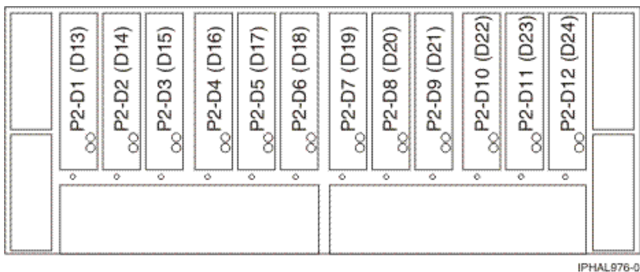
Figura 70. Vista posterior de los alojamientos de las unidades de discos SCSI 5786, 5787, 7031-D24 y 7031-T24
