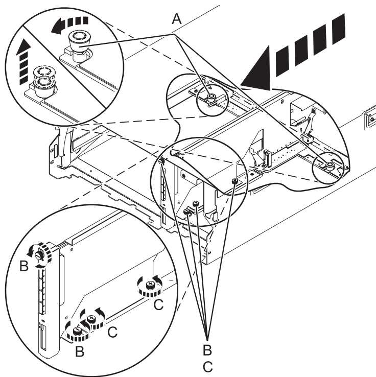
Figura 102. Extraer la tarjeta de conducto SAS y la pieza central
