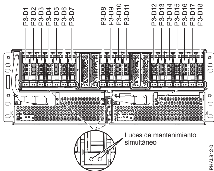
Figura 68. Ubicaciones de las unidades de disco
