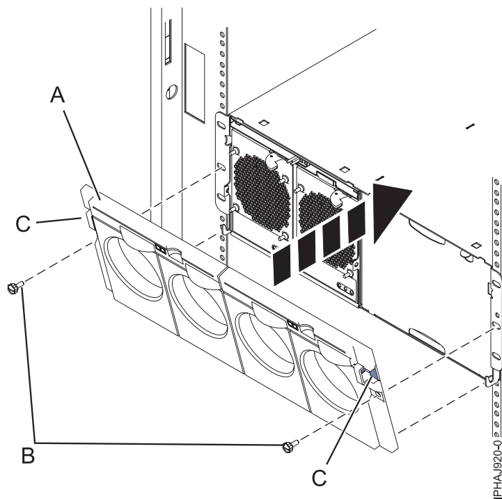
Figura 109. Cubierta frontal de un modelo 7314-G30 o 5796
