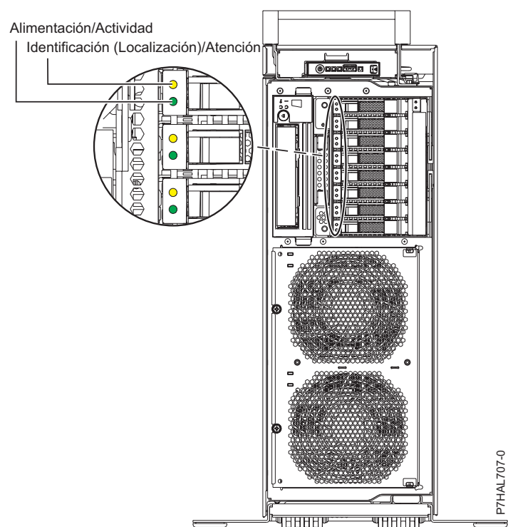
Figura 67. Ubicaciones de los indicadores de servicio para el sistema autónomo
