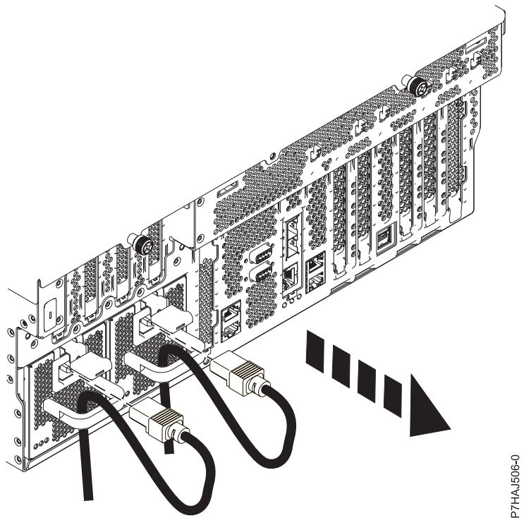
Figura 125. Quitar los cables de alimentación de un sistema montado en bastidor
