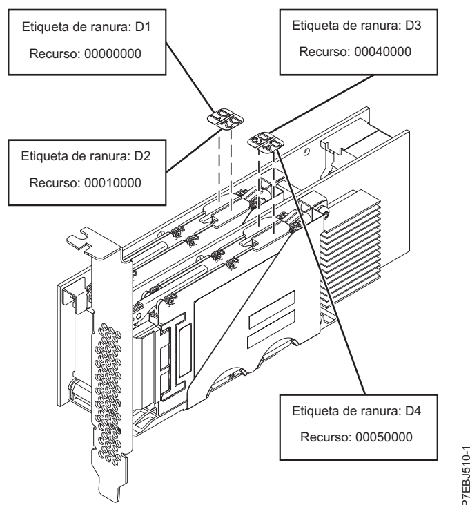
Figura 63. Ubicaciones del adaptador PCIe RAID y SSD SAS
