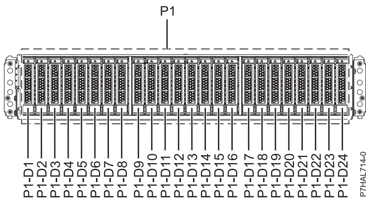
Figura 75. Vista frontal de Alojamiento de unidad de disco 5887 que muestra las ubicaciones de las unidades de disco.
