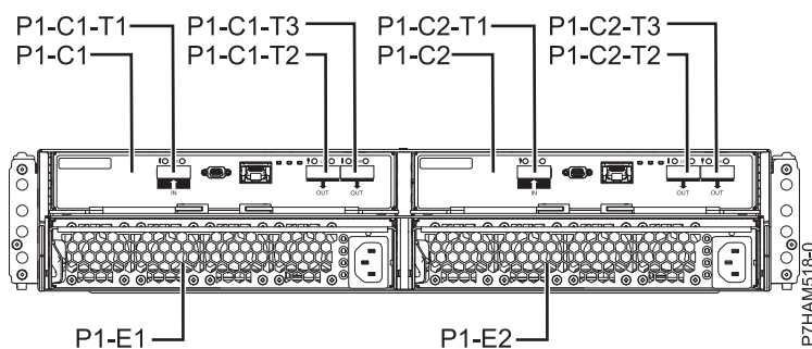
Figura 76. Vista posterior de Alojamiento de unidad de disco 5887
