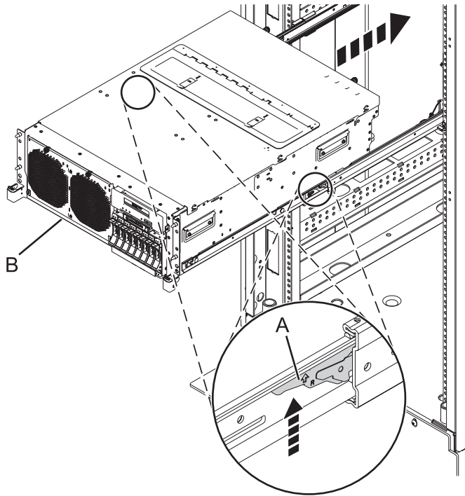
Figura 123. Colocación del sistema en posición operativa
