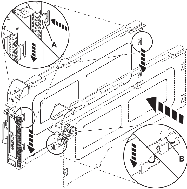
Figura 23. Cubierta que se ha sustituido de la casete de adaptador PCI
