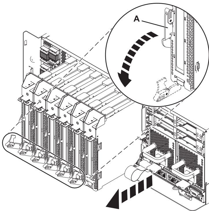
Figura 12. Extracción de una casete de adaptador PCI del sistema
