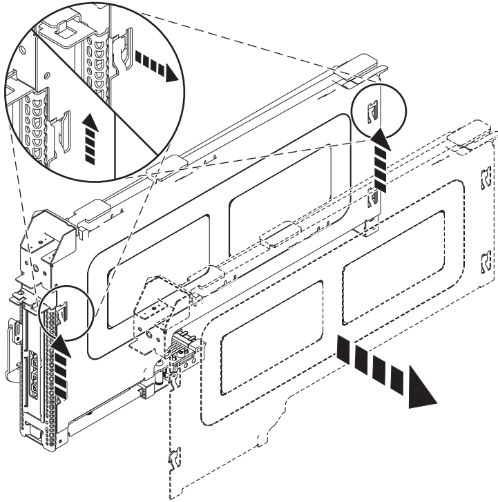
Figura 26. Se ha quitado la cubierta de la casete del adaptador PCI
