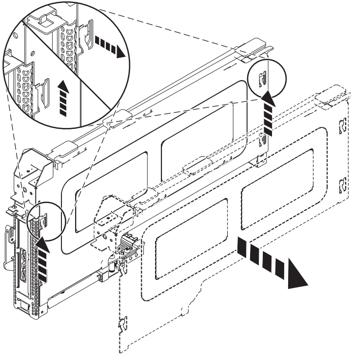
Figura 21. Se ha quitado la cubierta de la casete del adaptador PCI
