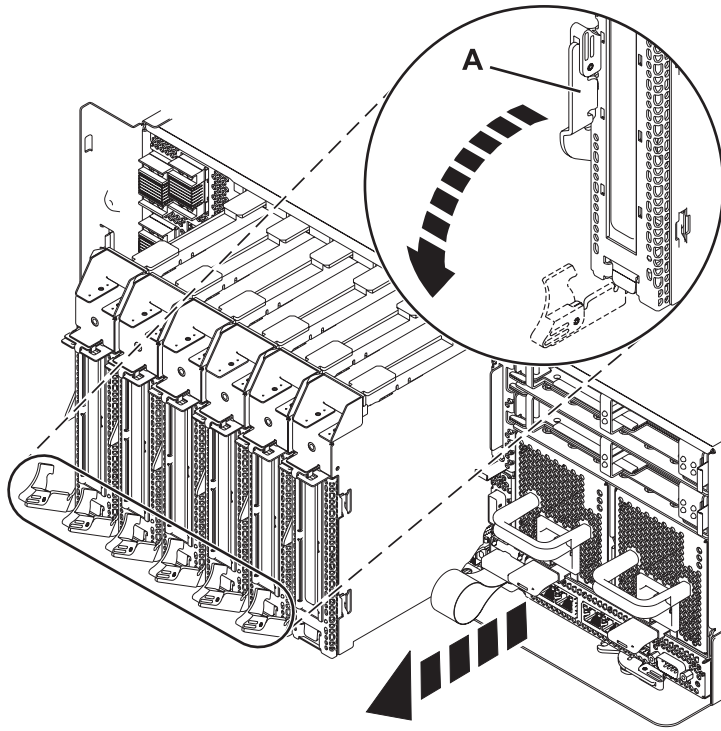
Figura 11. Extracción de una casete de adaptador PCI del sistema
