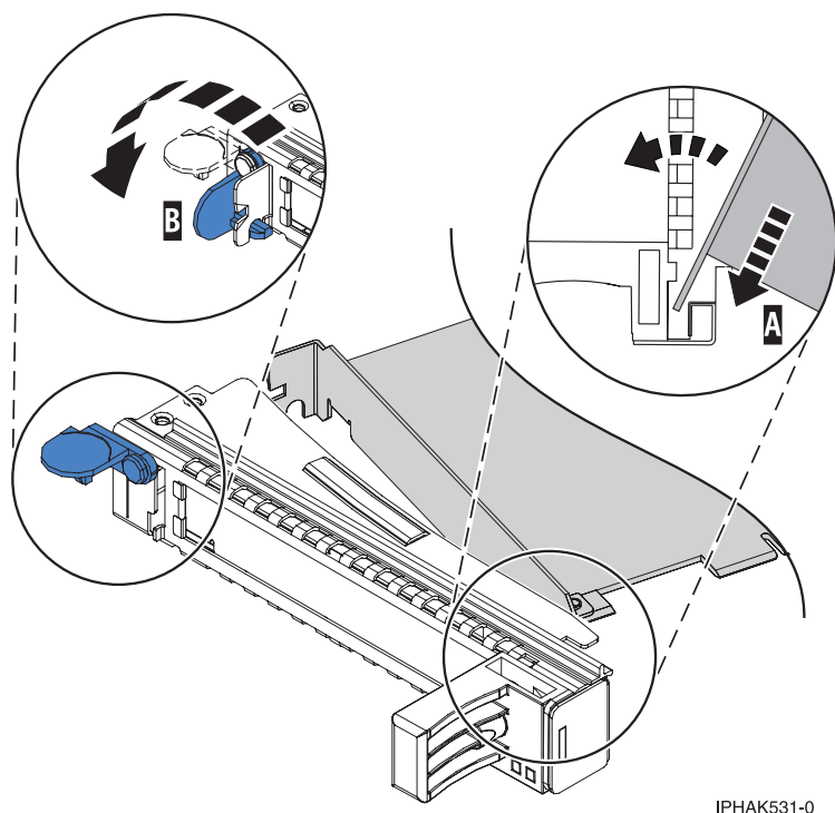
Figura 40. Adaptador que se ha quitado de la casete de adaptador PCI de anchura simple
