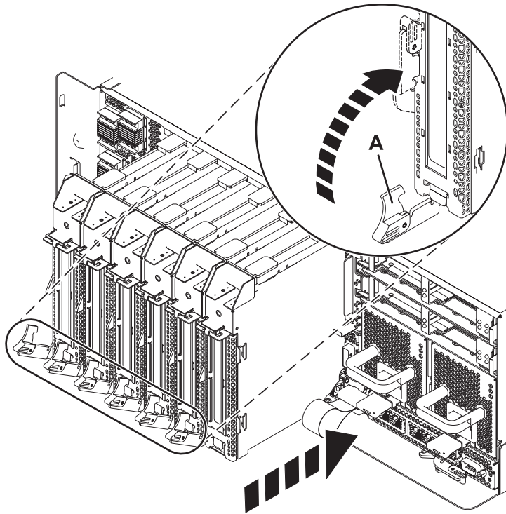
Figura 7. Instalación de la casete de adaptador PCI en el sistema
