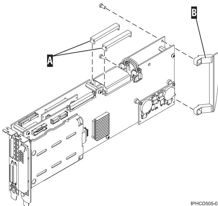
Figura 56. Preparación del adaptador para la colocación en una casete
