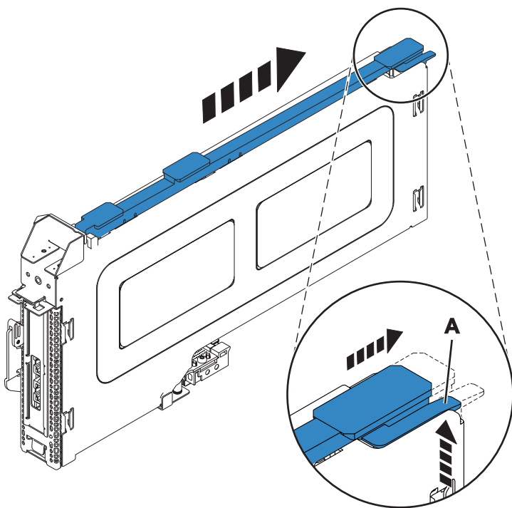
Figura 25. Se ha quitado el riel de guía de la casete de adaptador PCI
