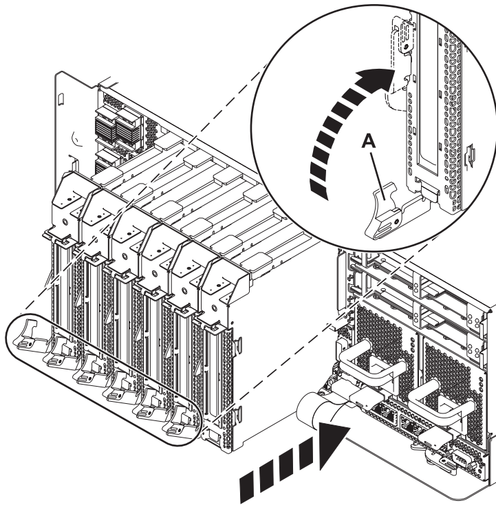
Figura 18. Instalación de una casete de adaptador PCI en el sistema
