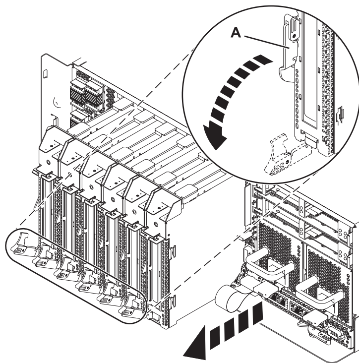
Figura 16. Extracción de una casete de adaptador PCI del sistema
