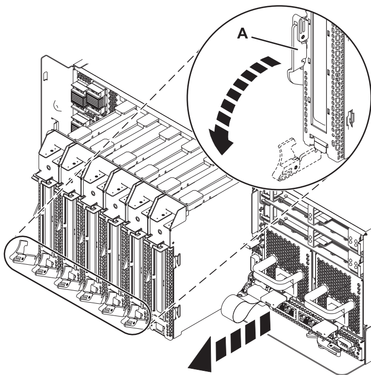
Figura 13. Extracción de una casete de adaptador PCI del sistema
