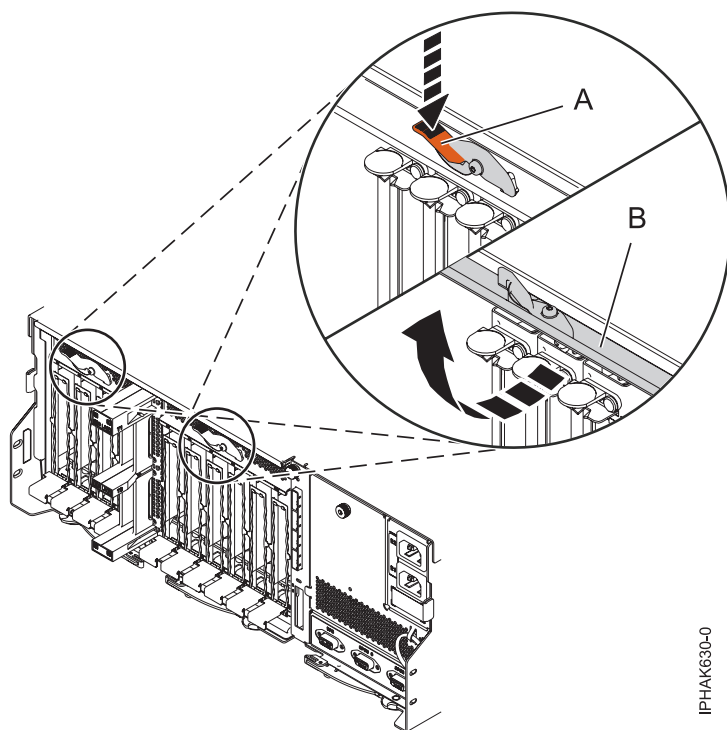
Figura 32. Apertura de la puerta de acceso
