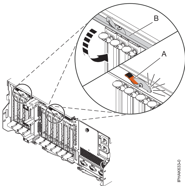
Figura 31. Cierre de la puerta de acceso
