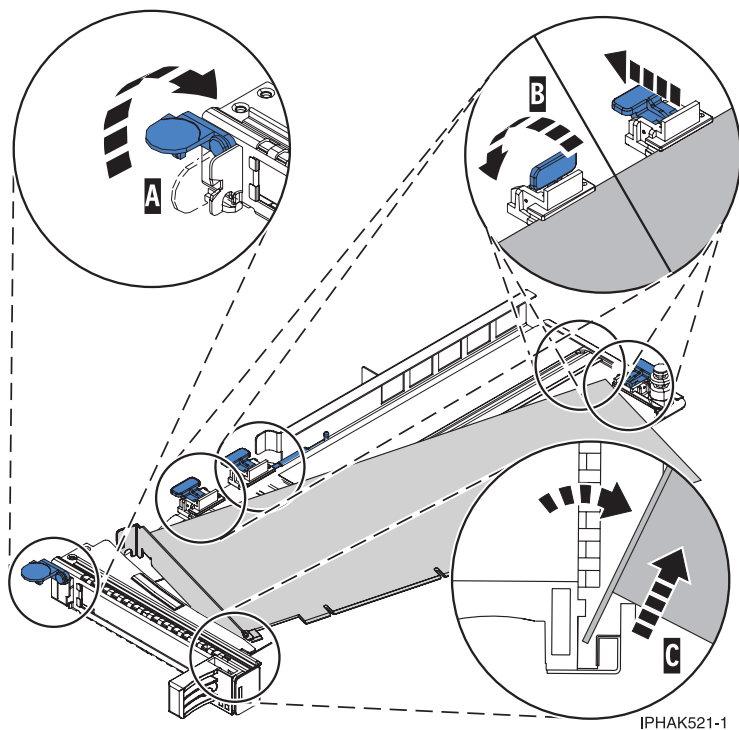
Figura 35. Adaptador que se ha quitado de la casete de adaptadores PCI
