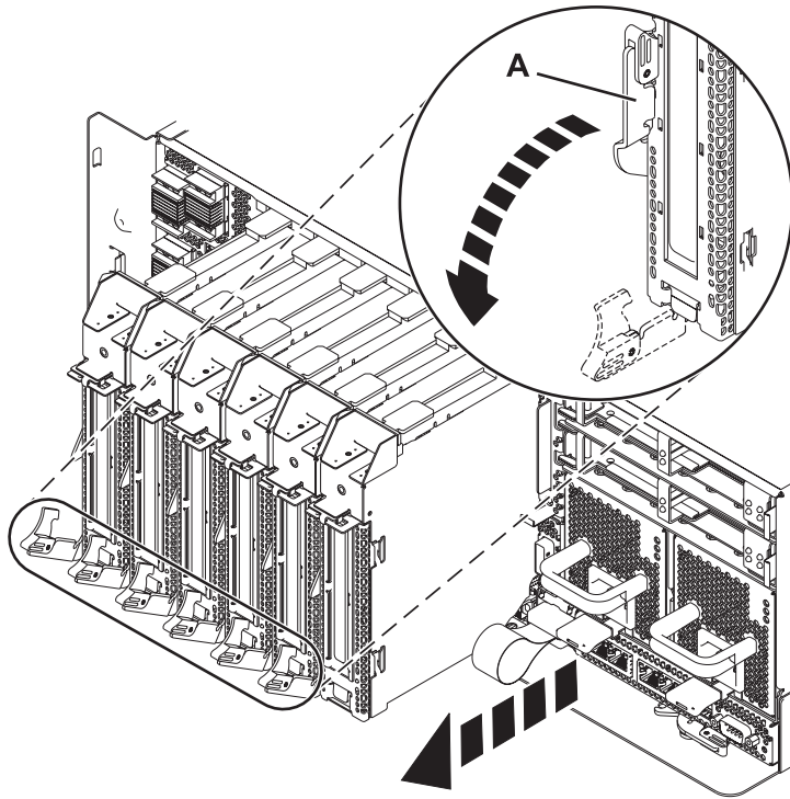
Figura 8. Extracción de una casete de adaptador PCI de la unidad del sistema
