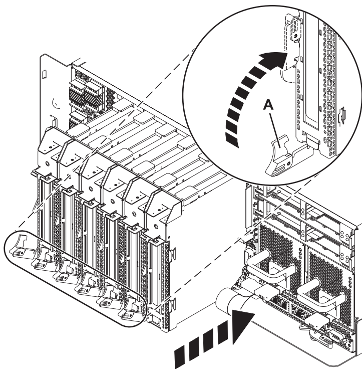
Figura 19. Instalación de una casete de adaptador PCI en el sistema
