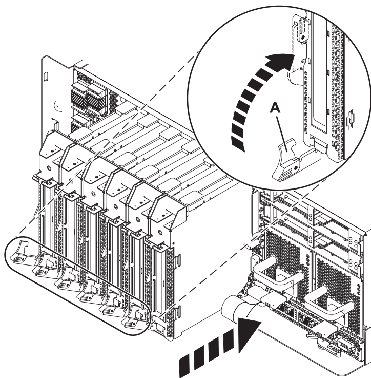
Figura 15. Instalación de una casete de adaptador PCI en el sistema
