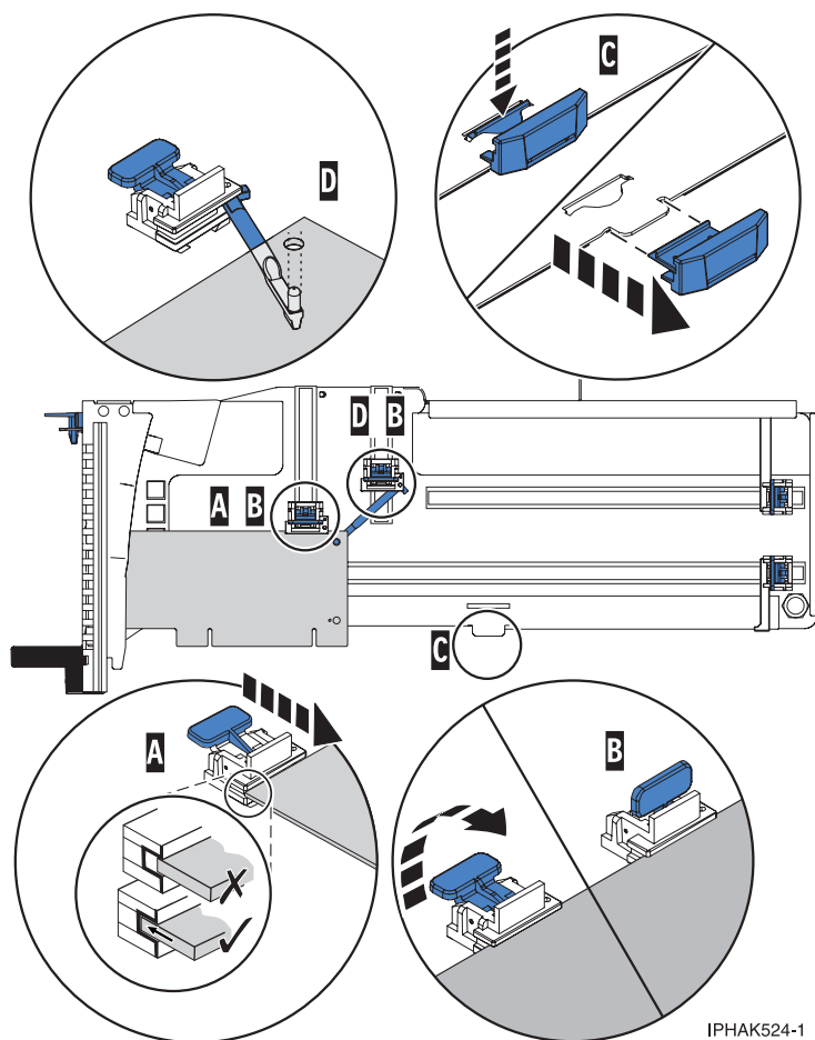
Figura 43. Adaptador pequeño en la casete de adaptador PCI con los soportes y el brazo de enganche en su sitio
