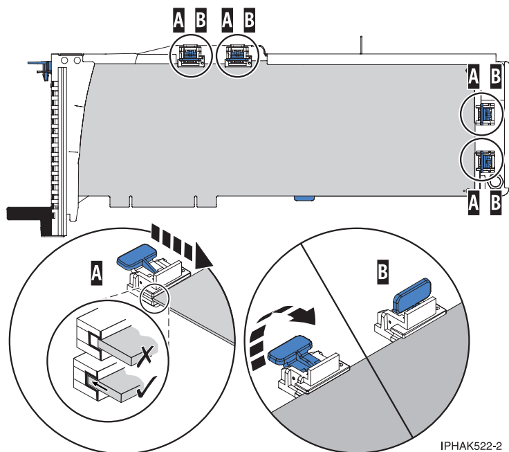
Figura 41. Adaptador grande en la casete de adaptador PCI con los soportes y el estabilizador en su sitio
