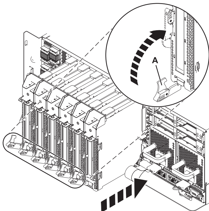
Figura 17. Instalación de una casete de adaptador PCI en el sistema
