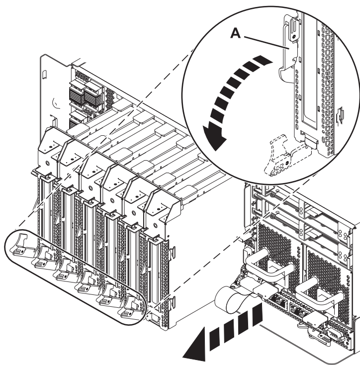
Figura 14. Extracción de una casete de adaptador PCI del sistema
