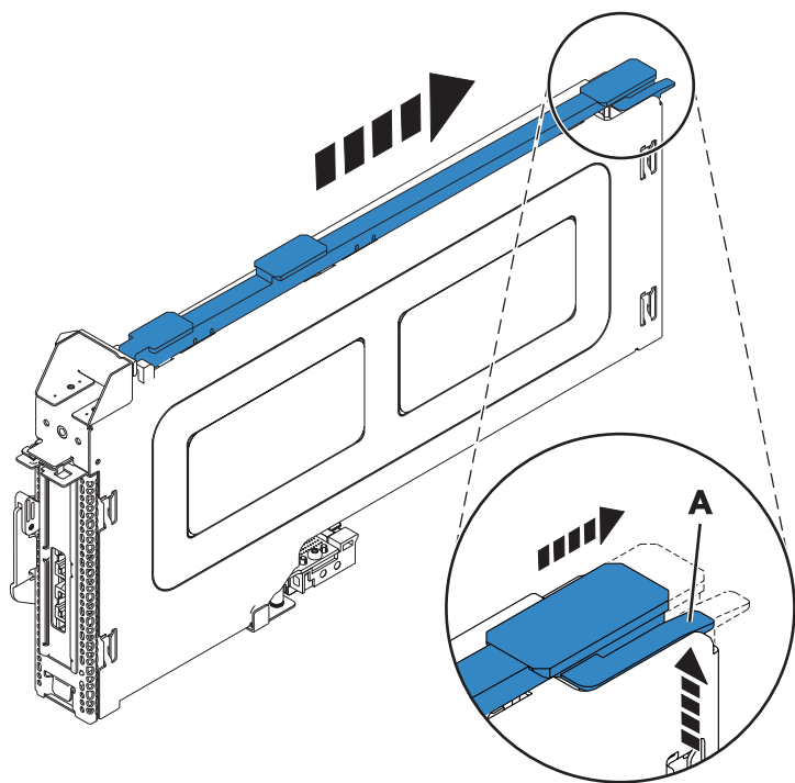
Figura 20. Se ha quitado el riel de guía de la casete de adaptador PCI
