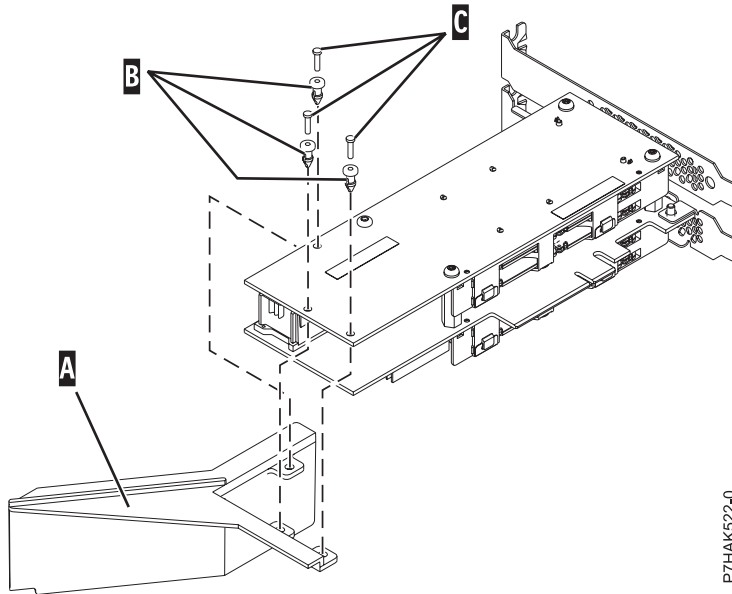
Figura 50. Instalación de un deflector de aire en el nuevo adaptador RAID PCIe y SAS SSD
