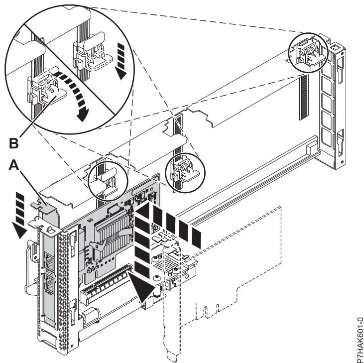
Figura 22. Adaptador instalado en la casete de adaptador PCI de anchura simple
