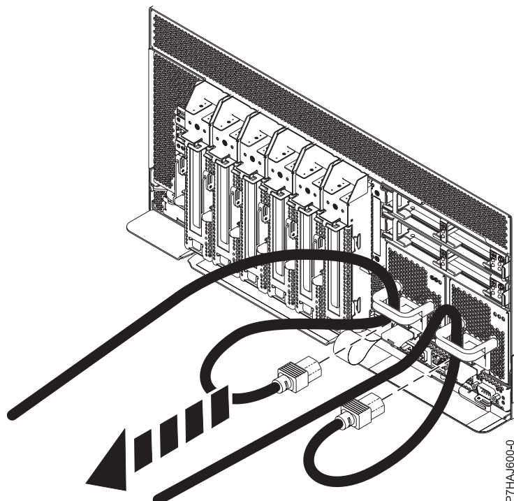
Figura 1. Desconexión de los cables de alimentación
