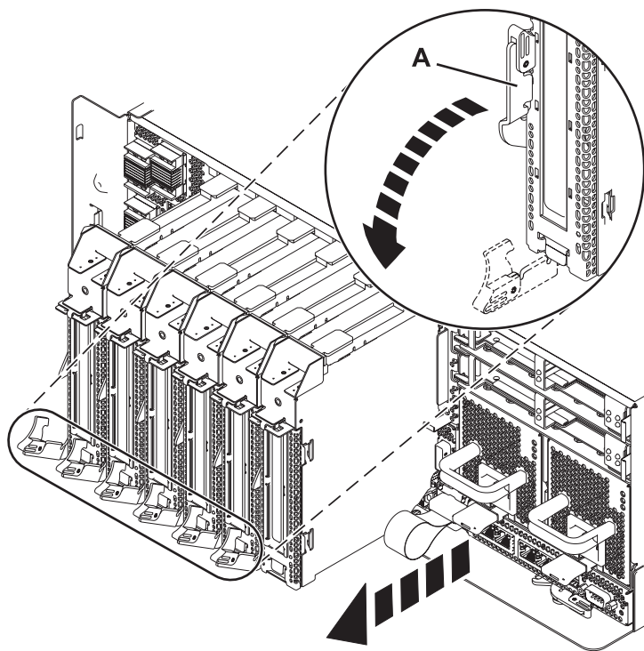
Figura 6. Extracción de la casete de adaptador PCI del sistema
