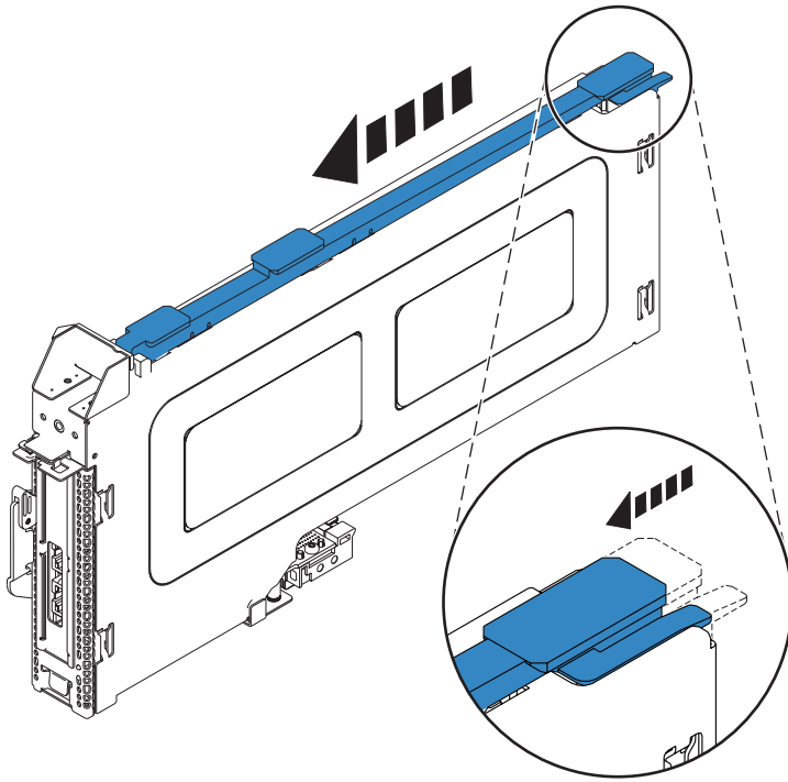
Figura 29. Se ha bloqueado el riel de guía de la casete de adaptador PCI
