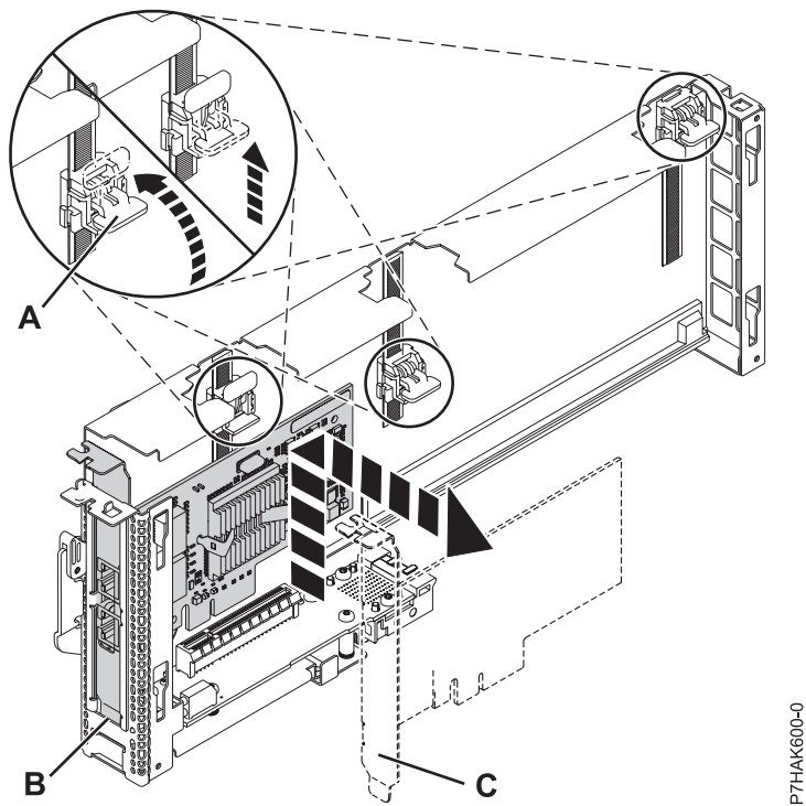
Figura 27. Adaptador que se ha quitado de la casete de adaptadores PCI
