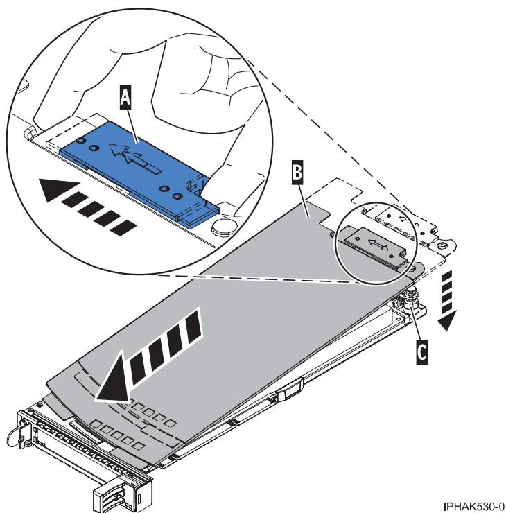
Figura 36. Cubierta que se ha sustituido de la casete de adaptador PCI
