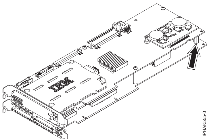
Figura 57. Quitar el elemento de separación
