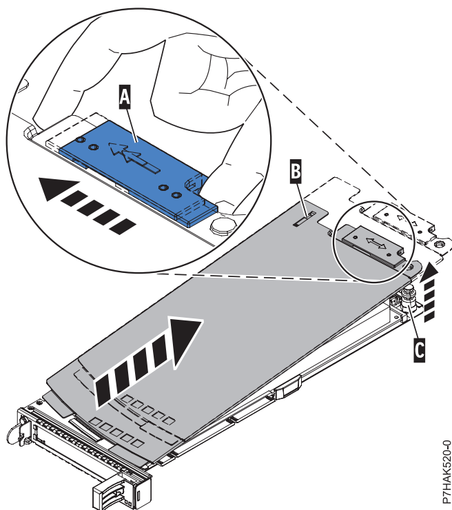
Figura 34. Se ha quitado la cubierta de la casete del adaptador PCI
