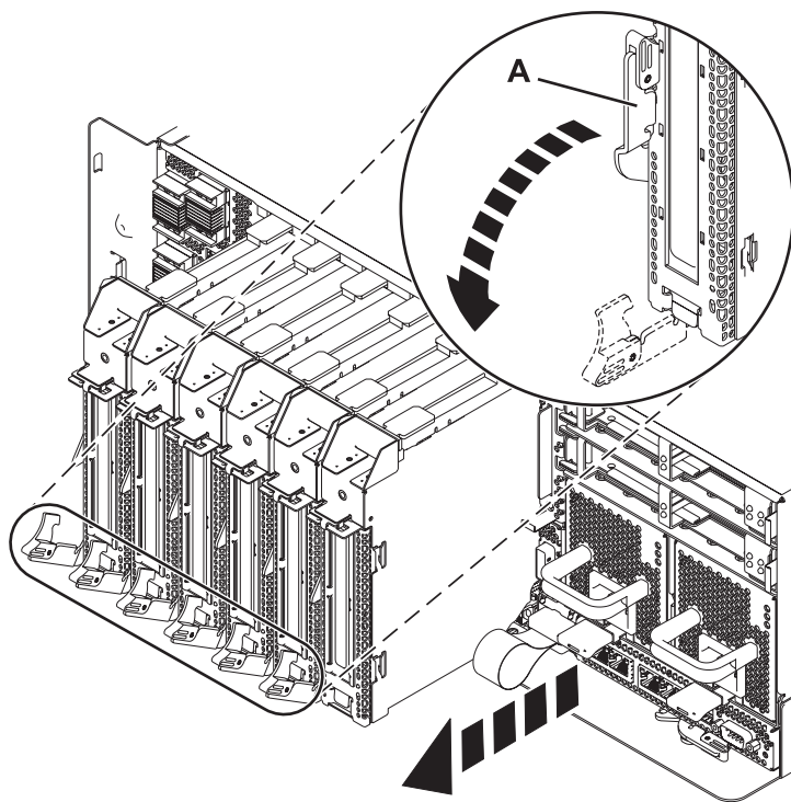
Figura 4. Extracción de la casete de adaptador PCI del sistema
