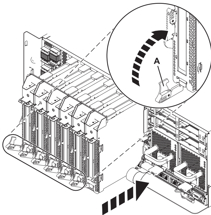
Figura 3. Instalación de una casete de adaptador PCI en el sistema
