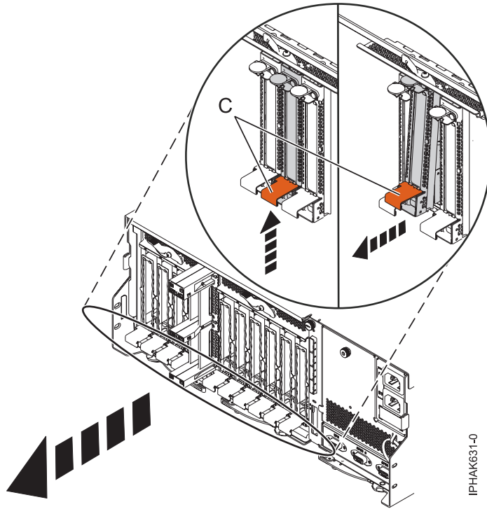
Figura 33. Extracción de una casete de adaptador PCI
