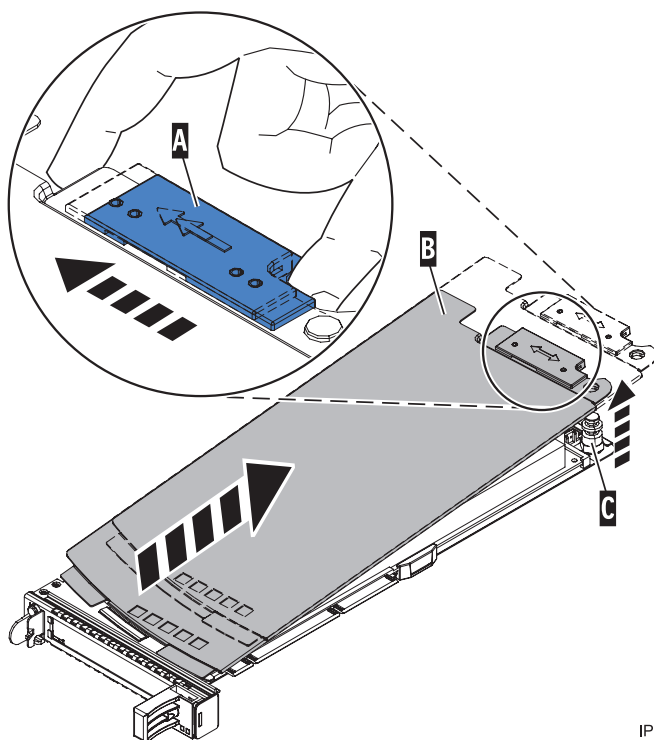
Figura 37. Cubierta que se ha quitado de la casete de adaptadores PCI de anchura simple
