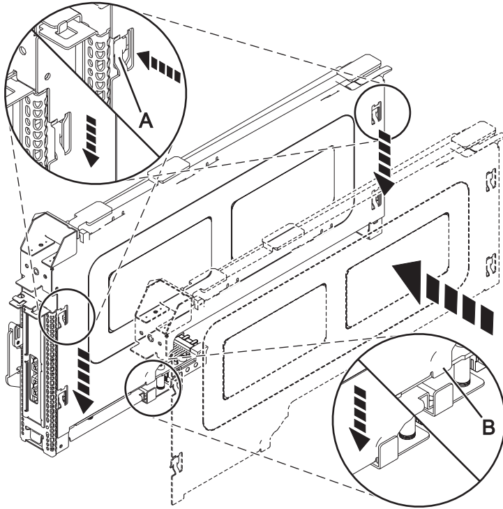
Figura 28. Cubierta que se ha sustituido de la casete de adaptador PCI
