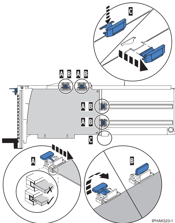
Figura 42. Adaptador de longitud mediana en la casete de adaptador PCI con los soportes en su sitio
