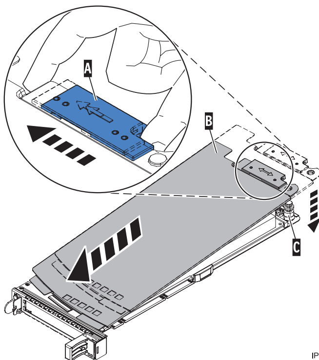
Figura 44. Cubierta que se ha sustituido de la casete de adaptador PCI
